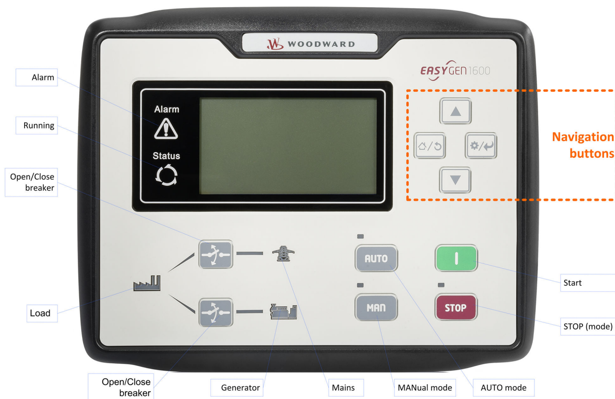
插图 2: HMI ( 前面板 ) easYgen-1600
