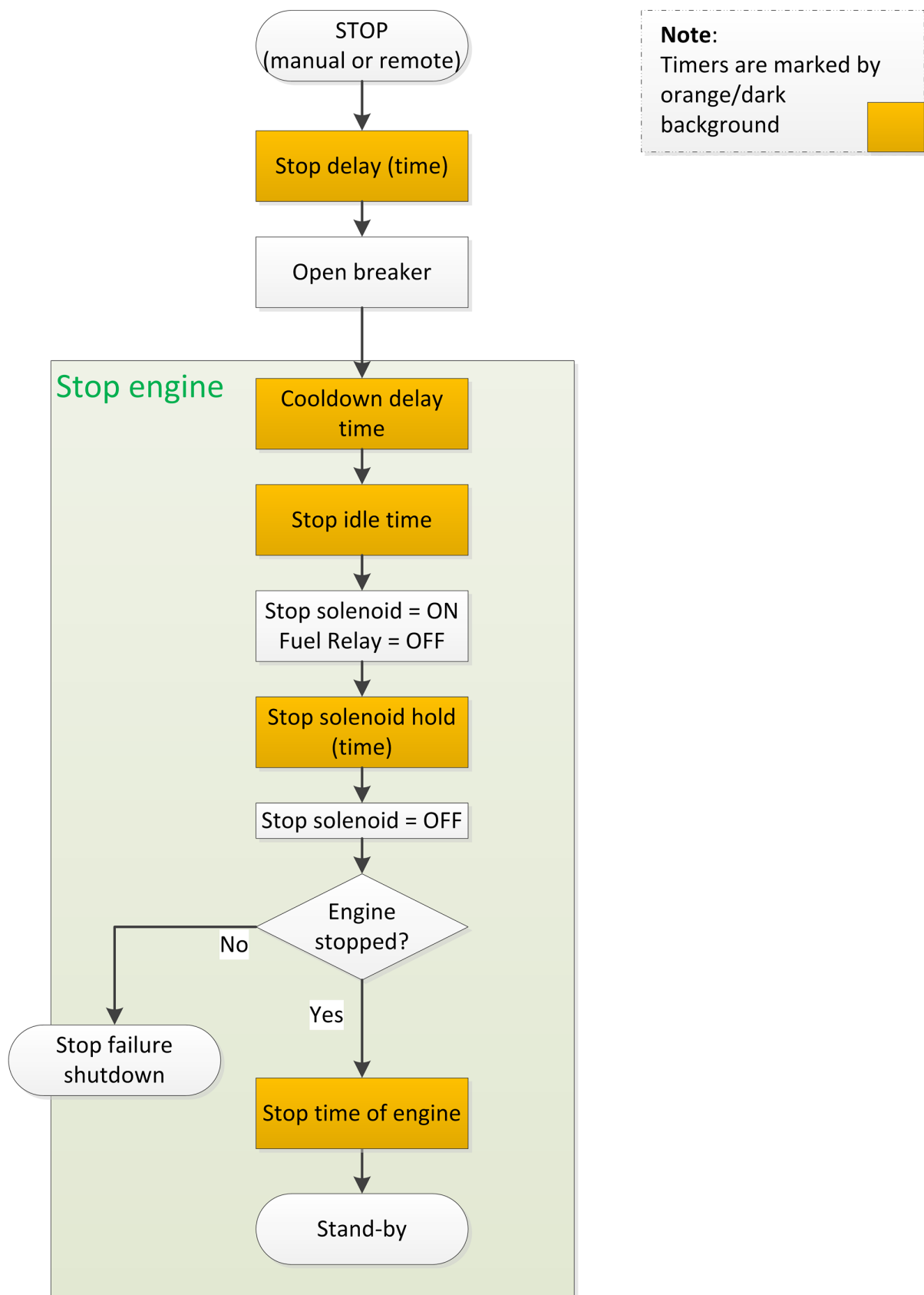
Fig. 4 : Procédure d'arrêt/mise en attente du moteur
