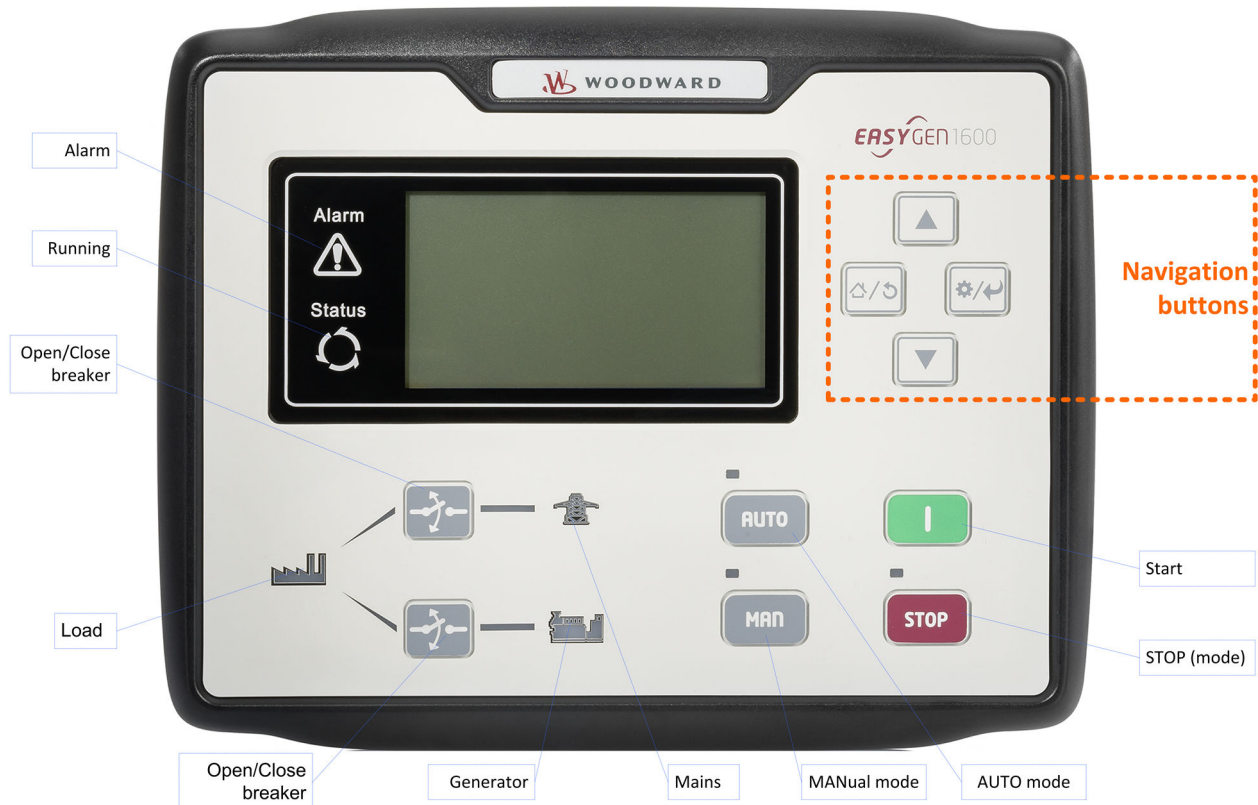
図 2: HMI (フロント パネル) easYgen-1600
