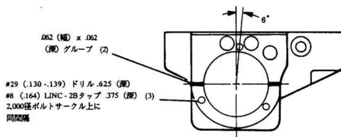
図-2. 17フート・ポンドサーボシリンダの屋外対策用ブーツ穴加工寸法図
