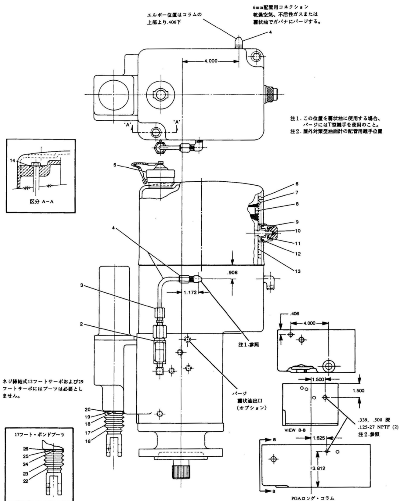
図-1. PG-PL及びPGAガバナ部品参照番号及び屋外対策用継手位置指示図
