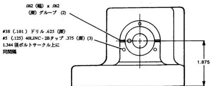
図-3. 29フート・ポンドサーボシリンダの屋外対策用ブーツ穴加工寸法図
