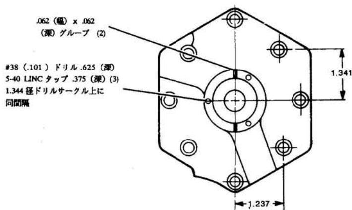
図-3. 29フート・ポンドサーボシリンダの屋外対策用ブーツ穴加工寸法図
