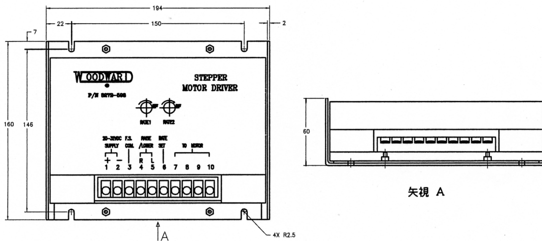
(ドライバー外形図)
