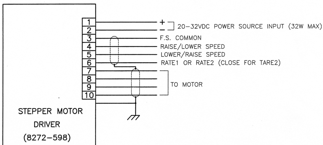
(配線図)
