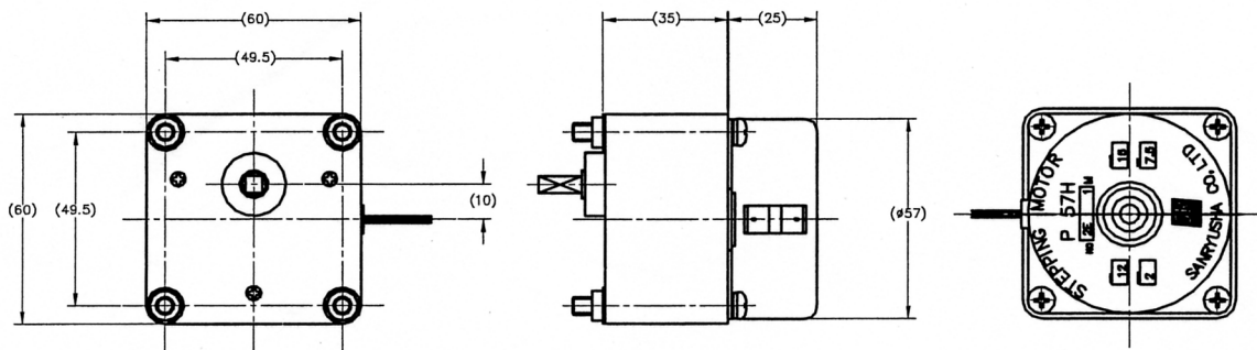
(モータ外形図)
