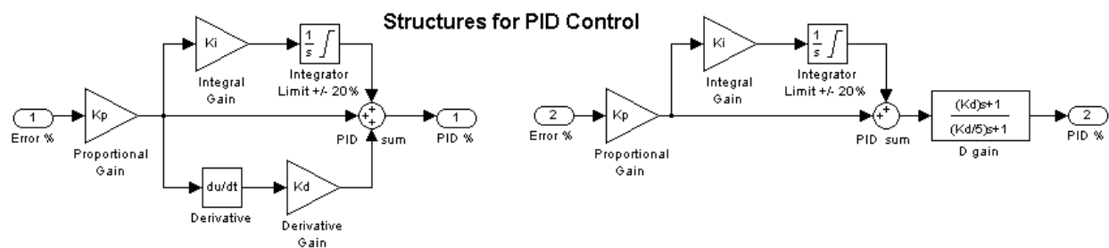
그림 3-5. PID 제어에 대한 구조
