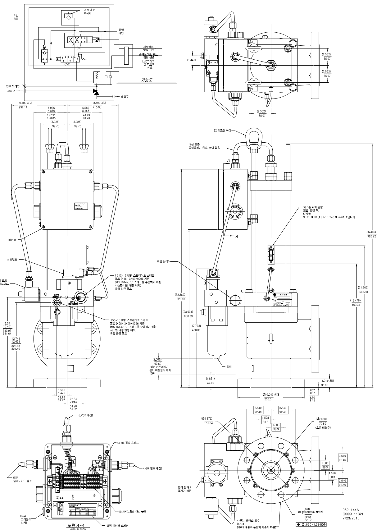
그림 1-7a. 외형도(이중 인입 박스를 가진 4인치 제어 밸브)
