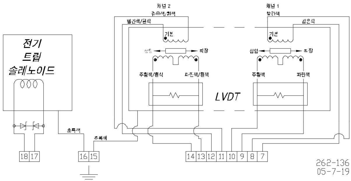
그림 1-11b. 배선도 – 이중 인입 도관 박스
