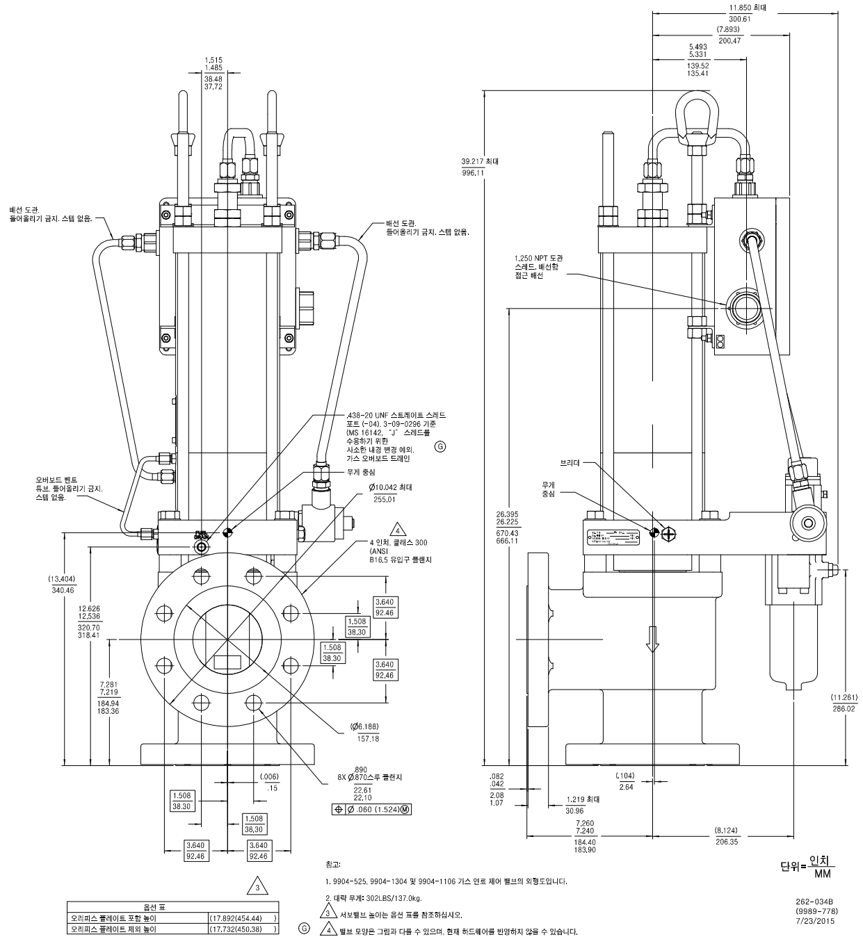
그림 1-6b. 외형도(단일 인입 박스를 가진 4인치 제어 밸브)
