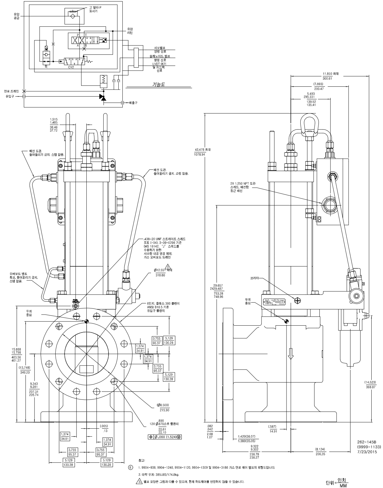
그림 1-9b. 외형도(이중 인입 박스를 가진 6인치 제어 밸브)
