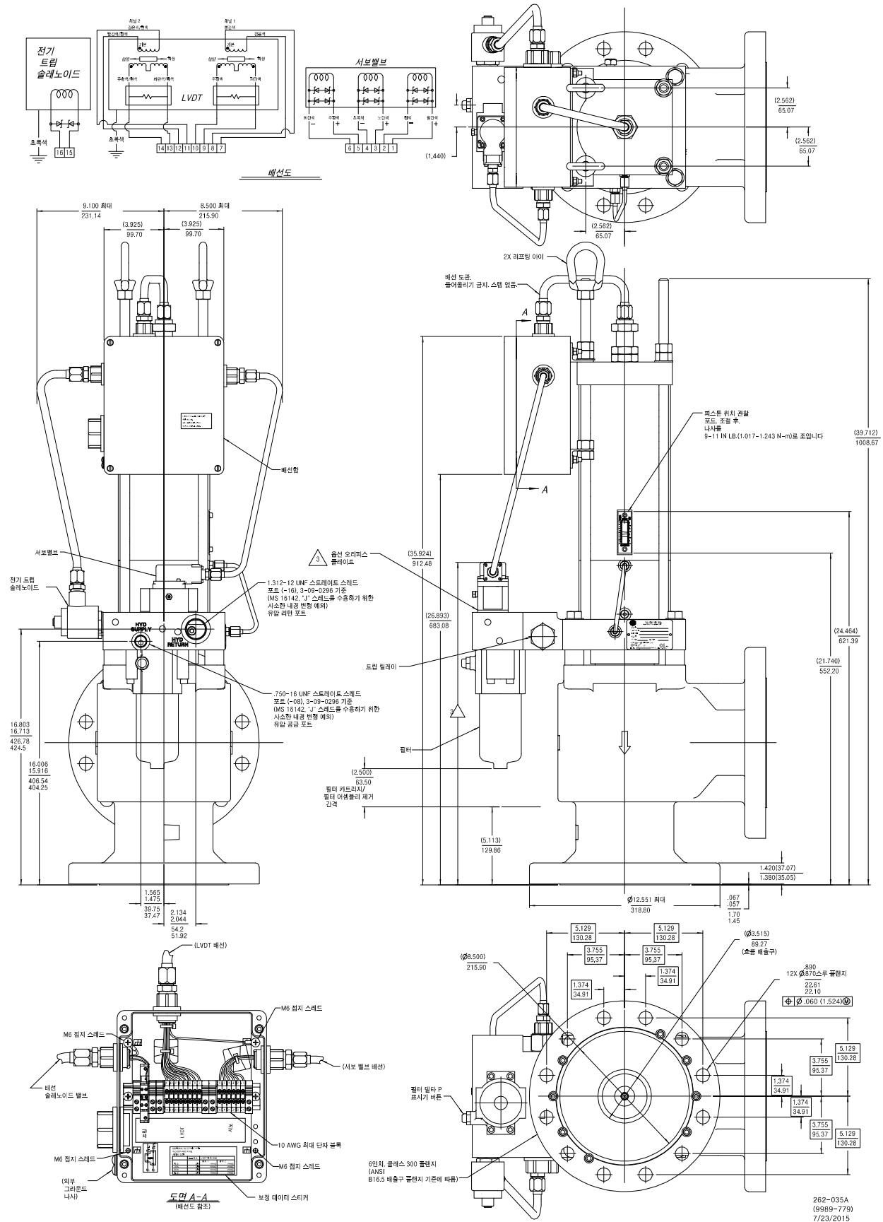
그림 1-8a. 외형도(단일 인입 박스를 가진 6인치 제어 밸브)
