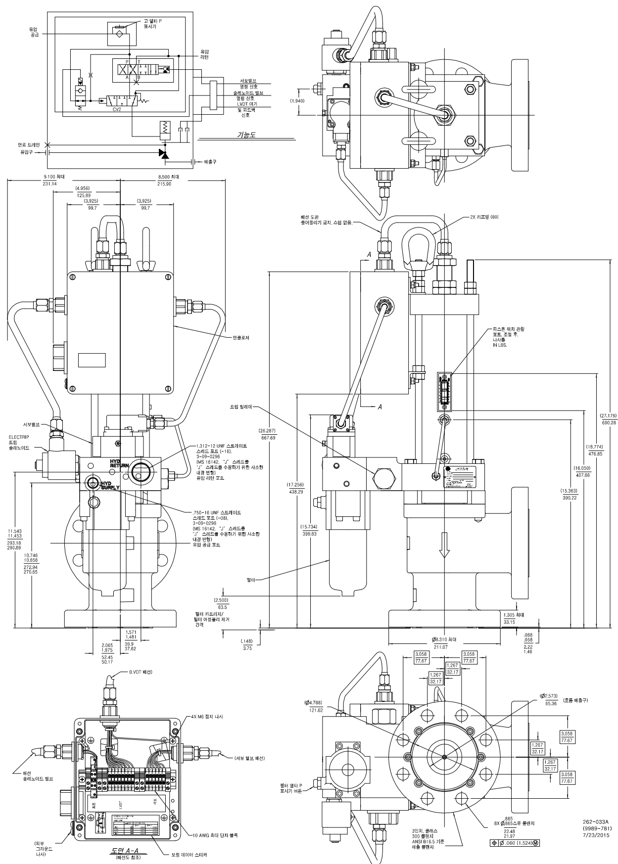
그림 1-4a. 외형도(단일 인입 박스를 가진 3인치 제어 밸브)
