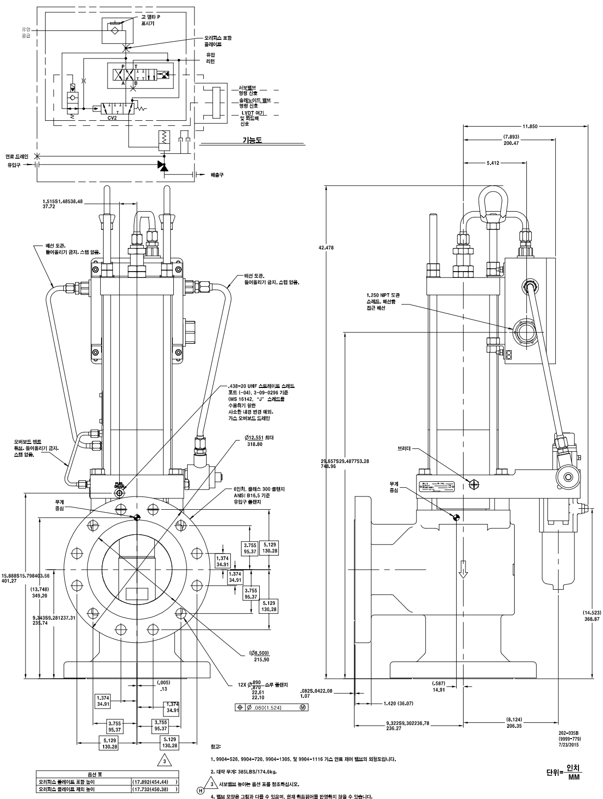
그림 1-5b. 외형도(이중 인입 박스를 가진 3인치 제어 밸브)
