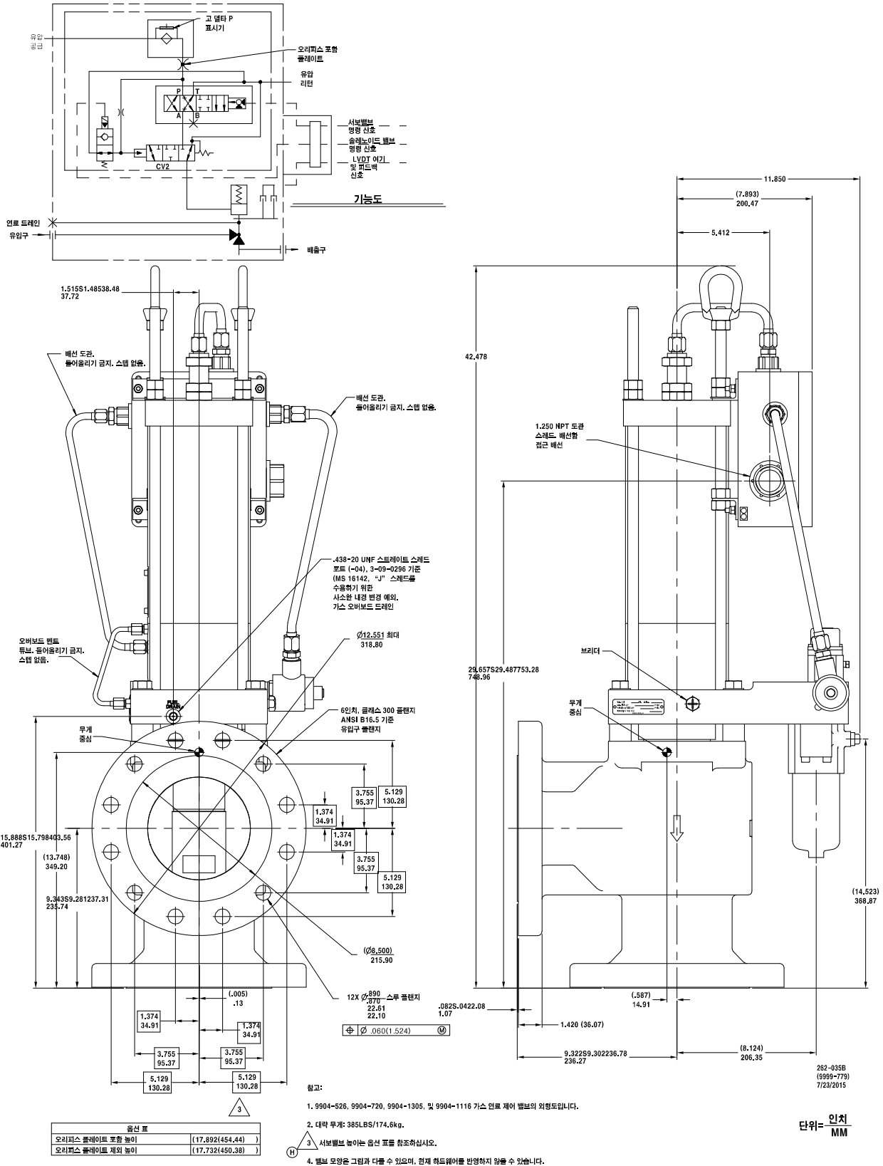
그림 1-8b. 외형도(단일 인입 박스를 가진 6인치 제어 밸브)
