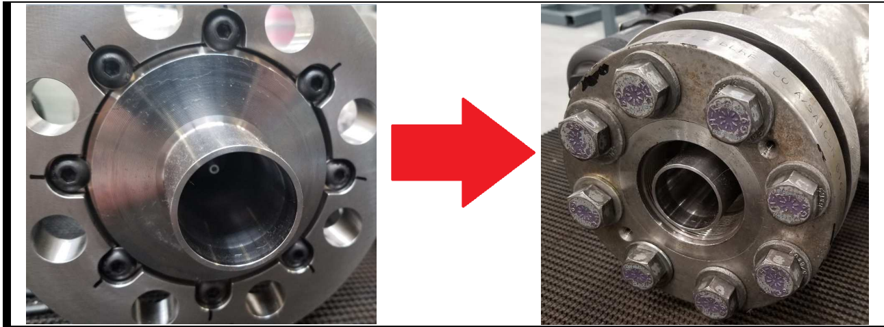
그림 3-3. Extension 스타일 분기 슬리브의 그림
