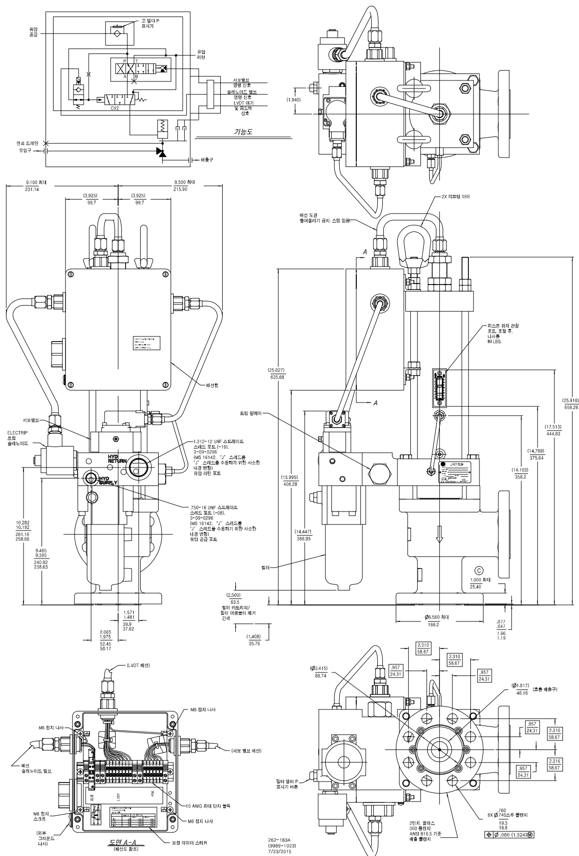
그림 1-2a. 외형도(단일 인입 박스를 가진 2인치 제어 밸브)
