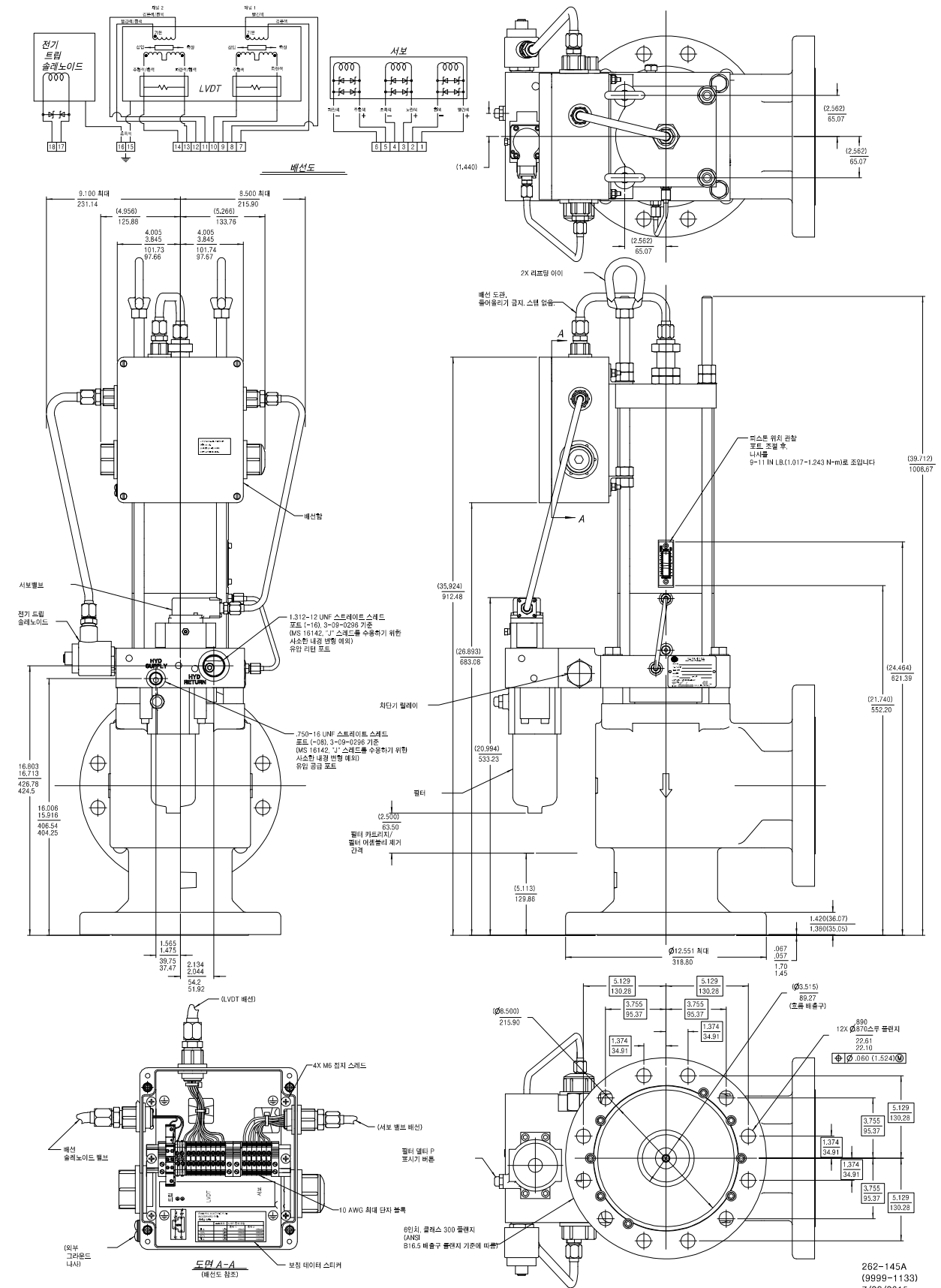
그림 1-9a. 외형도(이중 인입 박스를 가진 6인치 제어 밸브)
