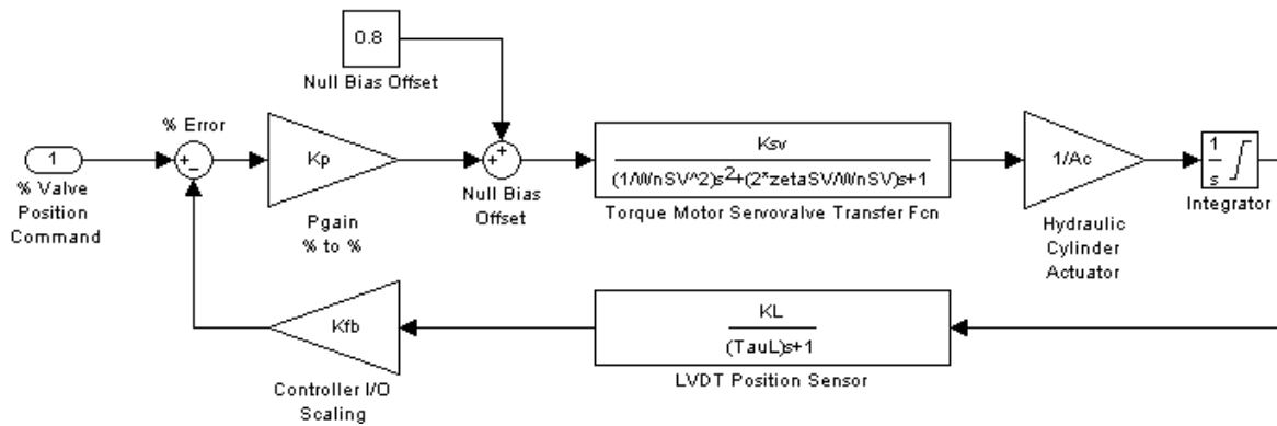
그림 3-4. 가스 연료 제어 밸브 블록도
