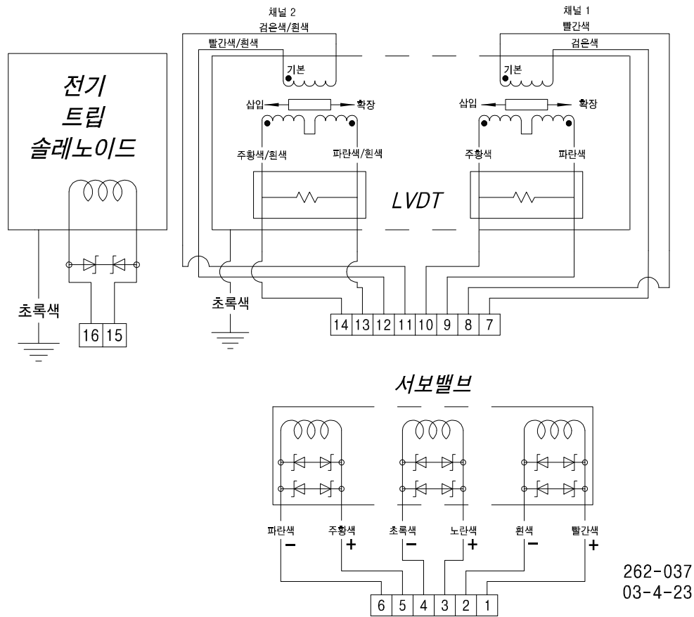
그림 1-11a. 배선도 – 단일 인입 도관 박스
