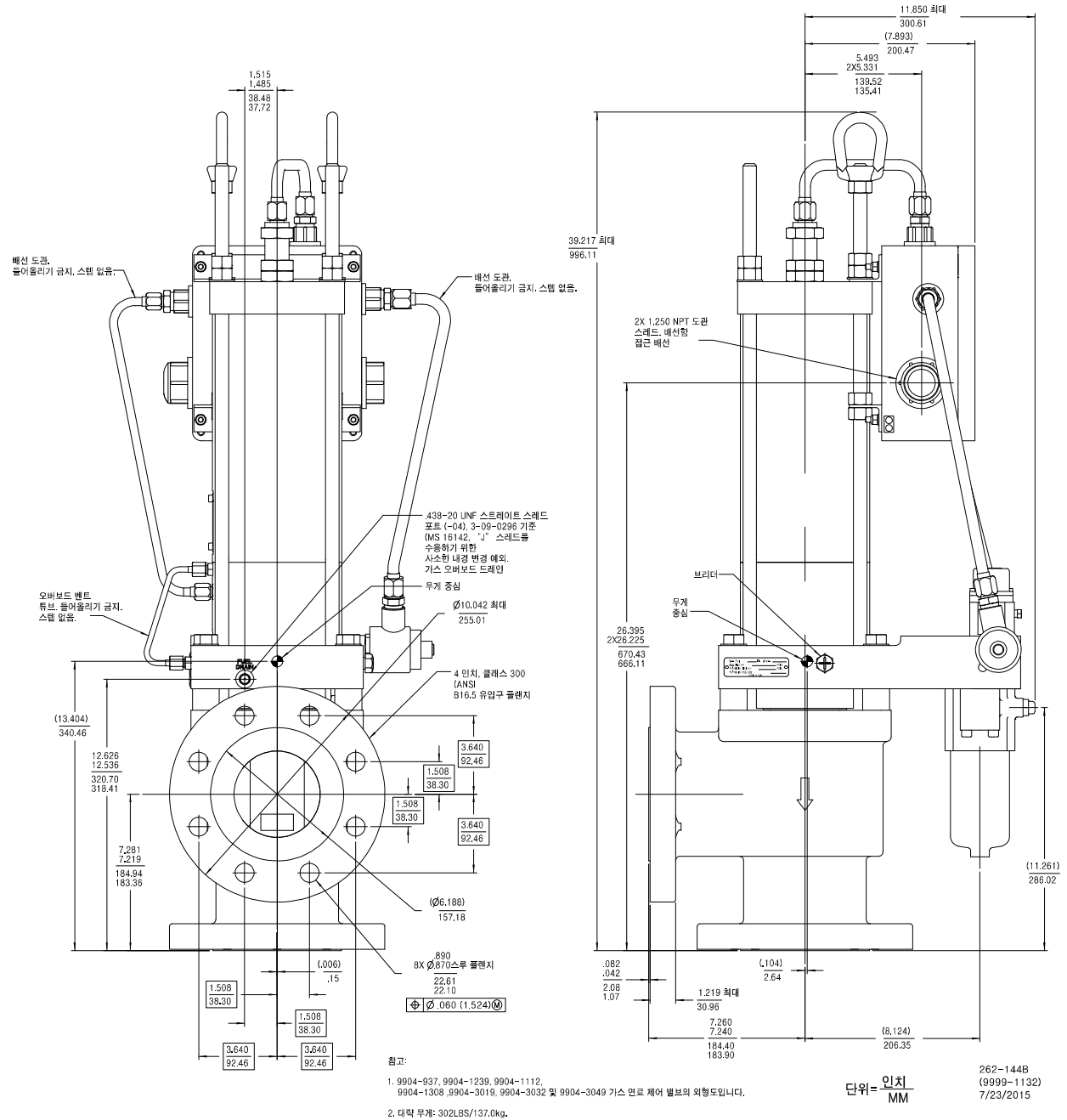
그림 1-7b. 외형도(이중 인입 박스를 가진 4인치 제어 밸브)
