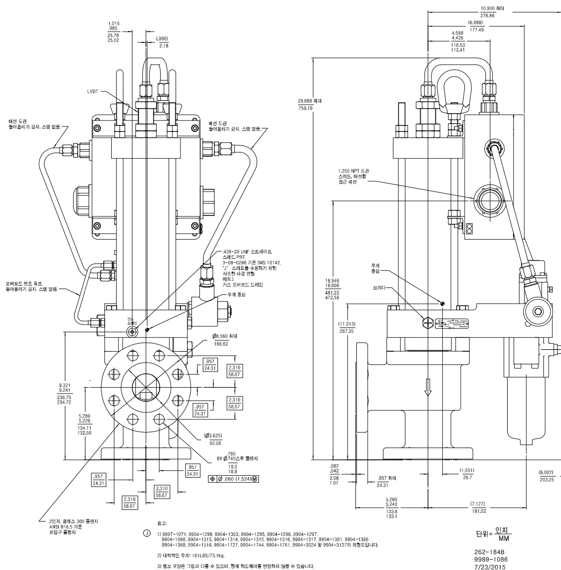
그림 1-3b. 외형도(이중 인입 박스를 가진 2인치 제어 밸브)
