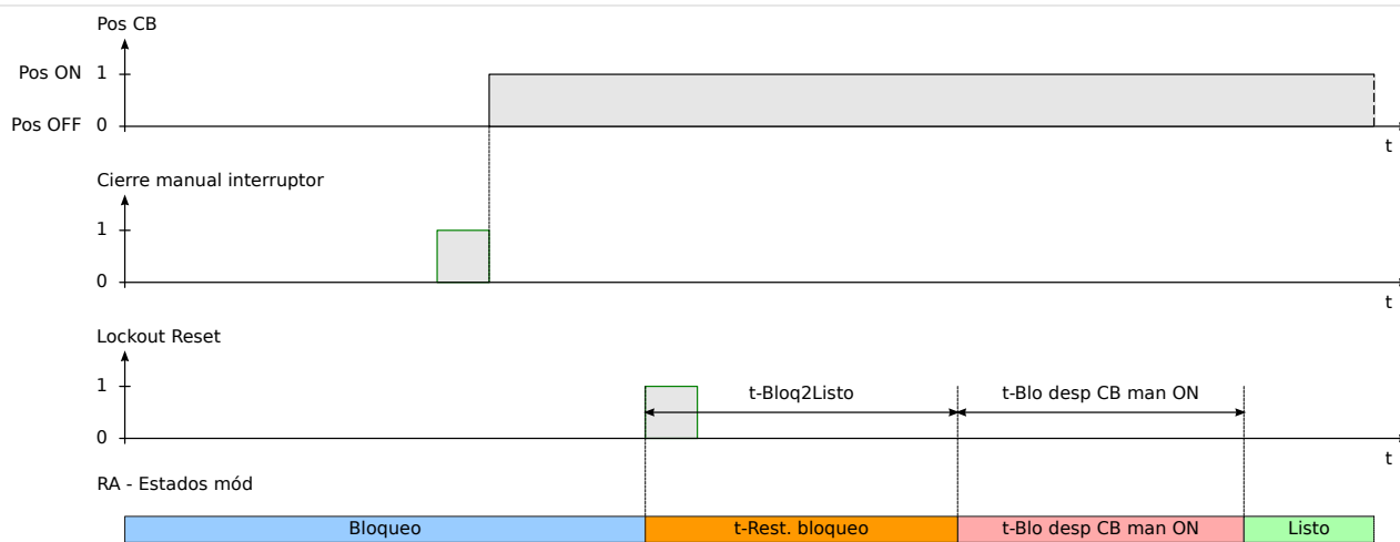
Fig. 108: Lógica de reinicio de bloqueo de AR en caso de que el reinicio de bloqueo llegue después de que se cierre el interruptor manualmente.
