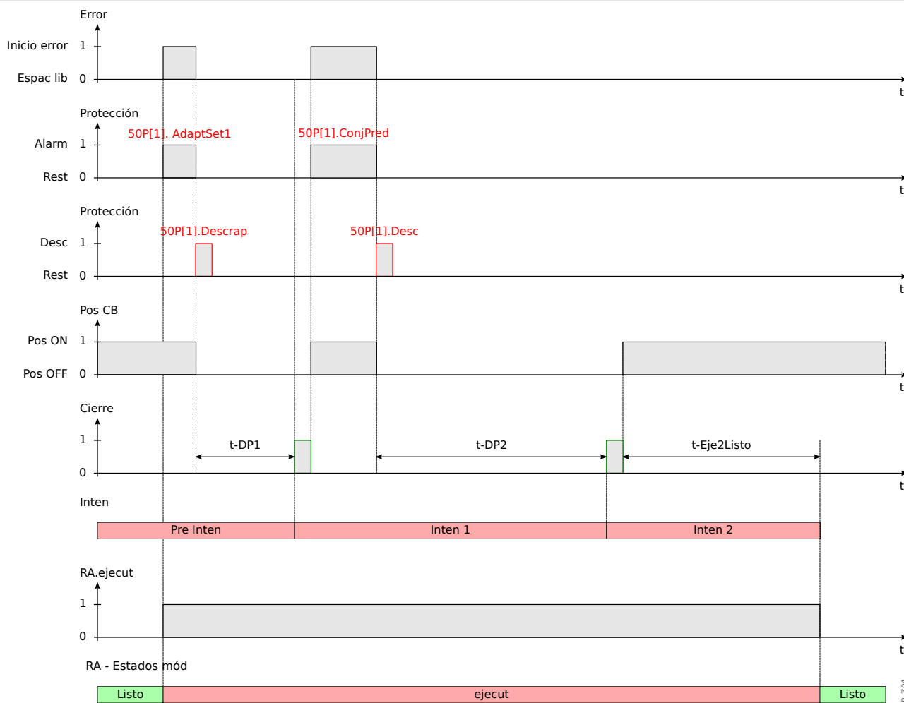
Fig. 104: Diagrama de tiempo de reconexión automática para el esquema de reconexión automática de dos intentos successful (correctos) con aceleración en un intento previo.
