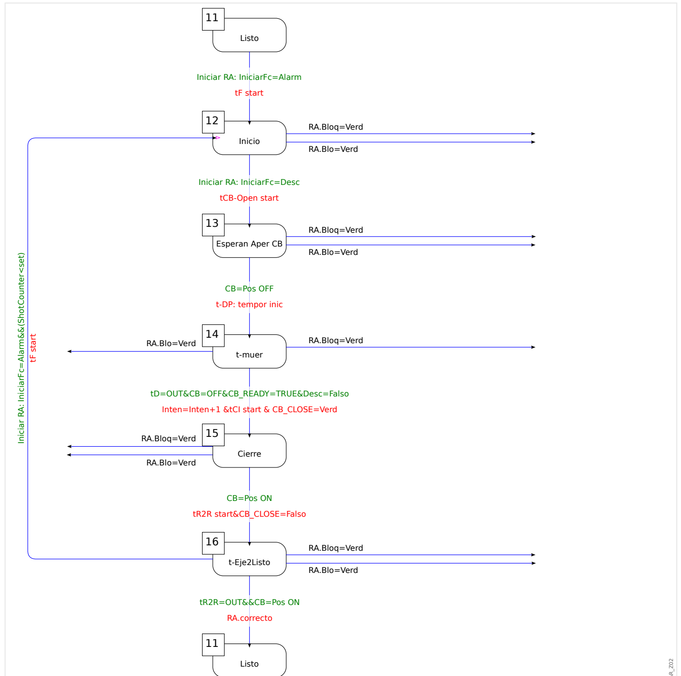
Fig. 102: Ciclo de ejecución de RA (estado 4).
