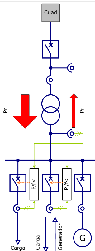
Fig. 96: Reducción de carga descentralizada por subfrecuencia en redes eléctricas con alimentación temporal.
