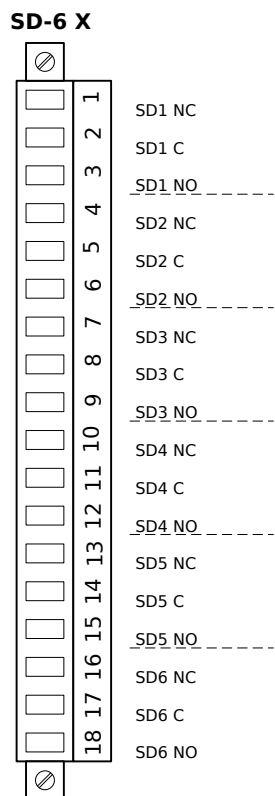
Fig. 13: Asignación electromecánica
