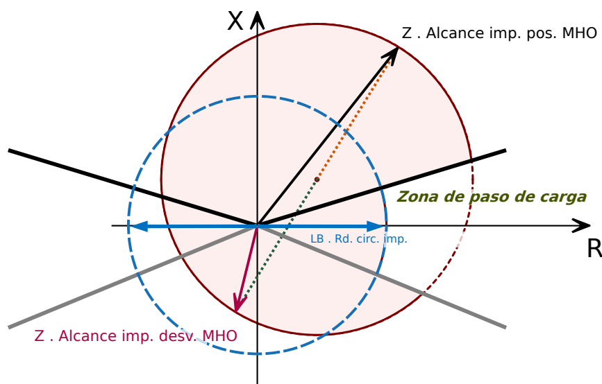
Fig. 98: Característica de operación de impedancia (en color rojo brillante) con paso de carga activa.
