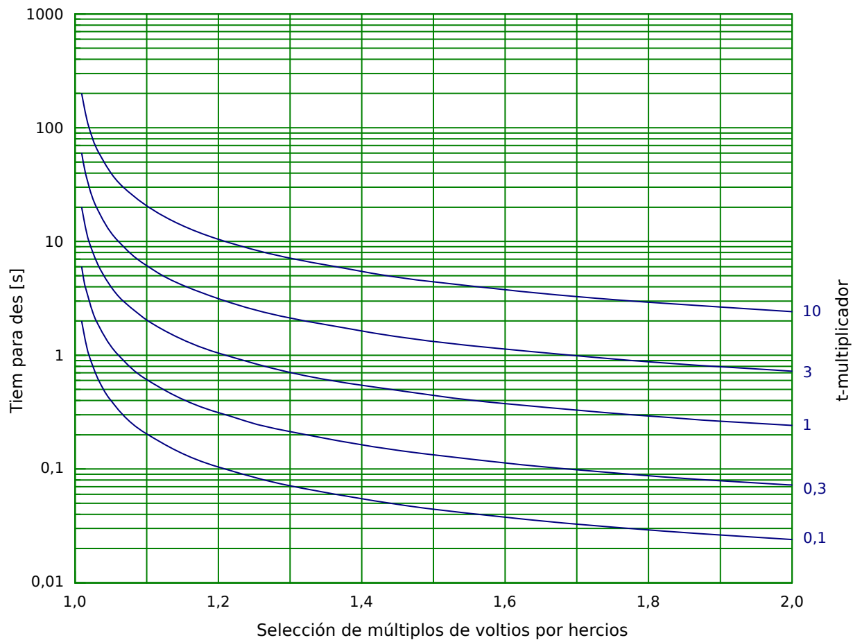
Fig. 120: Características/Forma curva: INV C
