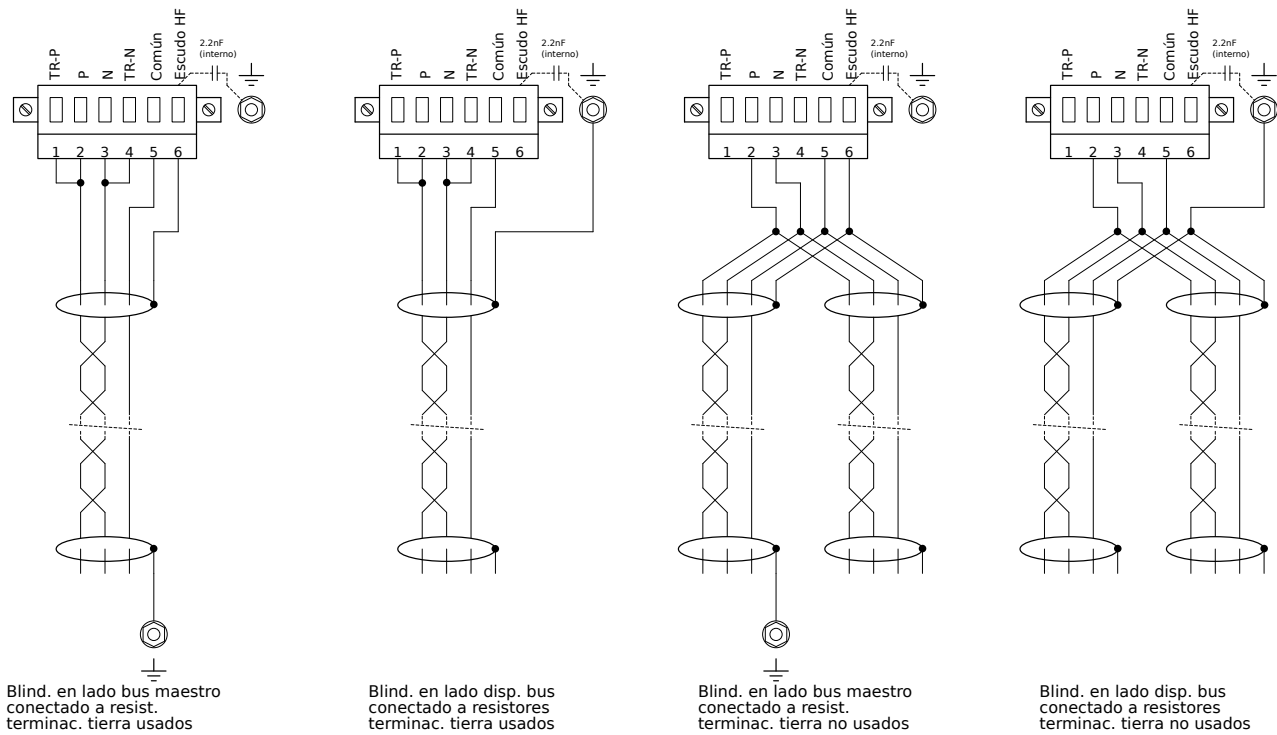
Fig. 59: Opciones de blindaje (3 cables + blindaje)
