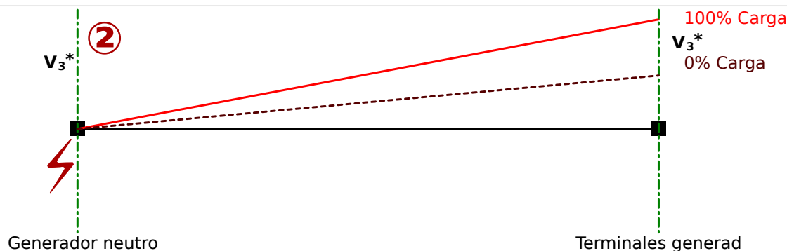
Fig. 127: Distribución de la tensión del tercer armónico V_3 , fallo en el lado neutro.
