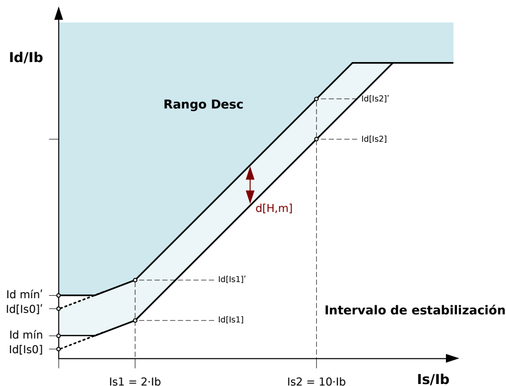
Fig. 85: Aumento dinámico temporal de la característica de desconexión estática.
