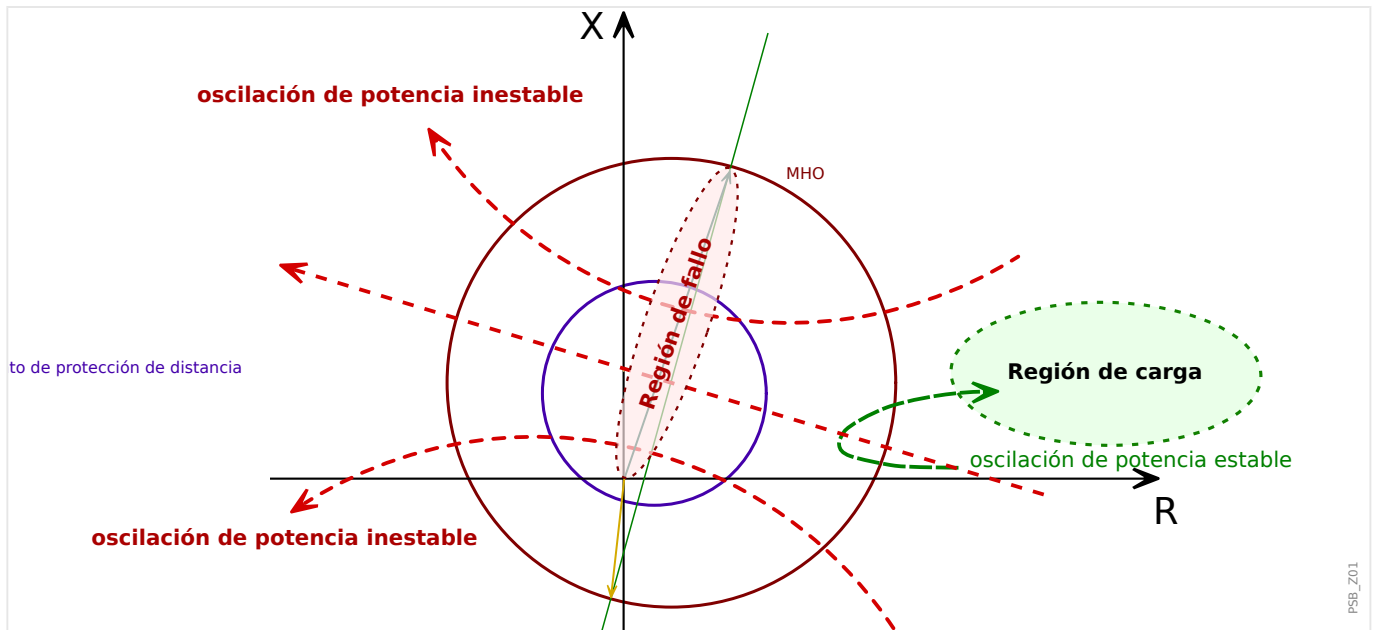
Fig. 106: Región de carga y trayectorias de impedancia.
