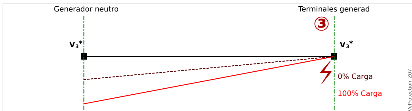
Fig. 128: Distribución de la tensión del tercer armónico V_3 , fallo en el lado del terminal.
