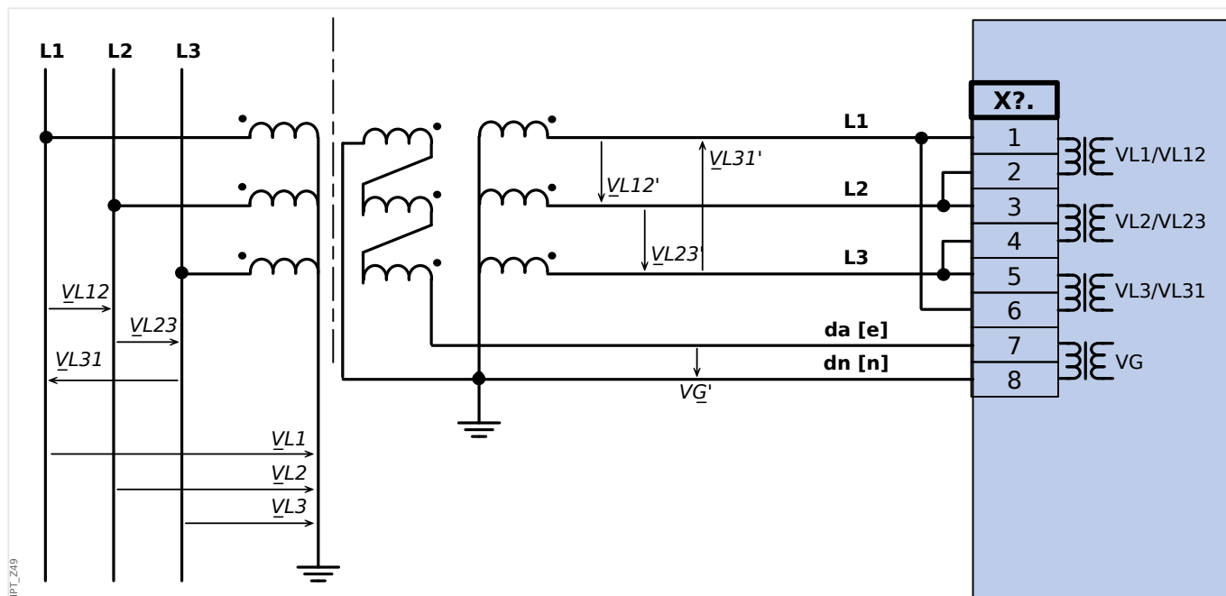
Fig. 41: Medida de tensión trifásica (cableado de las entradas de medición: "conexión delta") Medida del VG de voltaje residual a través de bobinas auxiliares (e-n) "delta roto"
