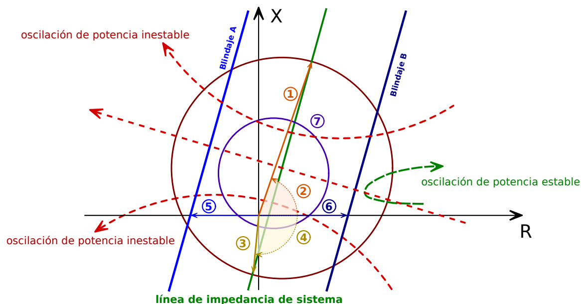
Fig. 107: Característica PSB.
