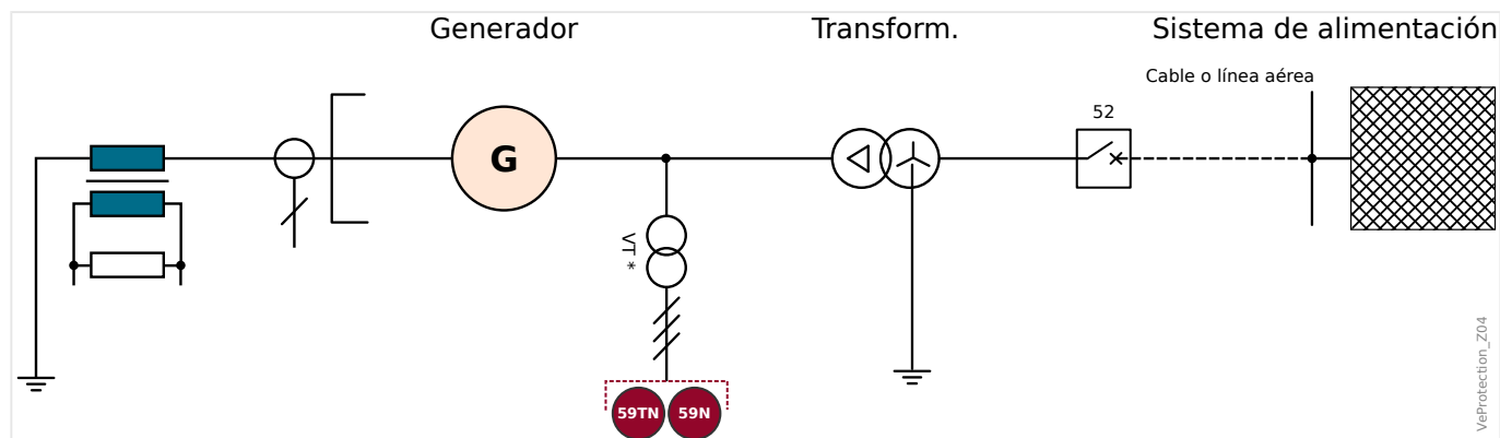
Fig. 130: Protección de fallo de tierra de estator del 100 % obtenida con la combinación ANSI 59TN/59N.
