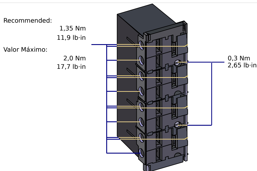
Fig. 174: Conector enchufable con cortocircuitador integrado (entradas de corriente convencionales)
