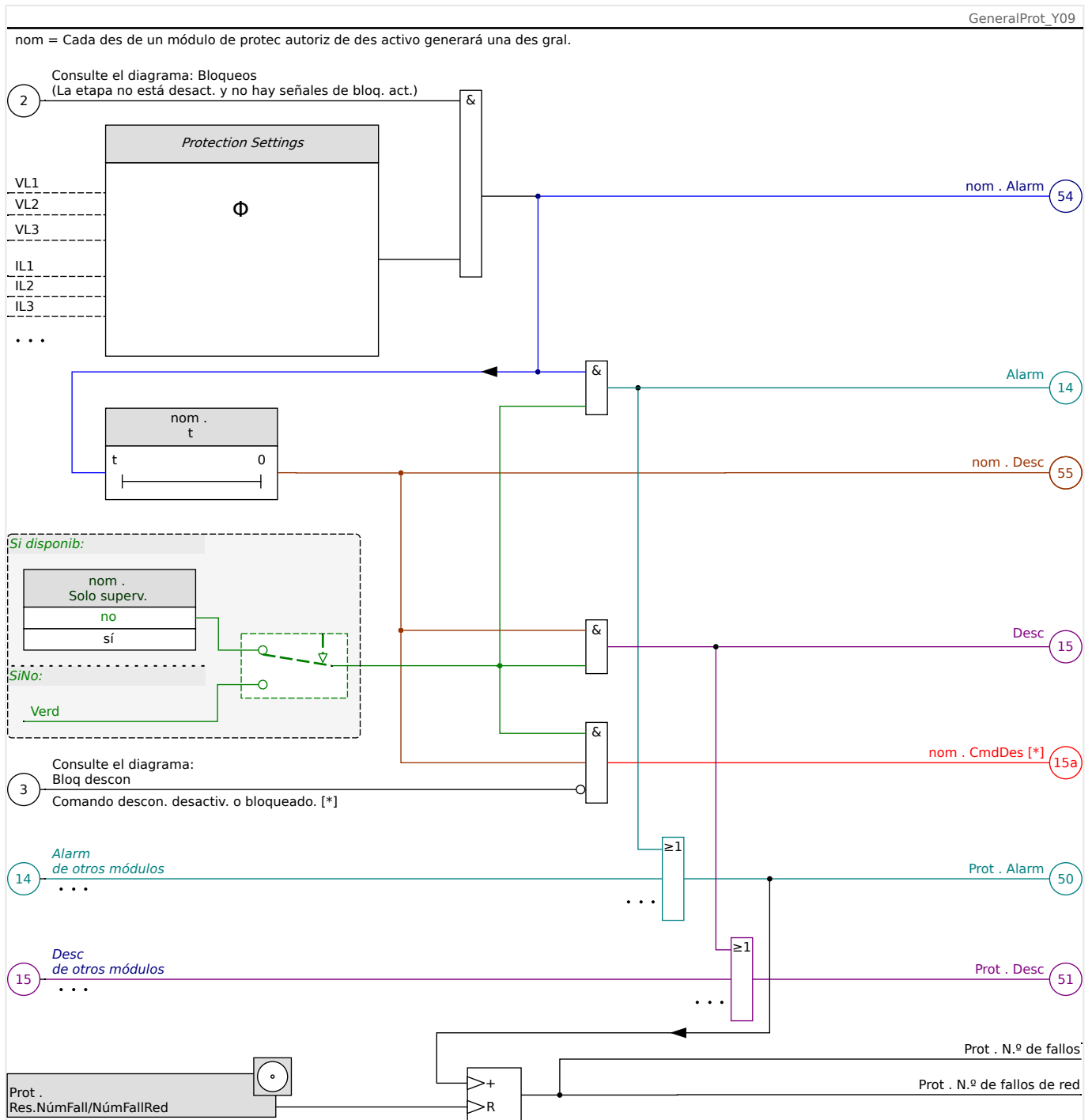
Fig. 72: Descripción a grandes rasgos de la funcionalidad de cualquier elemento de protección de HighPROTEC.
