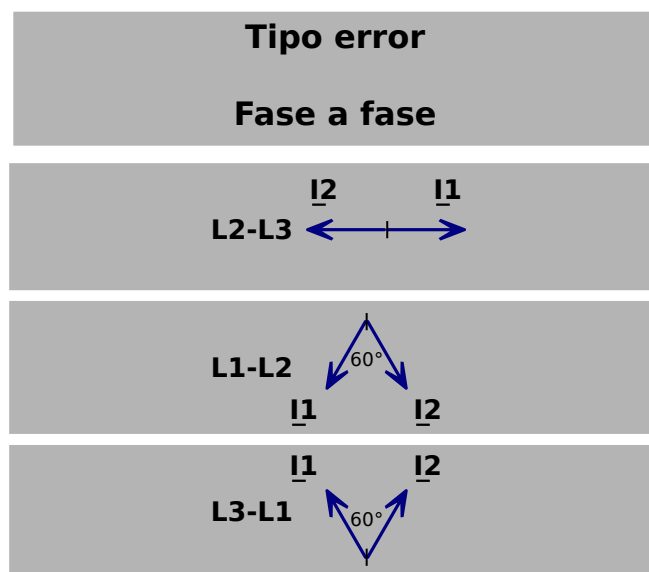
Fig. 92: Fasores de corriente de secuencia de fase positiva y negativa para distintos tipos de fallo.
