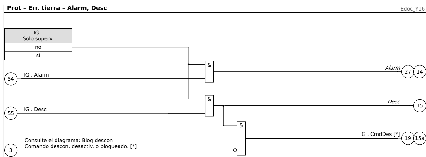
Fig. 114: Protección de sobrecarga de tierra, parte 2 (comando de desconexión y activación de alarma general y desconexión general).
