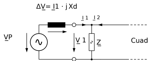
Fig. 131: Circuito equivalente en generador sincrónico en paralelo con la red de suministro eléctrico.
