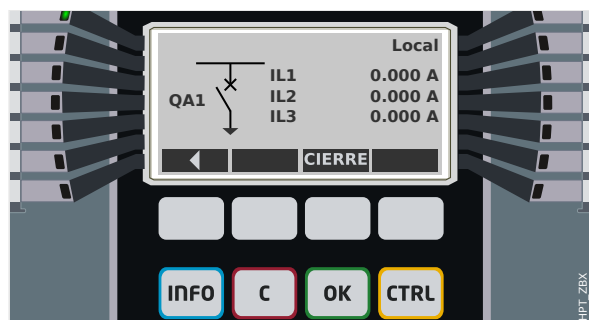
Fig. 158: Ejemplo de página de control, con el circuito en posición abierta.
