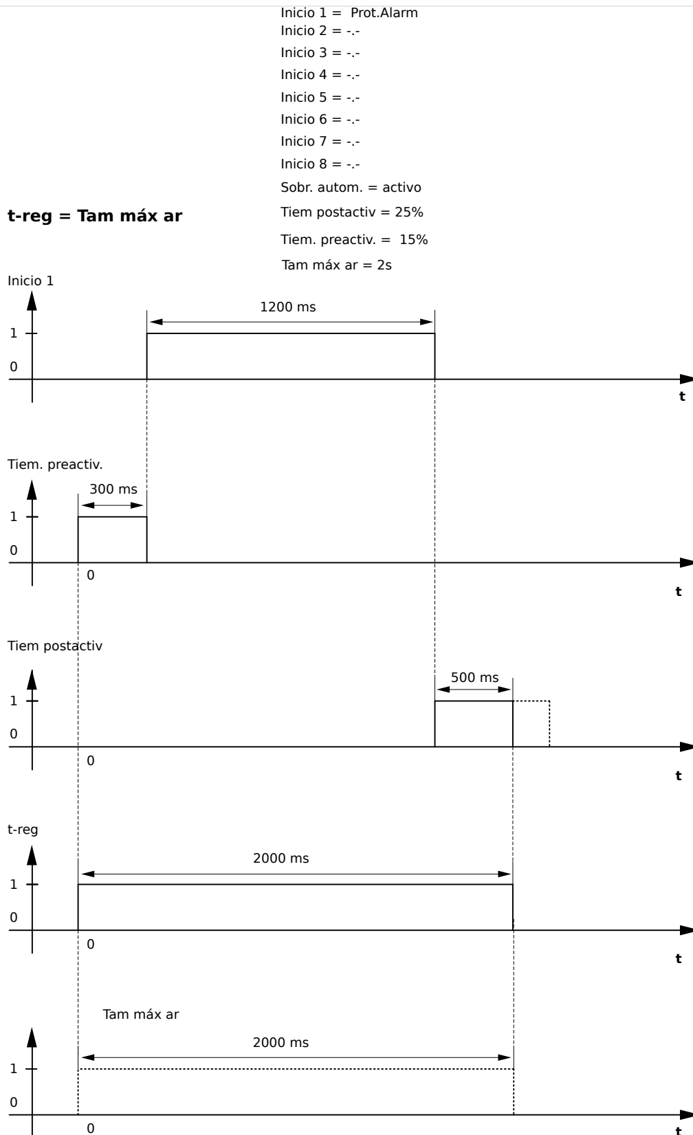
Fig. 164: Ejemplo 1: cuadro de intervalos del registrador de perturbaciones
