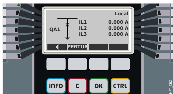
Fig. 156: Ejemplo de página de control, con el circuito en posición cerrada.
