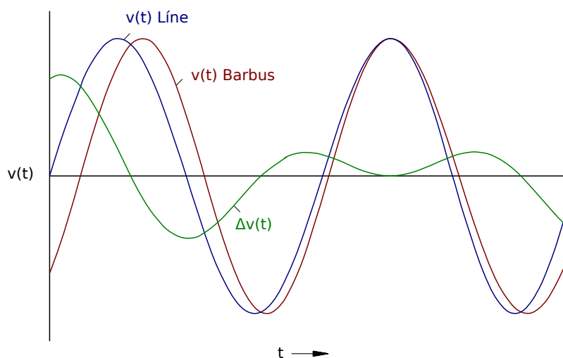
Fig. 138: Curva de tensión con resolución ampliada.
