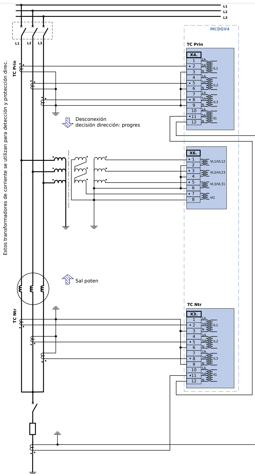
Fig. 43: Generador con conexión a tierra de baja resistencia con protección diferencial de fase y tierra
