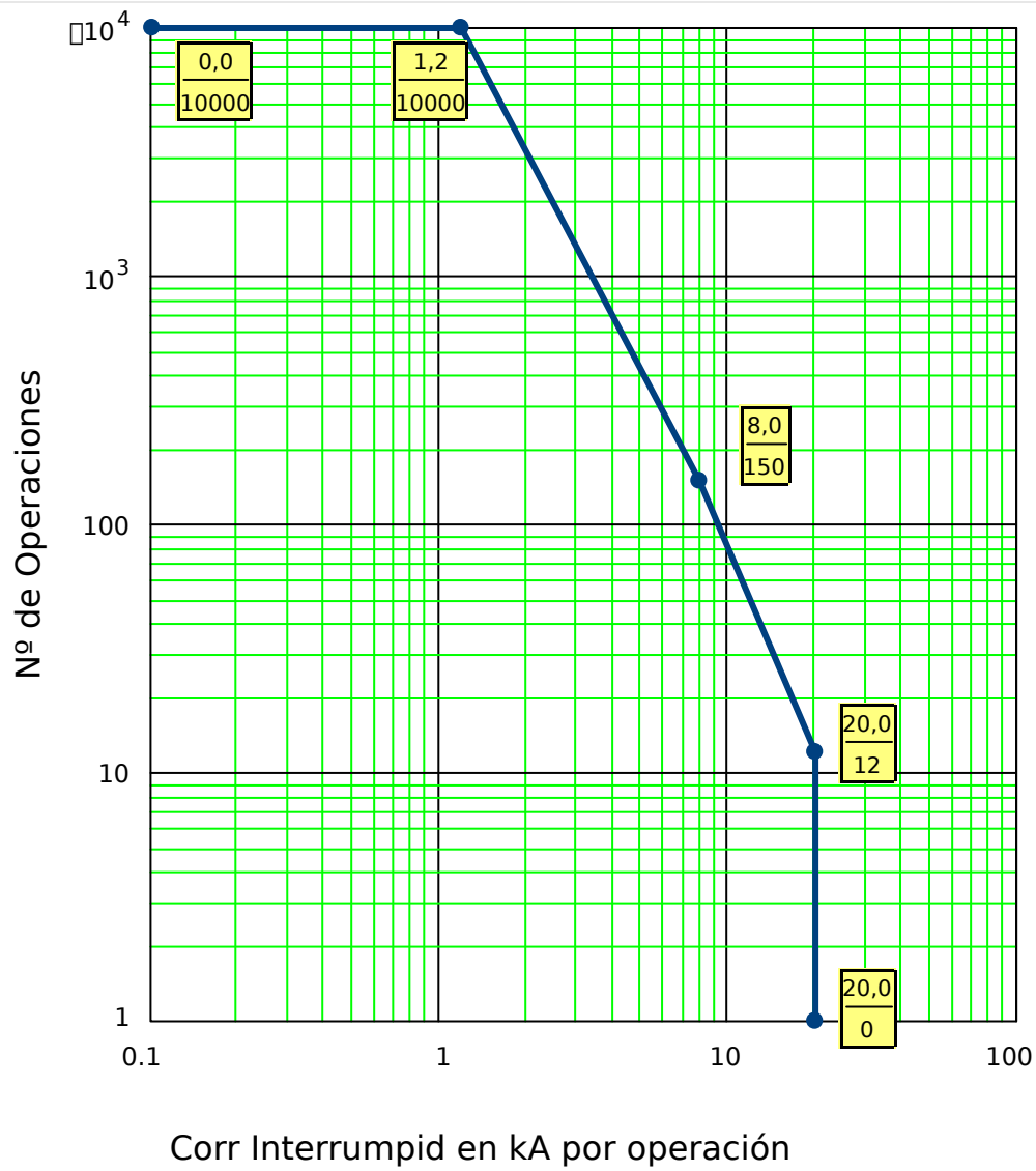
Fig. 161: Curva Mantenim Interruptor para Interrupt Circuito típico 25kV
