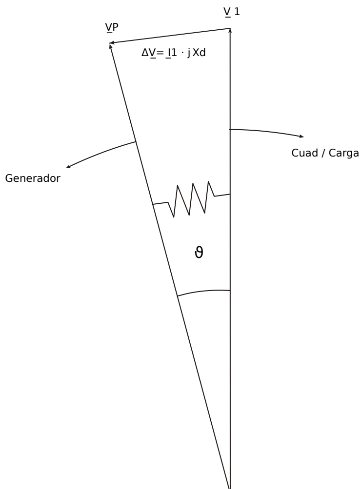
Fig. 132: Vectores de tensión en funcionamiento en paralelo con la red de suministro eléctrico.
