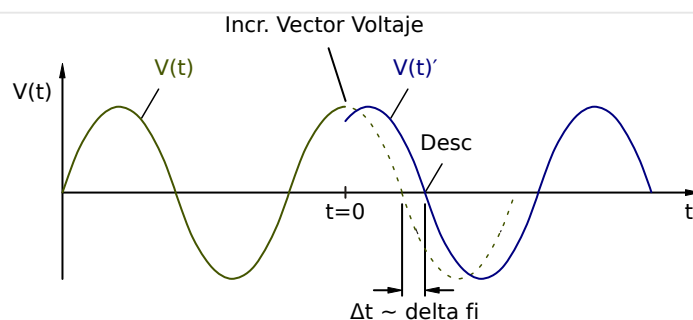
Fig. 135: Incremento vectorial de tensión.
