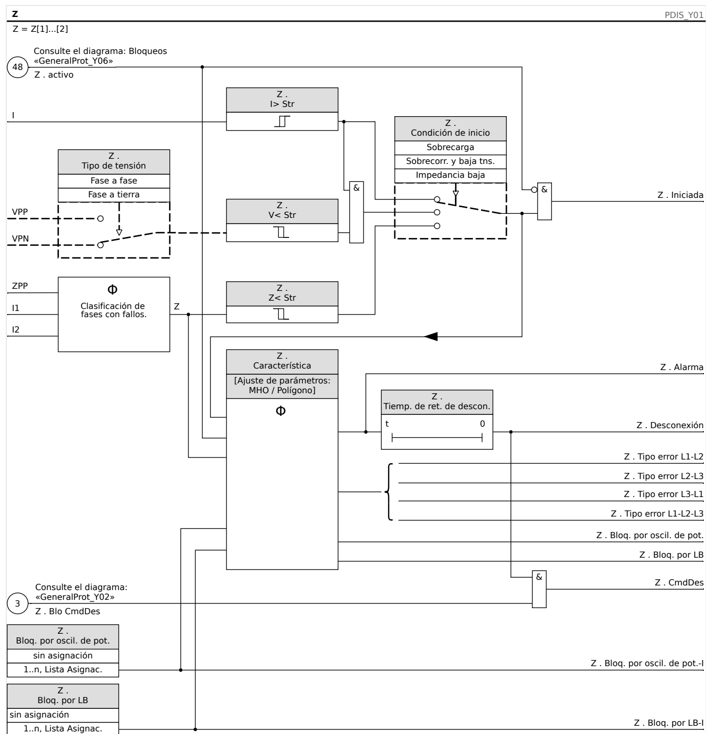
Fig. 99: Funcionalidad del módulo Z.
