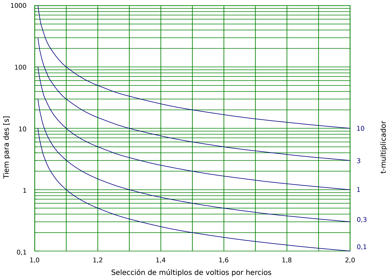
Fig. 119: Características/Forma curva: INV B
