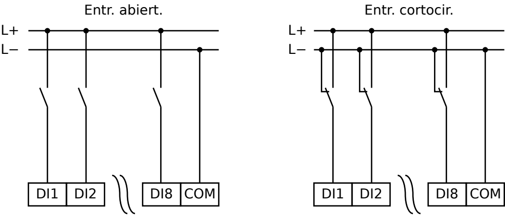
Fig. 177: Estado seguro de entradas digitales
