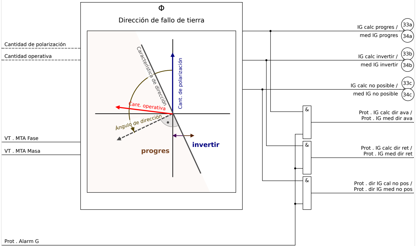
Fig. 76: Detección de dirección en todos los métodos, excepto " \cos(\phi) ", " \sin(\phi) ".
