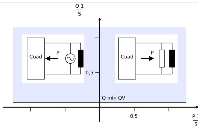
Fig. 143: Método 2: Supervisión de potencia reactiva pura.
