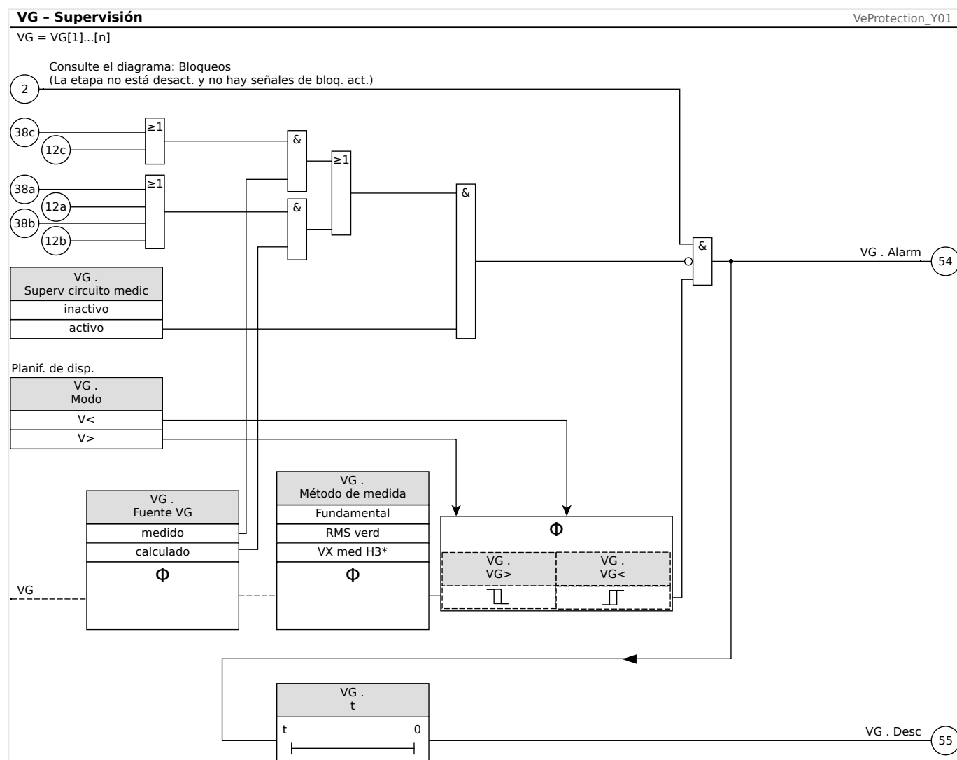
Fig. 124: VG, VX Supervisión de tensión, parte 1 (función de supervisión, decisión de desconexión).
