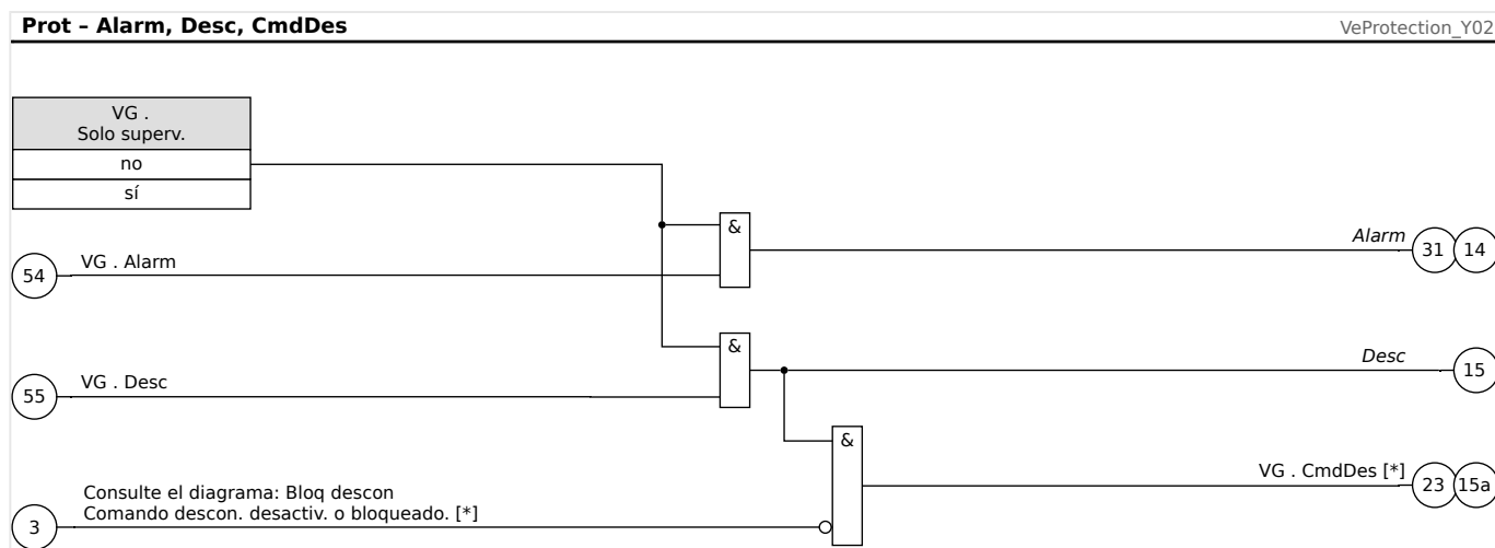
Fig. 125: VG, VX Supervisión de tensión, parte 2 (comando de desconexión y activación de alarma general y desconexión general).
