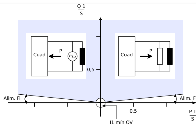
Fig. 142: Método 1: Supervisión de ángulo de potencia
