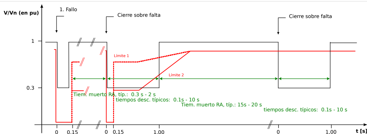
Fig. 145: Recorrido de la curva de tensión durante dos intentos fallidos de reconexión automática; fuente: Technische Richtlinie, Erzeugungsanlagen am Mittelspannungsnetz, Ausgabe Juni 2008, BDEW Bundesverband der Energie- und Wasserwirtschaft e.V. (Página 89).
