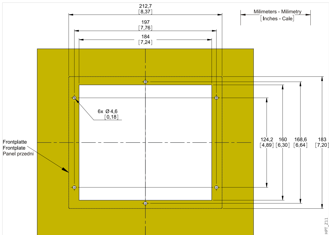
Fig. 6: Corte de puerta de carcasa B2 (versión de 8 botones) Todas las dimensiones se expresan en mm, excepto las dimensiones entre paréntesis [pulg.]
