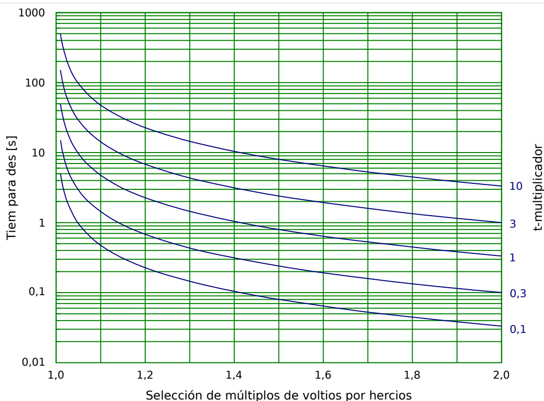
Fig. 118: Características/Forma curva: INV A
