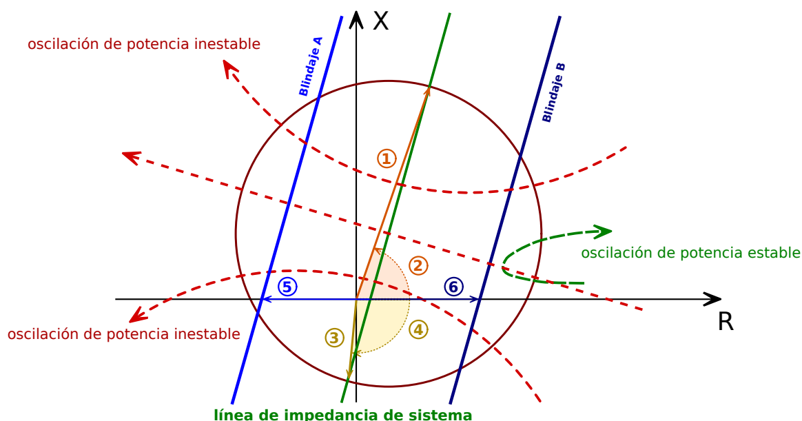
Fig. 103: Característica de salto de vector y esquema de blindaje de esquema único.
