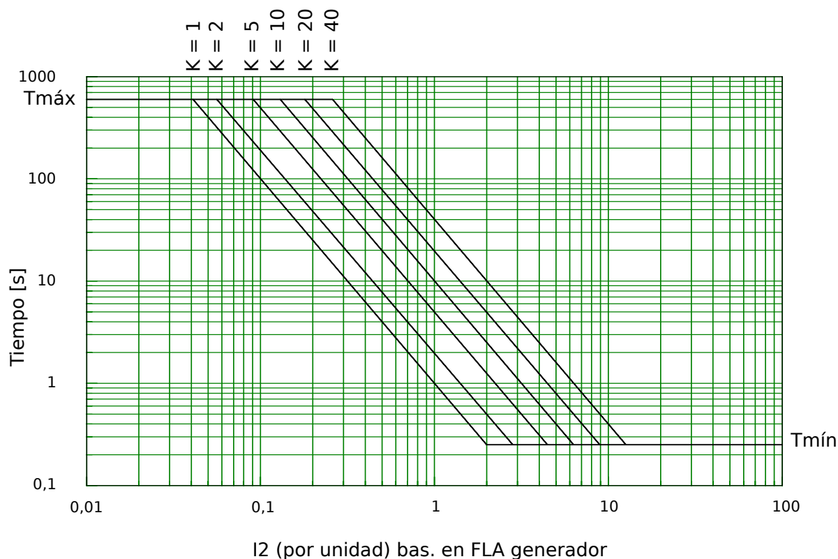
Fig. 115: Curvas de desconexión de desequilibrio del generador.
