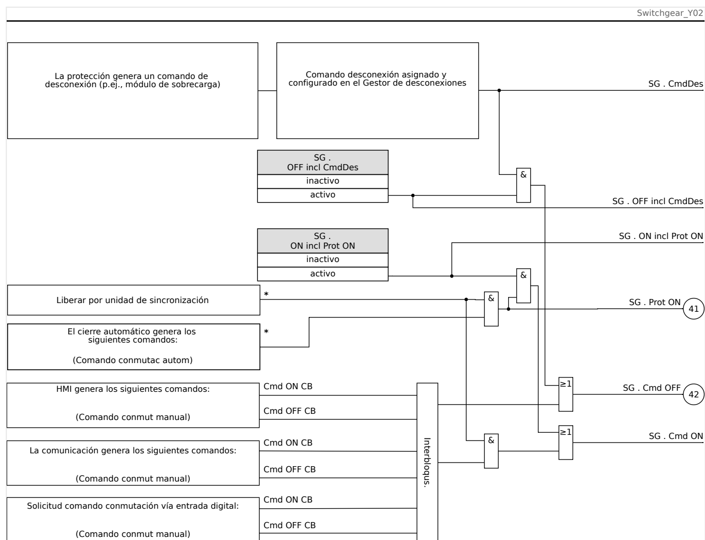
Fig. 159: Interbloqueos. La disponibilidad de las partes etiquetadas con “*” depende del tipo de dispositivo pedido.
