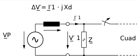
Fig. 133: Circuito equivalente en fallo de red eléctrica.
