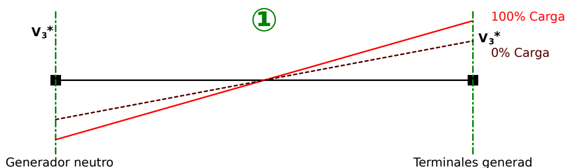
Fig. 126: La distribución de la tensión del tercer armónico V_3 en condiciones normales.
