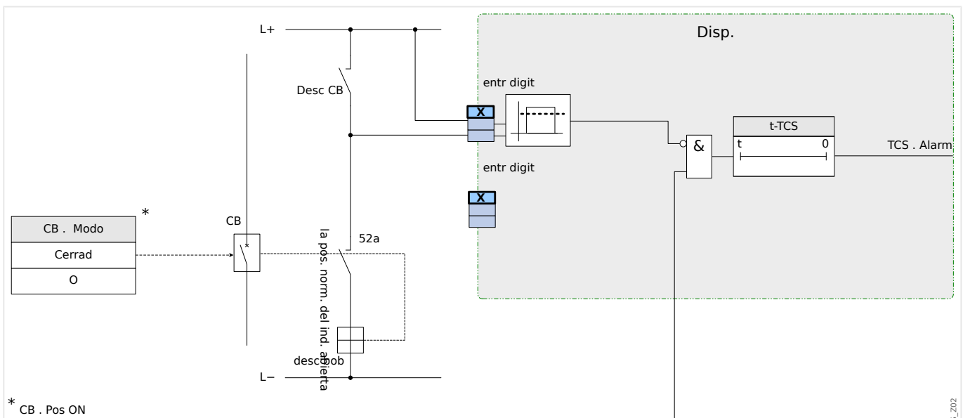
Fig. 153: Ejemplo de conexión: Supervisión del circuito de desconexión solo con un contacto auxiliar CB »Aux ON« (52a).
