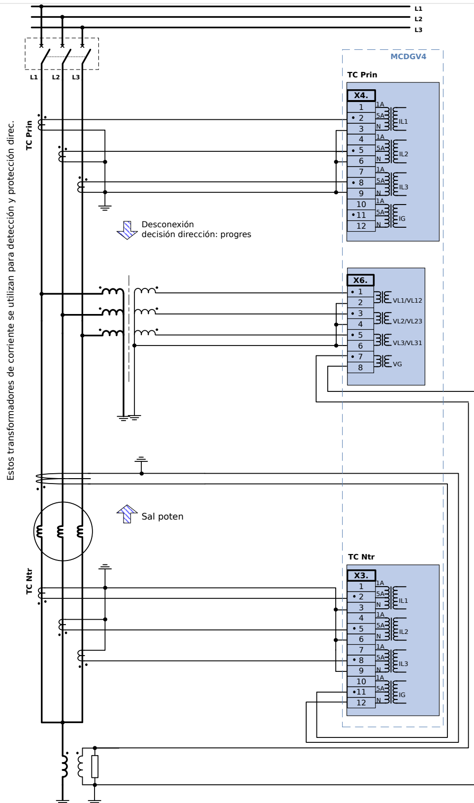
Fig. 45: Generador con conexión a tierra de alta impedancia con protección diferencial de fase y protección de tierra con estator 100%
