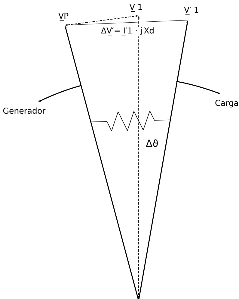
Fig. 134: Fallo de los vectores de tensión en la red.
