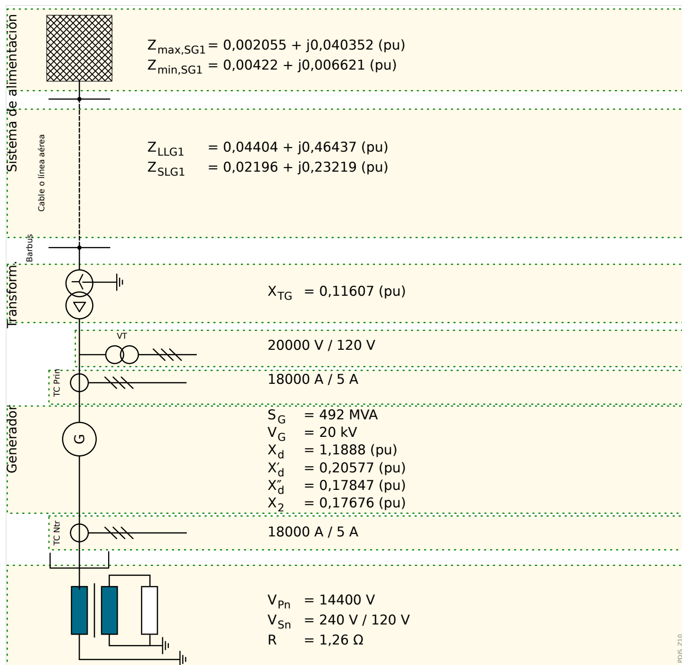
Fig. 101: Diagrama de línea única con datos basados en el generador.
