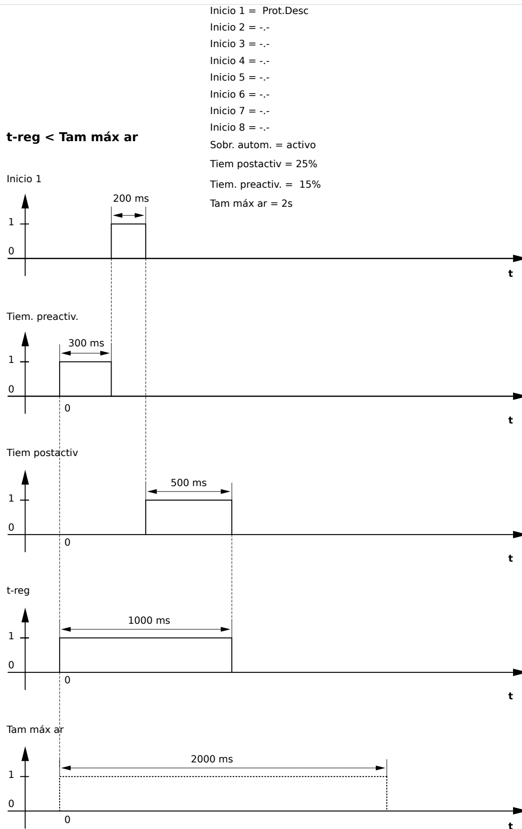
Fig. 165: Ejemplo 2: cuadro de intervalos del registrador de perturbaciones
