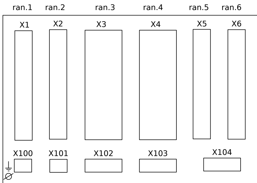
Fig. 7: Carcasa B2 - diagrama esquemático.
