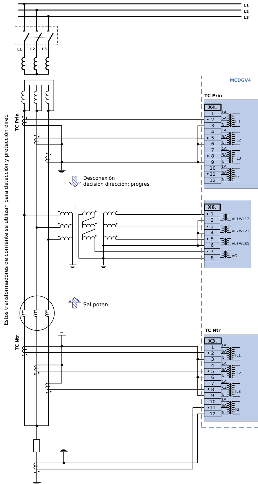
Fig. 47: Generador con conexión a tierra de baja resistencia y unidad de transformador elevador solo con protección diferencial de fase de generador
