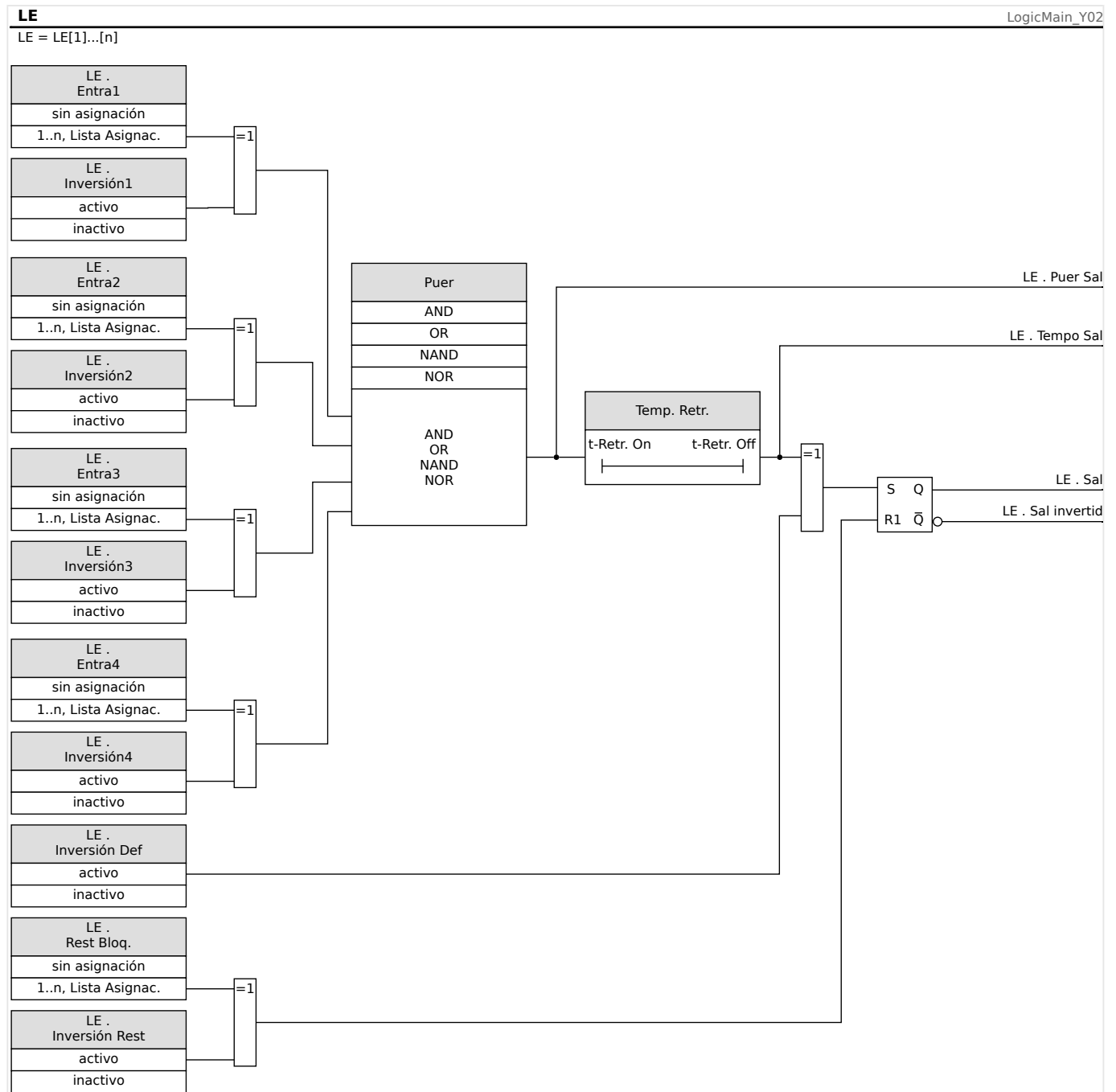
Fig. 168: Descripción detallada - Diagrama de lógica general.
