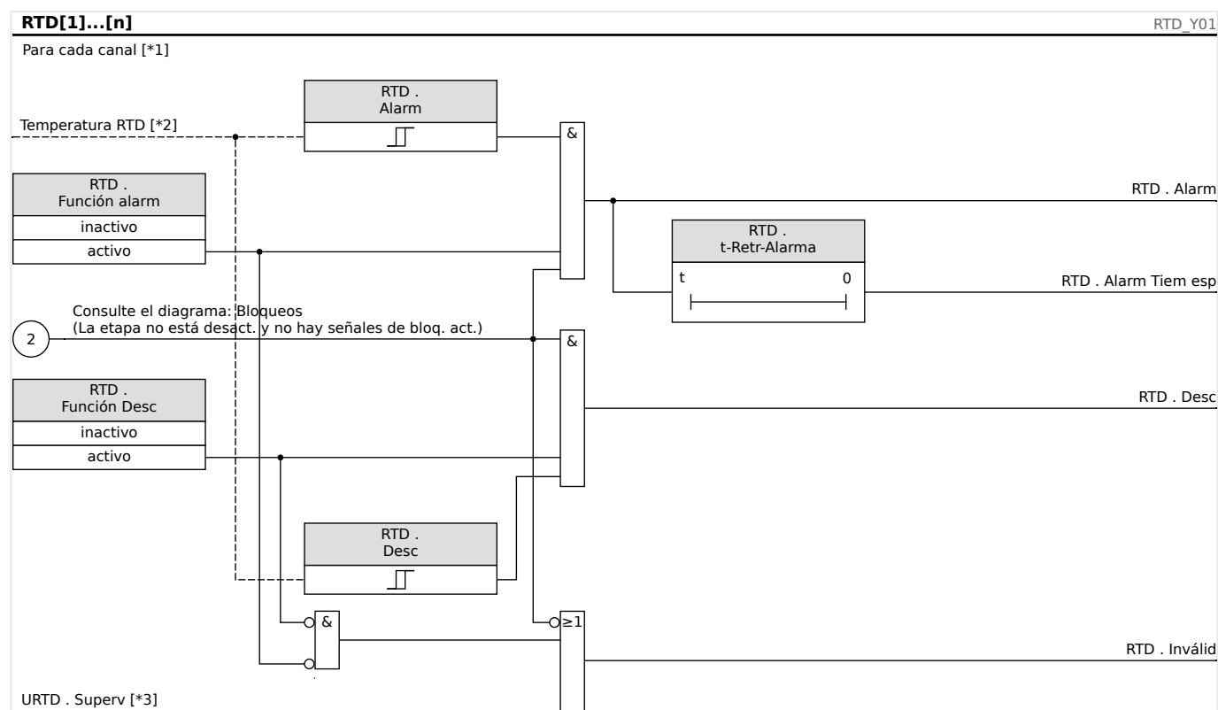
Fig. 150: El principio de funcionamiento general (alarma retrasada, desconexión sin retraso).
