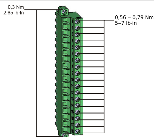
Fig. 155: Bornes de mesure de tension des cartes de mesure « TU-OR5 » et « TU-DI8 ».
