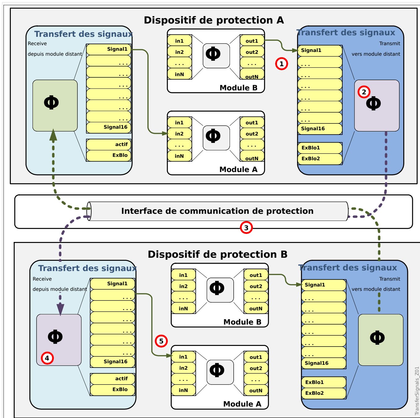
Fig. 84: Principe de la fonctionnalité «Sig-Trans».
