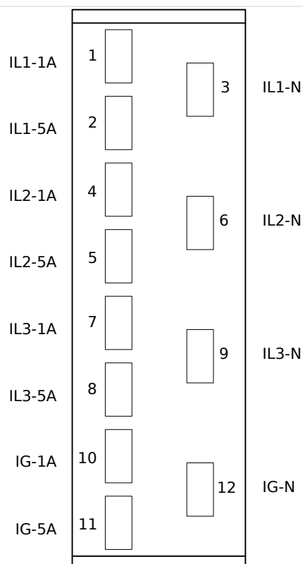
Fig. 16: TI - Affectation électromécanique
