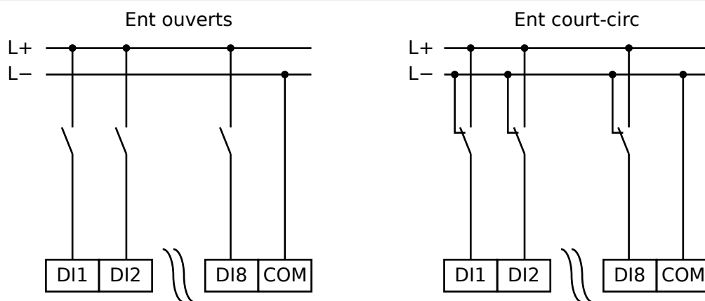
Fig. 156: État sécuritaire des entrées numériques
