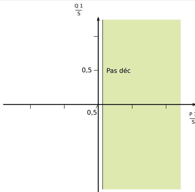
Fig. 124: Méthode 2 (Surveillance de la puissance active pure) : »Méthode UFLS« = "Surveillance de la puissance active pure".
