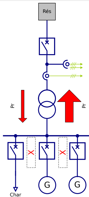
Fig. 122: Utilisation décentralisée au sein de réseaux avec alimentation prédominante.
