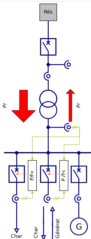
Fig. 120: Délestage de charge de sous-fréquence décentralisé au sein de réseaux avec alimentation temporaire.
