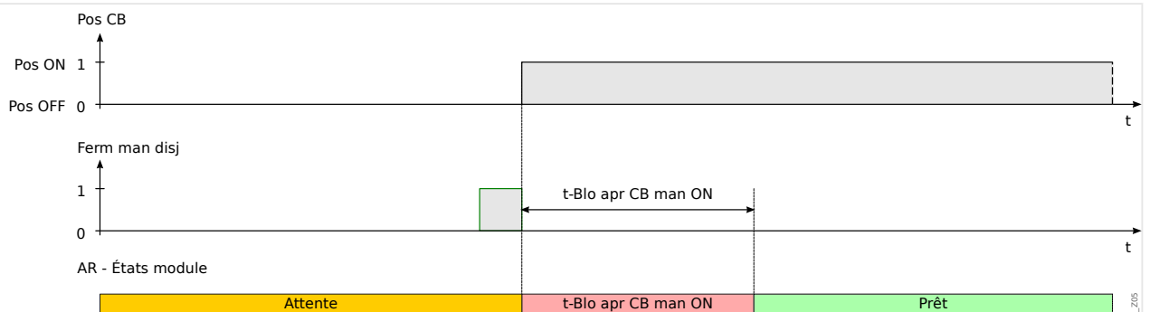
Fig. 96: États du réenclenchement automatique pendant la fermeture manuelle du disjoncteur.
