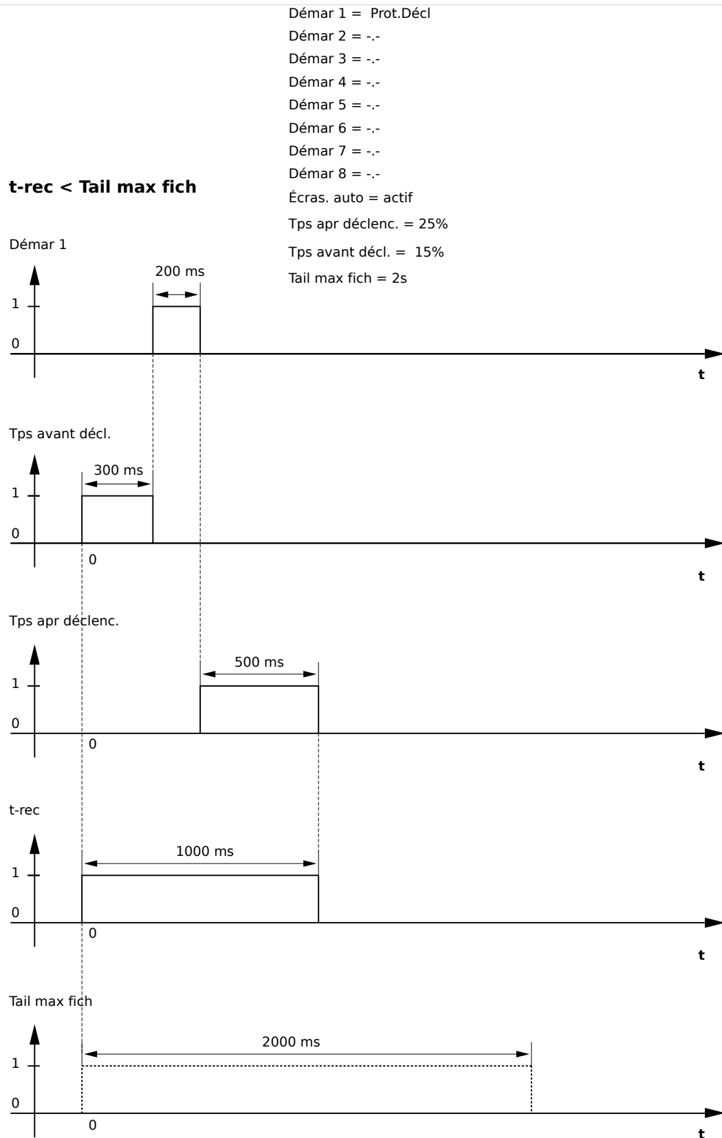
Fig. 144: Exemple de diagramme des temps de l'enregistreur de perturbations II
