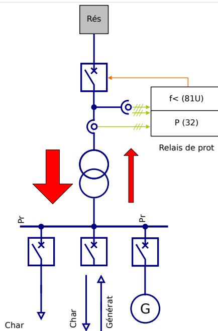
Fig. 119: Délestage de charge de sous-fréquence centralisé au sein de réseaux avec alimentation temporaire.
