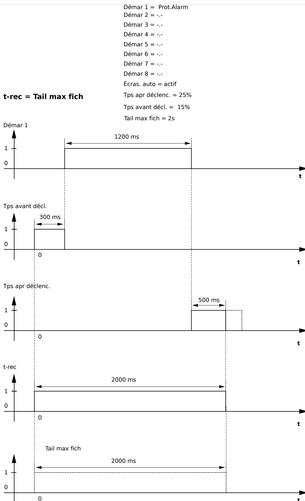
Fig. 143: Exemple de diagramme des temps de l'enregistreur de perturbations I
