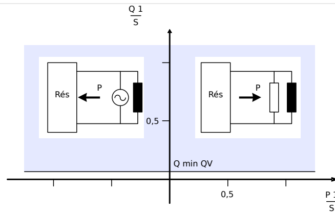
Fig. 116: Méthode 2 : Surveillance de la puissance réactive pure
