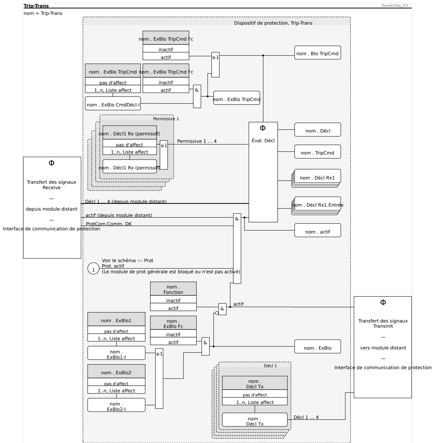
Fig. 82: Fonctionnalité du module »Trip-Trans«. La sous-routine « Éval. Décl » est détaillée dans le schéma suivant.
