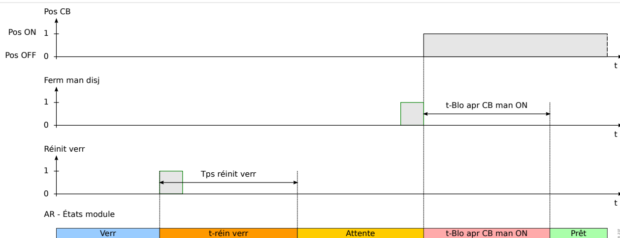
Fig. 98: Logique de réinitialisation du verrouillage du réenclenchement automatique si la réinitialisation du verrouillage se produit avant la fermeture du disjoncteur manuelle.
