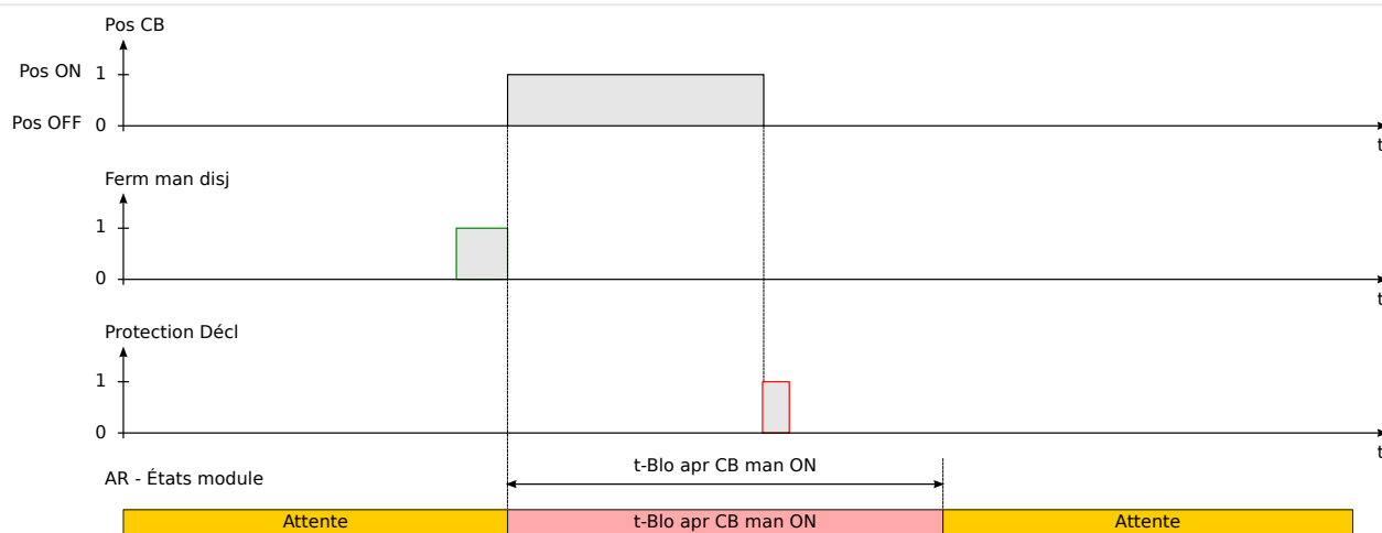
Fig. 97: Déclenchement de la protection pendant l'écoulement de la temporisation du blocage de fermeture manuelle.
