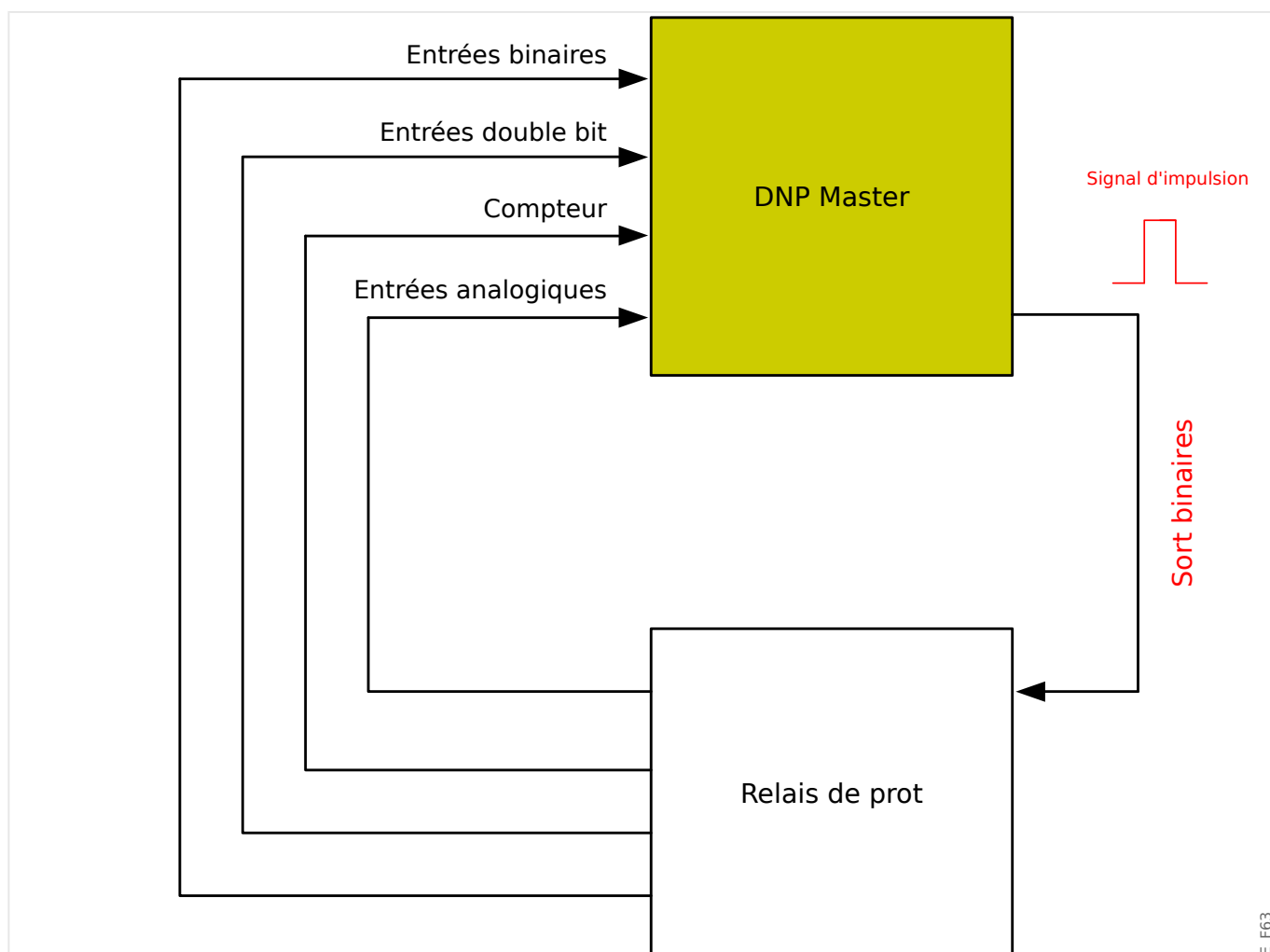
Fig. 58: Cartographie des points
