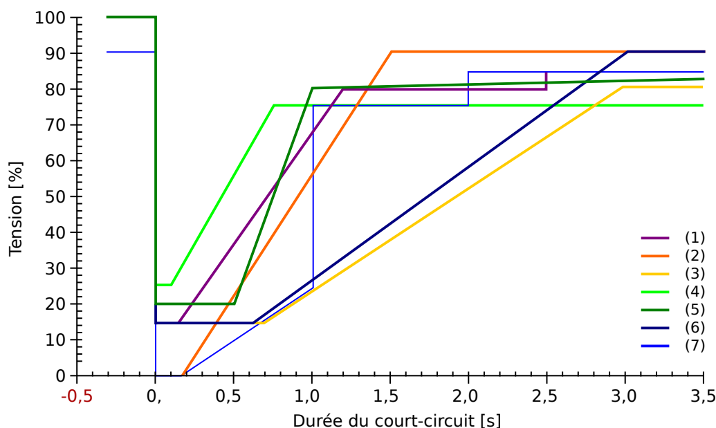
Fig. 125: Normes LVRT ; source : eBWK Bd. 60 (2008) N° 4. Auteurs: Dipl.-Ing. Thomas Smolka, Dr.-Ing. Karl-Heinz Weck, Zertifizierungstelle der FGH e.V., Mannheim, sowie Dipl.-Ing. (FH) Matthias Bartsch, Enercon GmbH, Aurich.
