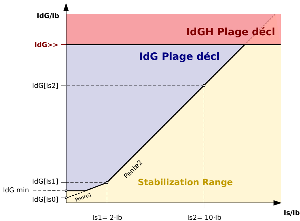
Fig. 81: Valeur d'excitation »IdG>>« du courant différentiel à la terre en fonction du courant nominal »Ib« de l'objet de protection associé.
