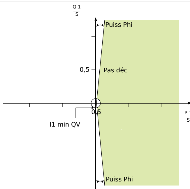
Fig. 123: Méthode 1 (Surveillance de l'angle de charge) : «Méthode UFLS» = "Surveillance de l'angle de charge".
