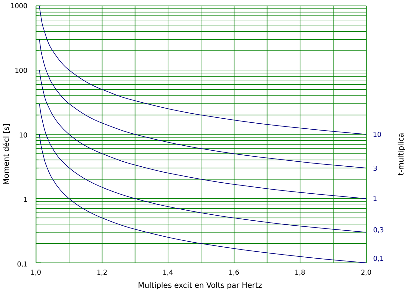
Fig. 89: Caractéristiques / forme de la courbe : INV B
