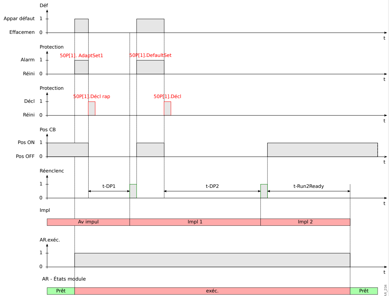
Fig. 95: Diagramme de temporisation de réenclenchement automatique pour un schéma de réenclenchement automatique à 2 impulsions réussi avec une accélération à la pré-impulsion.
