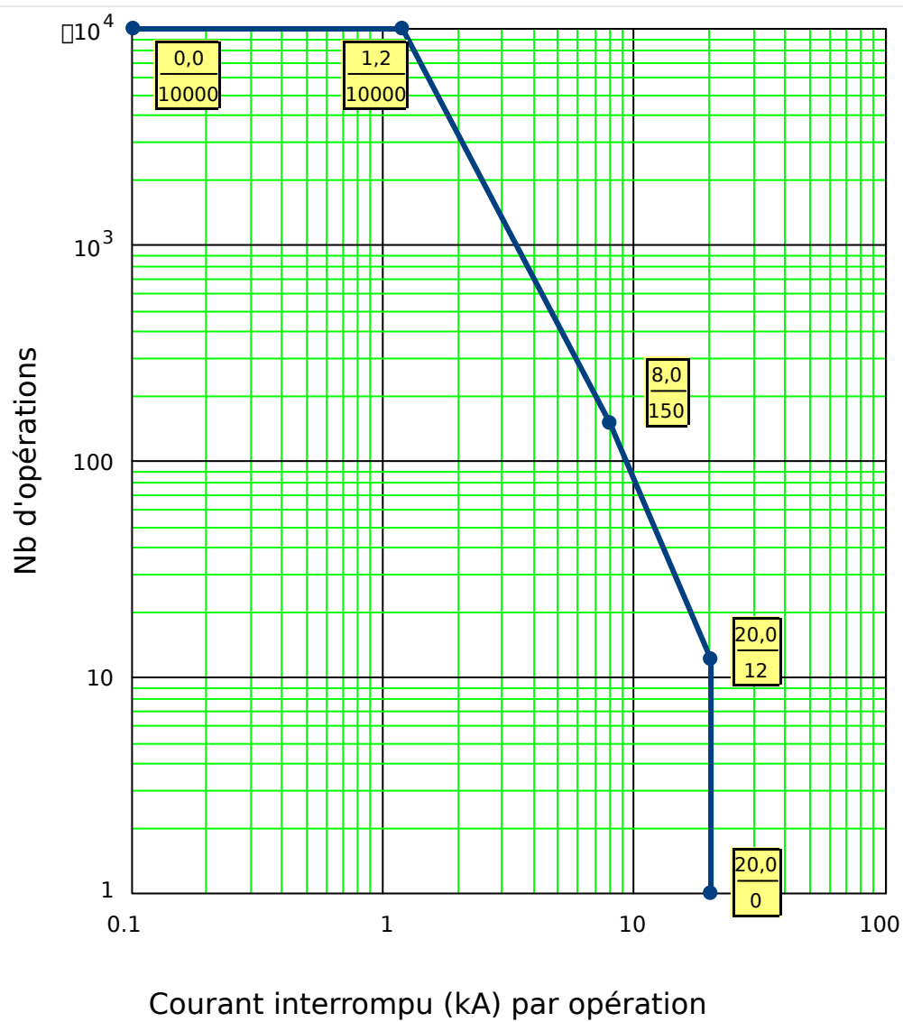
Fig. 140: Courbe de maintenance du disj pour un disj 25 ~kV typique
