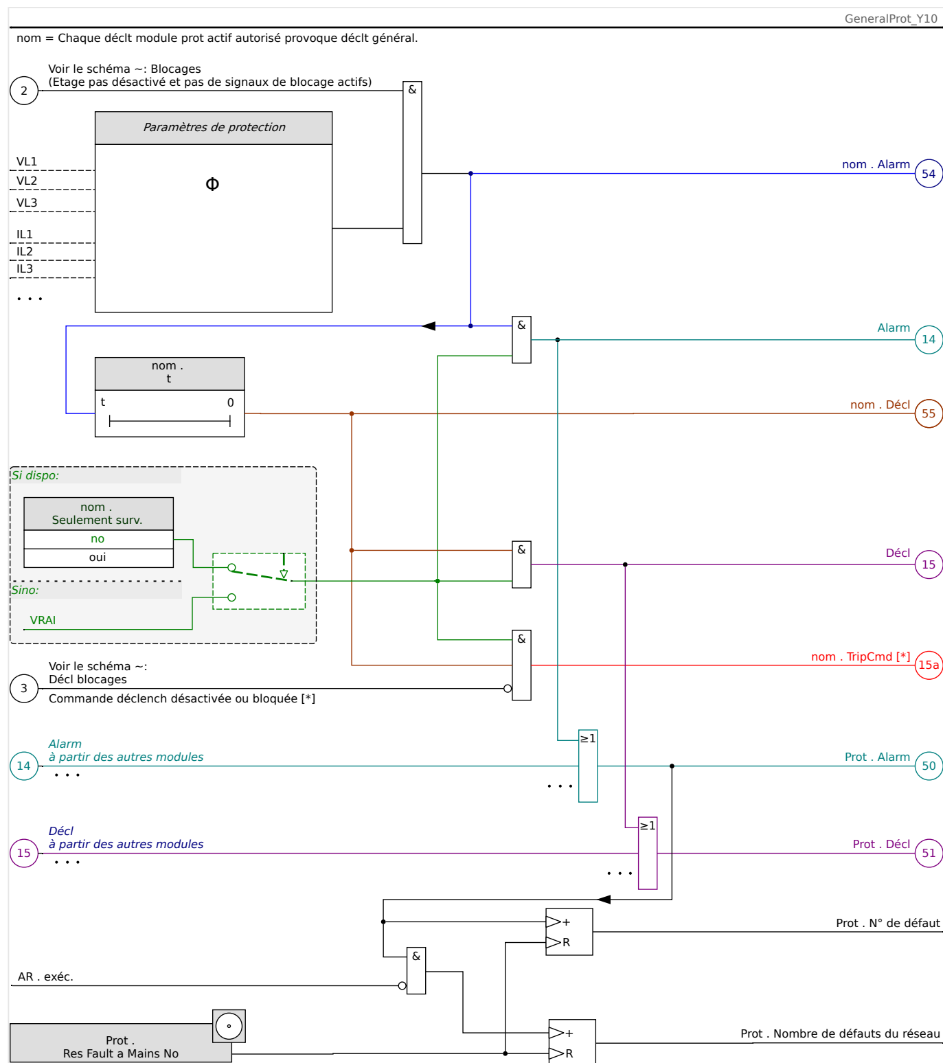
Fig. 63: Schéma de fonctionnalité des éléments de protection HighPROTEC.
