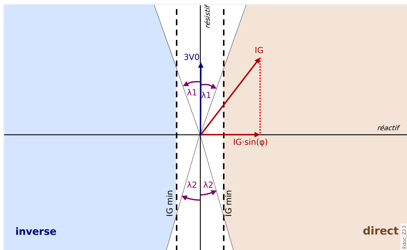
Fig. 69: Principe de détermination de la direction pour la méthode « \sin(\phi) ».
