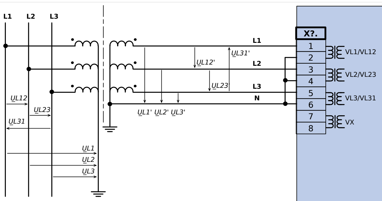
Fig. 30: VT Wye : Mesure de tension triphasée - câblage des entrées de mesure: "connex étoile"
