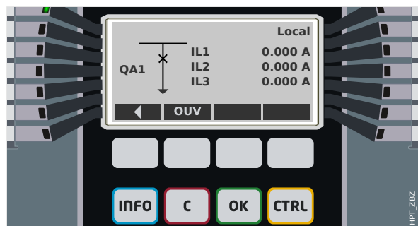
Fig. 135: Exemple de page de contrôle, avec le « disjoncteur » en position fermée.
