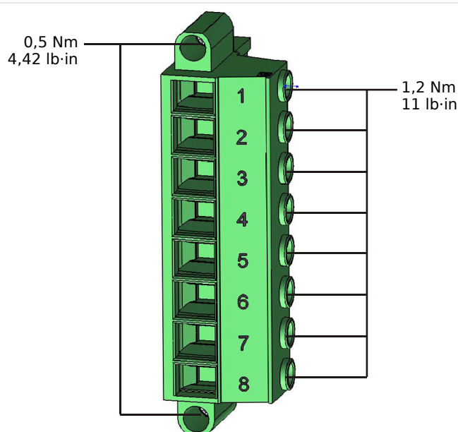
Fig. 154: Bornes de mesure de tension de la carte de mesure « TU » (➡ « 2.6.1 TU - Entrées de mesure de tension »).
