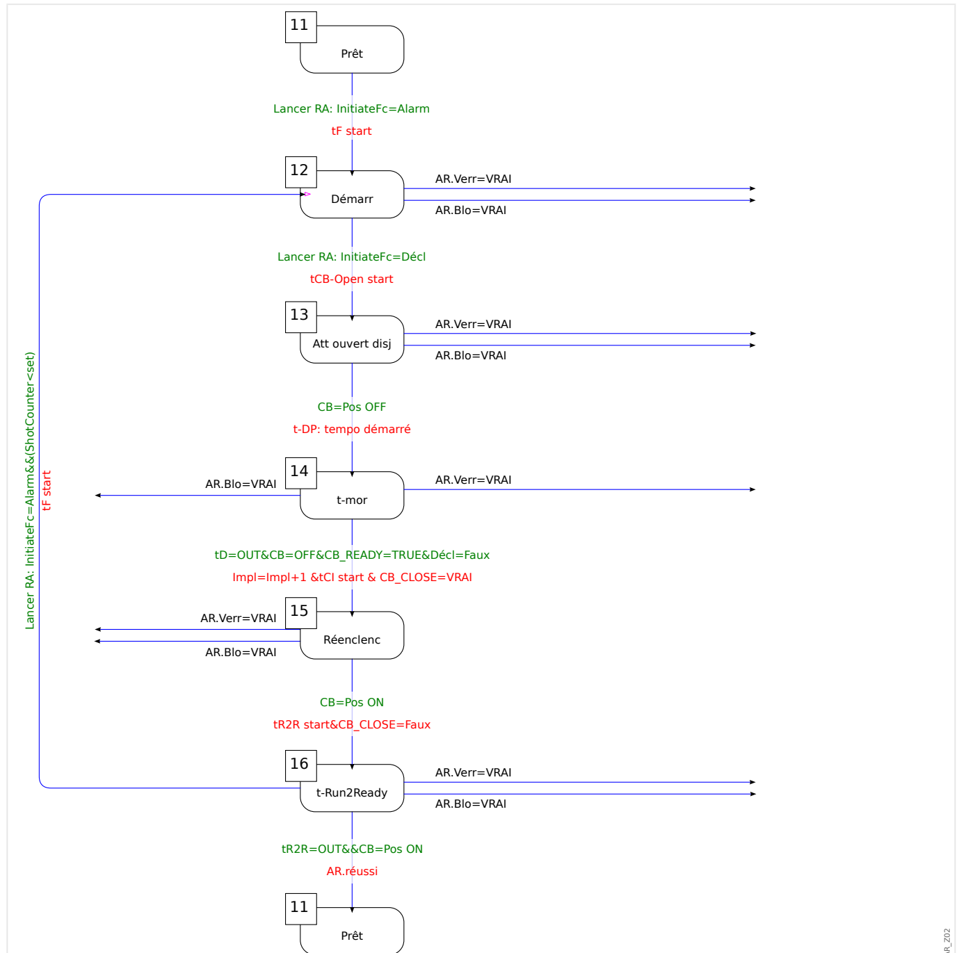
Fig. 93: Cycle d'exécution du AR (état 4).
