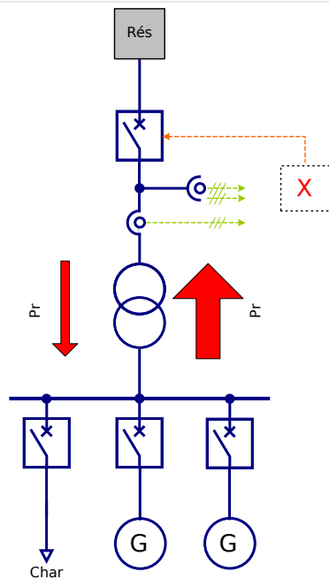
Fig. 121: Utilisation centralisée au sein de réseaux avec alimentation prédominante.
