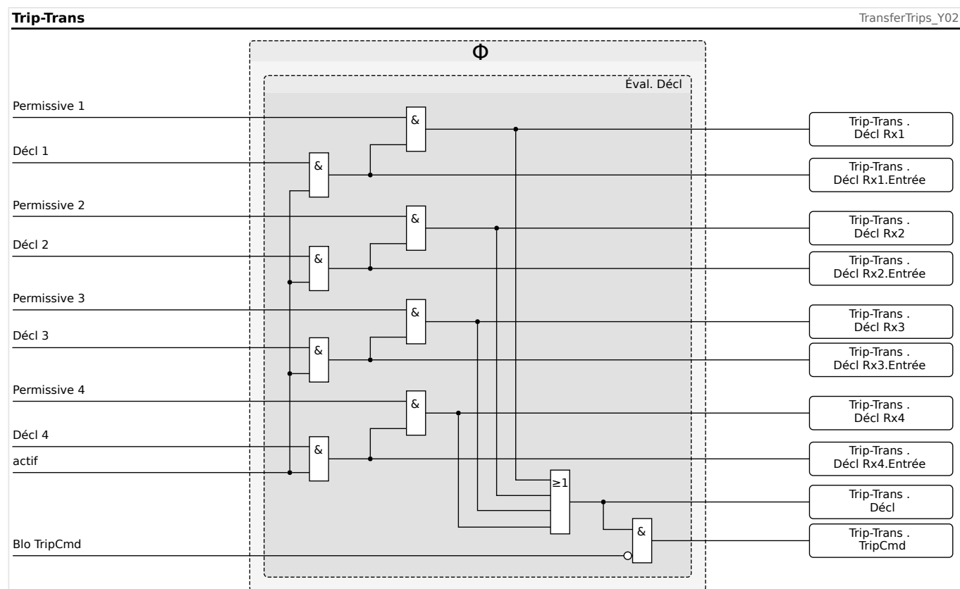
Fig. 83: Fonctionnalité du module »Trip-Trans« (partie 2).
