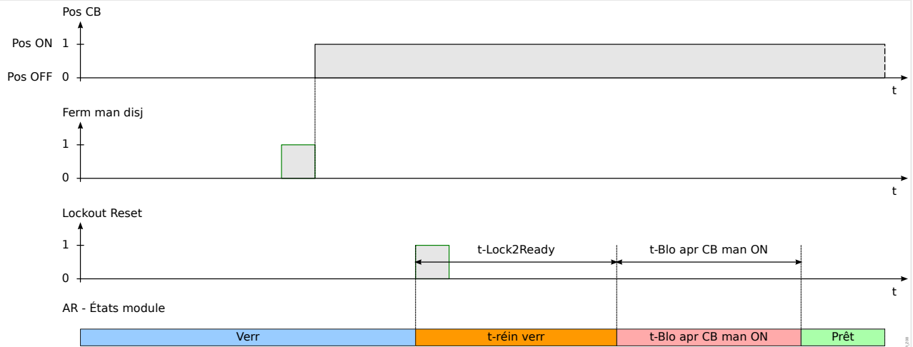
Fig. 99: Logique de réinitialisation du verrouillage du réenclenchement automatique si la réinitialisation du verrouillage se produit après la fermeture du disjoncteur manuelle.
