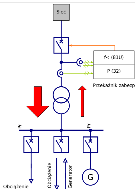
Rys. 119: Scentralizowane podczęstotliwościowe zmniejszanie obciążenia w sieciach z tymczasowym zasilaniem.
