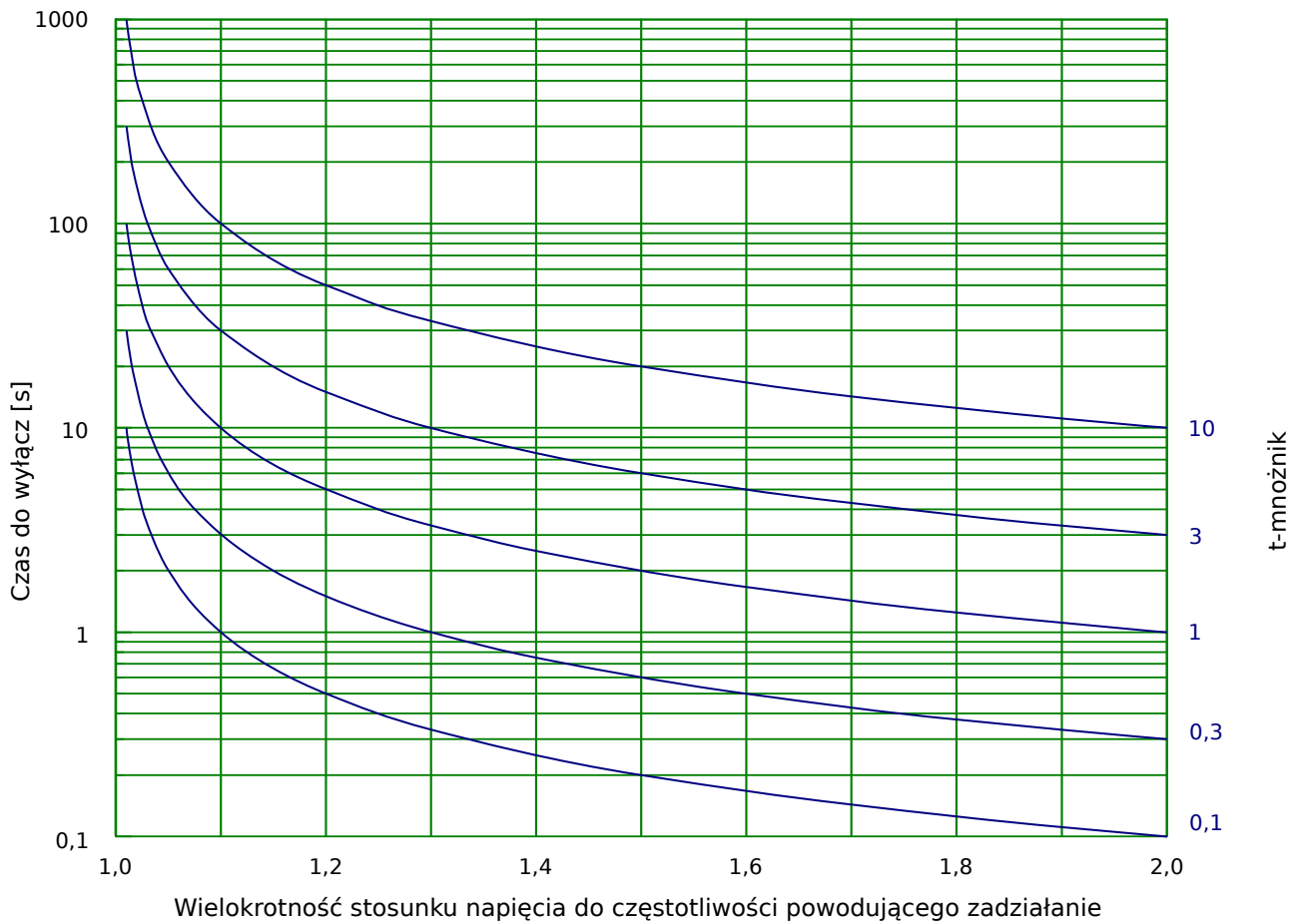
Rys. 89: Kształt krzywej/charakterystyki: ODW B
