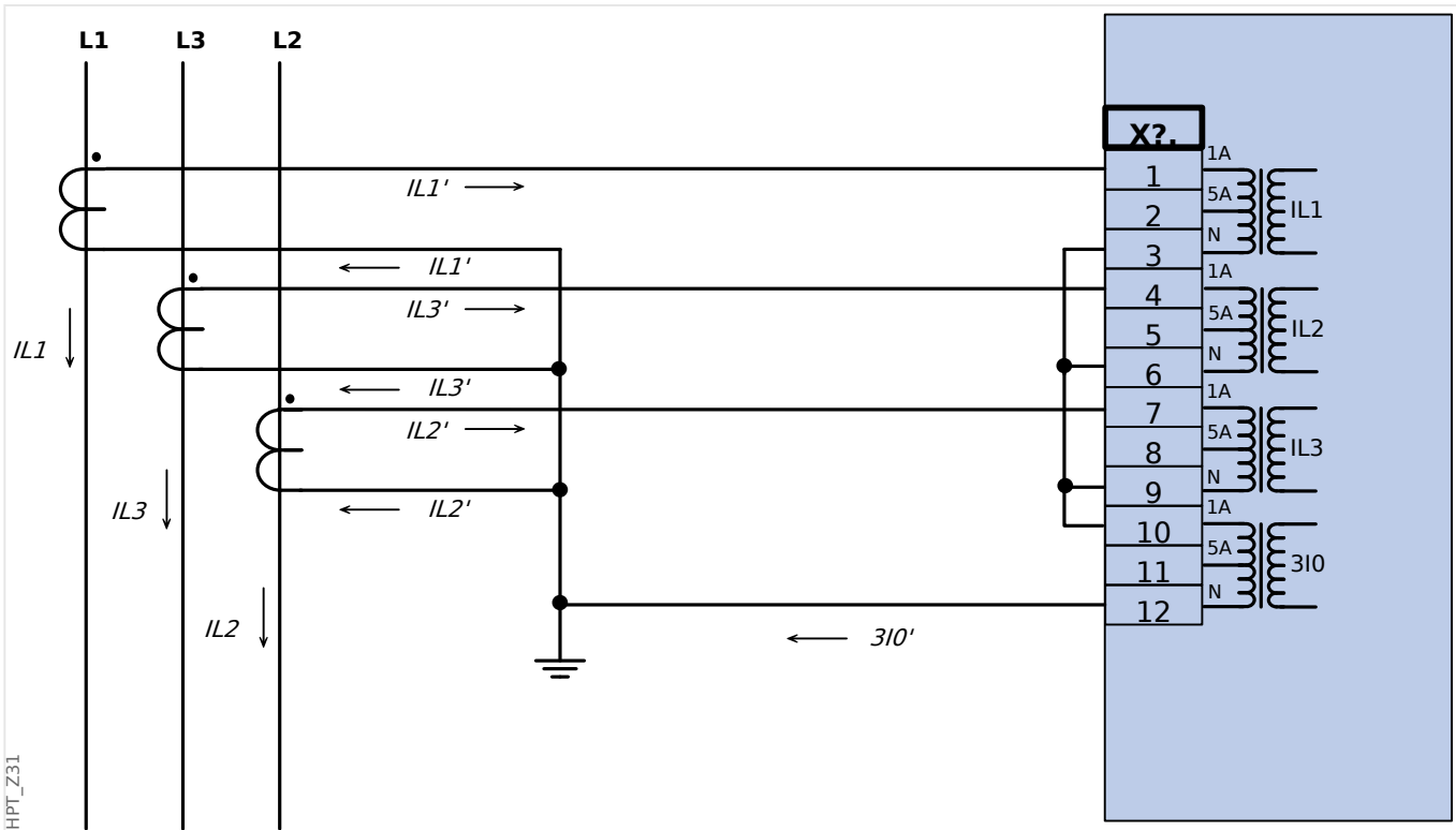
Rys. 24: Trójfazowy pomiar prądu; I_n wtórny = 1 A. Pomiar prądu doziemnego w układzie Holmgreena 3I0n wtórny = 1 A.
