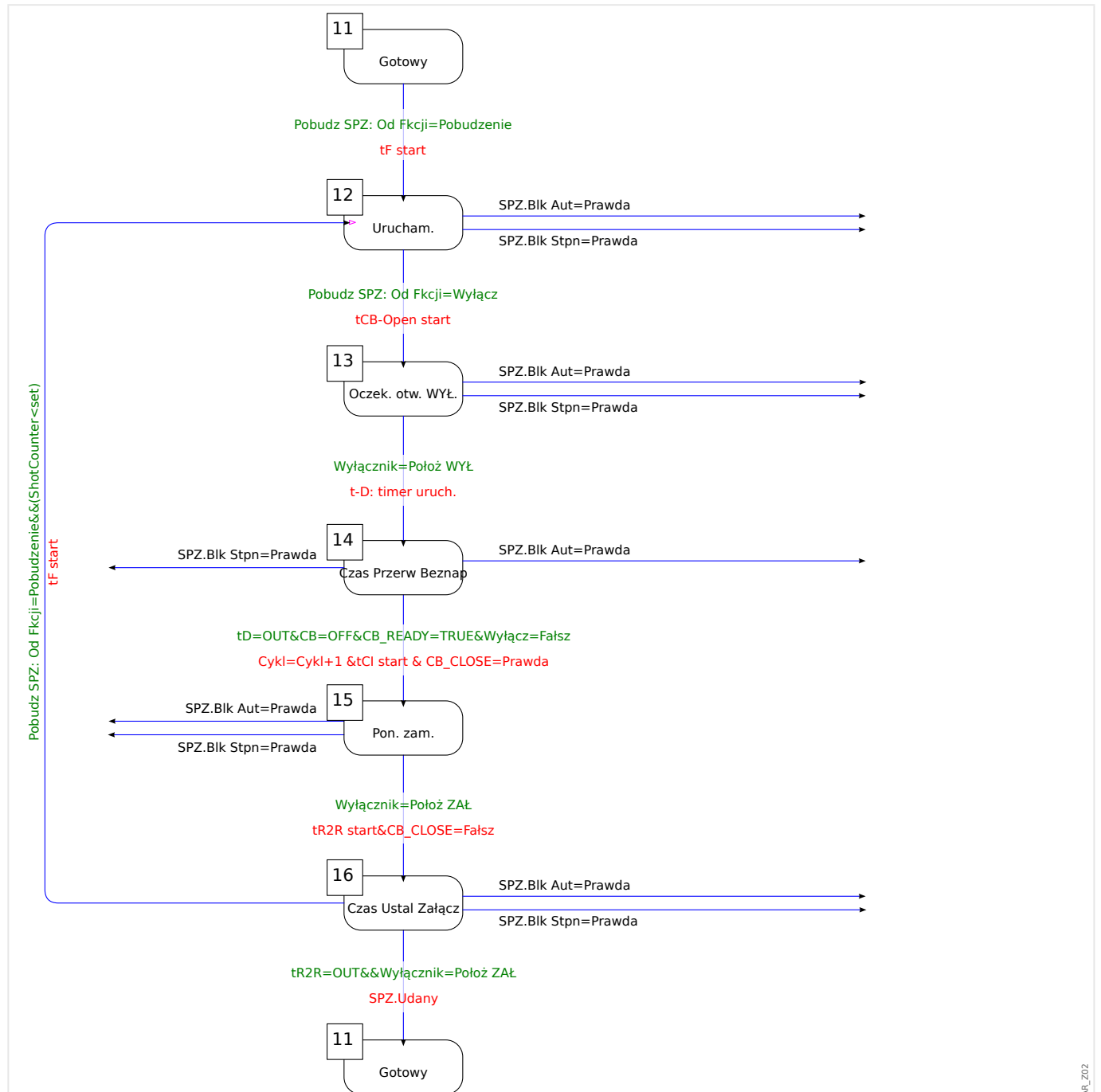
Rys. 93: Cykl pracy SPZ (stan 4).
