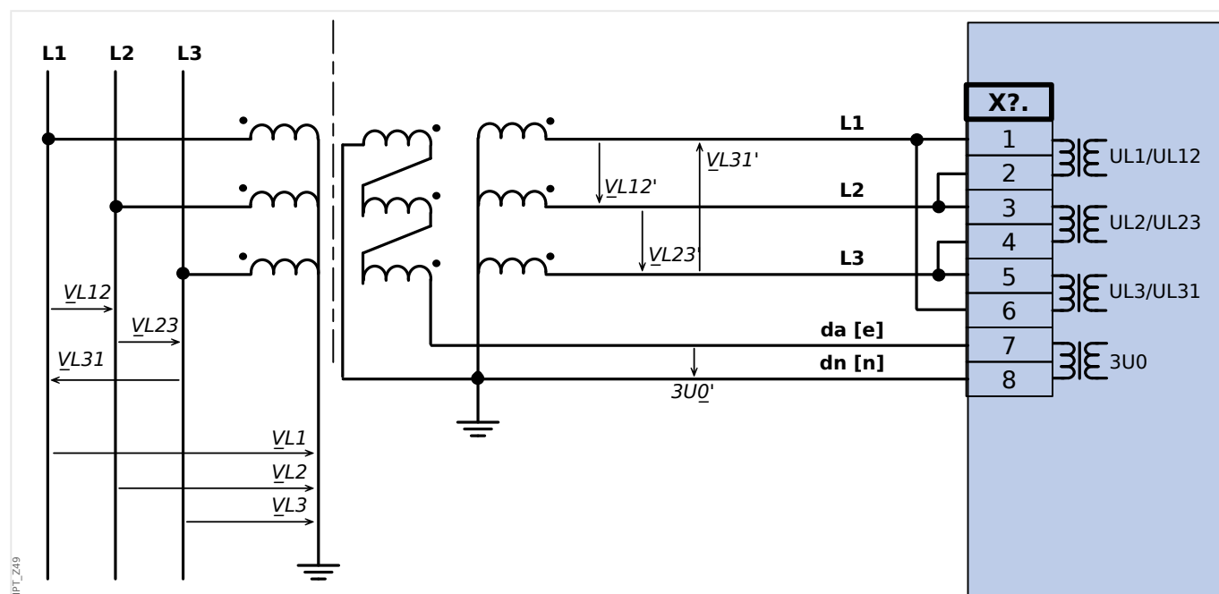
Rys. 33: Trójfazowy pomiar napięcia w układzie trójkąta: połączenie przewodów wejść pomiarowych: "połączenie w trójkąt" Pomiar 3U_0 napięcia szcztkowego poprzez dodatkowe uzwojenia (e-n) w układzie otwartego trójkąta
