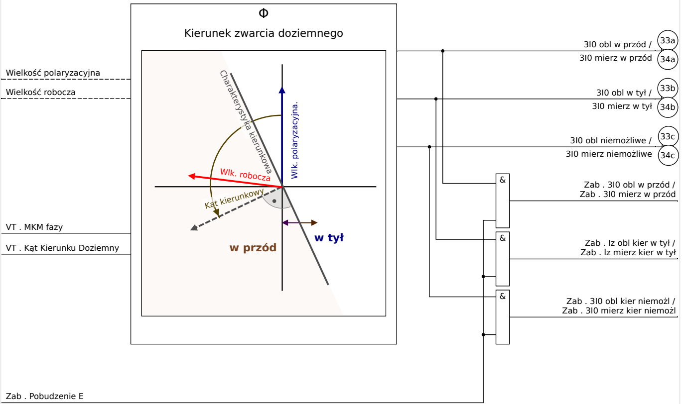
Rys. 67: Zasada określania kierunku obowiązująca dla wszystkich metod z wyjątkiem „ \cos(\phi) ”, „ \sin(\phi) ”.
