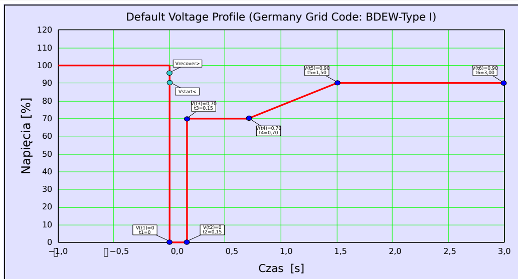
Rys. 128: Profil domyślny LVRT (BDEW typ I).
