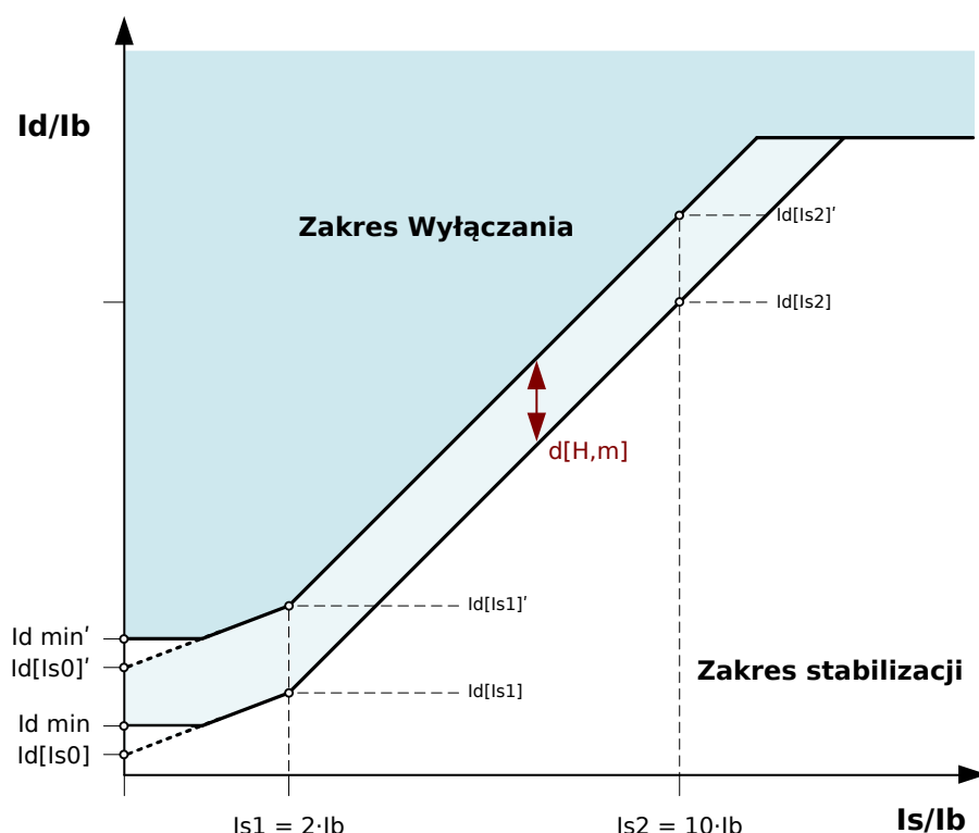
Rys. 77: Tymczasowe podniesienie dynamiczne charakterystyki wyzwania statycznego.
