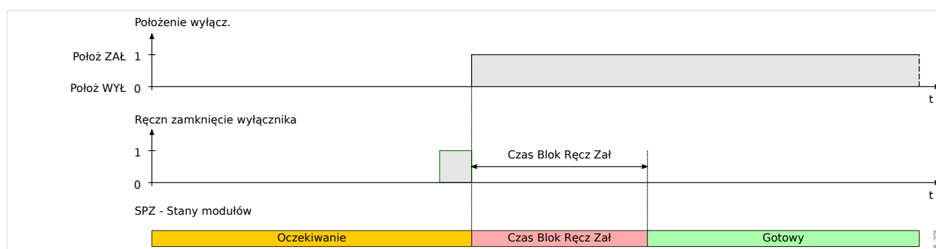
Rys. 96: Stany SPZ podczas ręcznego zamykania wyłącznika.
