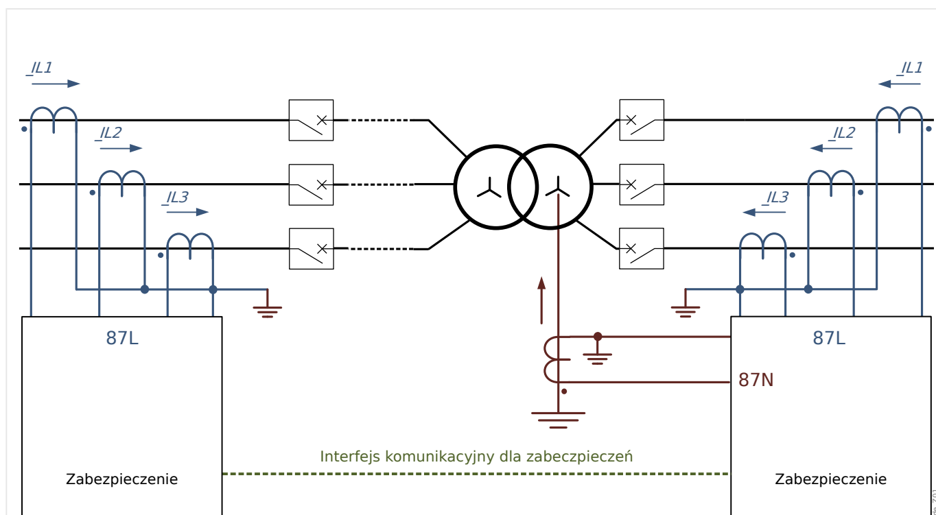
Rys. 80: Zasada działania zabezpieczenia różnicowego ziemnozwarciowego
