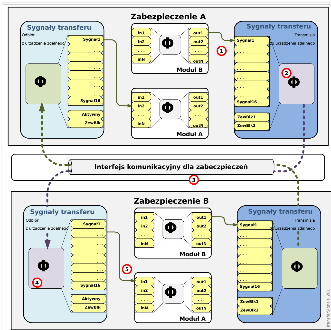
Rys. 84: Zasada działania modułu „Transfer sygnału”.
