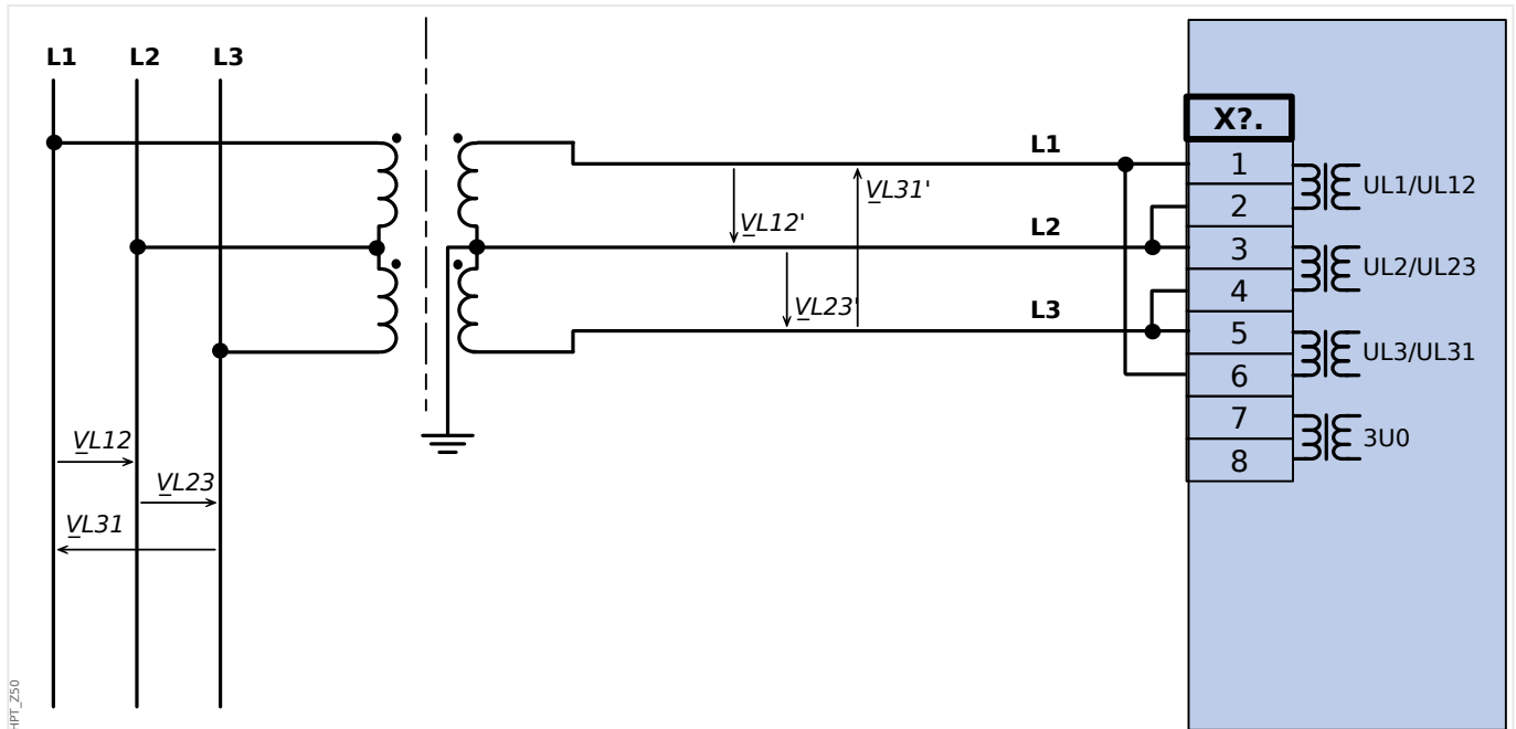
Rys. 34: Pomiar napięcia dla dwóch faz w układzie otwartego trójkąta
