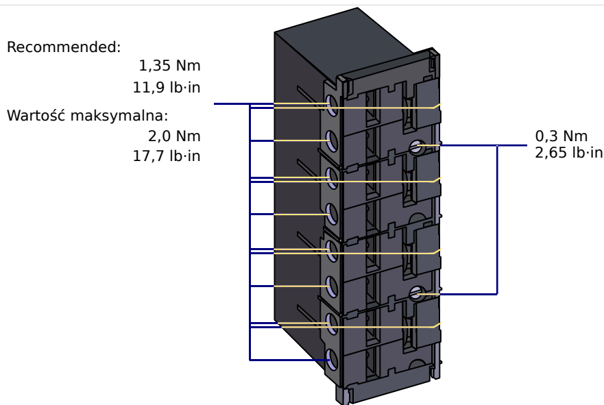
Rys. 153: Łącznik wtykowy ze zintegrowanym elementem zwarciovym (konwencjonalne wejścia prądowe)
