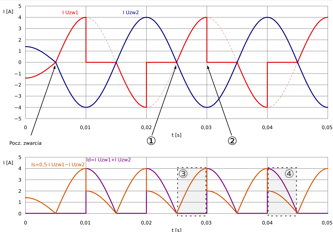
Rys. 78: Charakterystyka I_d i I_s z nasyceniem po stronie W1 przekładnika prądowego w przypadku zwarcia zewnętrznego.
