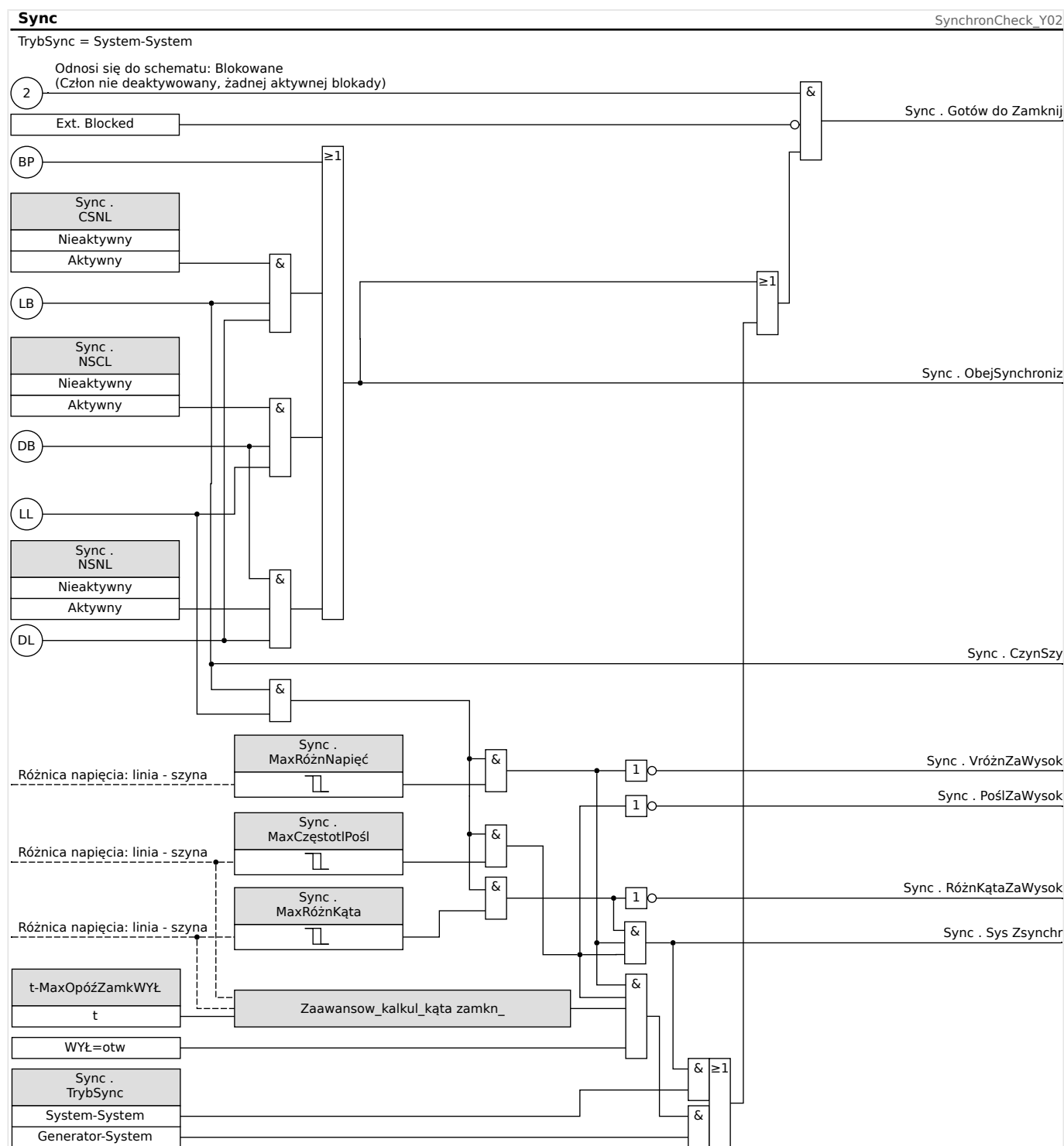
Rys. 113: Działanie modułu „Sync”, „System-System”.
