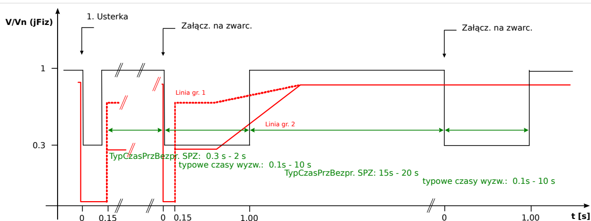
Rys. 126: Przebieg krzywej napięcia podczas nieudanego dwukrotnego SPZ; źródło: Technische Richtlinien, Erzeugungsanlagen am Mittelspannungsnetz, Ausgabe Juni 2008, BDEW Bundesverband der Energie- und Wasserwirtschaft e.V. (strona 89).
