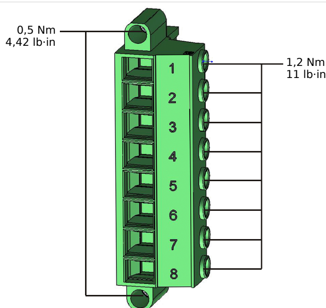
Rys. 154: Zaciski pomiaru napięcia karty pomiarowej „TU” (➡ „2.6.1 TU — wejścia do pomiaru napięcia”).
