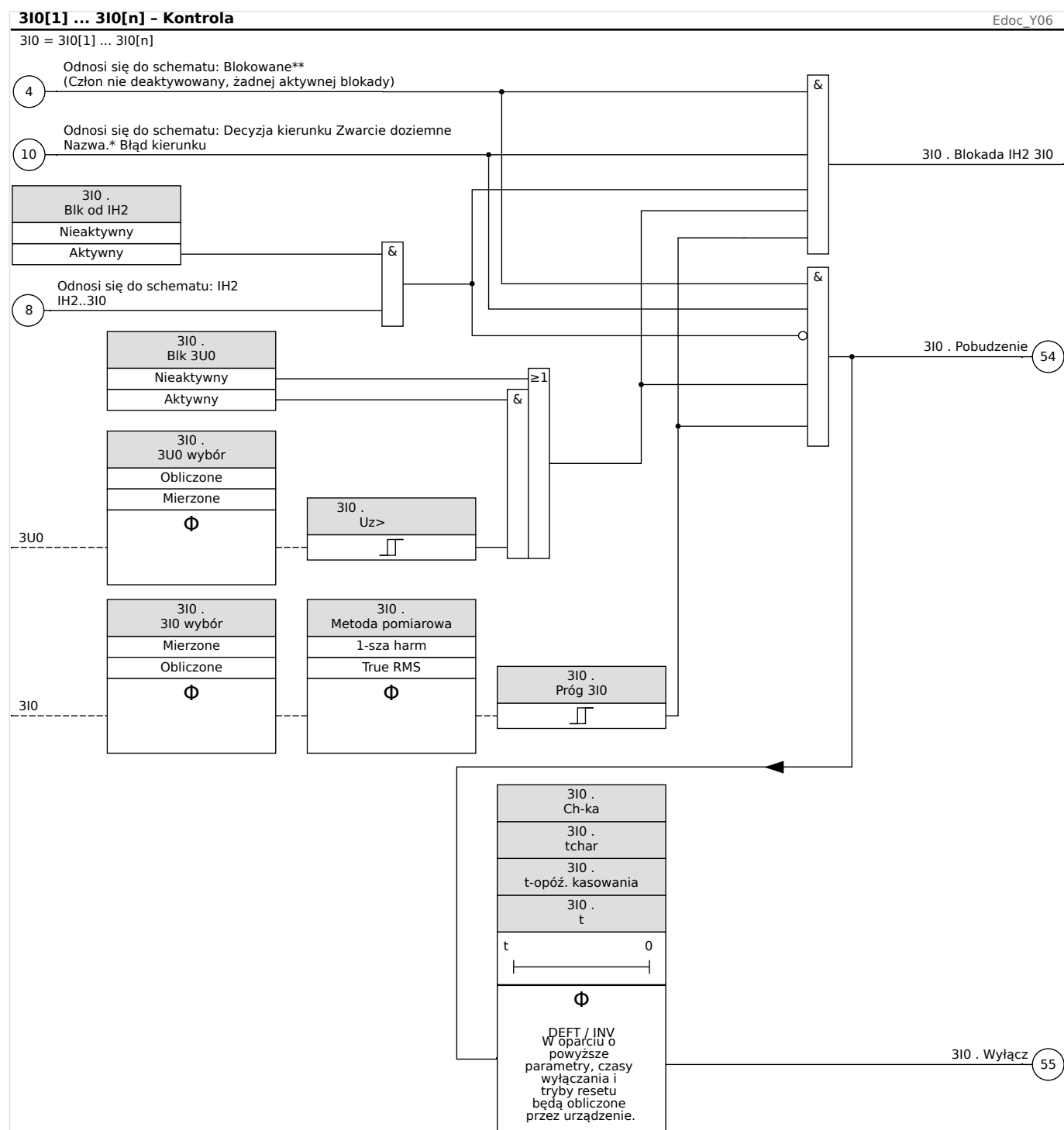
Rys. 85: Zabezpieczenie nadprądowe ziemnozwarciowe, część 1 (funkcja kontroli, decyzja o wyzwoleniu).
