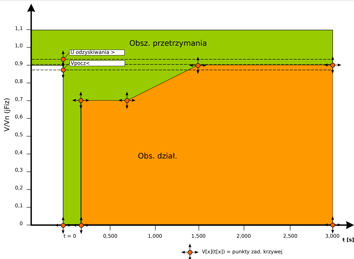
Rys. 127: Obszar „przetrzymania” i obszar „wyzwolenia”.
