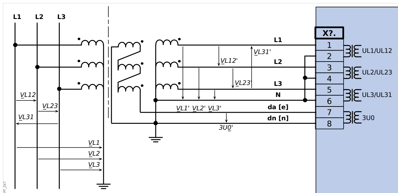
Rys. 31: Przekładnik napięciowy połączony w gwiazdę z otwartym trójkątem.
