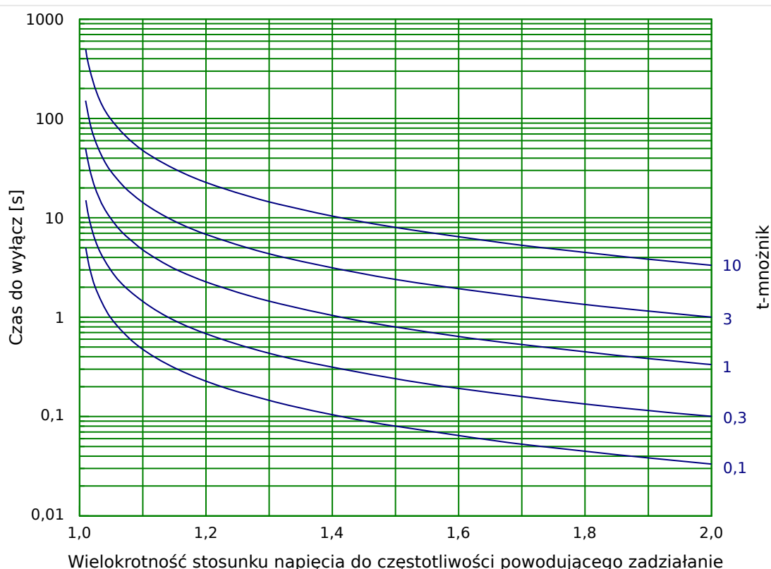
Rys. 88: Kształt krzywej/charakterystyki: ODW A
