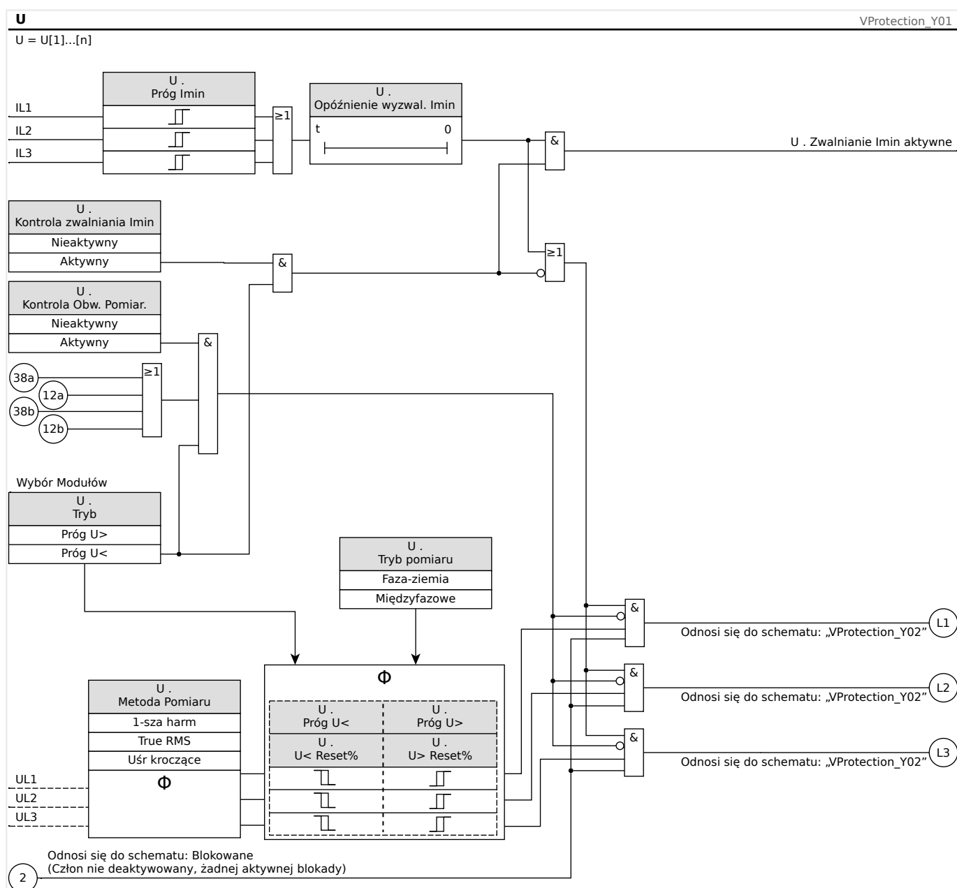
Rys. 100: Działanie modułu zabezpieczenia napięciowego, część 1.
