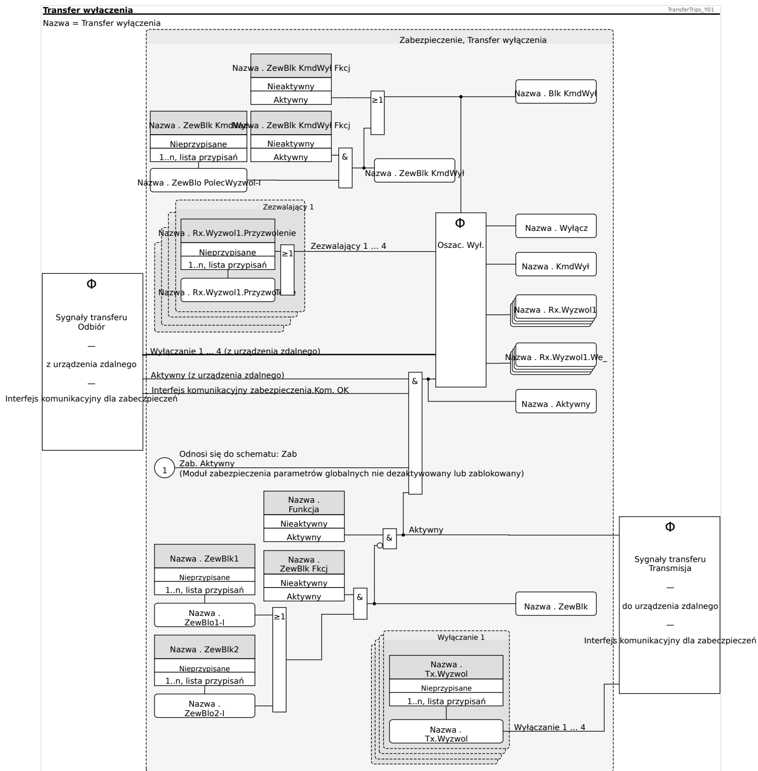
Rys. 82: Działanie modułu „Transfer wyłączenia”. Podprogram „Eval. Trip” szczegółowo przedstawiono na poniższym schemacie.
