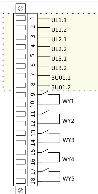
Rys. 29: Przypisanie elektromechaniczne
