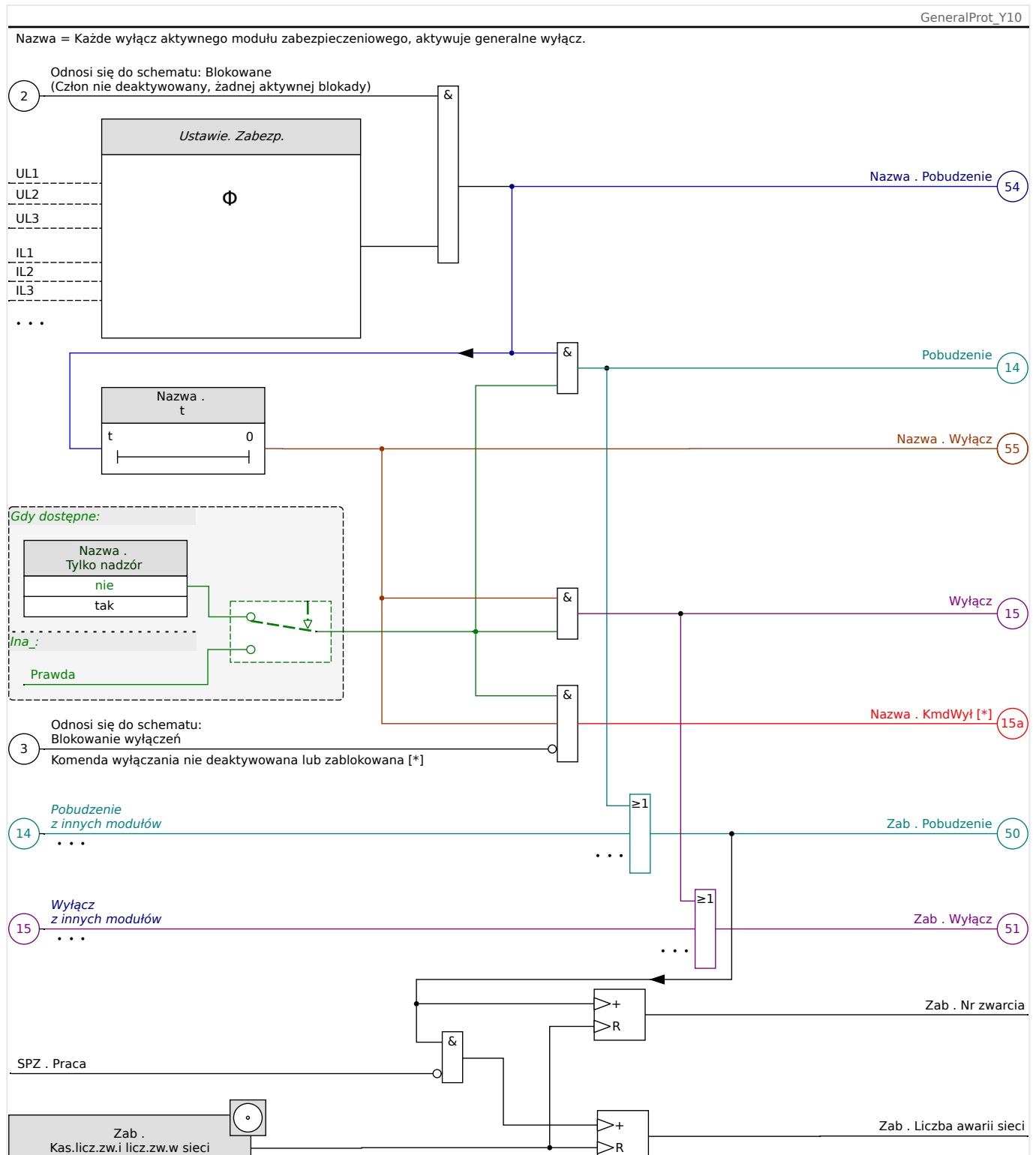
Rys. 63: Schemat ogólny działania każdego elementu zabezpieczającego HighPROTEC.
