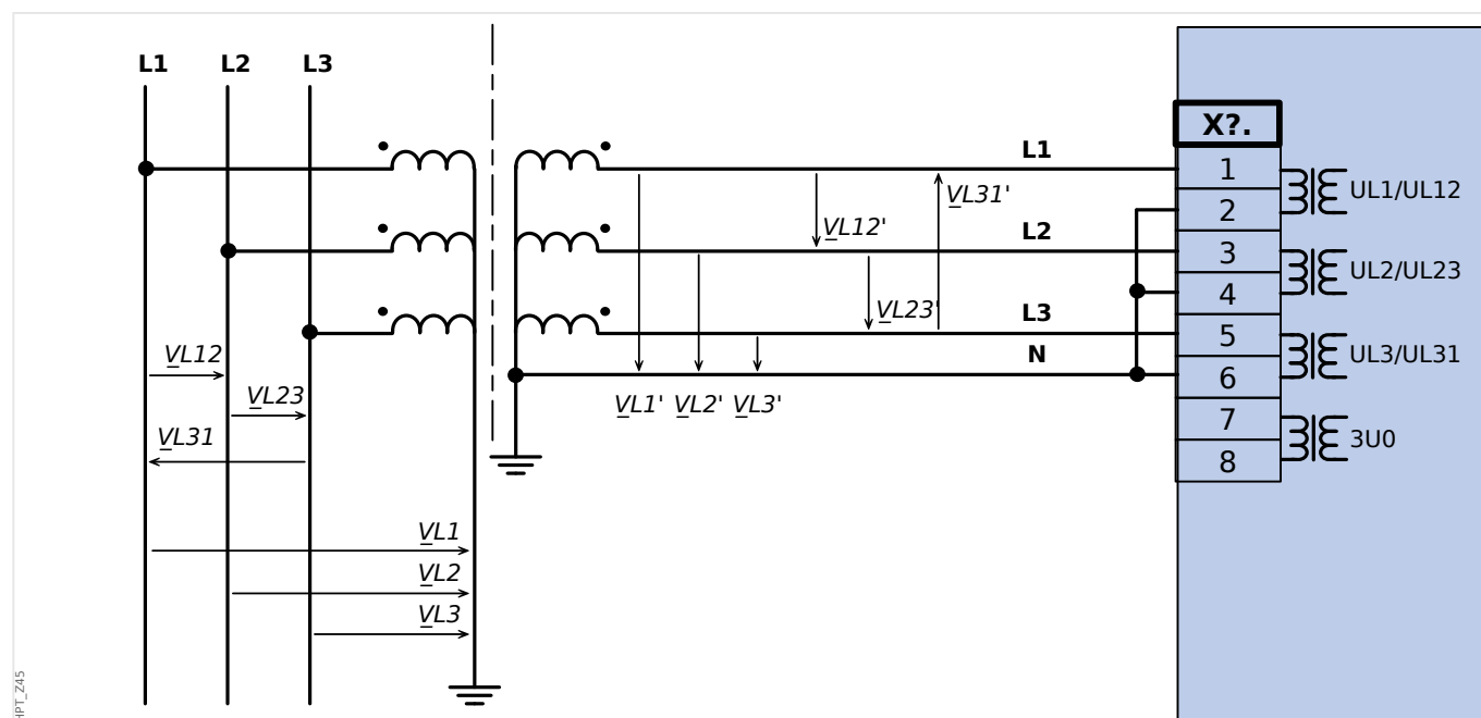
Rys. 30: Przekładnik napięciowy połączony w gwiazdę: Trójfazowy pomiar napięcia w układzie gwiazdy
