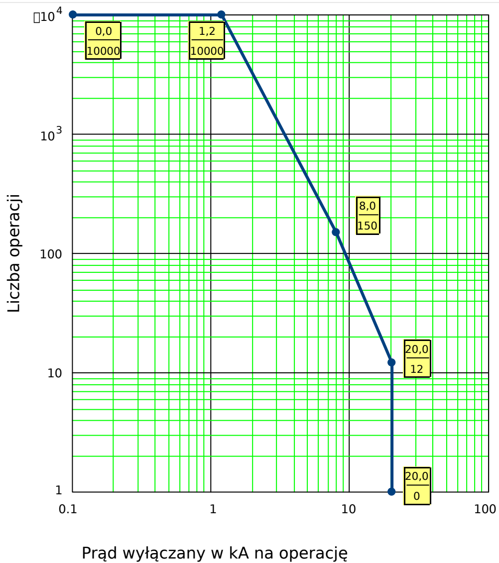
Rys. 140: Krzywa konserwacji wyłącznika typowego wyłącznika 25 kV
