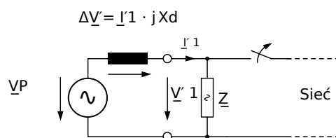
Rys. 106: Schemat zastępczy przy awarii sieci.
