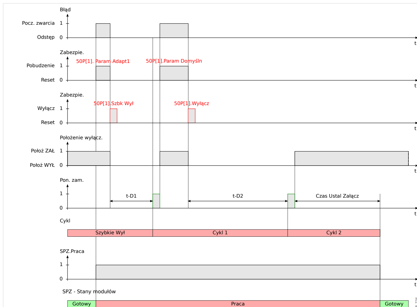
Rys. 95: Schemat czasów SPZ w przypadku udanego planu SPZ z 2 próbami i przyspieszeniem przy próbie wstępnej
