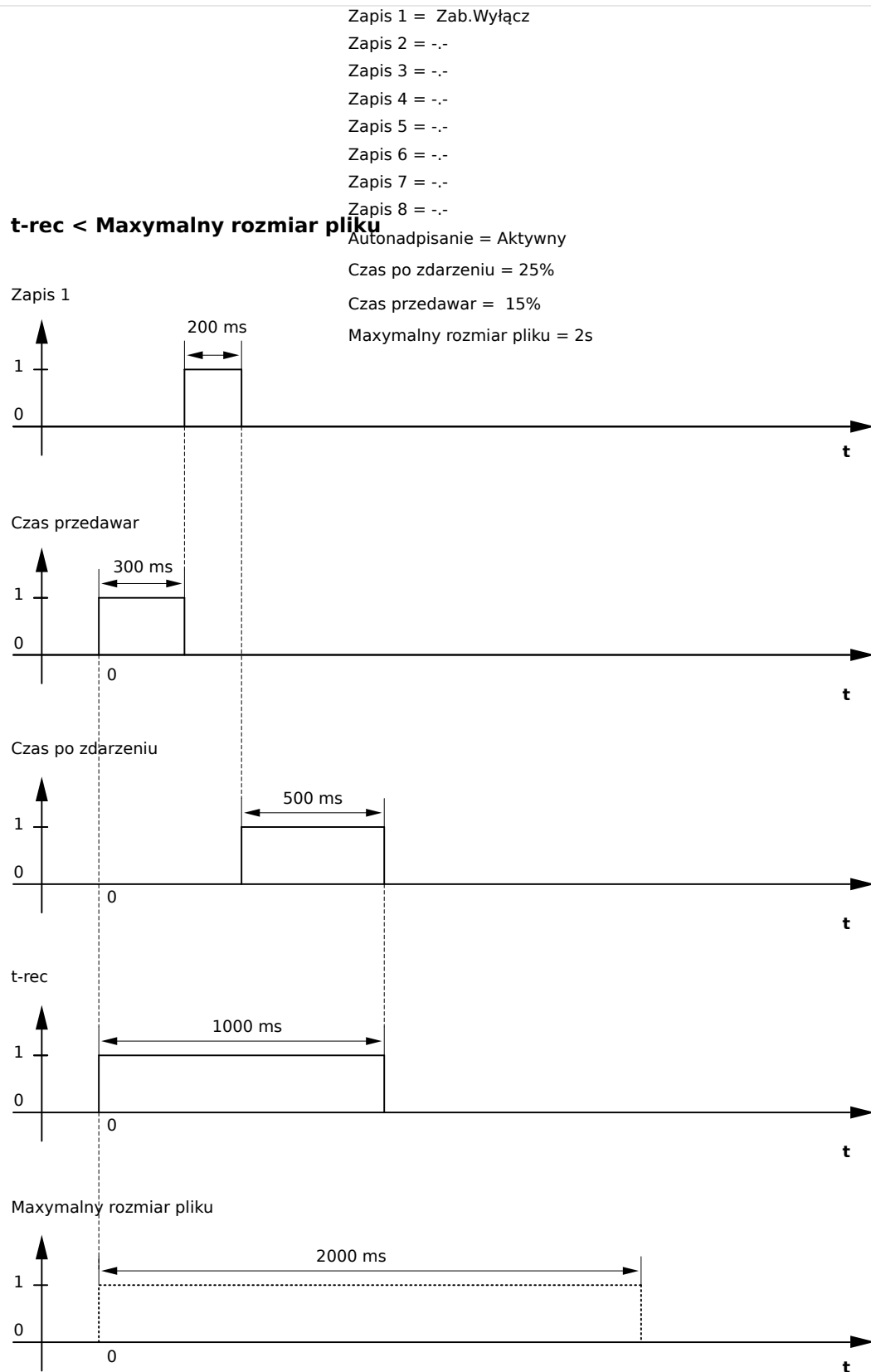
Rys. 144: Przykładowy wykres czasów pracy rejestratora zakłóceń II
