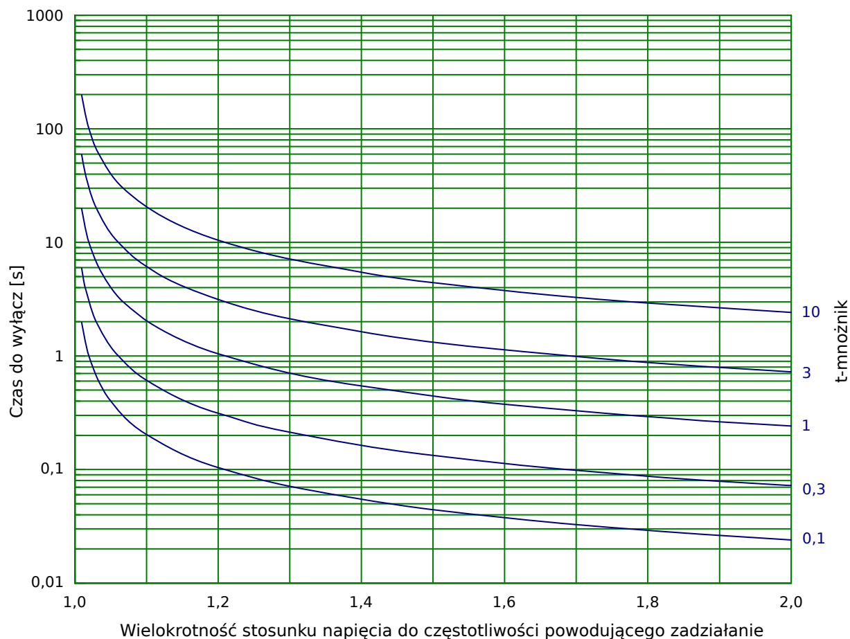
Rys. 90: Kształt krzywej/charakterystyki: ODW C
