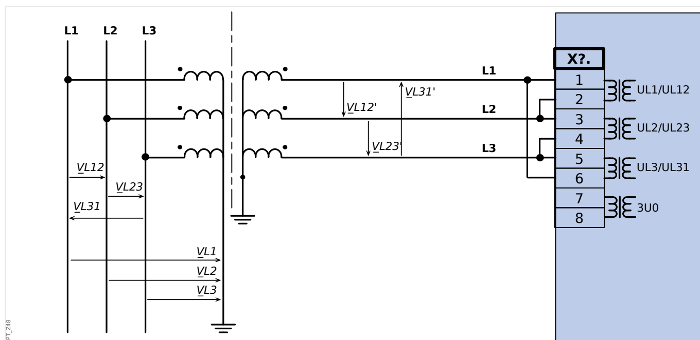
Rys. 32: Trójfazowy pomiar napięcia w układzie trójkąta: połączenie przewodów wejść pomiarowych: "połączenie w trójkąt"
