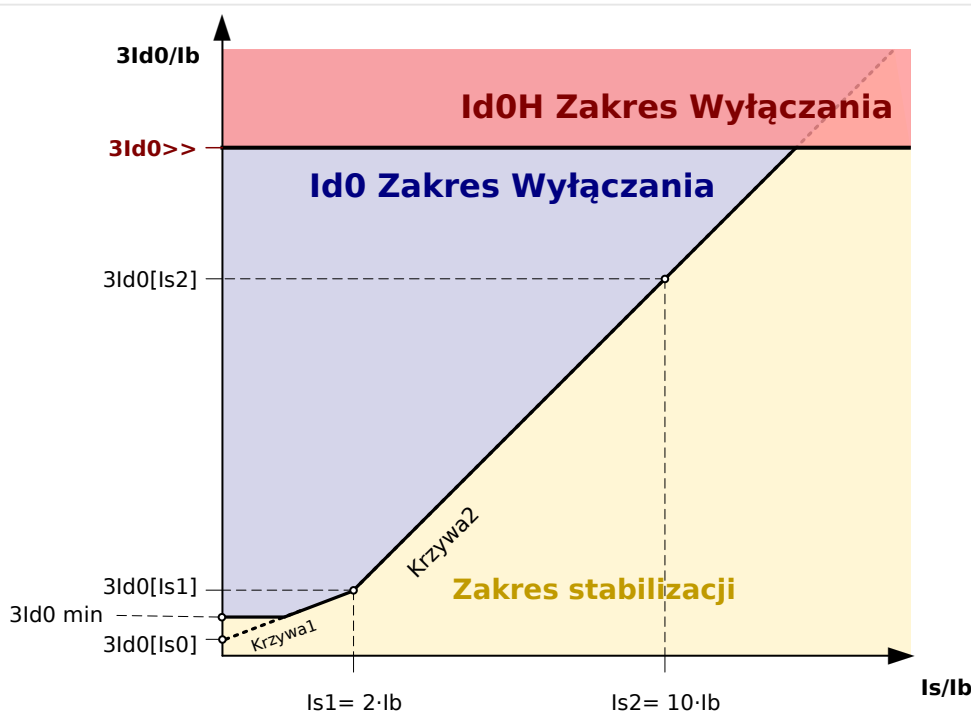
Rys. 81: Wartość pobudzenia „3Id0>>” prądu różnicowego doziemnego w oparciu o prąd znamionowy „Ib” obiektu zabezpieczanego.
