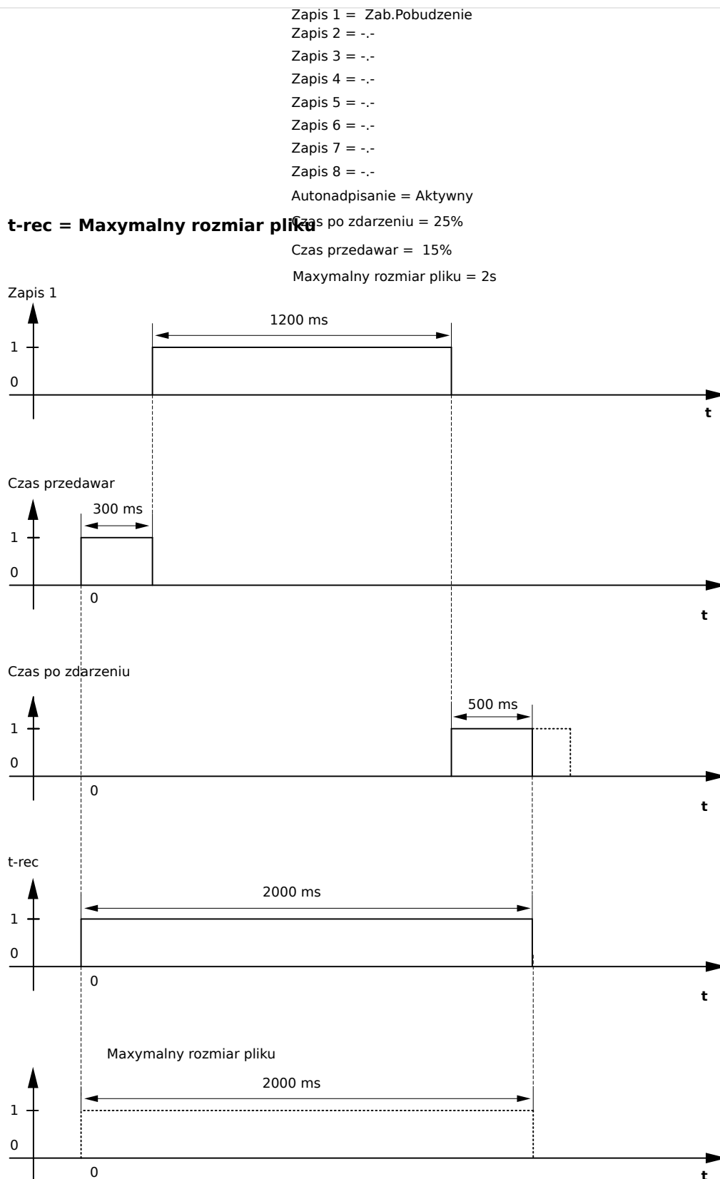
Rys. 143: Przykładowy wykres czasów pracy rejestratora zakłóceń I
