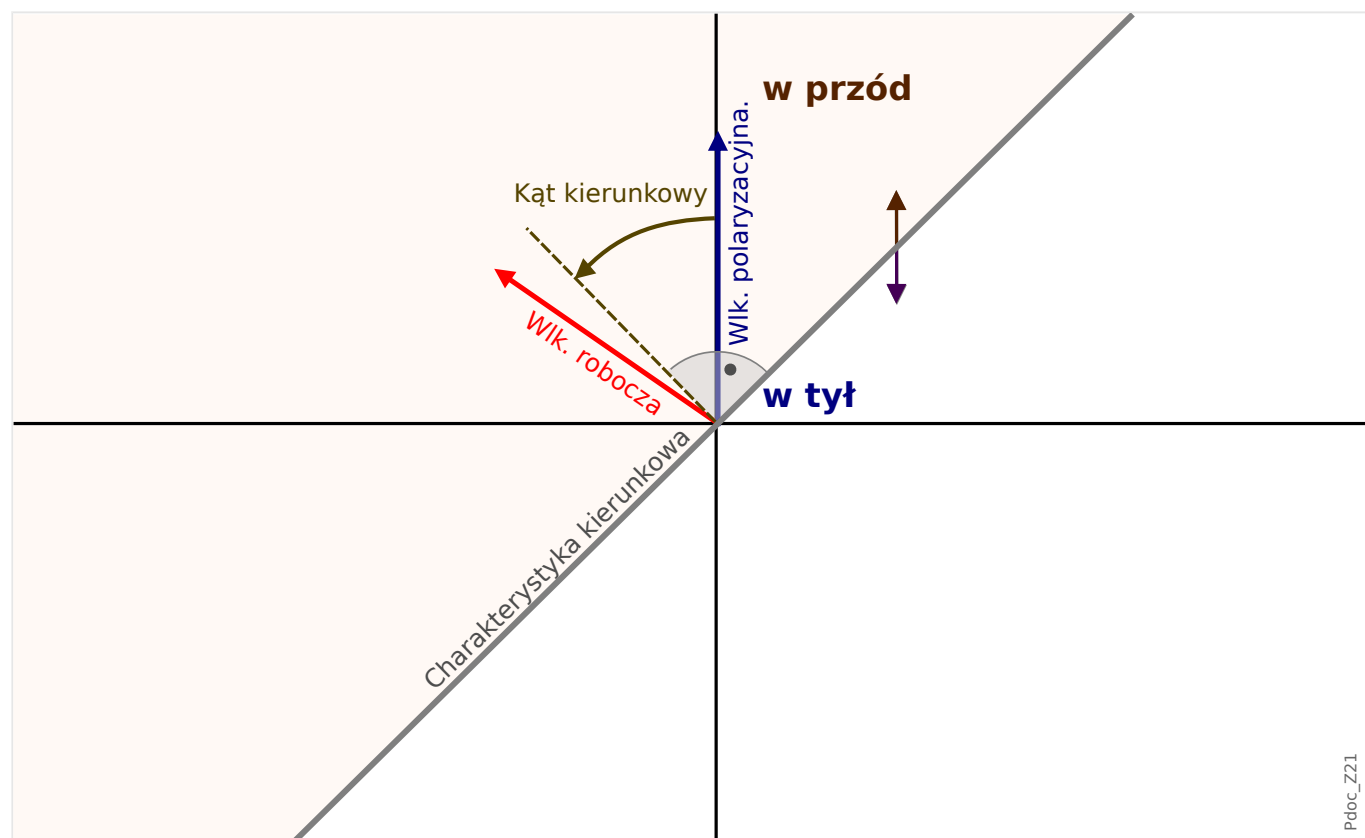
Rys. 64: Zasada wykrywanie kierunku zwarcia międzyfazowego.
