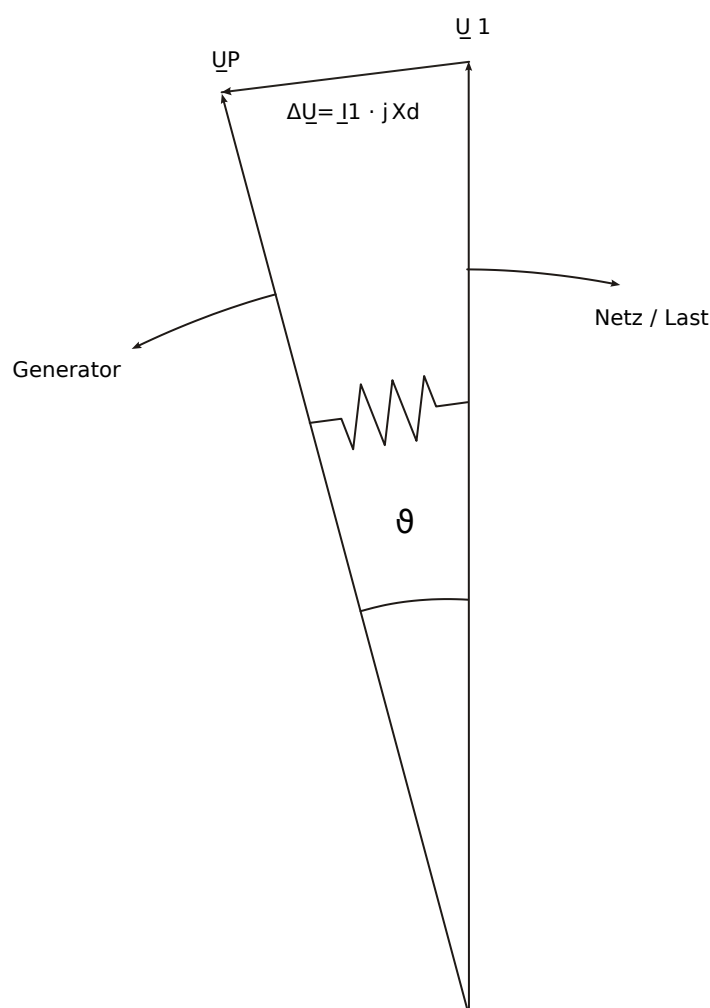
Abb. 92: Polradwinkel bei konstanter Belastung des Generators.
