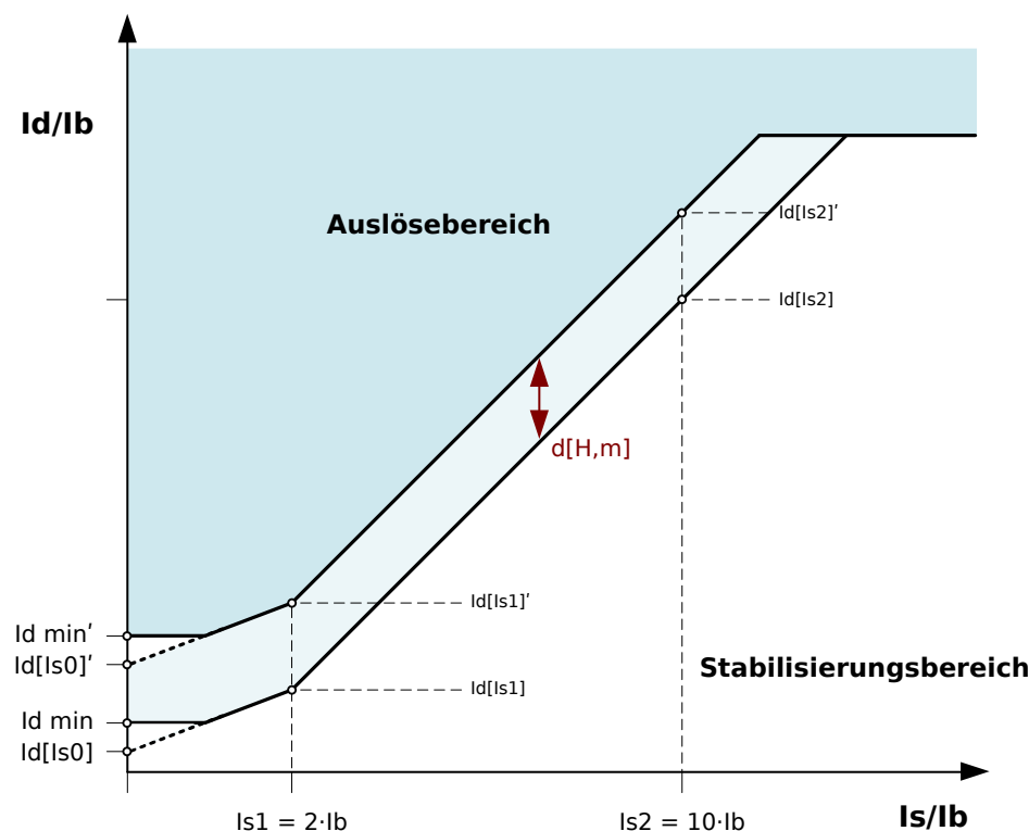
Abb. 75: Temporäre dynamische Anhebung der statischen Auslösekennlinie.
