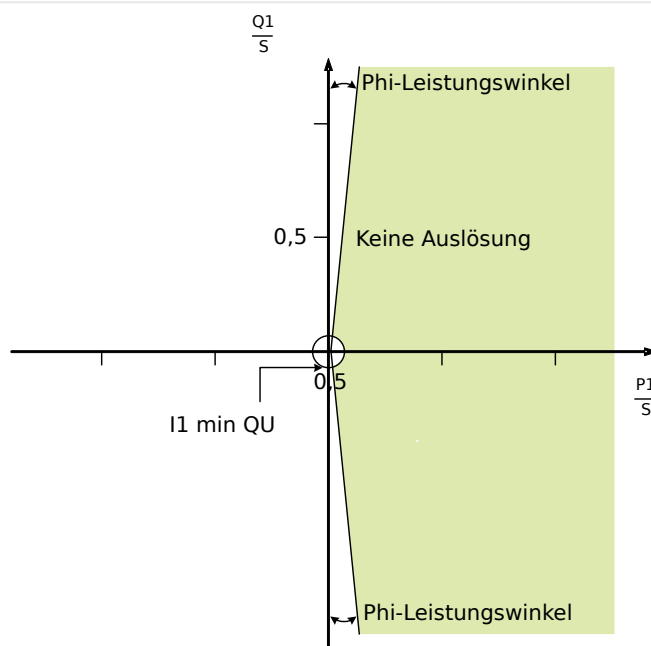
Abb. 110: Variante 1 (Leistungswinkel-Überwachung): »AFE Methode« = „Leistungswinkel-Überwachung“.
