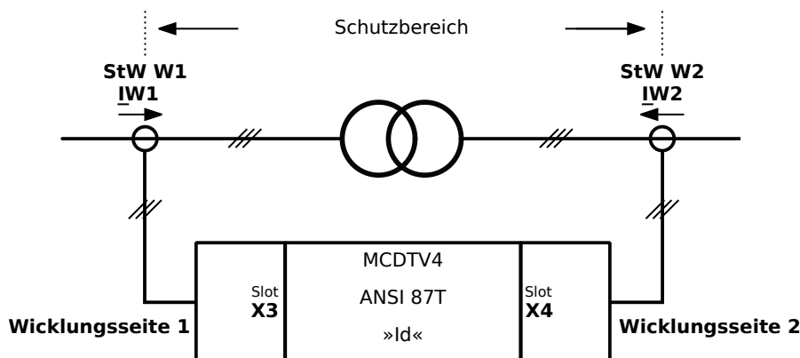
Abb. 73: ANSI 87T: Transformator-Phasenstrom-Differenzialschutz.
