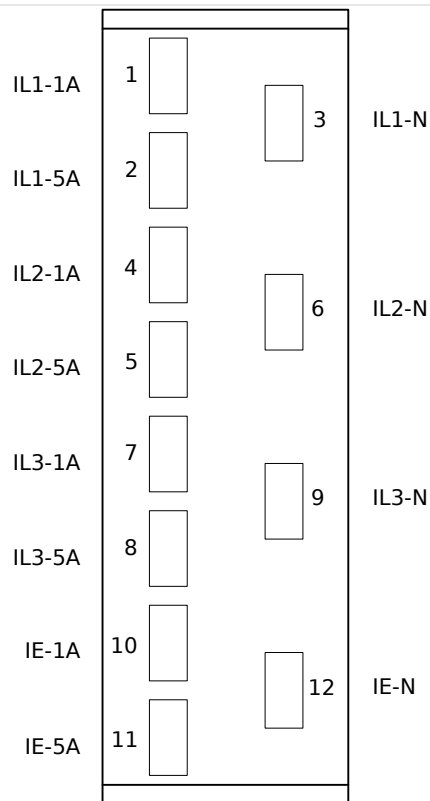
Abb. 19: TIs - Elektromechanische Zuordnung
