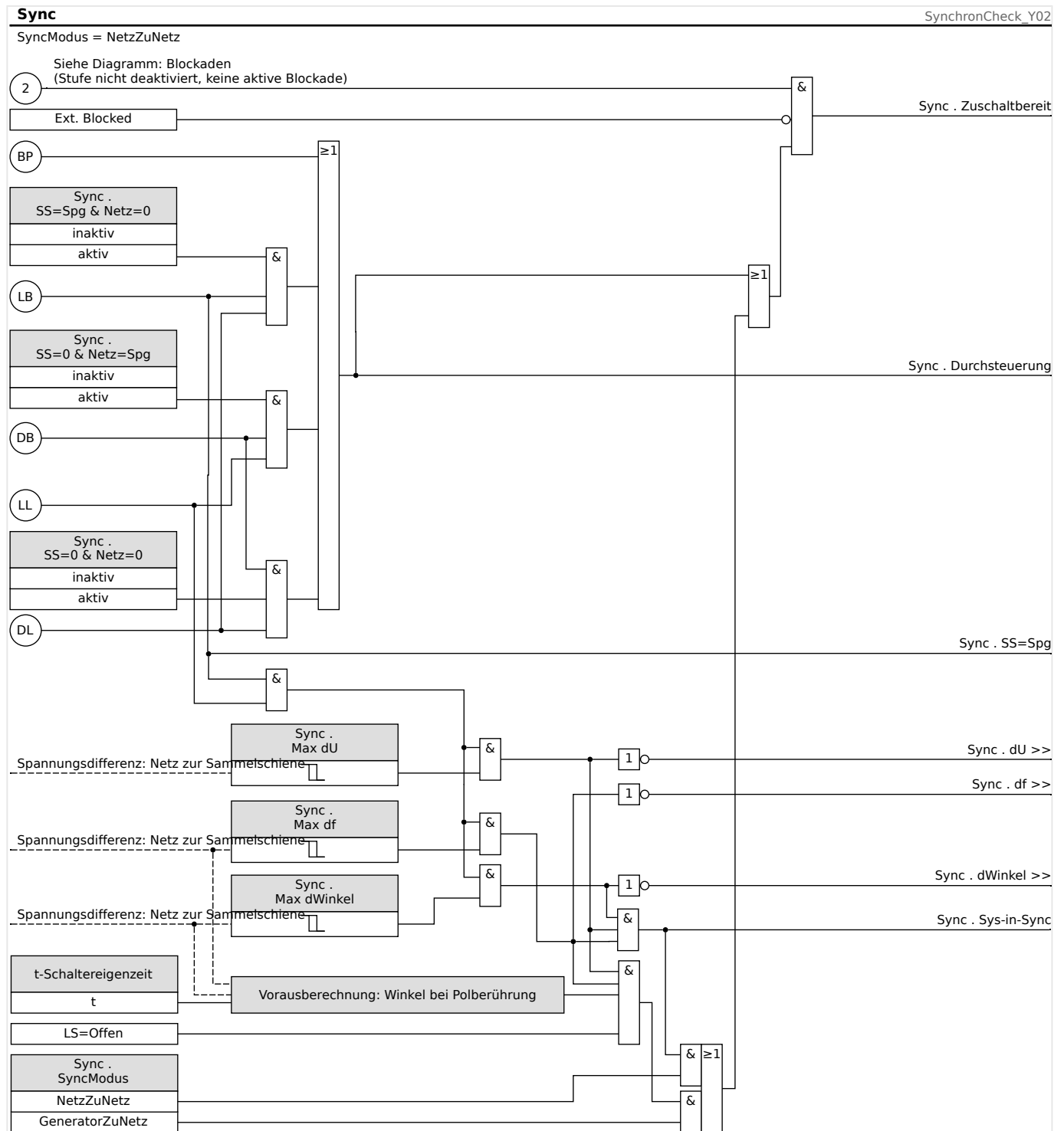
Abb. 100: Funktionalität des »Sync«-Moduls, „NetzZuNetz“.
