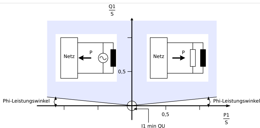
Abb. 102: Variante 1: Leistungswinkelüberwachung.
