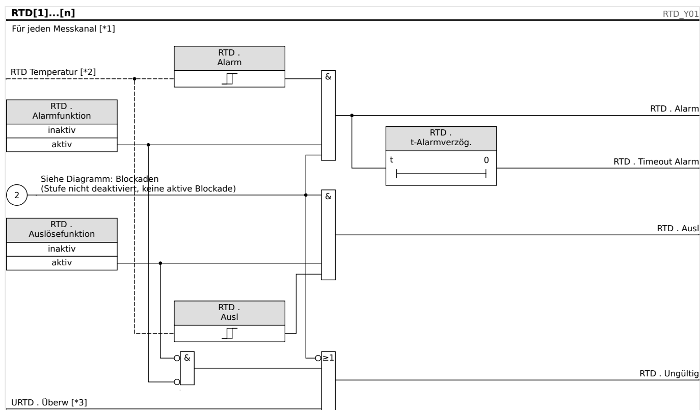
Abb. 118: Generelles RTD-Funktionsprinzip.
