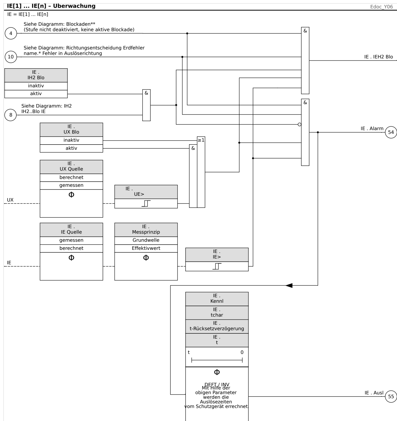
Abb. 80: Erdüberstromschutz, Teil 1 (Überwachungsfunktion, Auslöse-Entscheidung).
