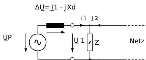
Abb. 91: Ersatzschaltbild netzparalleler Synchrongenerator
