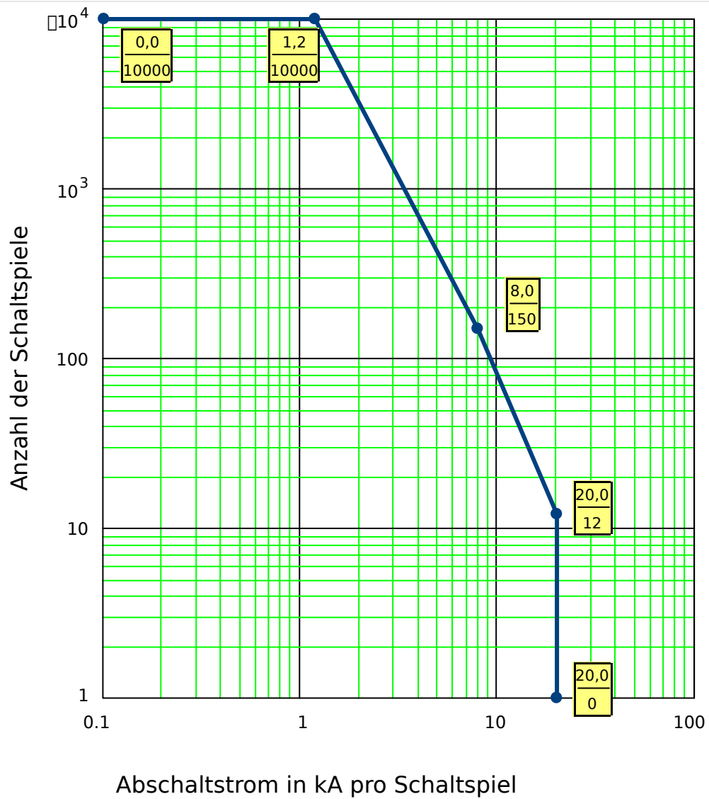
Abb. 128: Wartungskurve für einen typischen 25 kV Leistungsschalter
