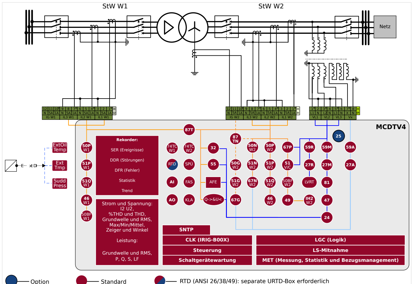
Abb. 1: Funktionsübersicht für das MCDTV4.
