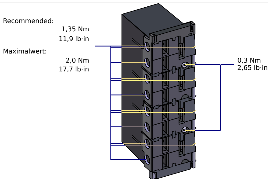
Abb. 141: Steckverbinder mit integrierten Kurzschließern (konventionelle Stromeingänge)
