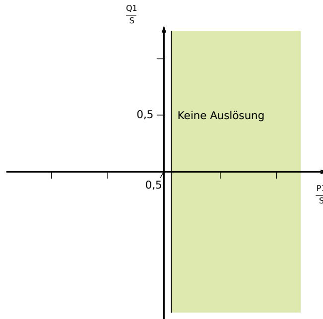
Abb. 111: Variante 2 (Reine Wirkleistungsschwellwertüberwachung): »AFE Methode« = „Reine Wirkleistungsschwelle“.
