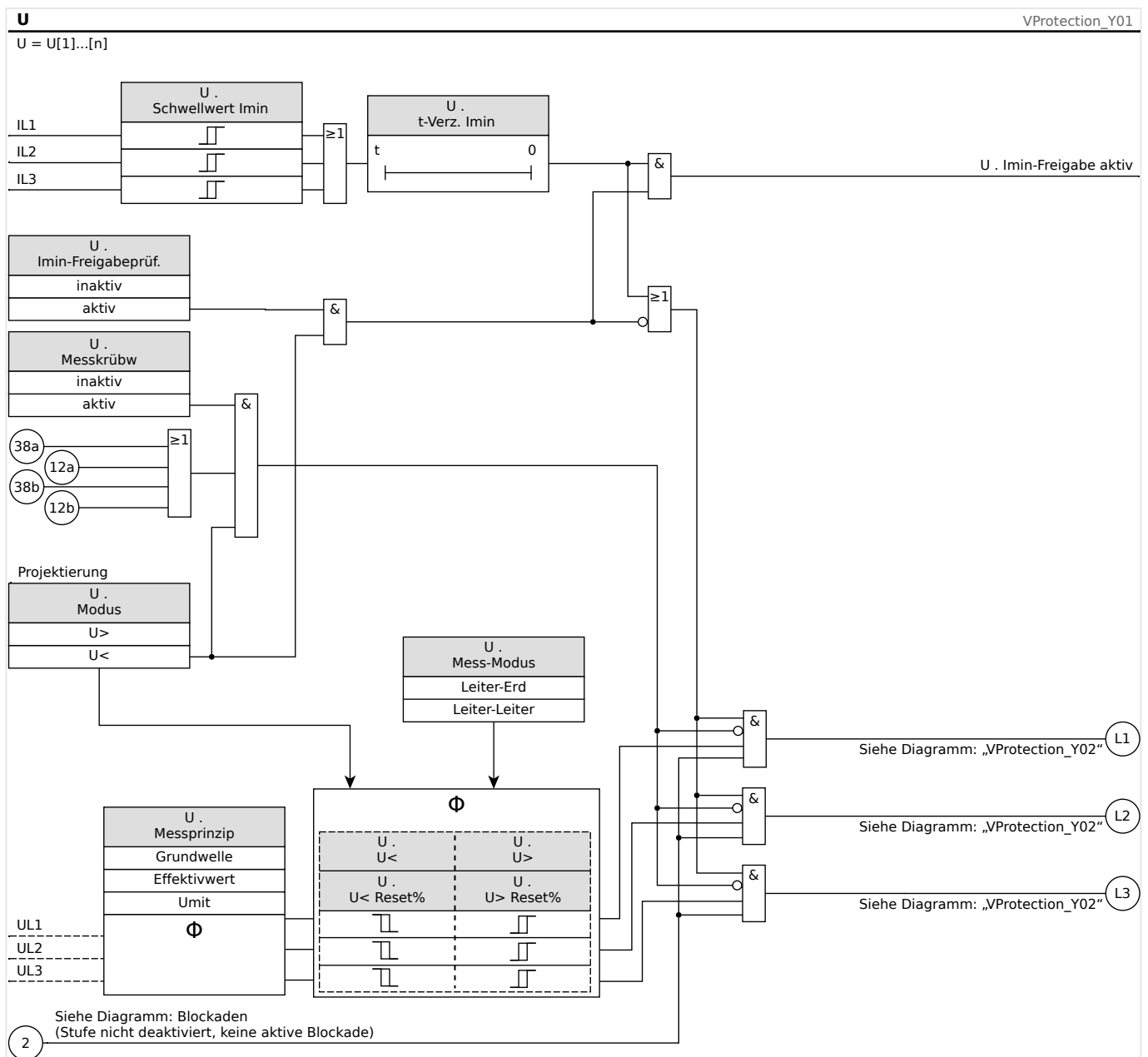
Abb. 87: Funktionalität des Spannungsschutzmoduls, Teil 1.
