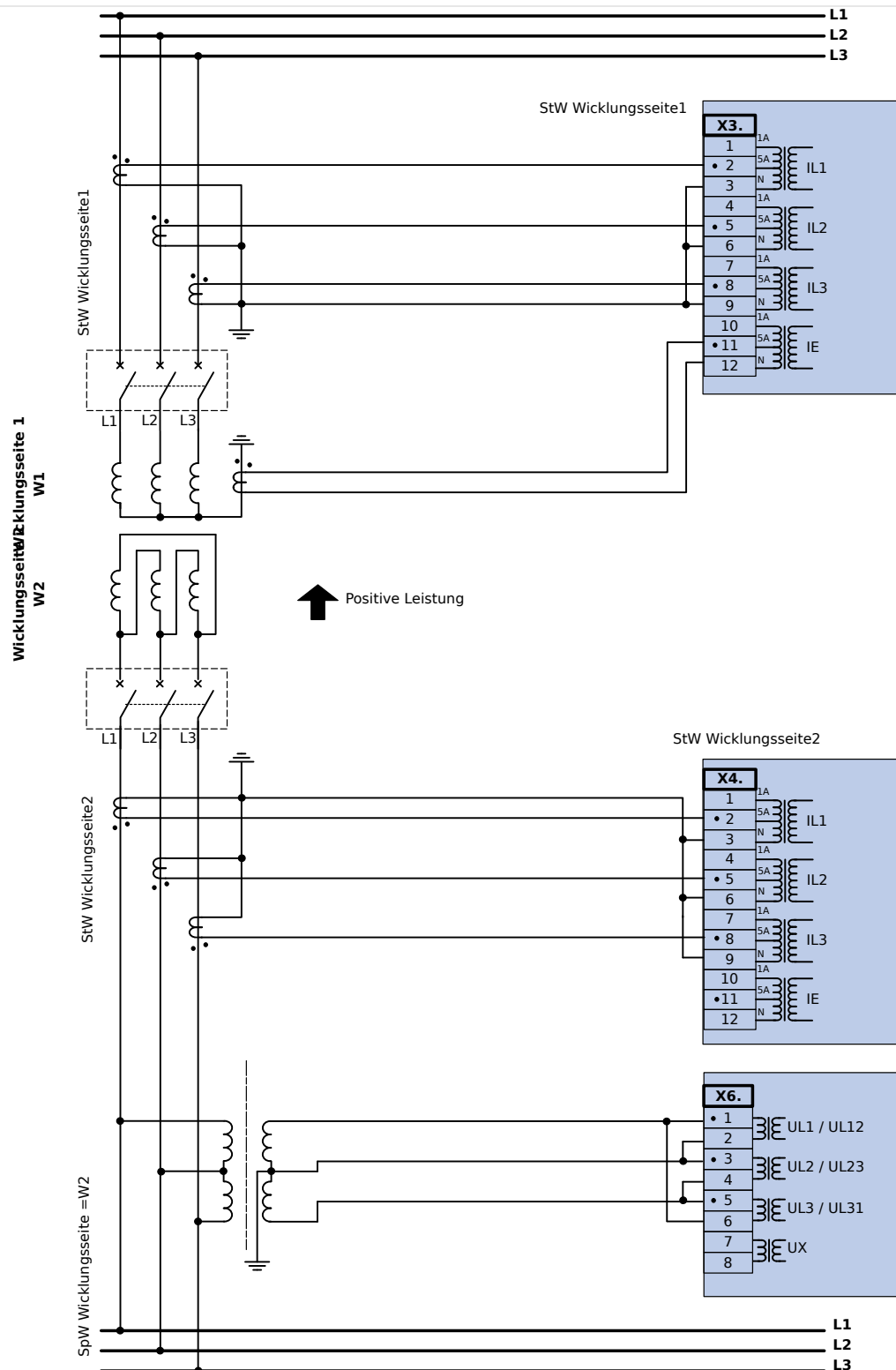
Abb. 40: DY-Transformator mit Phasendifferenzialschutz, REF auf W1 and SpW auf W2 (V-Schaltung).
