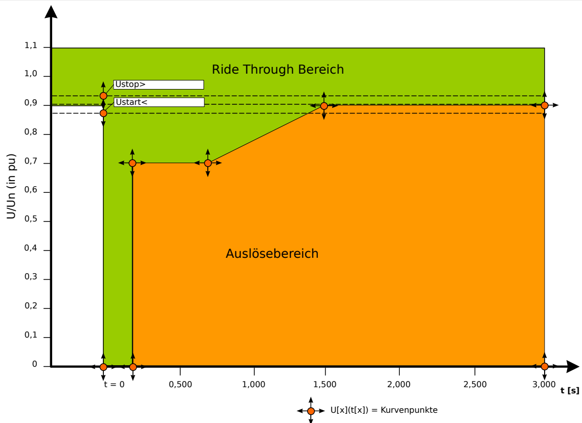
Abb. 114: Spannungs-Zeit-Profil und Auslösebereich.
