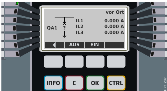
Abb. 124: Beispiel einer Steuer-Seite mit „Leistungsschalter“ in Störstellung (bzw. unplausiblem Zustand).
