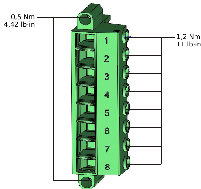
Abb. 142: Spannungsmessstecker der Spannungsmesskarte „TU“ (↳ „2.8.1 TU - Spannungsmesseingänge“).
