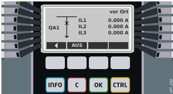
Abb. 123: Beispiel einer Steuer-Seite mit geschlossenem „Leistungsschalter“.
