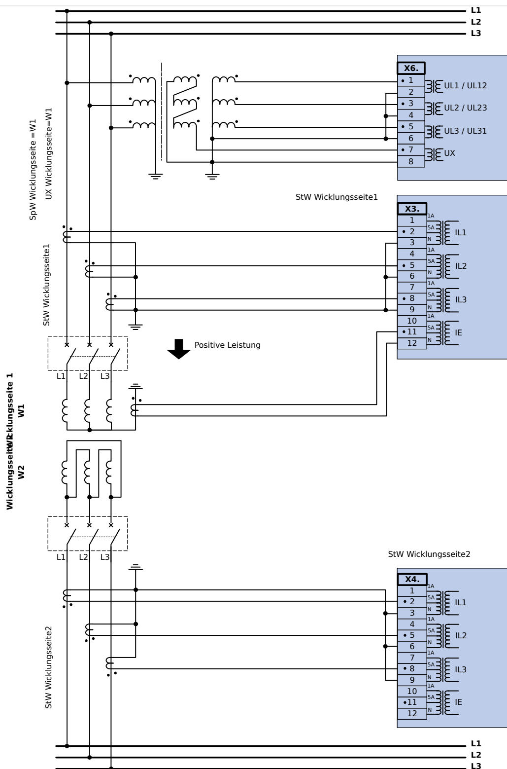
Abb. 39: DY-Transformator mit Phasendifferenzialschutz und Erddifferenzialschutz auf der Seite W1.
