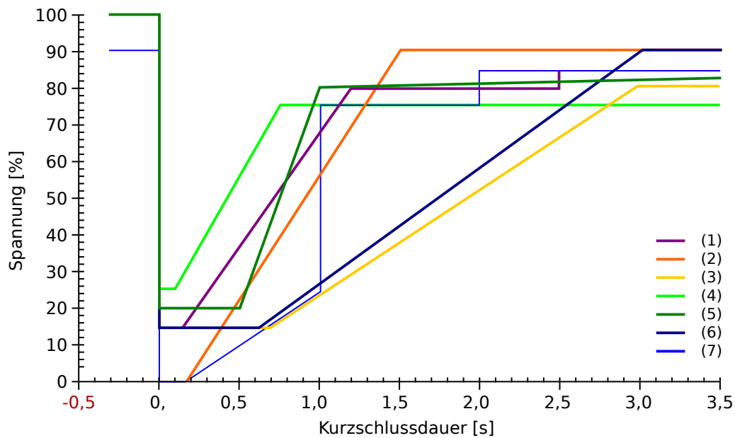
Abb. 112: Nationale LVRT-Standards, aus: eBWK Bd. 60 (2008) Nr. 4. Autoren: Dipl.-Ing. Thomas Smolka, Dr.-Ing. Karl-Heinz Weck, Zertifizierungstelle der FGH e.V., Mannheim, sowie Dipl.-Ing. (FH) Matthias Bartsch, Enercon GmbH, Aurich.
