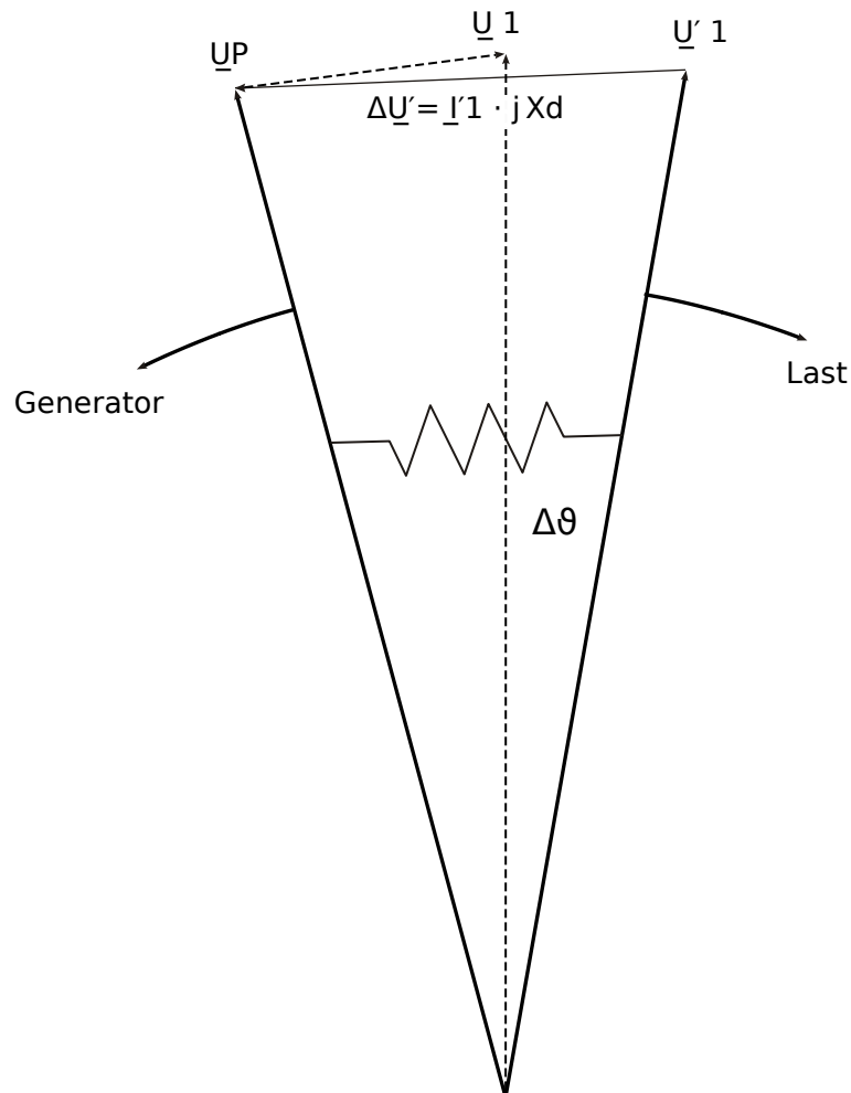
Abb. 94: Änderung des Polradwinkels bei plötzlicher Belastung des Generators.
