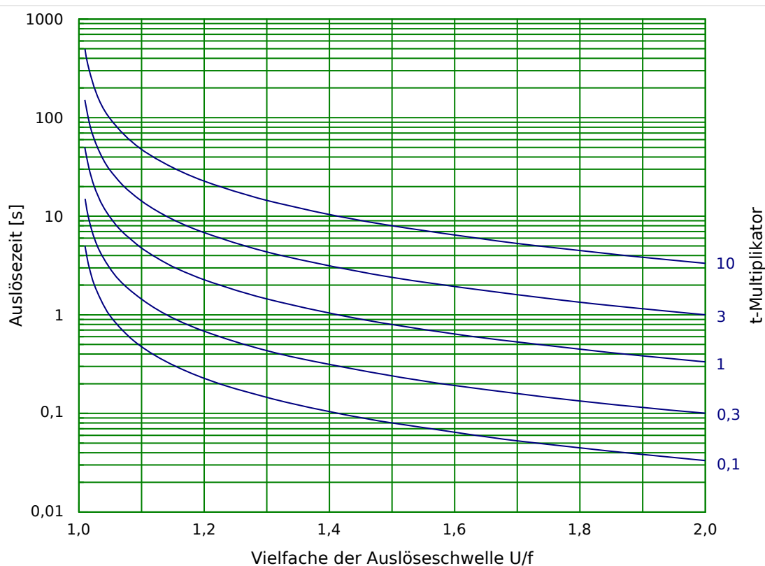
Abb. 83: Charakteristik/Kennlinie: INV A
