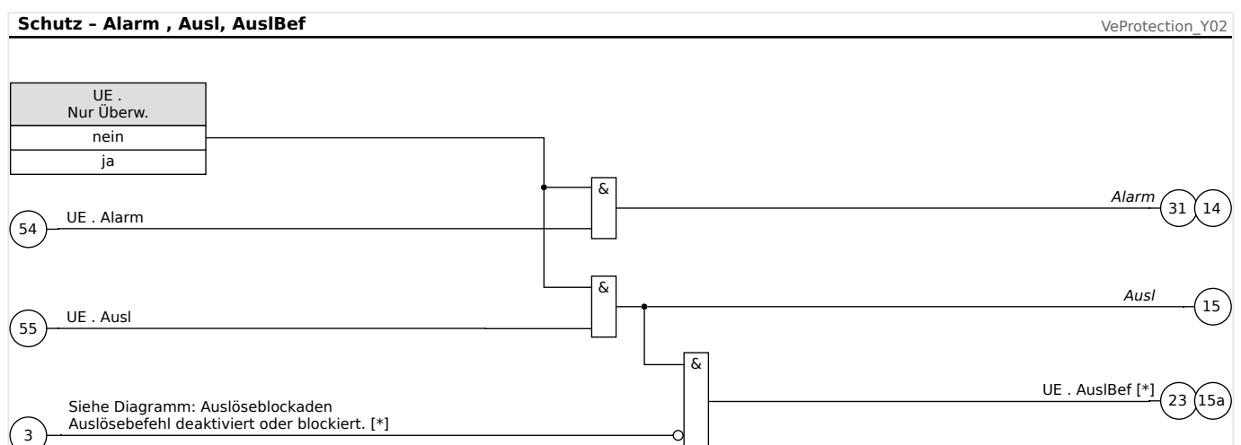
Abb. 90: UE/UX-Spannungsüberwachung, Teil 2 (Aus-Befehl und Anstoßen von Generalanregung und General-Auslösung).
