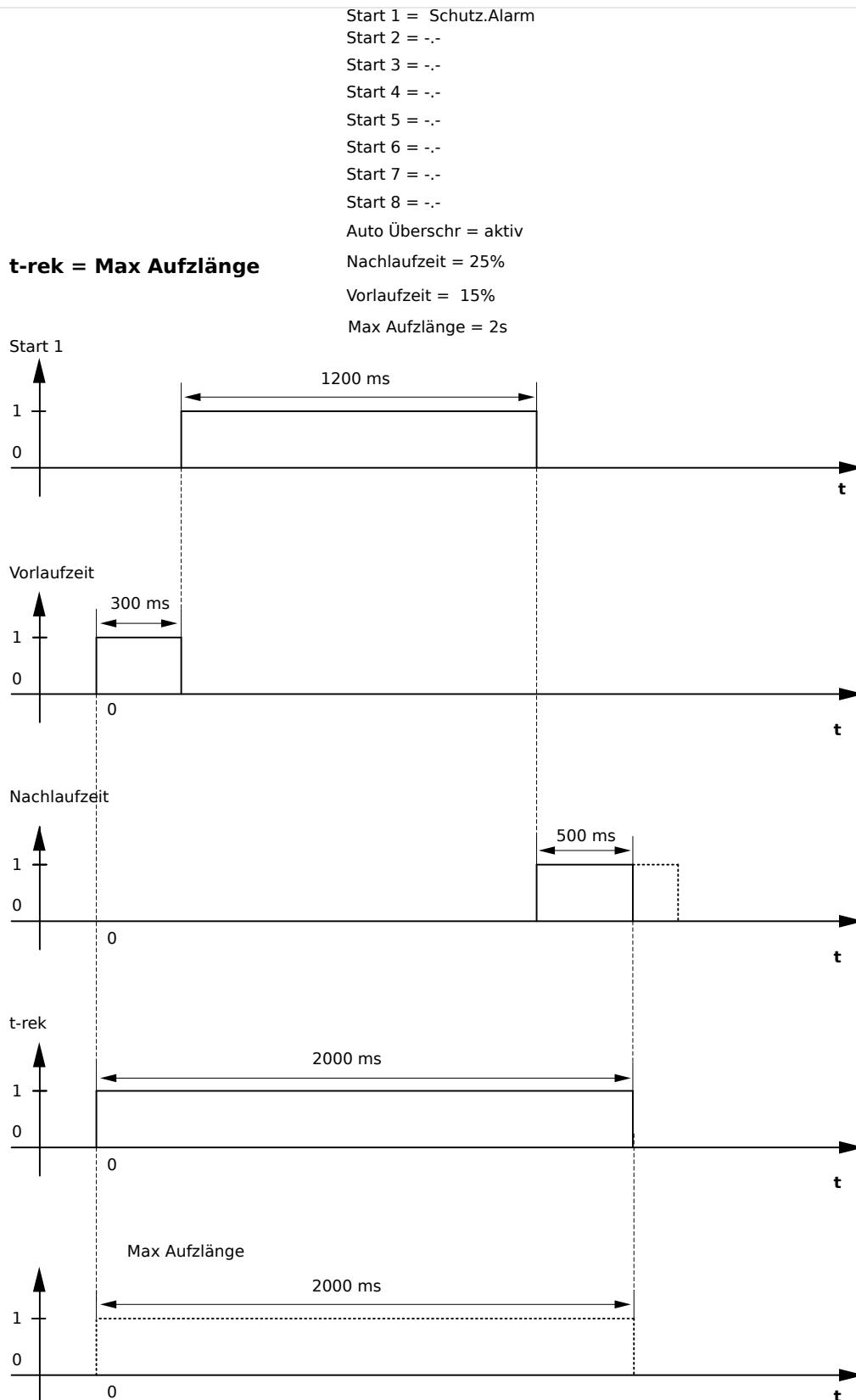
Abb. 131: Beispiel I Störschreiber-Ablaufdiagramm
