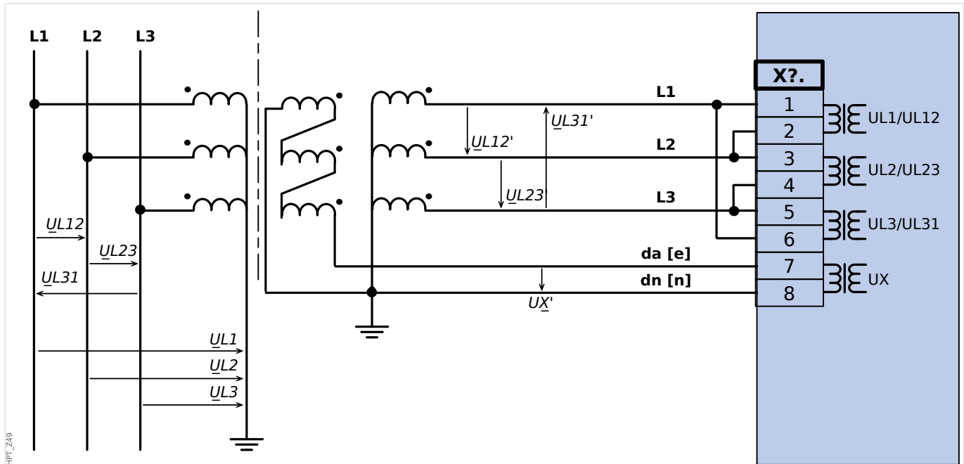
Abb. 37: Drei Spannungswandler mit Geräteanschluss in Dreieckschaltung Erfassung der Verlagerungsspannung \underline{U}_E mit offener Dreieckswicklung e-n
