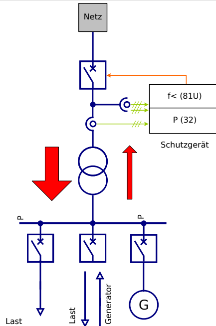
Abb. 106: Zentrale Automatische Frequenzentlastung in Netzen mit zeitweiser Rückspeisung.
