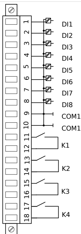
Abb. 28: Elektromechanische Zuordnung
