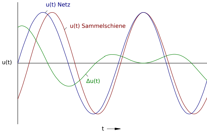
Abb. 98: Spannungsverlauf der Schwebespannung \Delta u(t) , vergrößert.
