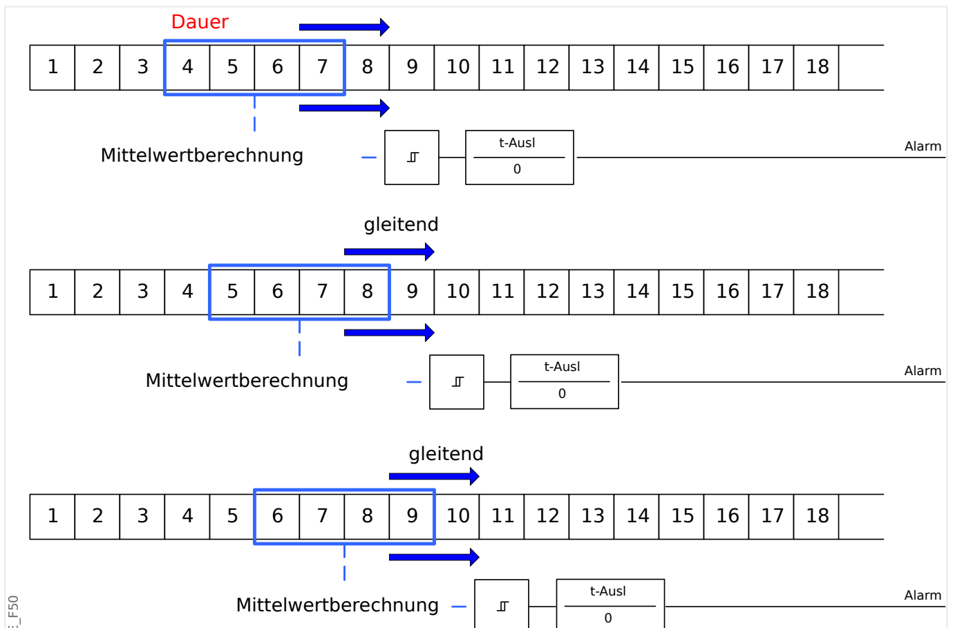
Abb. 129: Statistikmethode = gleitend
