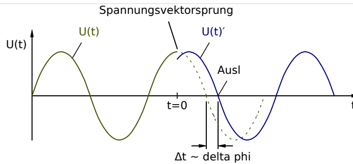
Abb. 95: Spannungsvektorsprung.
