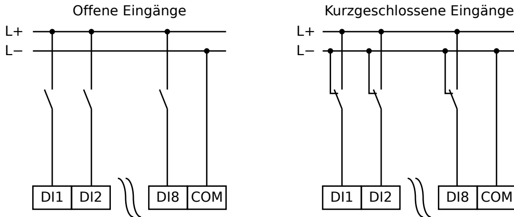
Abb. 143: Sicherer Zustand der digitalen Eingänge
