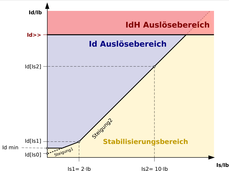
Abb. 74: Auslösekennlinie der Schutzfunktionen »Id« (blauer Bereich) und »IdH« (roter Bereich).
