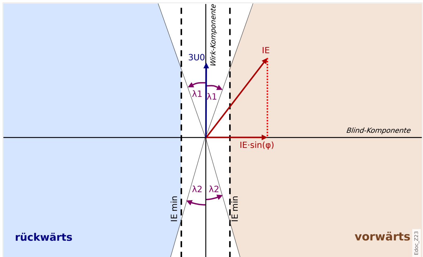
Abb. 69: Richtungserkennung nach der Methode „ \sin(\phi) “.
