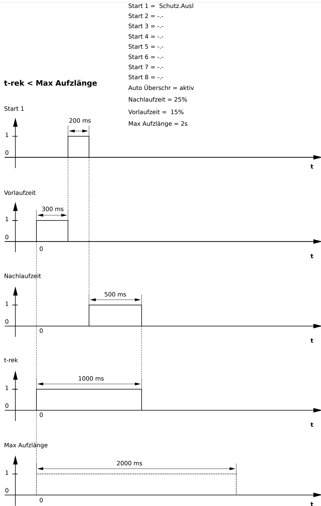
Abb. 132: Beispiel II Störschreiber-Ablaufdiagramm
