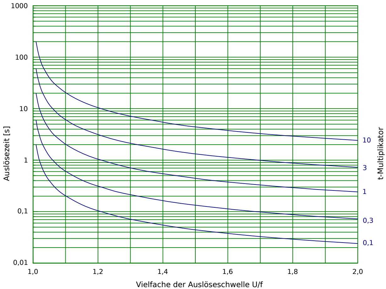
Abb. 85: Charakteristik/Kennlinie: INV C
