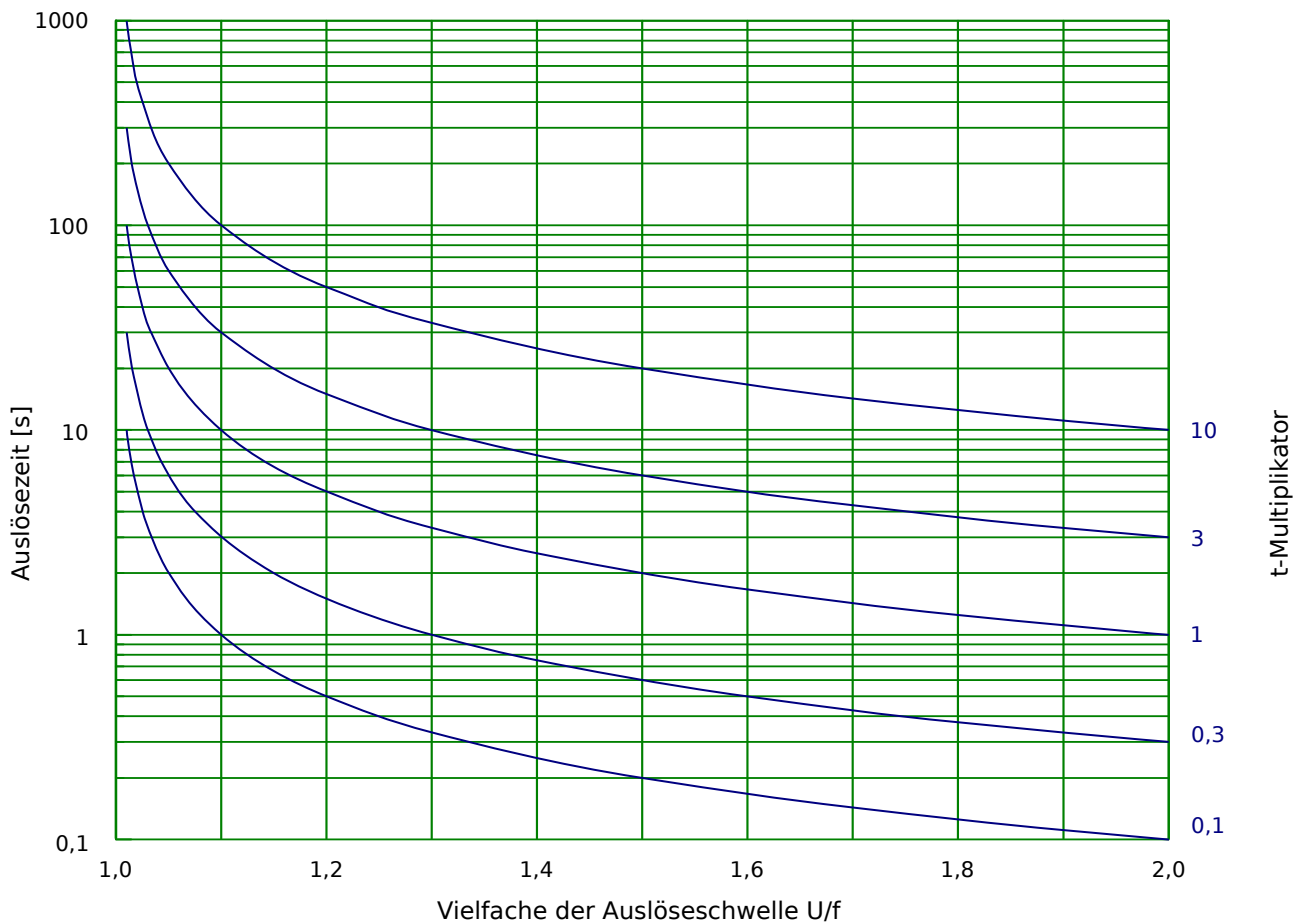
Abb. 84: Charakteristik/Kennlinie: INV B
