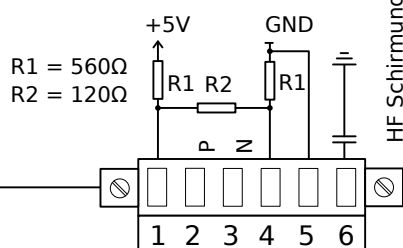
Abb. 47: Elektromechanische Zuordnung
