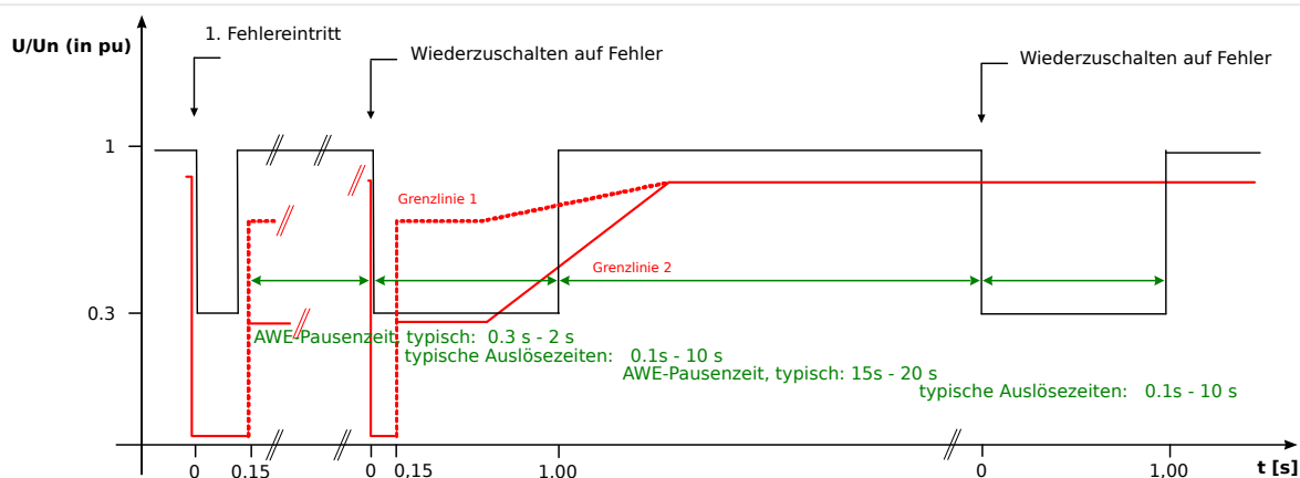
Abb. 113: Spannungsverlauf während einer zweischüssigen, nicht erfolgreichen AWE, aus: Technische Richtlinie, Erzeugungsanlagen am Mittelspannungsnetz, Ausgabe Juni 2008, BDEW Bundesverband der Energie- und Wasserwirtschaft e.V. (Page 89).
