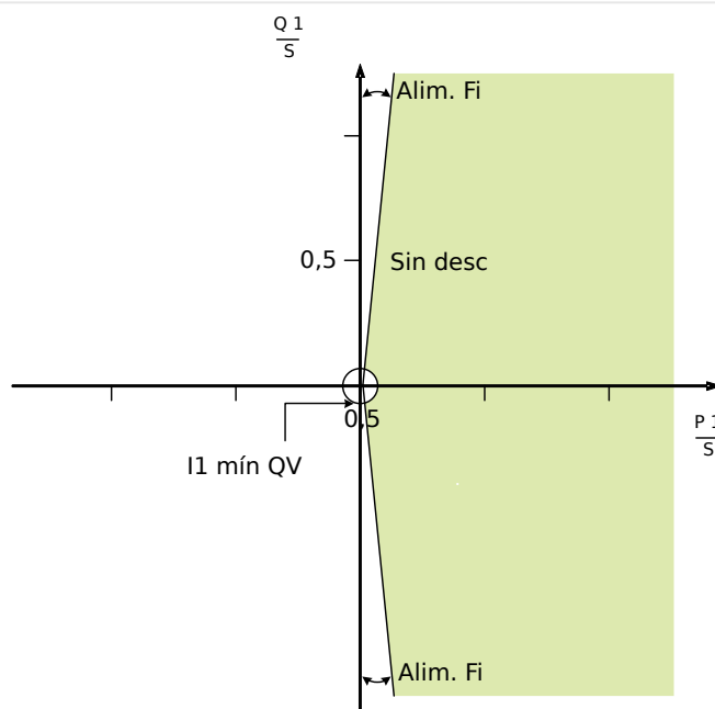
Fig. 111: Método 1 (supervisión de ángulo de potencia): «Método UFLS» = “Supervisión Ángulo Potencia”.
