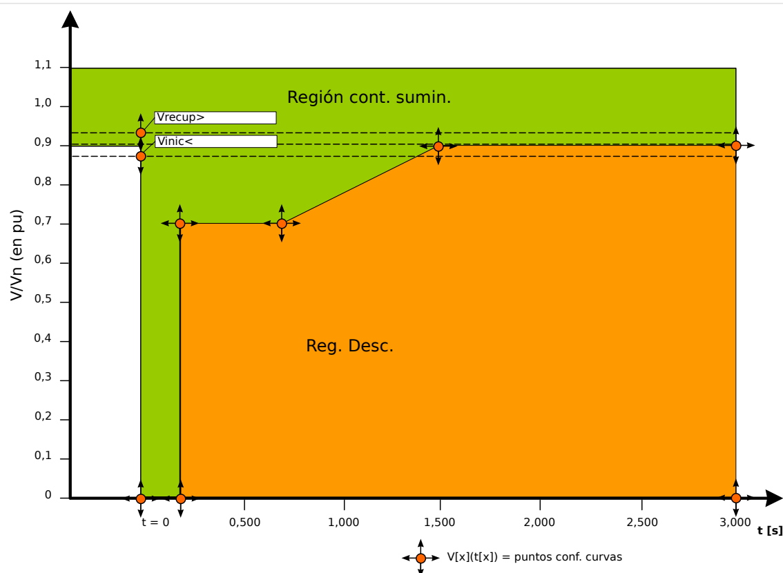
Fig. 115: Regiones de continuidad y desconexión.
