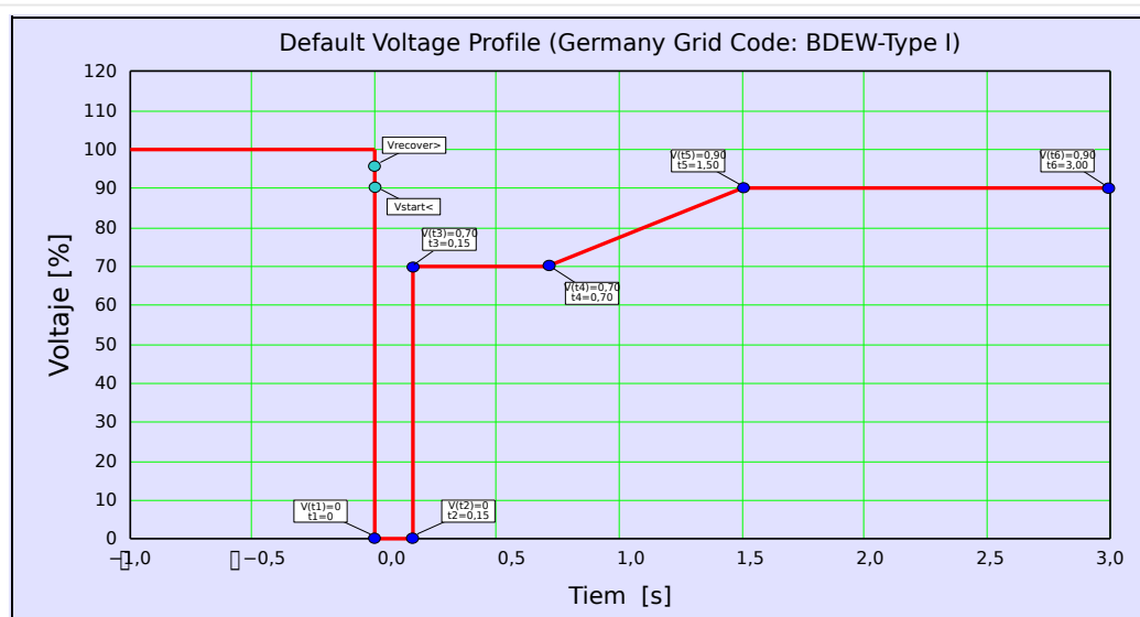
Fig. 116: Perfil de LVRT predeterminado (Tipo I de BDEW).
