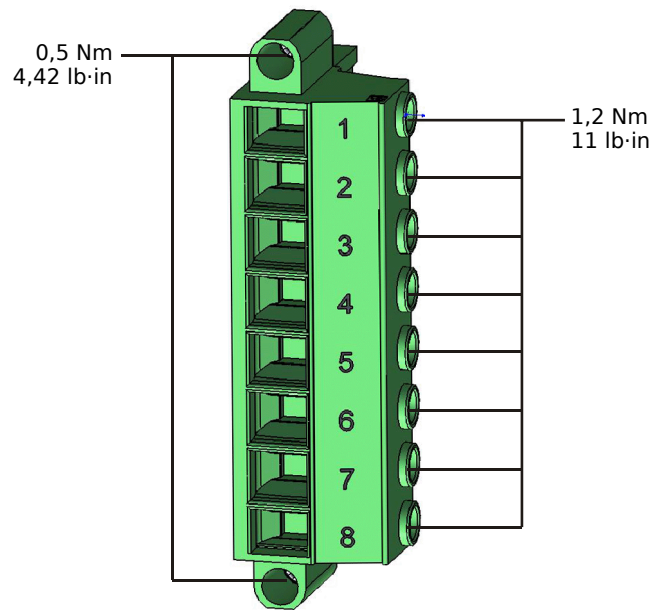
Fig. 143: Terminales de medición de tensión de la tarjeta de medición "TU" (→ «2.8.1 TU - Entradas de medición de tensión»).
