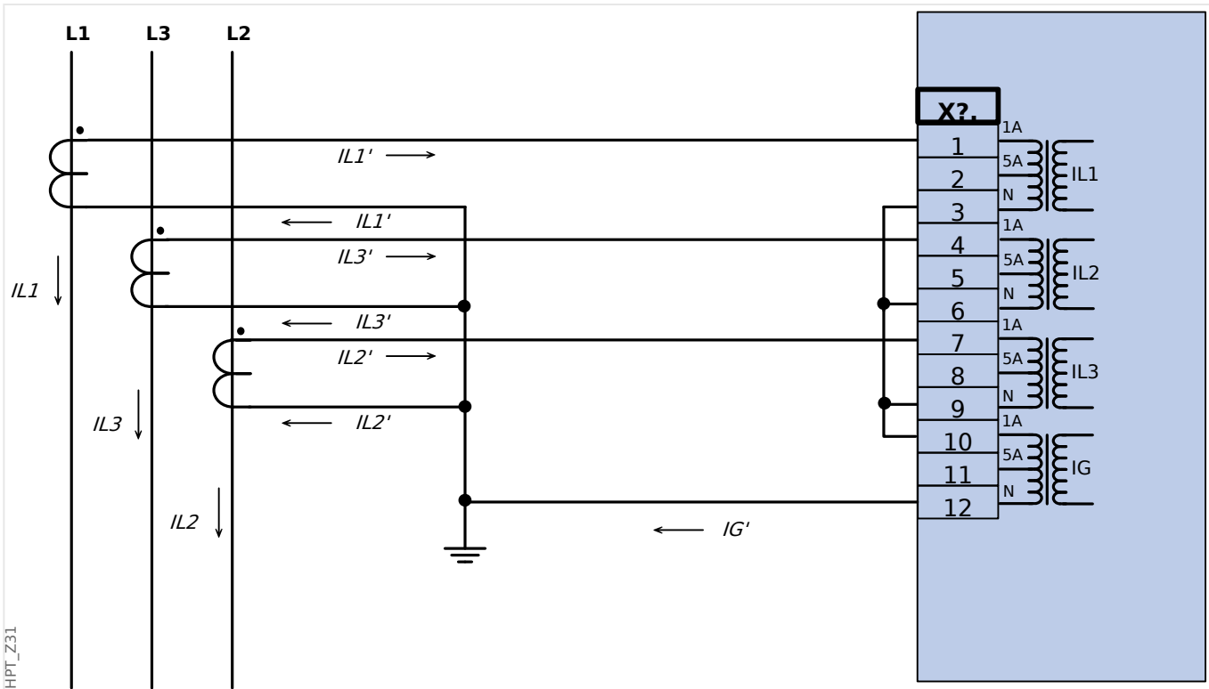
Fig. 25: Medida corriente trifásica; En secundario = 1 A. Medic corr de tierra mediante conexión Holmgreen; IG_{nom\ secund} = 1\text{ A} .
