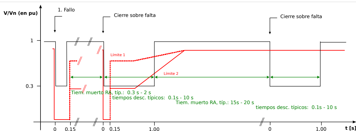
Fig. 114: Recorrido de la curva de tensión durante dos intentos fallidos de reconexión automática; fuente: Technische Richtlinie, Erzeugungsanlagen am Mittelspannungsnetz, Ausgabe Juni 2008, BDEW Bundesverband der Energie- und Wasserwirtschaft e.V. (Página 89).
