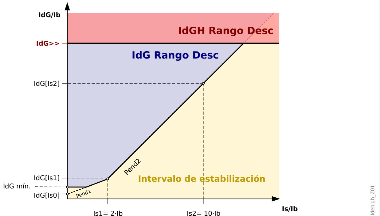
Fig. 80: Valor de selección »IdG>>« de la corriente de diferencial de tierra basada en la corriente nominal »lb« del objeto de protección relacionado.
