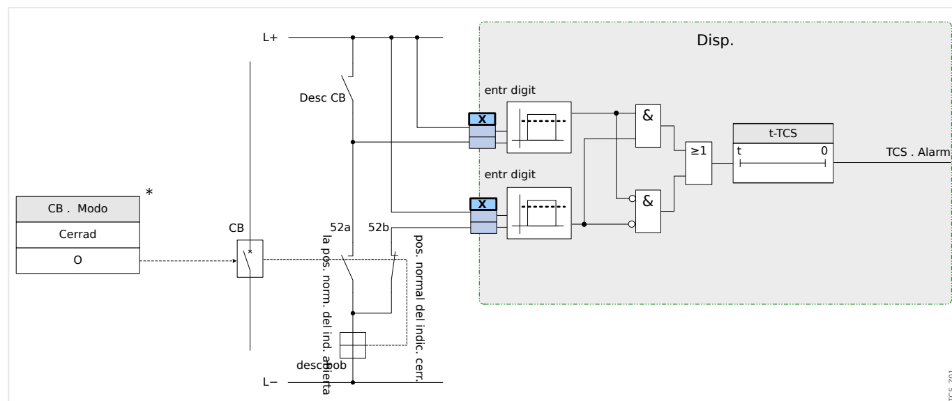
Fig. 120: Ejemplo de conexión: Supervisión del circuito de desconexión con dos contactos auxiliares CB »Aux ON« (52a) and »Aux OFF« (52b).
