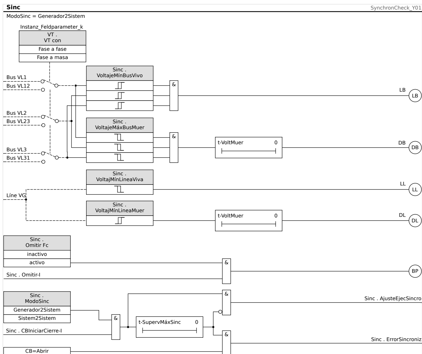
Fig. 100: Funcionalidad del módulo »Sinc«, «Generador2Sistem».
