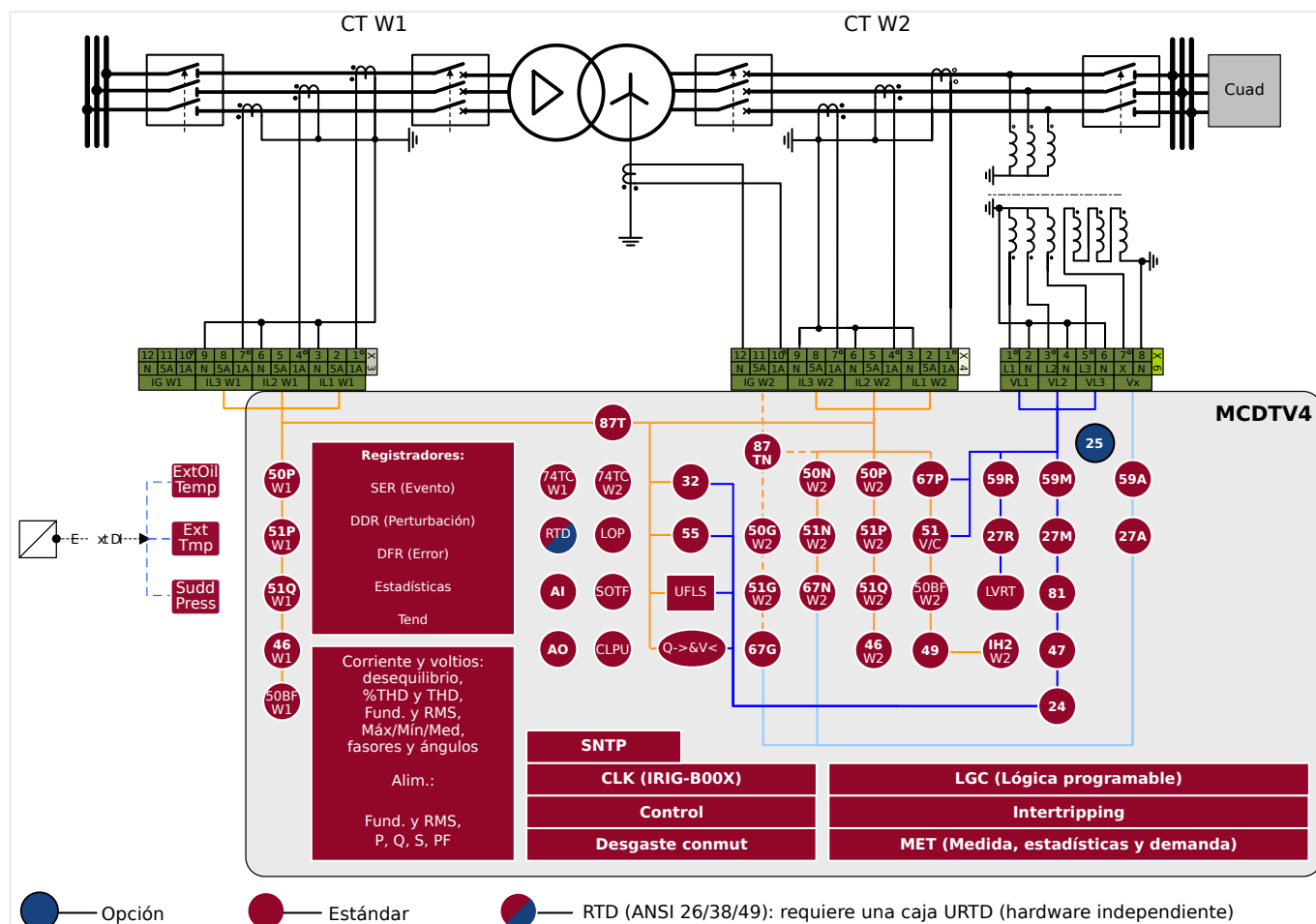
Fig. 1: Descripción funcional de MCDTV4
