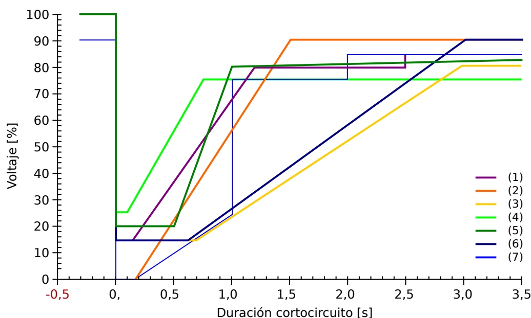
Fig. 113: Estándares de LVRT; fuente: eBWK Bd. 60 (2008) N.º 4. Autores: Dipl.-Ing. Thomas Smolka, Dr.-Ing. Karl-Heinz Weck, Zertifizierungstelle der FGH e.V., Mannheim, sowie Dipl.-Ing. (FH) Matthias Bartsch, Enercon GmbH, Aurich.
