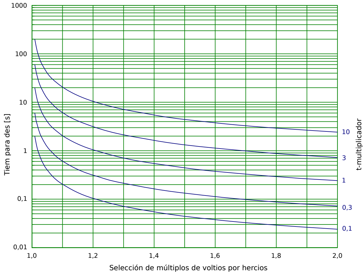
Fig. 86: Características/Forma curva: INV C
