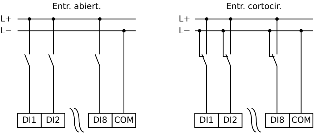
Fig. 144: Estado seguro de entradas digitales
