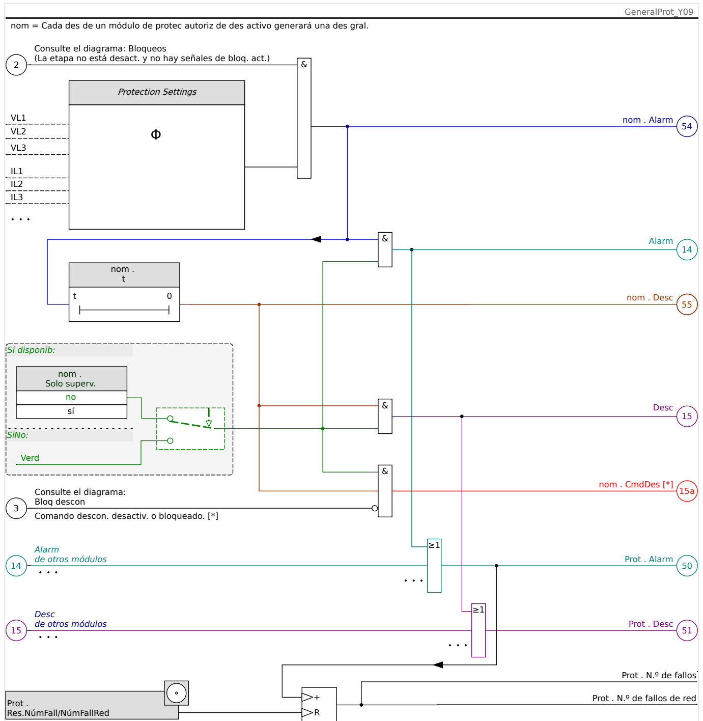
Fig. 64: Descripción a grandes rasgos de la funcionalidad de cualquier elemento de protección de HighPROTEC.
