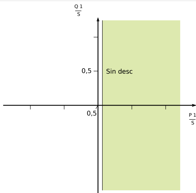
Fig. 112: Método 2 (supervisión de potencia activa pura): »Método UFLS« = “Superv. de potencia activa pura”.
