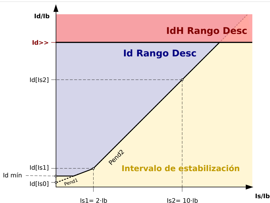
Fig. 75: Curvas de desconexión de »Id« (área azul) y funciones de protección de »IdH« (área roja).
