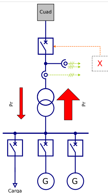
Fig. 109: Uso centralizado en redes con alimentación predominante.
