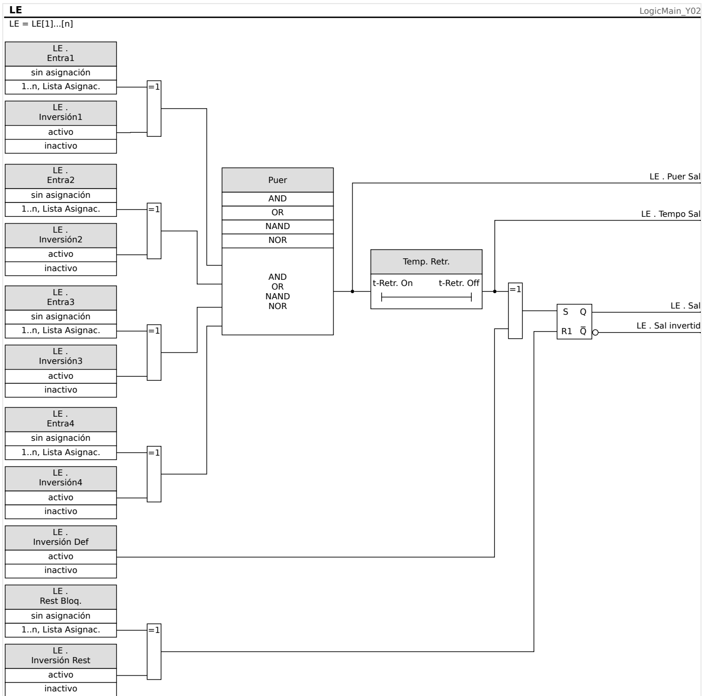
Fig. 136: Descripción detallada - Diagrama de lógica general.
