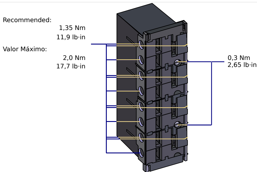
Fig. 142: Conector enchufable con cortocircuitador integrado (entradas de corriente convencionales)
