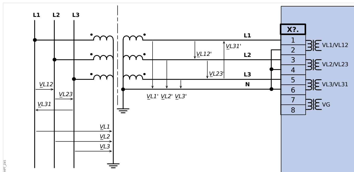
Fig. 34: VT Wye: Medida de voltaje trifásico: cableado de las entradas de medida: "conex. estrella"
