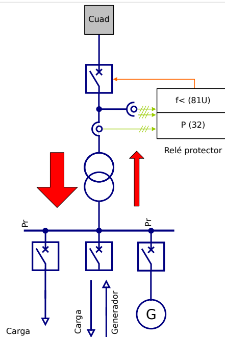
Fig. 107: Reducción de carga centralizada por subfrecuencia en redes eléctricas con alimentación temporal
