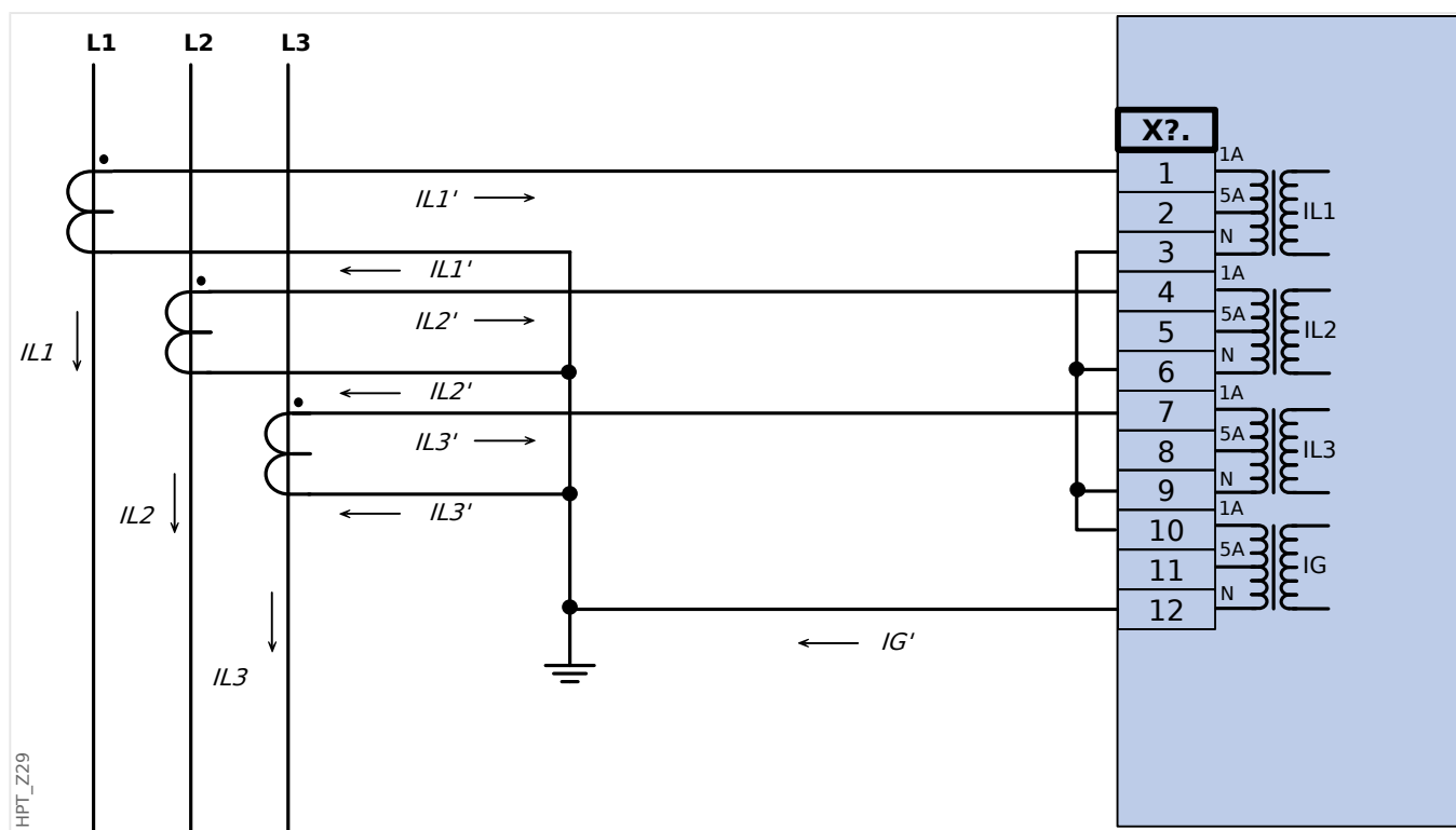
Fig. 23: Medida corriente trifásica; En secundario = 1 A. Medic corr de tierra mediante conexión Holmgreen; IGnom secund = 1 A.
