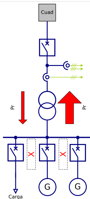
Fig. 110: Uso descentralizado en redes con alimentación predominante.
