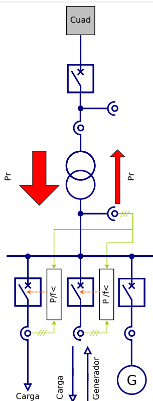
Fig. 108: Reducción de carga descentralizada por subfrecuencia en redes eléctricas con alimentación temporal.
