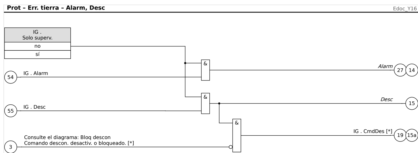
Fig. 82: Protección de sobrecarga de tierra, parte 2 (comando de desconexión y activación de alarma general y desconexión general).
