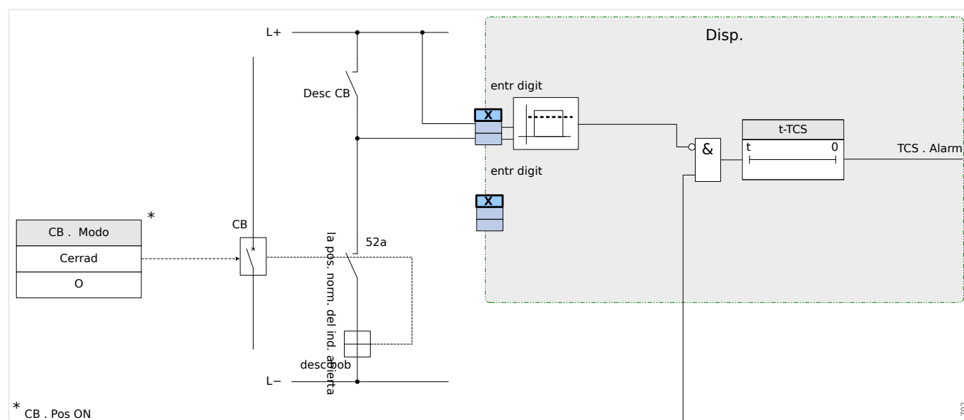
Fig. 121: Ejemplo de conexión: Supervisión del circuito de desconexión solo con un contacto auxiliar CB »Aux ON« (52a).
