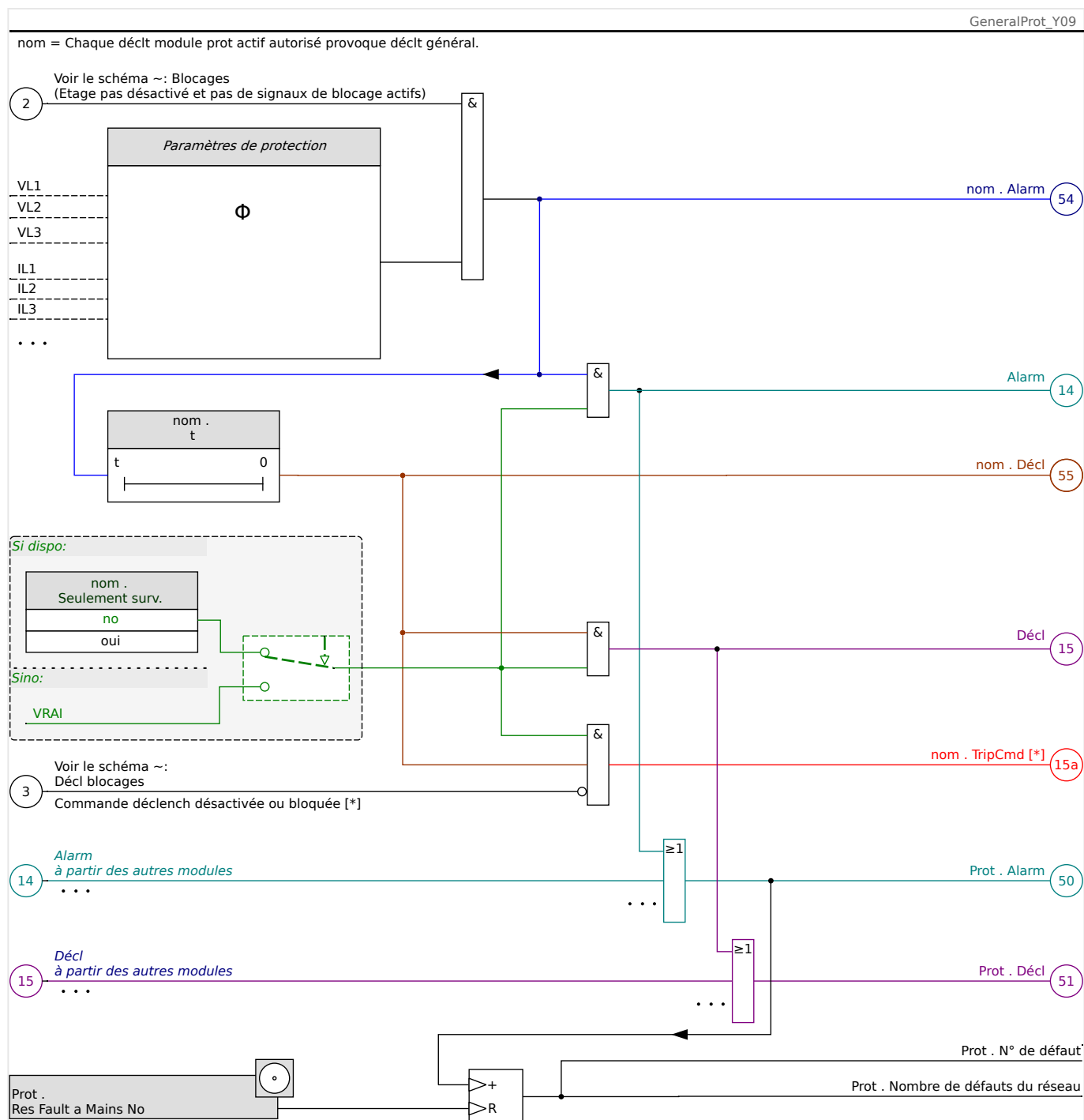
Fig. 64: Schéma de fonctionnalité des éléments de protection HighPROTEC.
