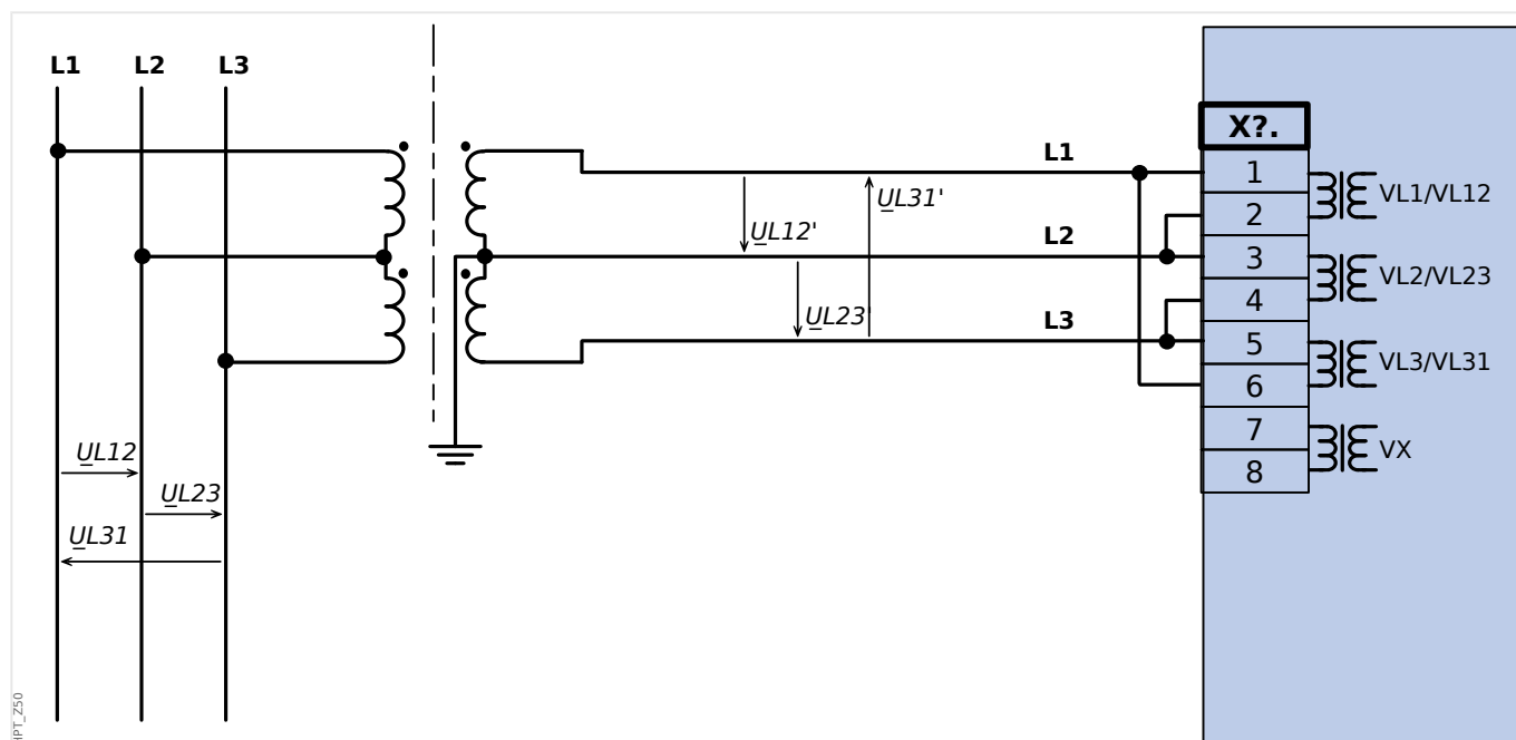
Fig. 38: Mesure de tension biphasée - câblage des entrées de mesure: "Trian ouv"
