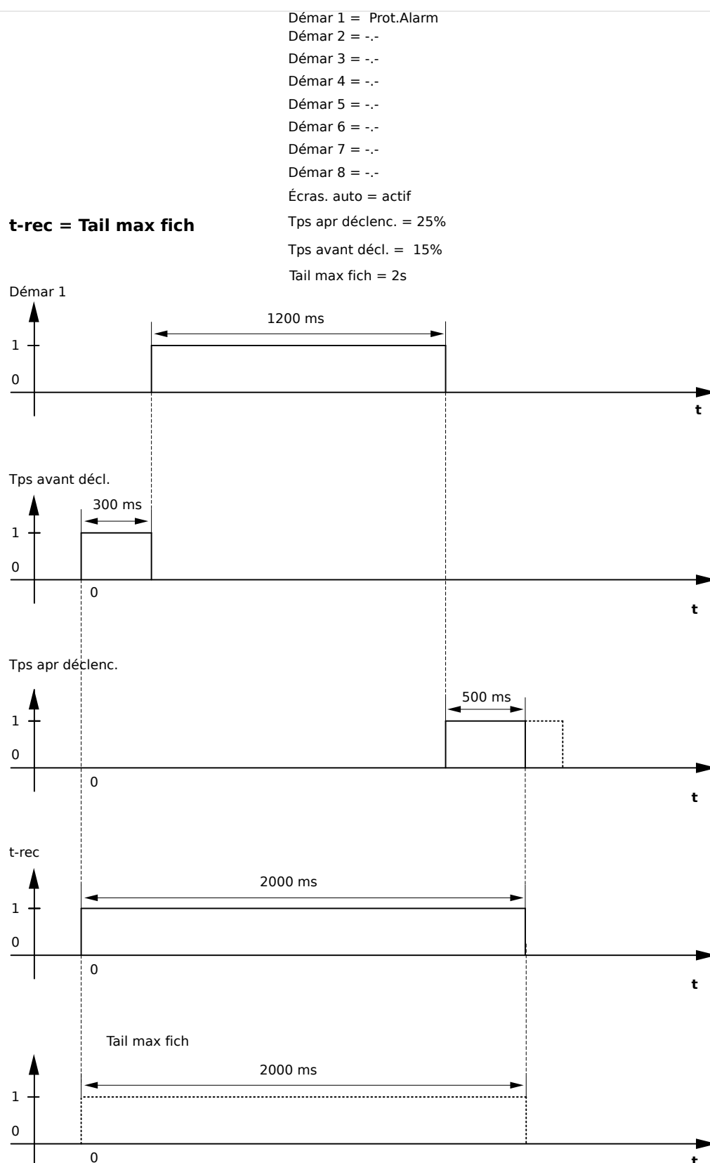
Fig. 132: Exemple de diagramme des temps de l'enregistreur de perturbations I
