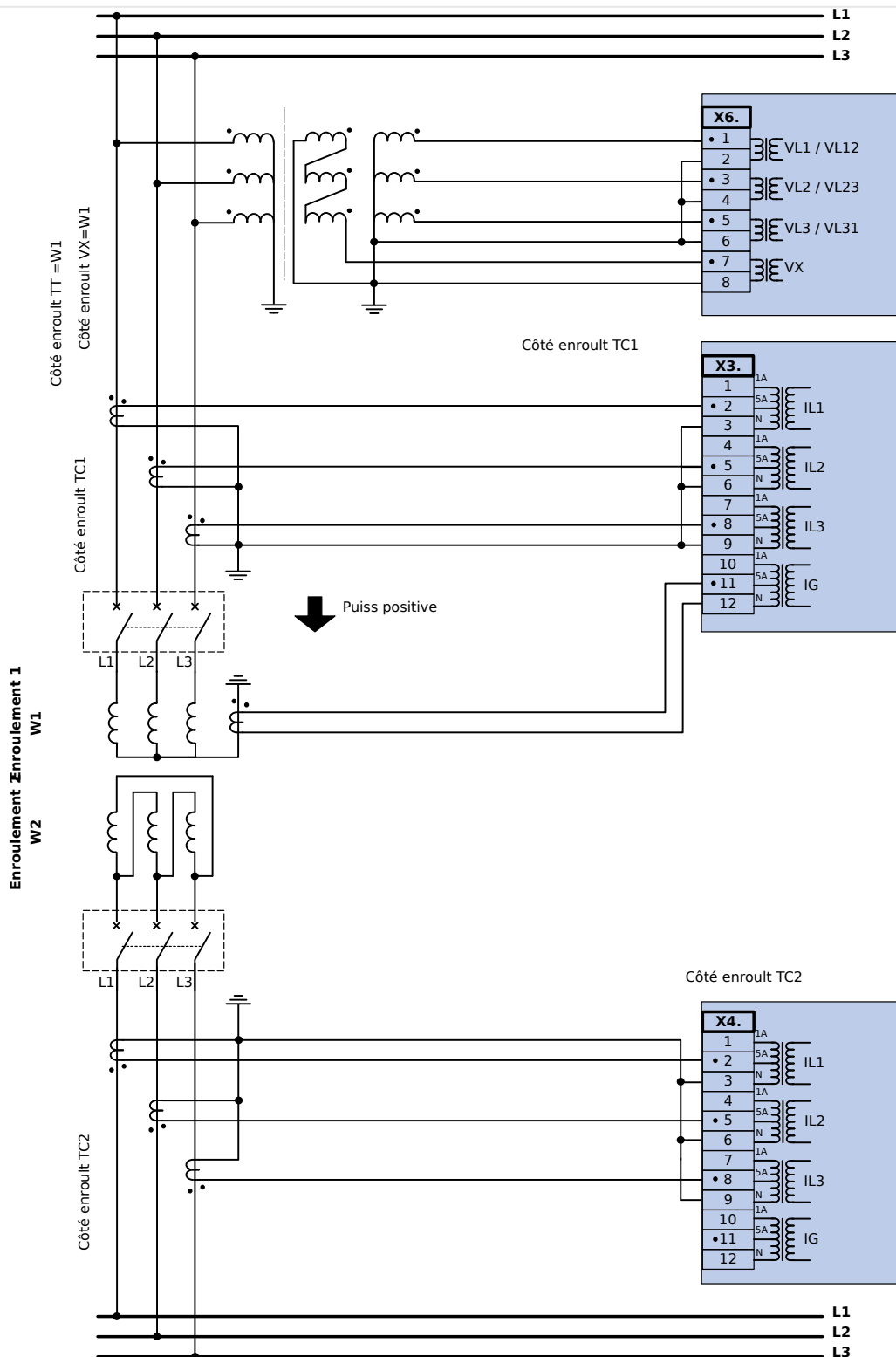
Fig. 39: Transformateur DY avec protection différentielle de phase et protection différentielle de terre sur la borne W1 uniquement.
