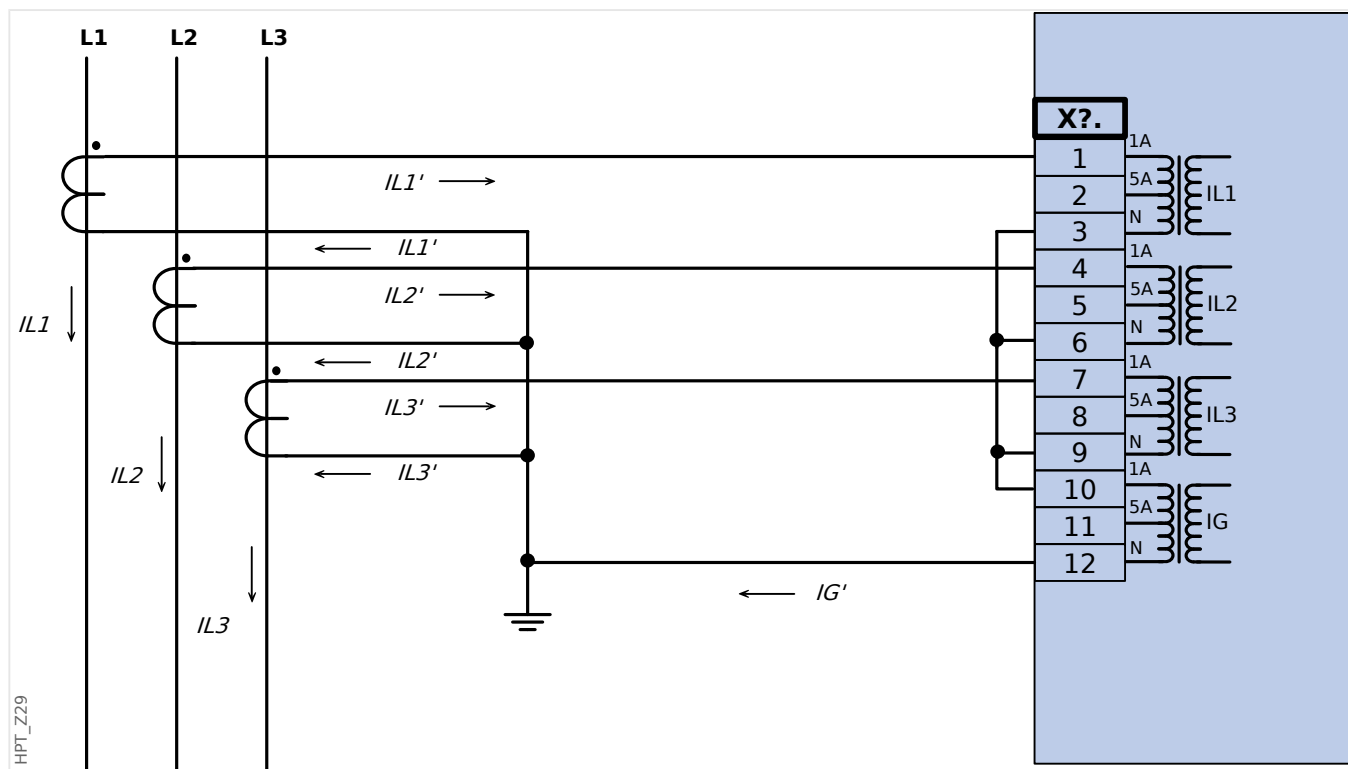
Fig. 23: Mesure de courant triphasé; I_n \text{ sec} = 1 \text{ A} Mesure courant via connexion de Holmgreen; I_{Gnom} \text{ sec} = 1 \text{ A}
