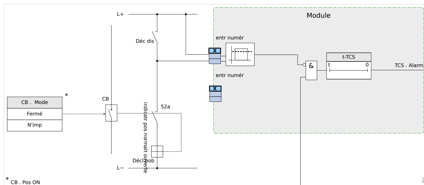
Fig. 121: Exemple de connexion : Surveillance du circuit de déclenchement avec un contact auxiliaire de disjoncteur »Aux ON« (52a).
