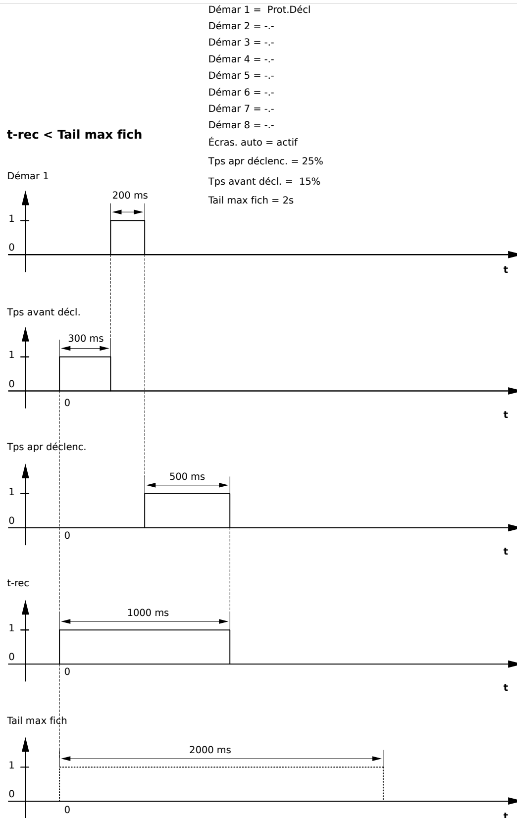
Fig. 133: Exemple de diagramme des temps de l'enregistreur de perturbations II
