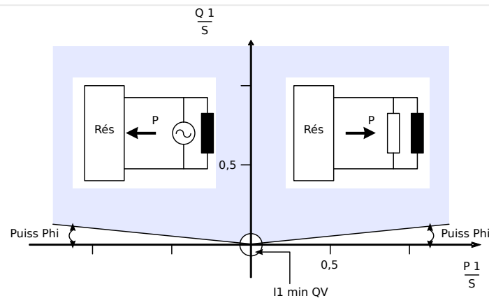
Fig. 103: Méthode 1 : Surveillance de l'angle de charge
