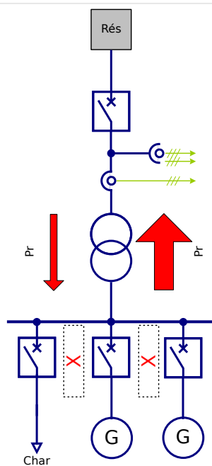
Fig. 110: Utilisation décentralisée au sein de réseaux avec alimentation prédominante.
