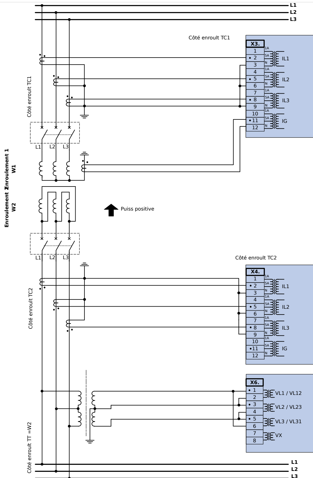
Fig. 40: Transformateur DY avec protection différentielle de phase, REF sur W1 et VT sur W2 (configuration en triangle ouvert).
