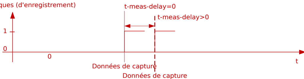
Fig. 134: Enregistreur de défaut : temps et durées
