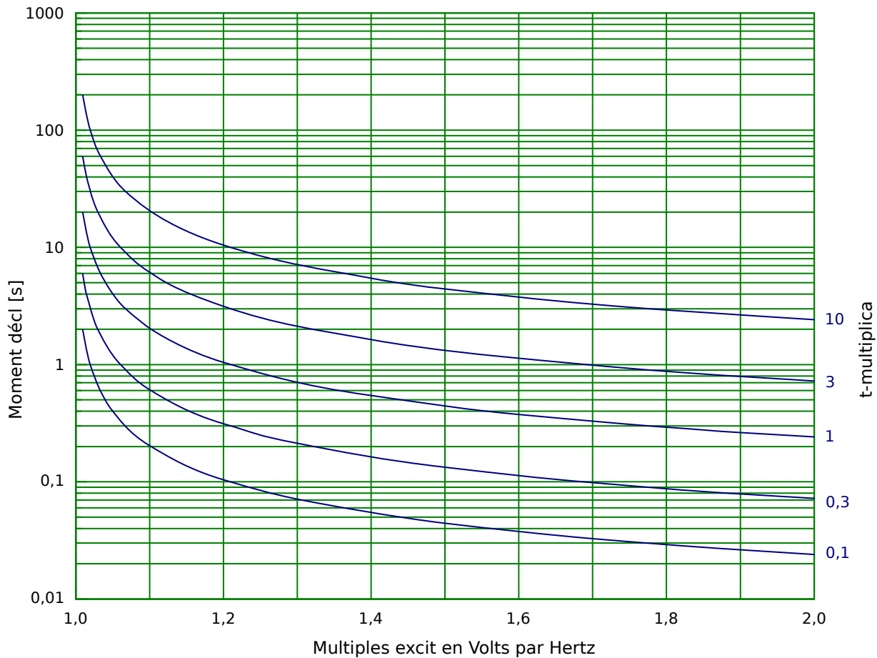
Fig. 86: Caractéristiques / forme de la courbe : INV C
