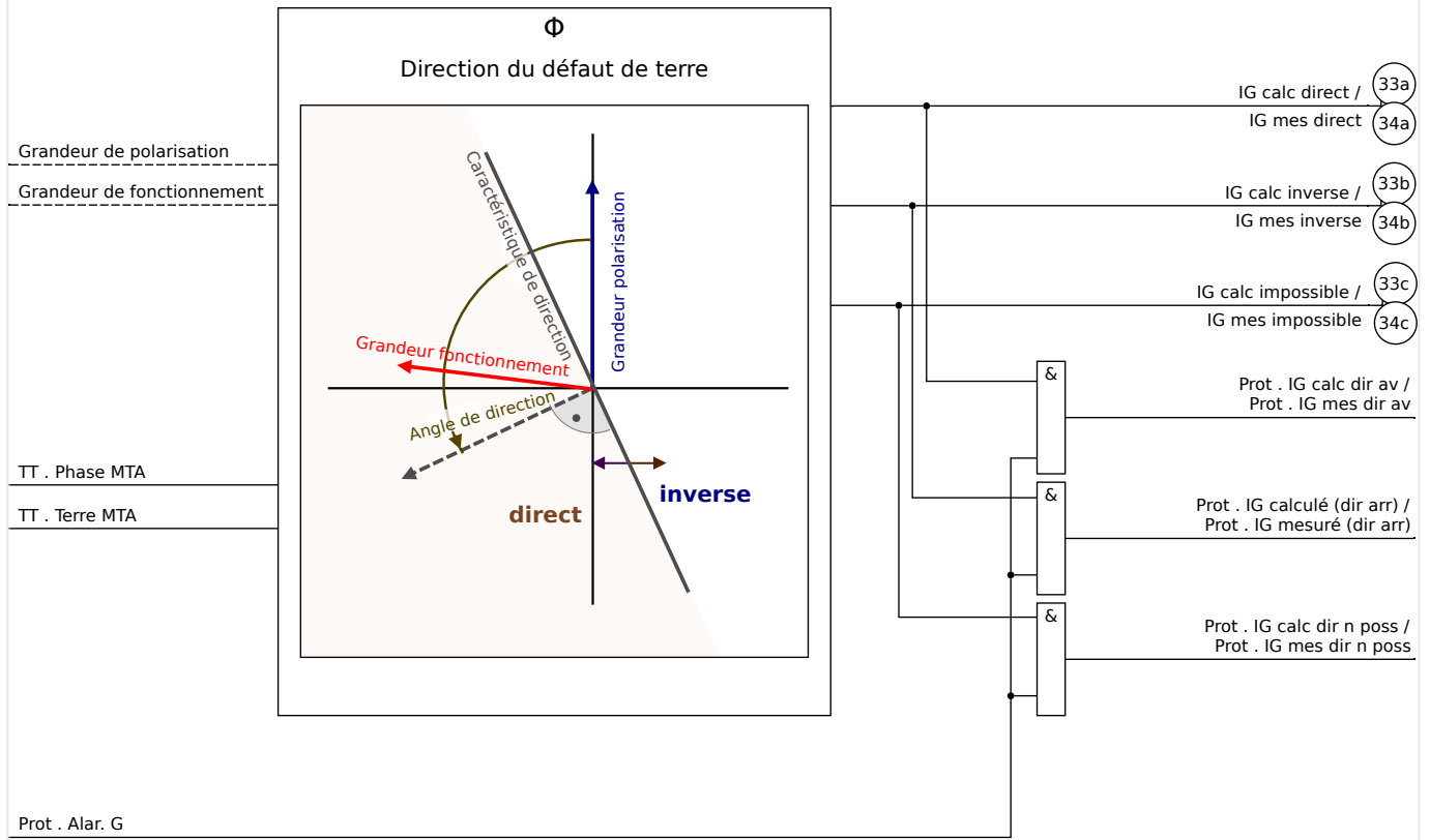
Fig. 68: Détermination de la direction pour toutes les méthodes excepté « \cos(\phi) », « \sin(\phi) ».
