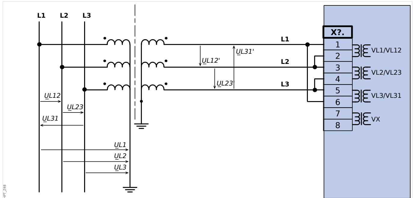
Fig. 36: Mesure de tension triphasée - câblage des entrées de mesure : "delta-connection" (Connexion en triangle).
