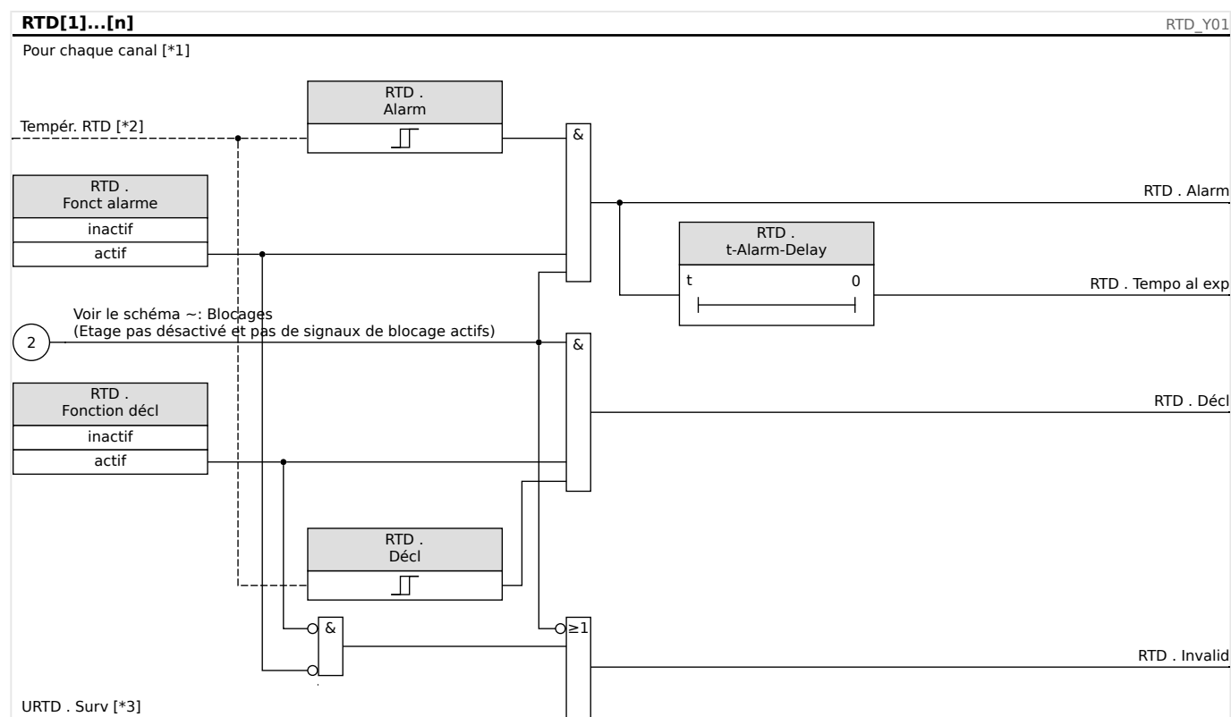
Fig. 119: Principe de fonctionnement général (alarme retardée, déclenchement non retardé).
