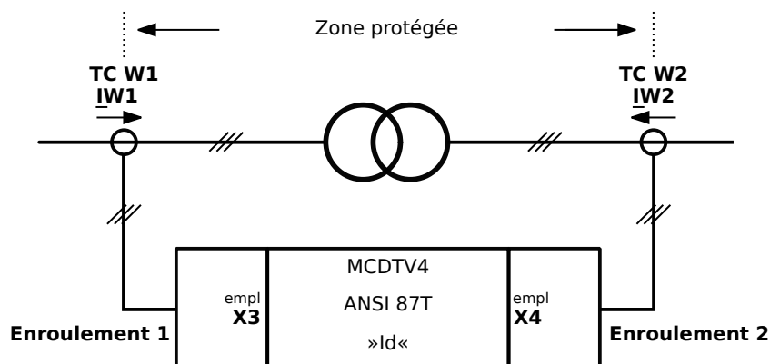
Fig. 74: ANSI 87T : Protection différentielle de phase de transformateur
