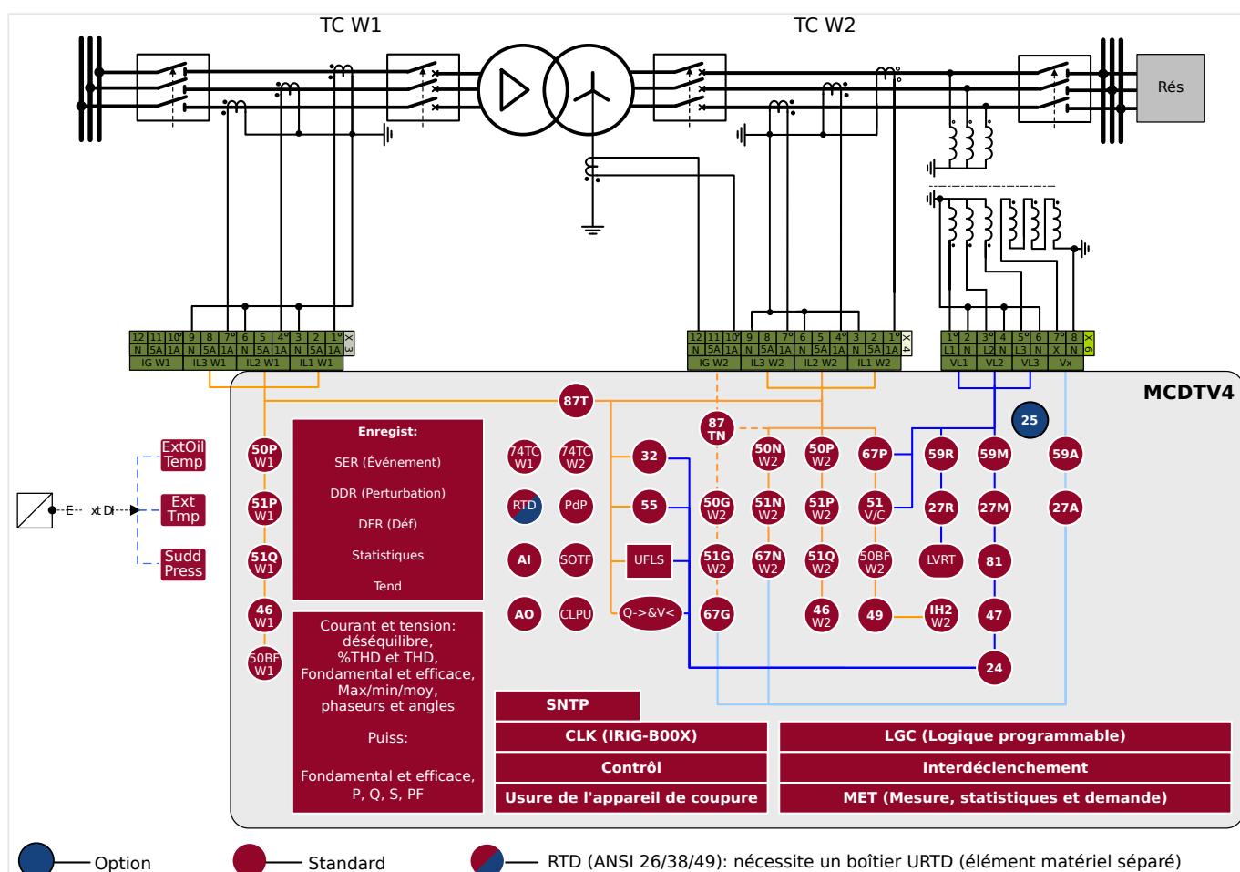
Fig. 1: Présentation fonctionnelle du MCDTV4.
