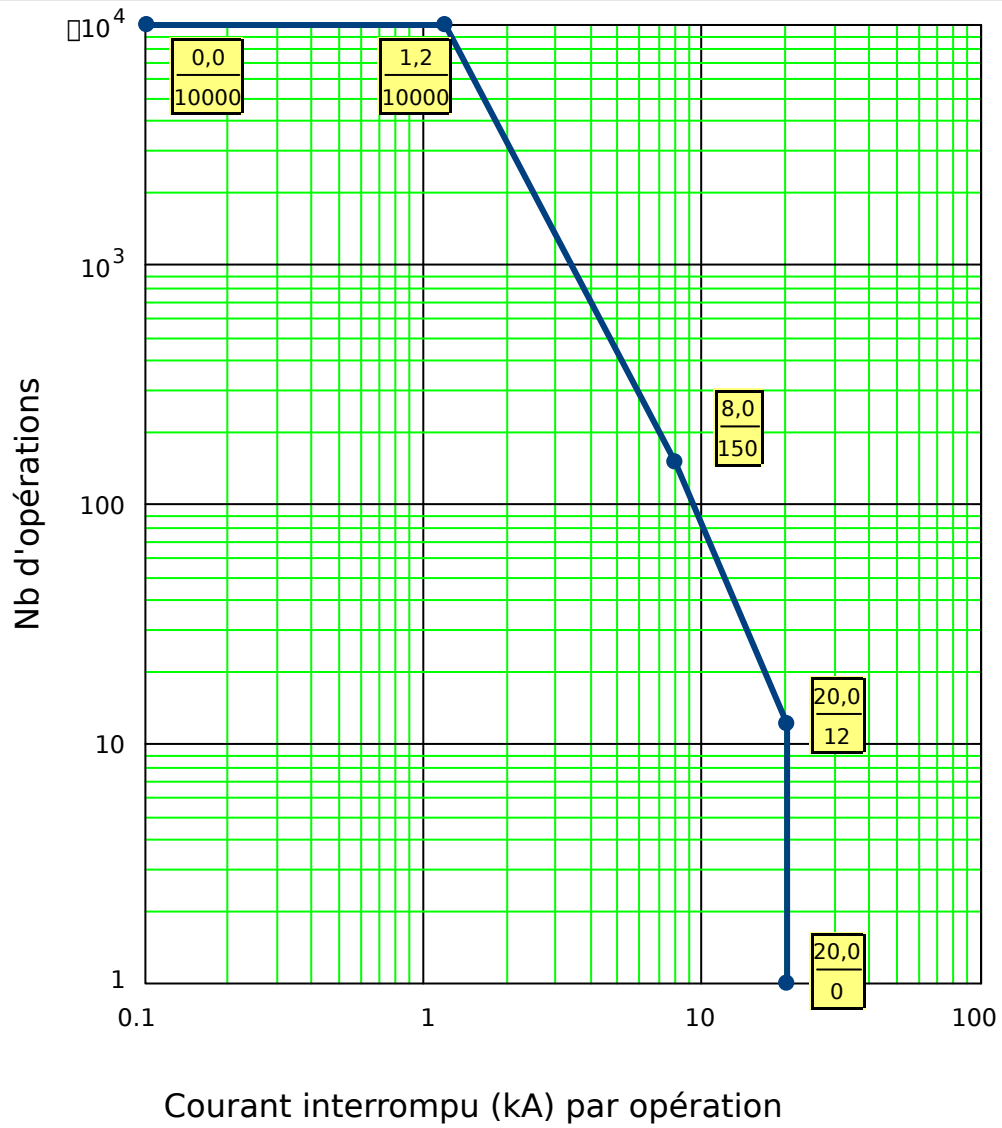
Fig. 129: Courbe de maintenance du disj pour un disj 25 ~kV typique
