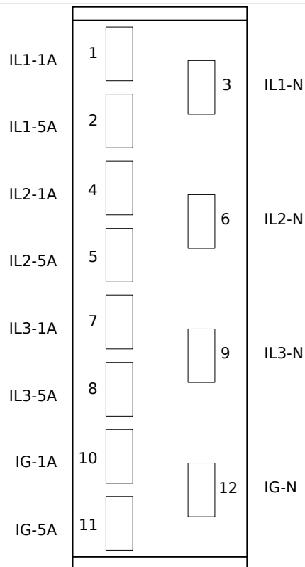
Fig. 19: TIs - Affectation électromécanique
