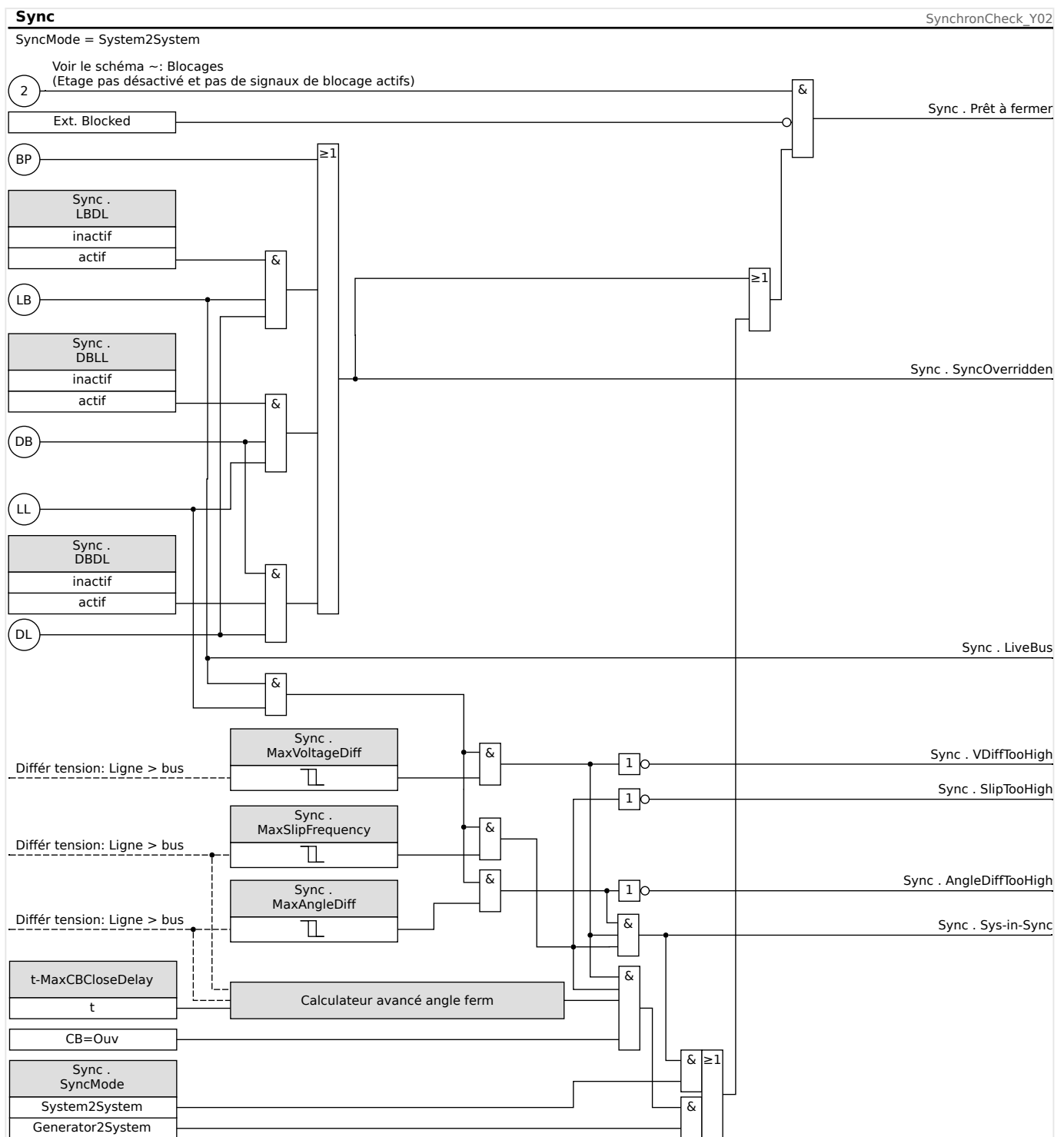
Fig. 101: Fonctionnalité du module «Sync», « System2System ».
