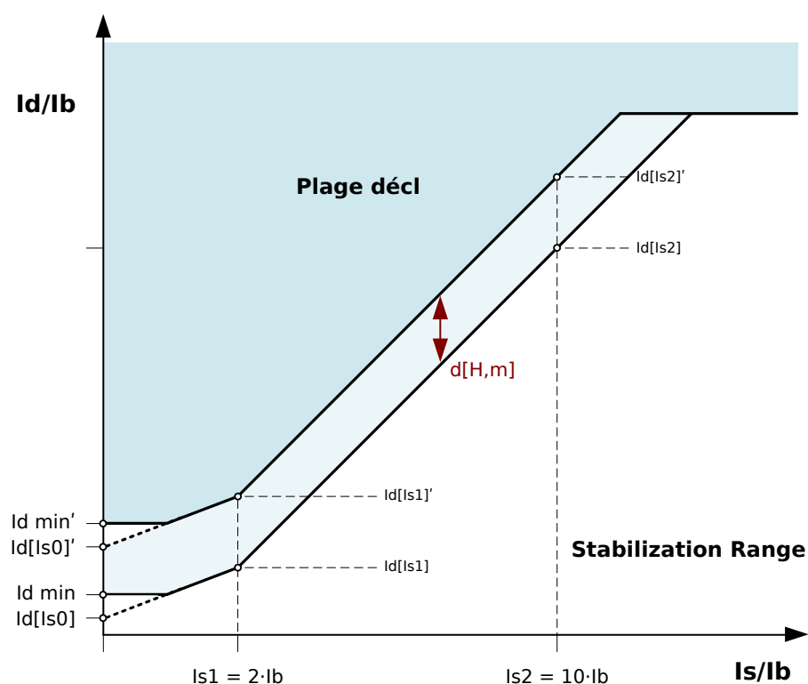
Fig. 76: Hausse dynamique temporaire de la caractéristique de déclenchement statique.
