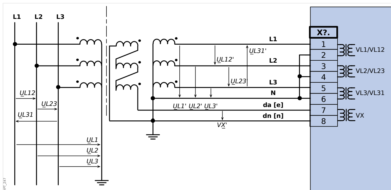
Fig. 35: VT Wye avec une connexion en triangle ouvert.
