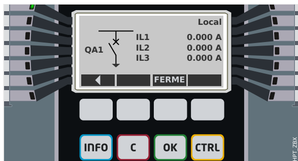
Fig. 126: Exemple de page de contrôle, avec le « disjoncteur » en position ouverte.
