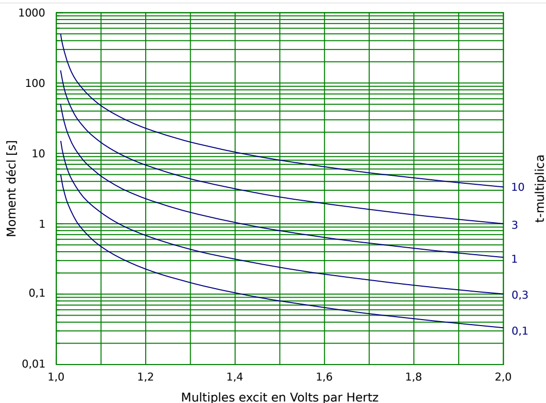
Fig. 84: Caractéristiques / forme de la courbe : INV A
