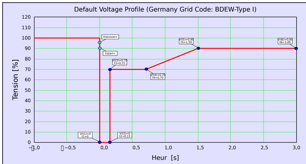
Fig. 116: Profil LVRT prédéfini en usine (BDEW-Type I).
