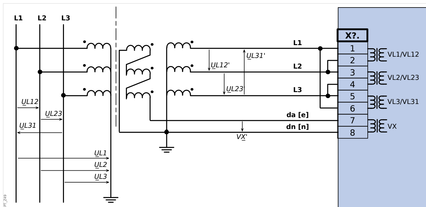
Fig. 37: Mesure de tension triphasée - câblage des entrées de mesure : "delta-connection" (Connexion en triangle). Mesure tension résid VG via enroults auxiliaires (e-n) "triangle fermé"
