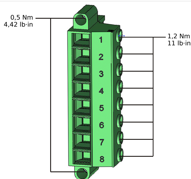
Fig. 143: Bornes de mesure de tension de la carte de mesure « TU » (➡ « 2.8.1 TU - Entrées de mesure de tension »).
