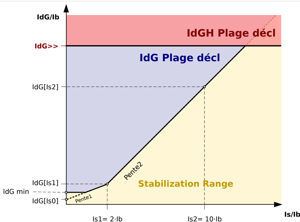
Fig. 80: Valeur d'excitation »IdG>>« du courant différentiel à la terre en fonction du courant nominal »Ib« de l'objet de protection associé.
