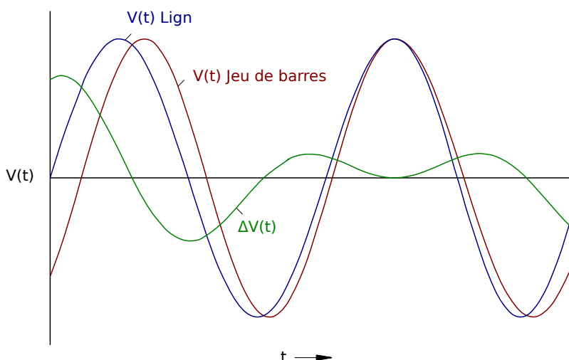
Fig. 99: Courbe de tension avec résolution agrandie
