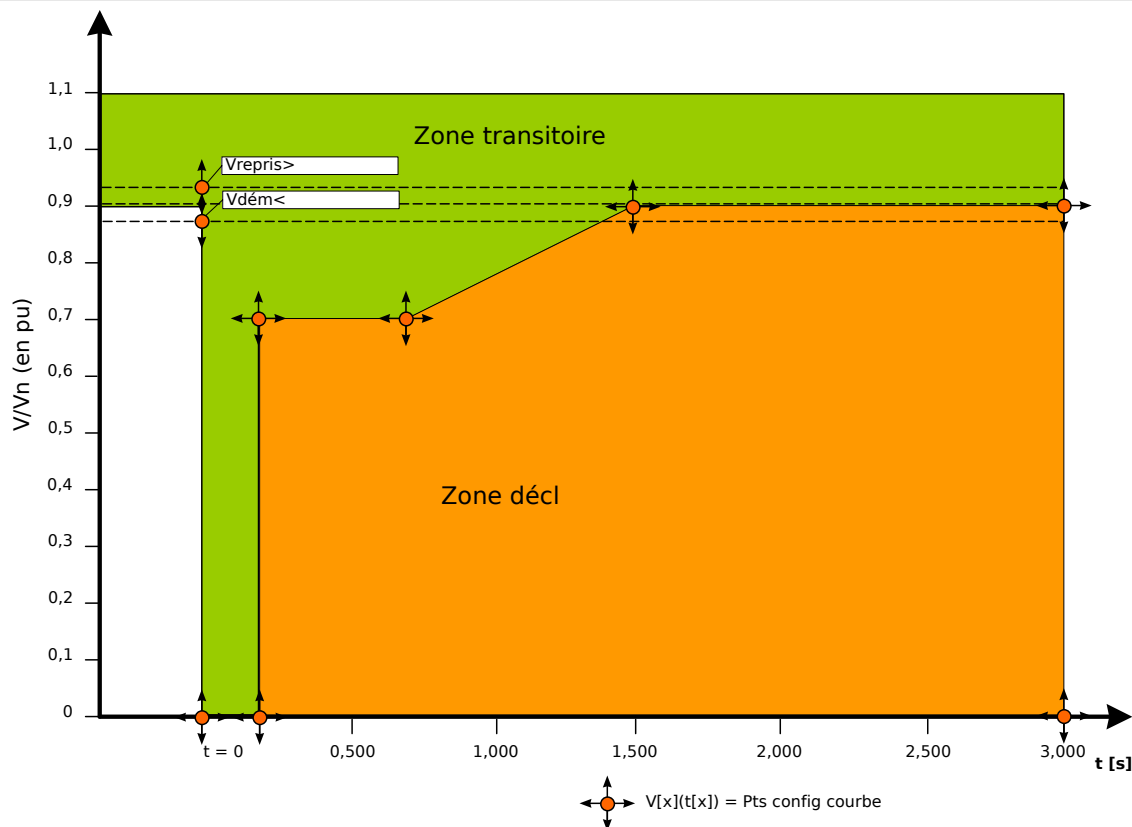
Fig. 115: Zone transitoire et zone de déclenchement
