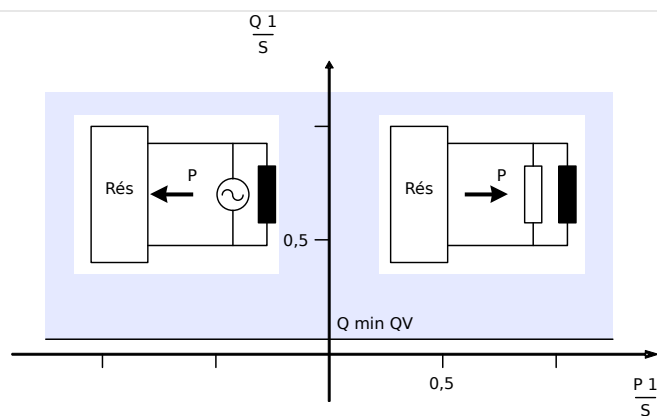
Fig. 104: Méthode 2 : Surveillance de la puissance réactive pure
