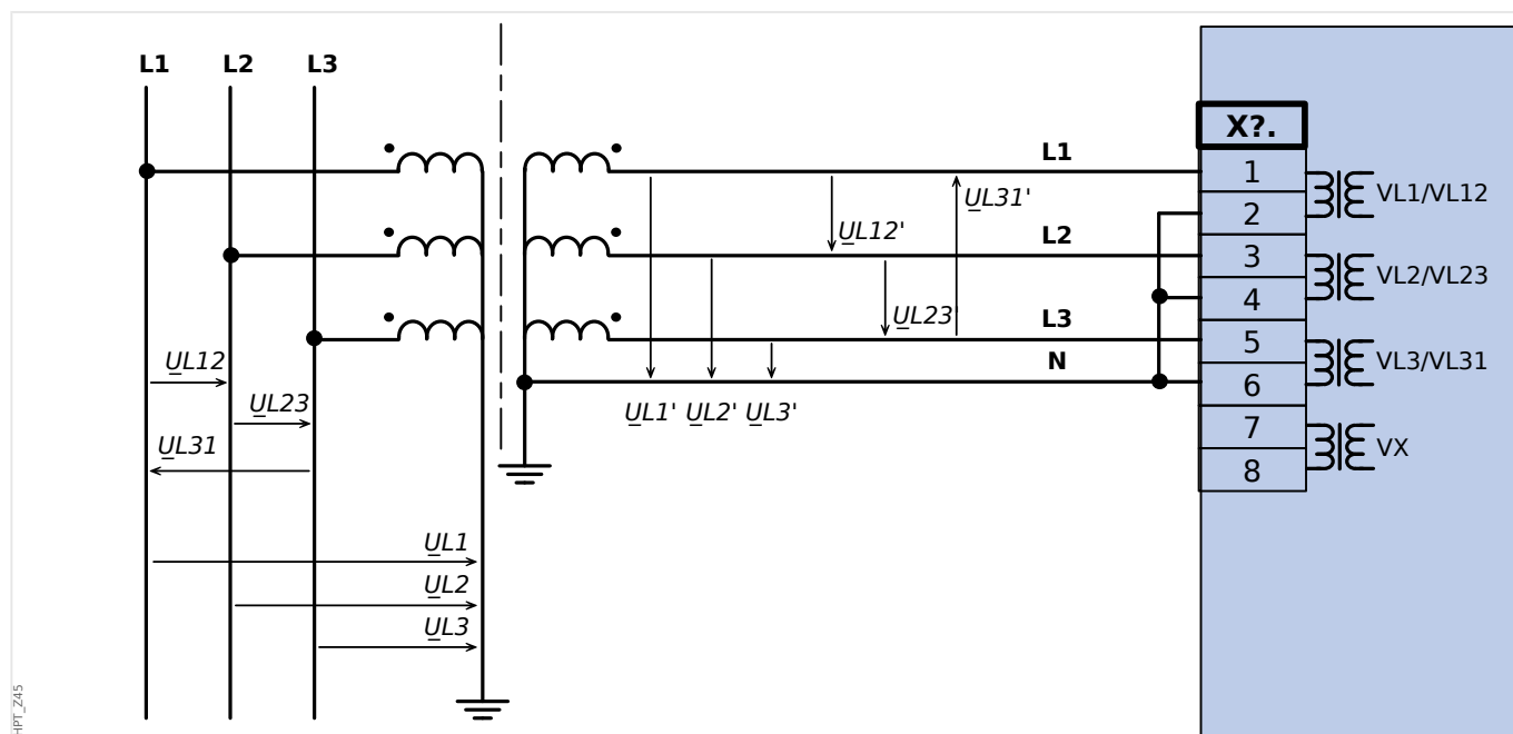
Fig. 34: VT Wye : Mesure de tension triphasée - câblage des entrées de mesure: "connex étoile"
