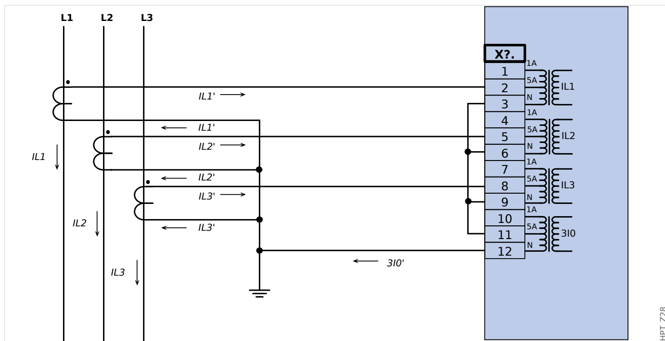
Rys. 22: Trójfazowy pomiar prądu; I_n wtórny = 5 A. Pomiar prądu doziemnego w układzie Holmgreena 3I_{0n} wtórny = 5 A.
