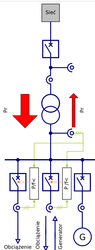
Rys. 108: Zdecentralizowane podczęstotliwościowe zmniejszanie obciążenia w sieciach z tymczasowym zasilaniem.
