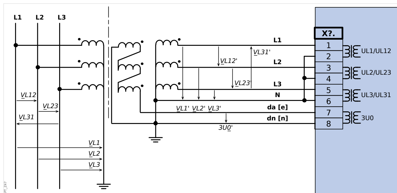
Rys. 35: Przekładnik napięciowy połączony w gwiazdę z otwartym trójkątem.
