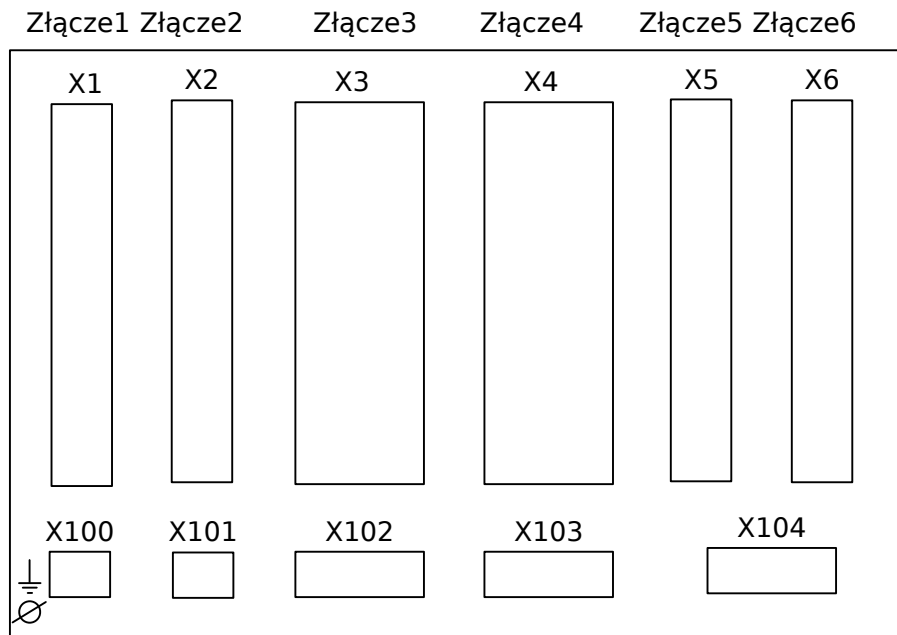
Rys. 7: Obudowa B2 — schemat.
