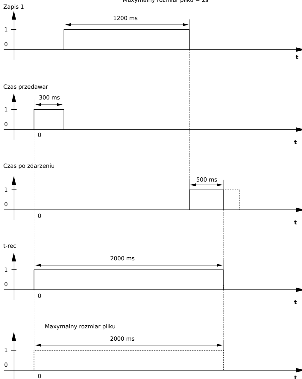
Rys. 132: Przykładowy wykres czasów pracy rejestratora zakłóceń I
