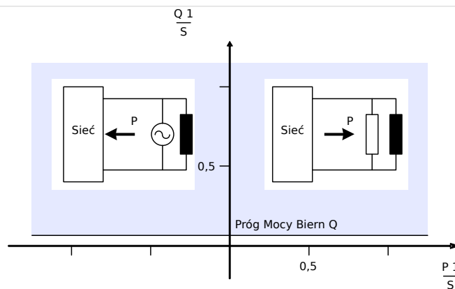
Rys. 104: Metoda 2: kontrola czystej mocy biernej.
