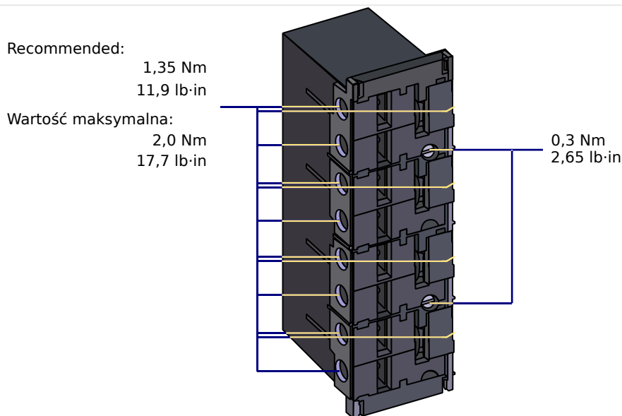
Rys. 142: Łącznik wtykowy ze zintegrowanym elementem zwarciovym (konwencjonalne wejścia prądowe)
