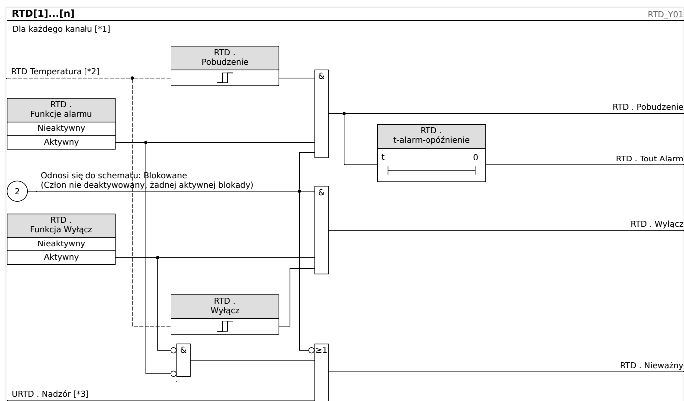
Rys. 119: Ogólna zasada działania (alarm z opóźnieniem, wyzwolenie bezzwłoczne).
