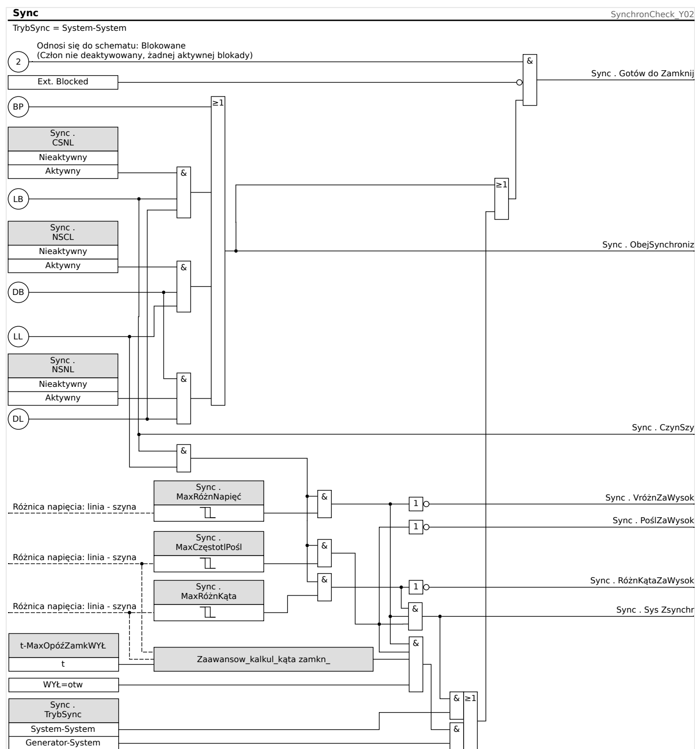
Rys. 101: Działanie modułu „Sync”, „System-System”.
