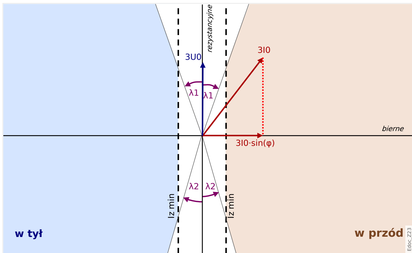
Rys. 70: Zasada określania kierunku metodą „sin(φ)”.
