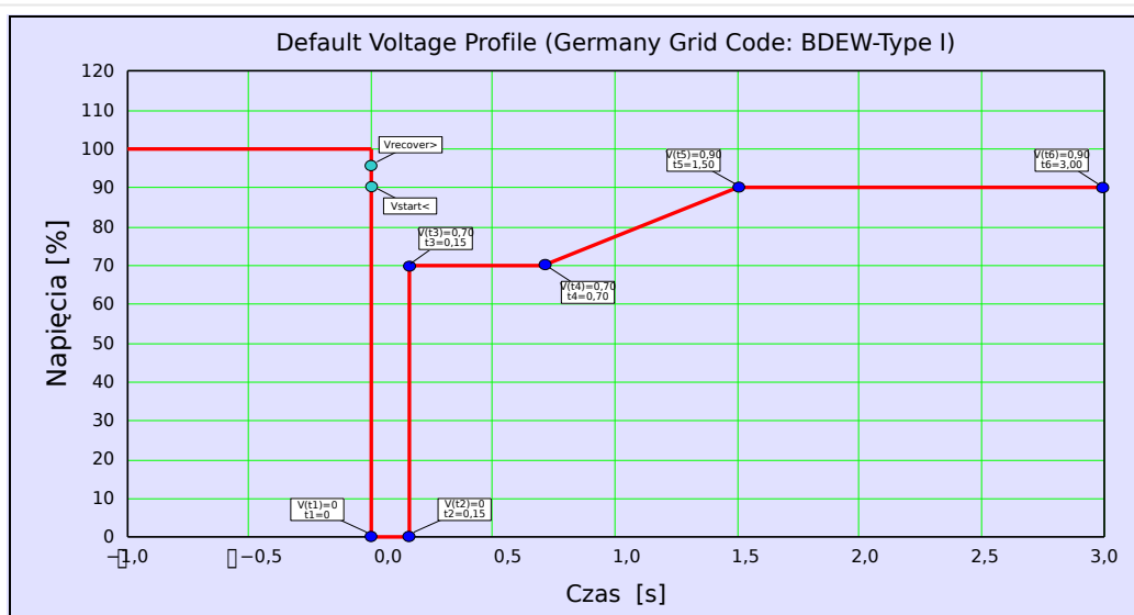
Rys. 116: Profil domyślny LVRT (BDEW typ I).
