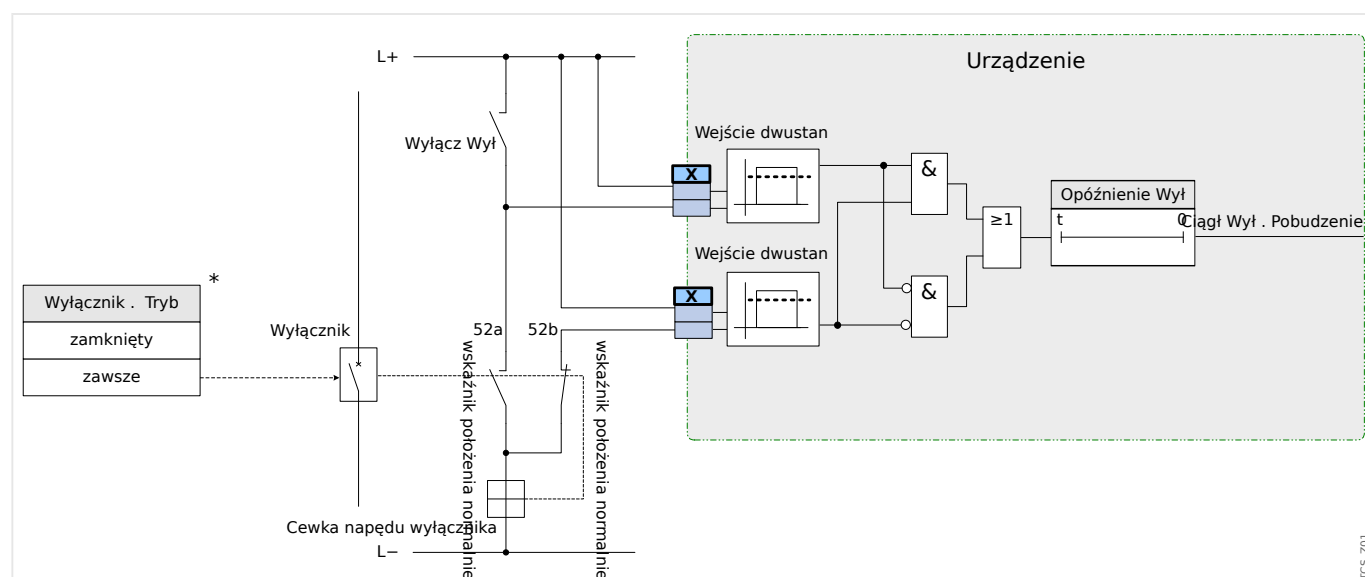
Rys. 120: Przykład okablowania: Układ kontroli ciągłości obwodów wyłącznika z dwoma stykami pomocniczymi wyłącznika „Położ ZAŁ” (52a) i „Położ WYŁ” (52b).
