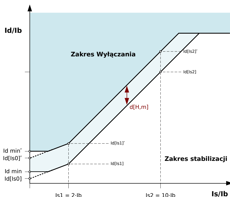
Rys. 76: Tymczasowe podniesienie dynamiczne charakterystyki wyzwania statycznego.
