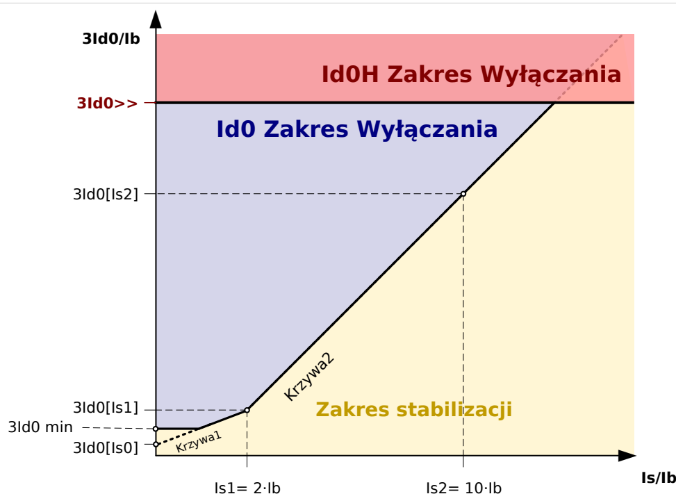
Rys. 80: Wartość pobudzenia „3Id0>>” prądu różnicowego doziemnego w oparciu o prąd znamionowy „Ib” obiektu zabezpieczanego.
