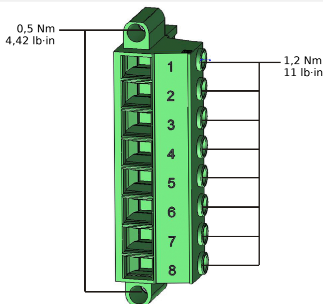
Rys. 143: Zaciski pomiaru napięcia karty pomiarowej „TU” (➡ „2.8.1 TU — wejścia do pomiaru napięcia”).
