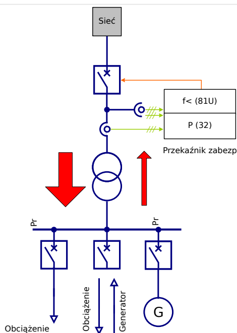
Rys. 107: Scentralizowane podczęstotliwościowe zmniejszanie obciążenia w sieciach z tymczasowym zasilaniem.
