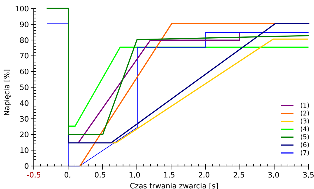
Rys. 113: Normy LVRT; źródło: eBWK Bd. 60 (2008) Nr 4. Autorzy: Dipl.-Ing. Thomas Smolka, Dr.-Ing. Karl-Heinz Weck, Zertifizierungstelle der FGH e.V., Mannheim, sowie Dipl.-Ing. (FH) Matthias Bartsch, Enercon GmbH, Aurich.
