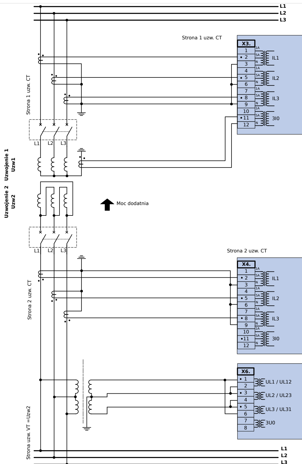
Rys. 40: Transformator DY z zabezpieczeniem różnicowoprądowym fazowym, REF w W1 i VT w W2 (połączenie V).
