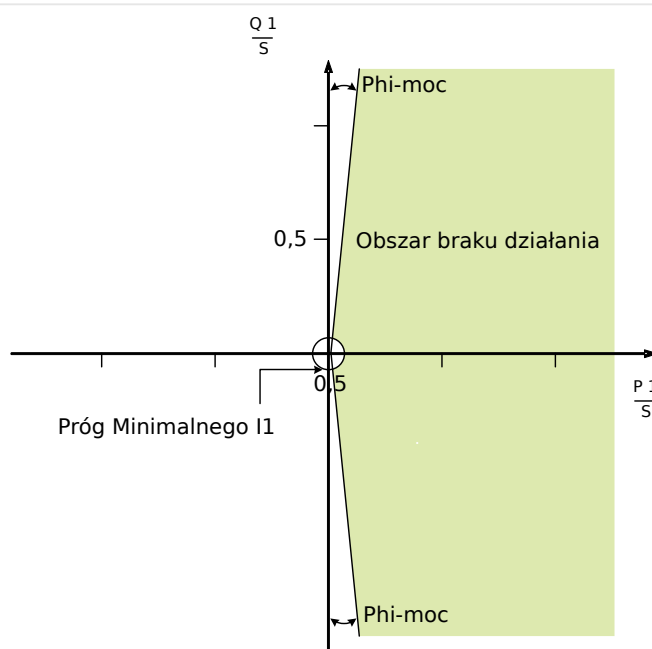
Rys. 111: Metoda 1 (kontrola kąta obciążenia): „Metoda UFLS” = „Nadzór kąta obciążenia”.
