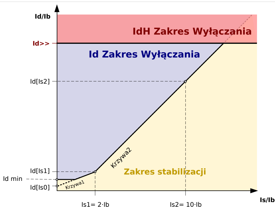
Rys. 75: Krzywe wyzwania funkcji zabezpieczających „Id” (obszar niebieski) i „IdH” (obszar czerwony).
