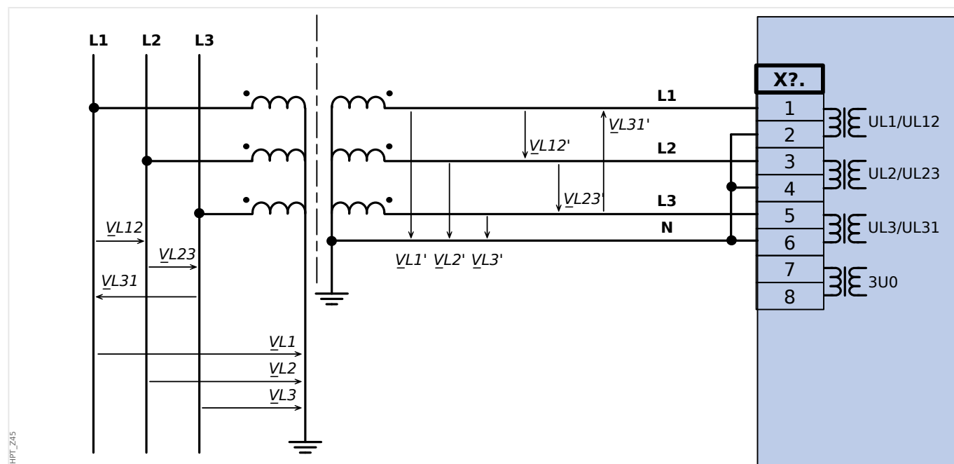
Rys. 34: Przekładnik napięciowy połączony w gwiazdę: Trójfazowy pomiar napięcia w układzie gwiazdy
