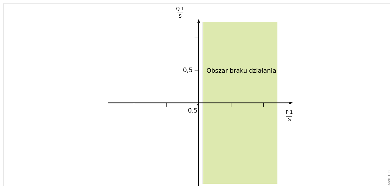
Rys. 112: Metoda 2 (kontrola czystej mocy czynnej). „Metoda UFLS” = „Nadzór Czystej Mocy Czyn”.
