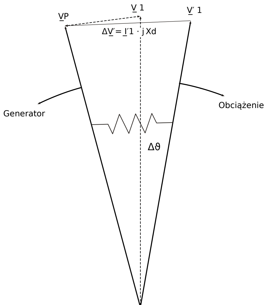
Rys. 95: Wektory napięcia przy awarii sieci.
