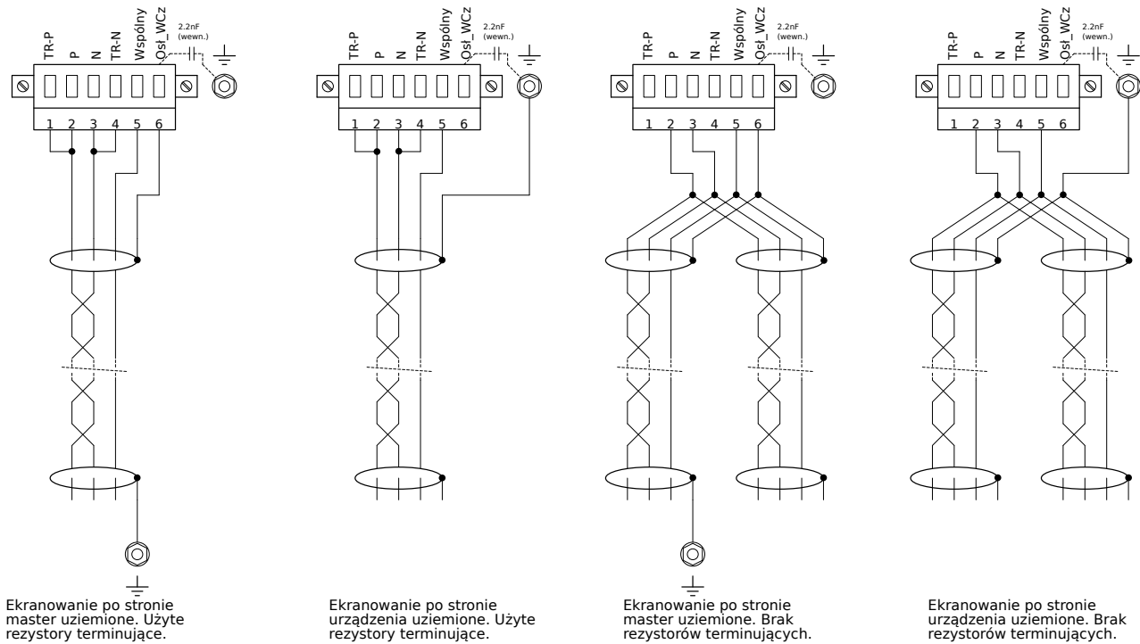
Rys. 51: Opcje ekranowania (3 żyły i ekran)
