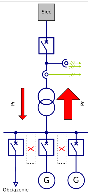
Rys. 110: Zastosowanie zdecentralizowane w sieciach z przeważającym zasilaniem.
