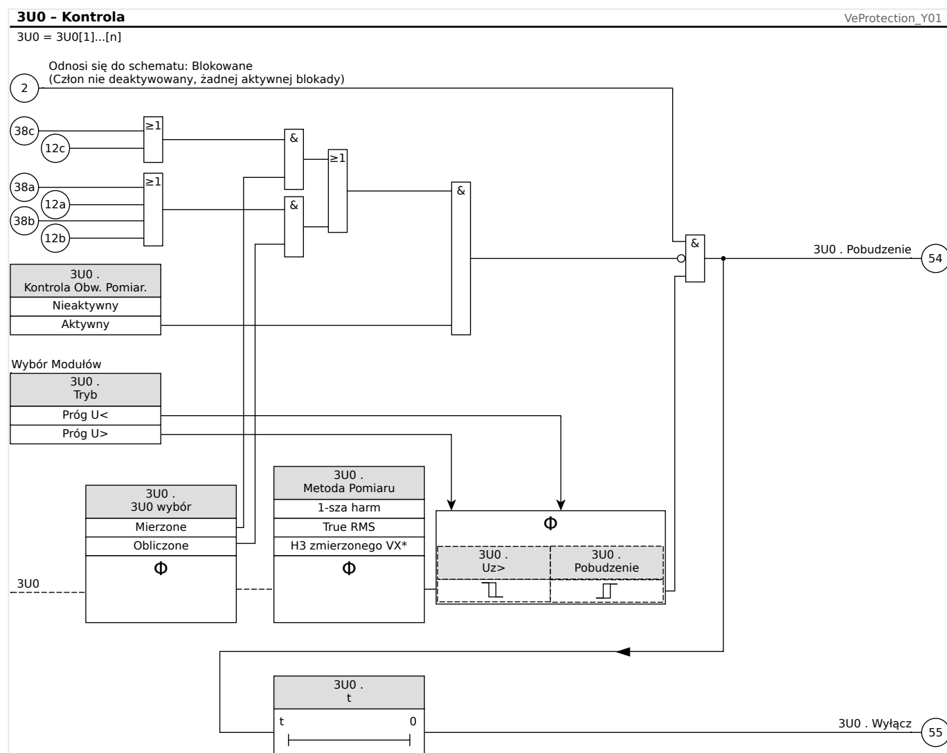
Rys. 90: Kontrola napięcia U0, UX, część 1 (funkcja kontroli, decyzja o wyzwoleniu).
