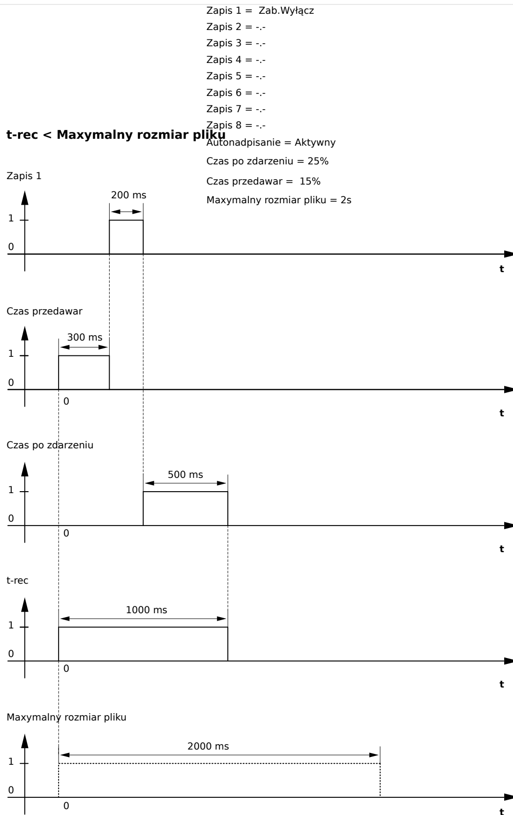
Rys. 133: Przykładowy wykres czasów pracy rejestratora zakłóceń II
