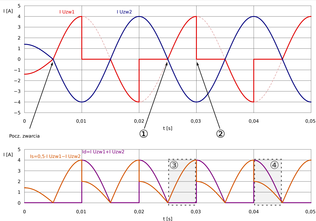
Rys. 77: Charakterystyka I_d i I_s z nasyceniem po stronie W1 przekładnika prądowego w przypadku zwarcia zewnętrznego.
