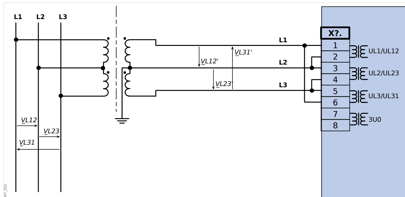
Rys. 38: Pomiar napięcia dla dwóch faz w układzie otwartego trójkąta
