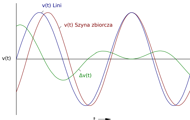
Rys. 99: Krzywa napięciowa ze zwiększoną rozdzielczością.
