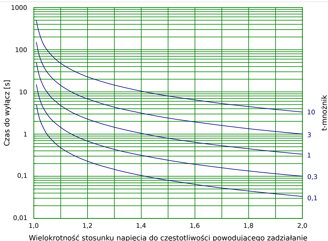
Rys. 84: Kształt krzywej/charakterystyki: ODW A
