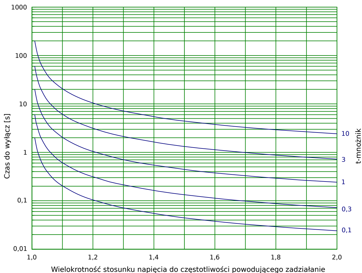
Rys. 86: Kształt krzywej/charakterystyki: ODW C
