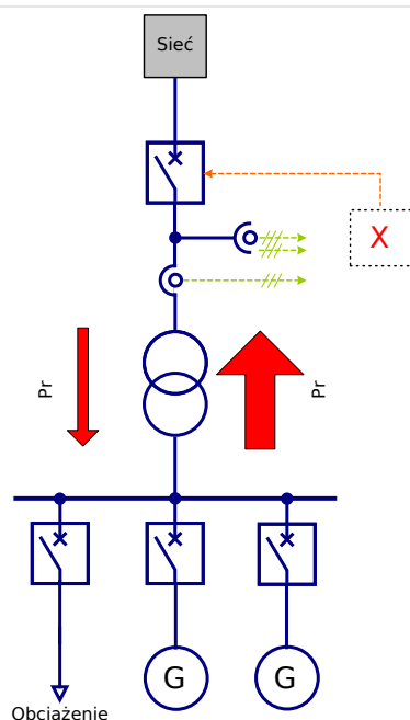
Rys. 109: Zastosowanie scentralizowane w sieciach z przeważającym zasilaniem.
