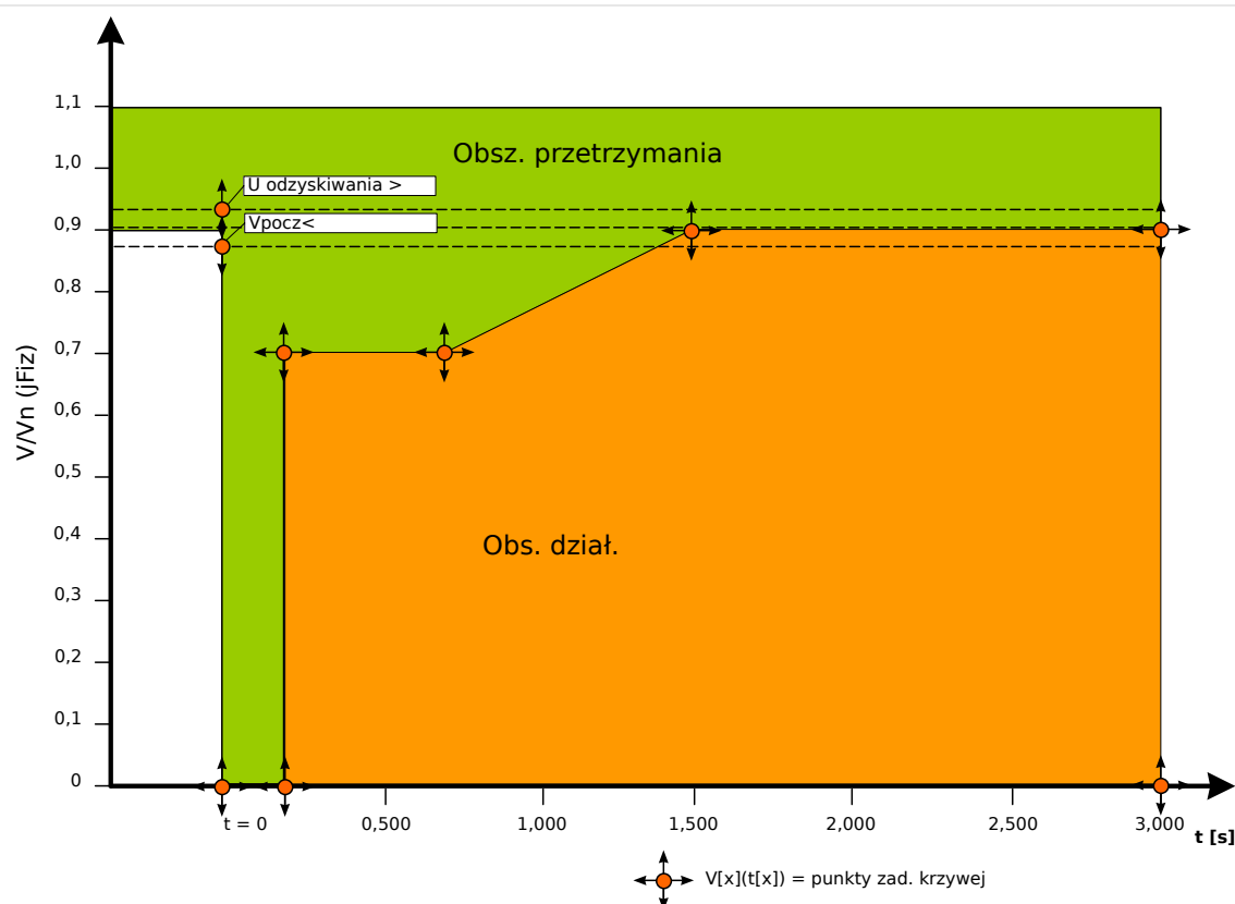
Rys. 115: Obszar „przetrzymania” i obszar „wyzwolenia”.
