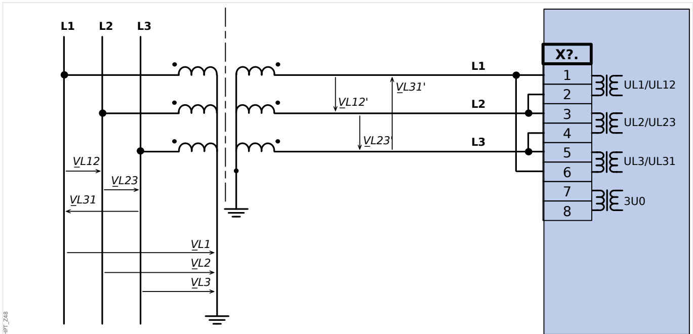
Rys. 36: Trójfazowy pomiar napięcia w układzie trójkąta: połączenie przewodów wejść pomiarowych: "połączenie w trójkąt"
