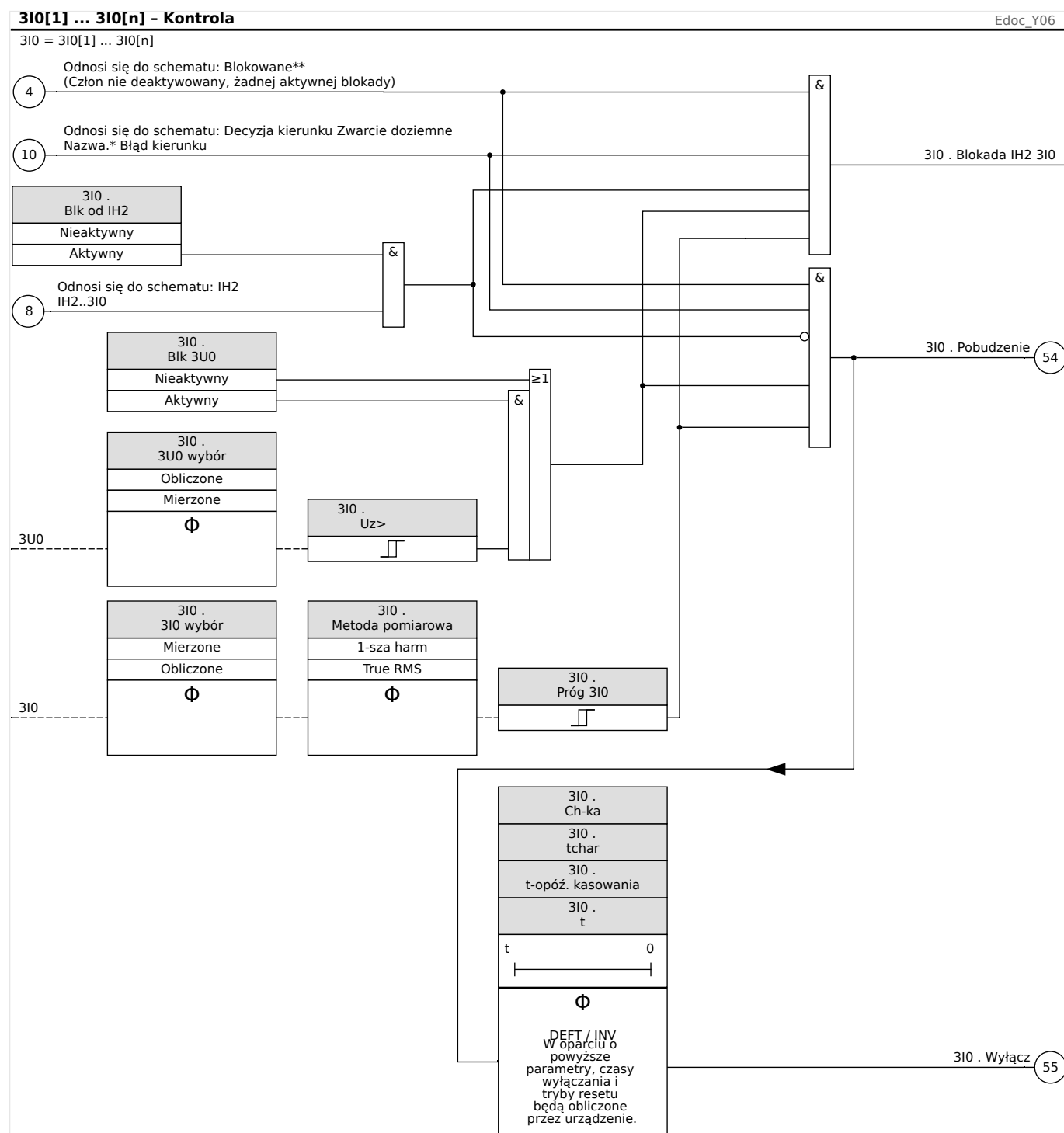
Rys. 81: Zabezpieczenie nadprądowe ziemnozwarciowe, część 1 (funkcja kontroli, decyzja o wyzwoleniu).
