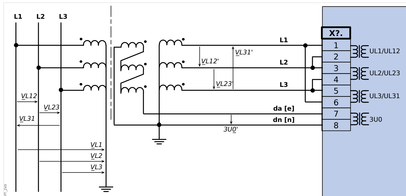
Rys. 37: Trójfazowy pomiar napięcia w układzie trójkąta: połączenie przewodów wejść pomiarowych: "połączenie w trójkąt" Pomiar 3U_0 napięcia szczytkowego poprzez dodatkowe uzwojenia (e-n) w układzie otwartego trójkąta
