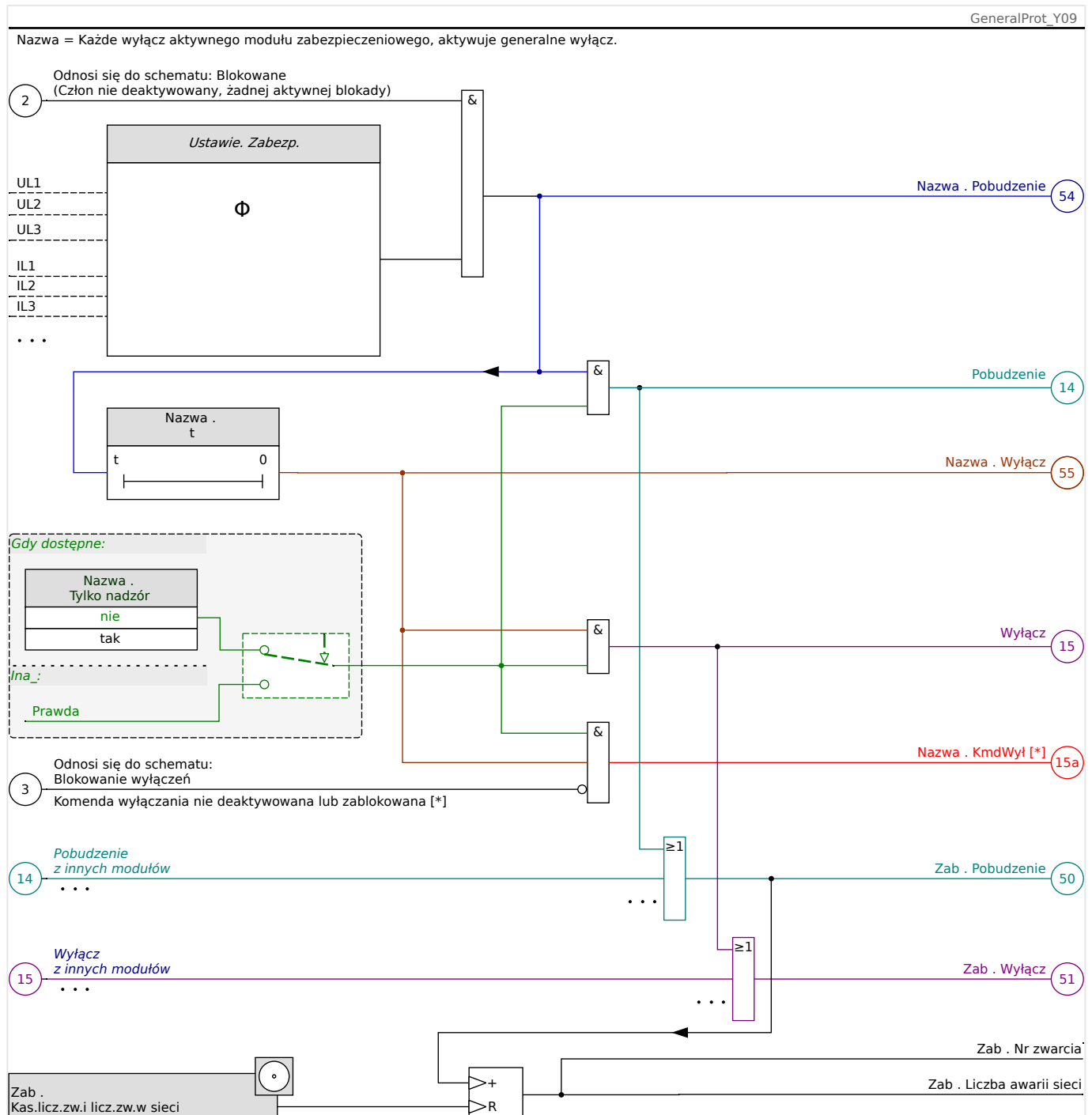
Rys. 64: Schemat ogólny działania każdego elementu zabezpieczającego HighPROTEC.
