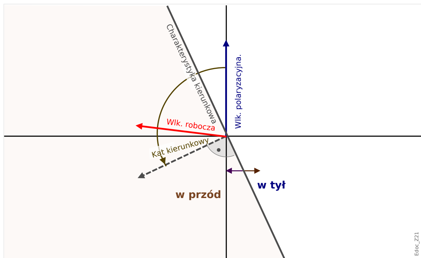
Rys. 67: Zasada określania kierunku obowiązująca dla wszystkich metod z wyjątkiem „ \cos(\phi) ”, „ \sin(\phi) ”.
