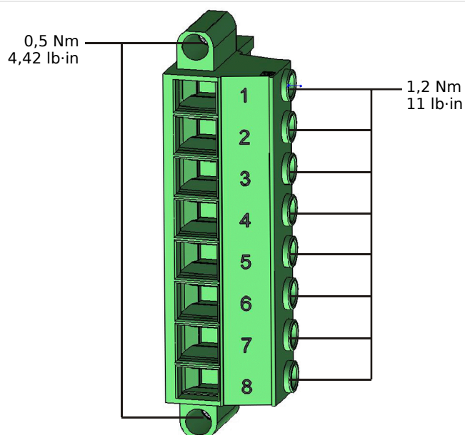
Fig. 143: Terminais de medição de tensão da placa de medição "TU" (↳ "2.8.1 TU - Entradas de Medição de Tensão").
