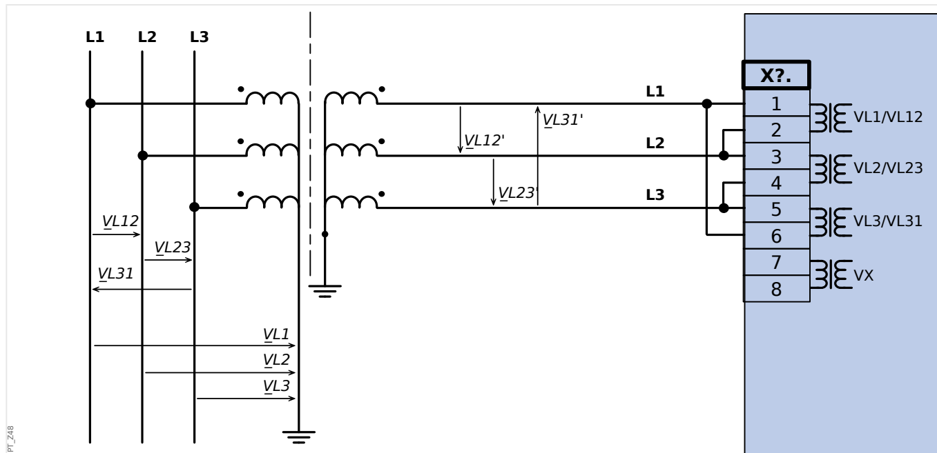
Fig. 36: Medição de tensão trifásica - fiação das entradas de medição: "conexão-delta"
