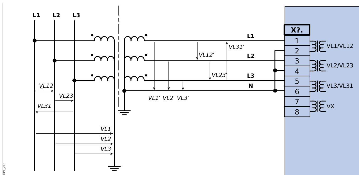
Fig. 34: VT Wye: Medição de voltagem trifásica - fiação das entradas de medição: "conexão estrela"
