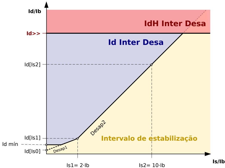
Fig. 75: As curvas de disparo das funções de proteção de “Id” (área azul) e de “IdH” (área vermelha).
