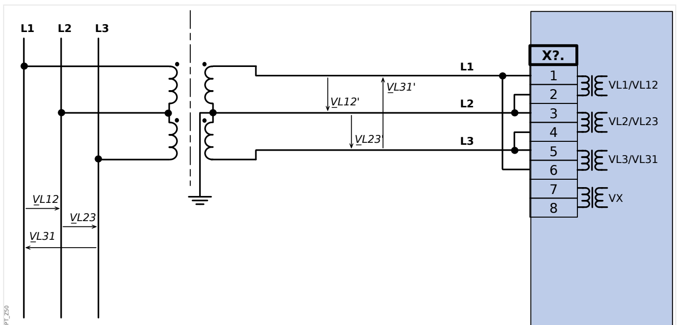
Fig. 38: Medição de tensão bifásica - fiação das entradas de medição: "Delta Aber"
