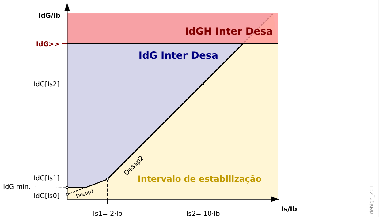
Fig. 80: Valor de arranque " I_{dG}>> " da corrente diferencial de aterramento com base na corrente nominal " I_b " do objeto de proteção relacionado.
