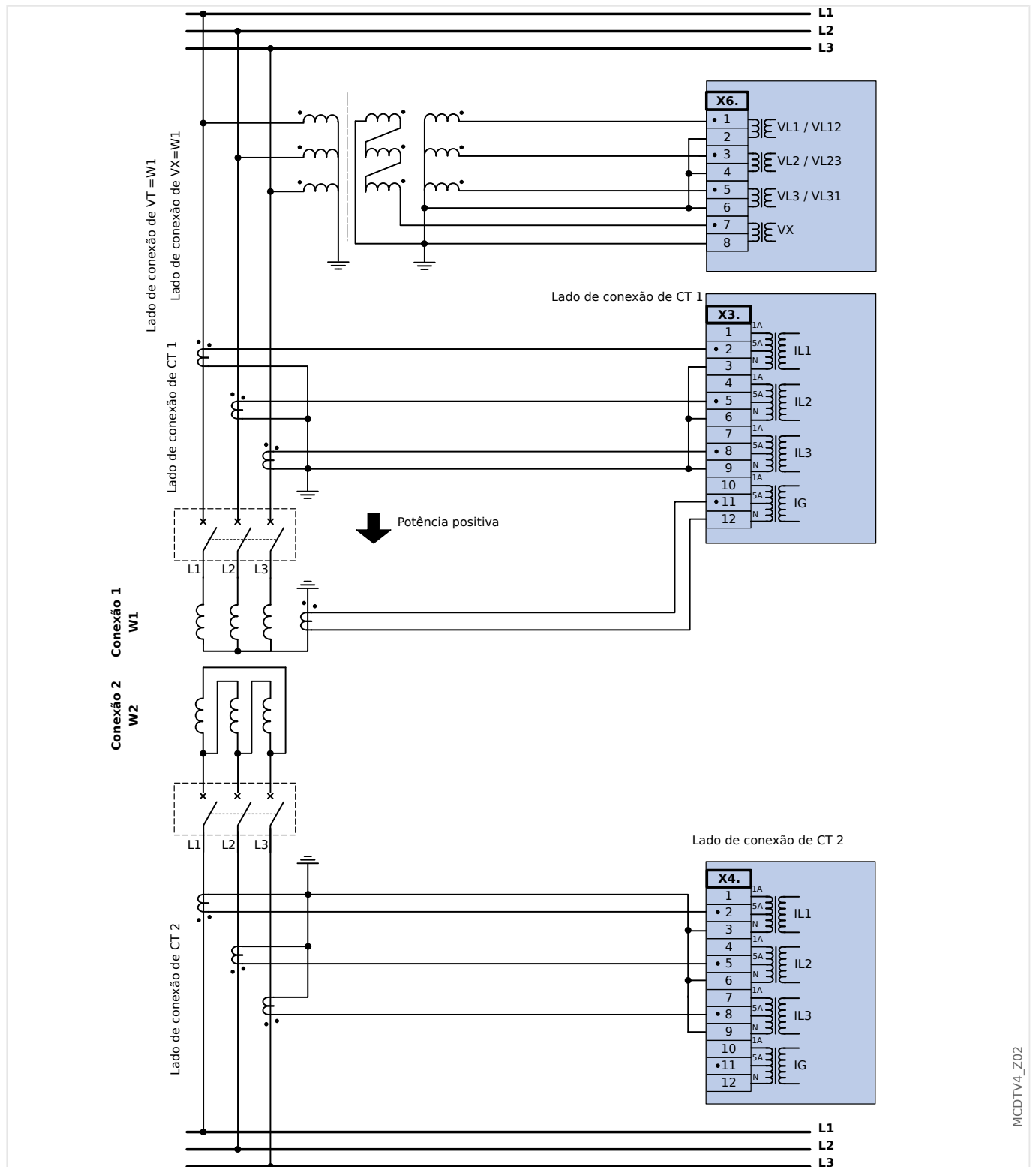
Fig. 39: Transformador DY com Proteção Diferencial de Fase e Proteção Diferencial de Terra no W1 apenas.
