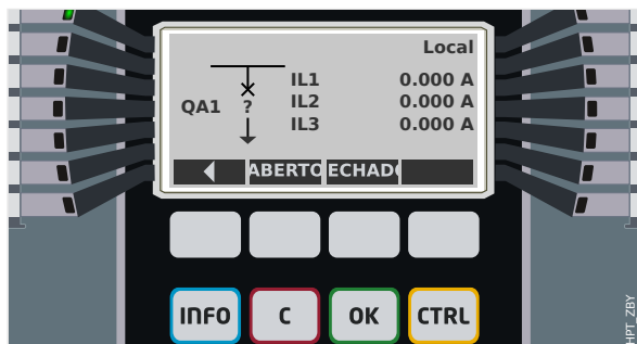
Fig. 125: Exemplo de página de controle, com o "Disjuntor" na posição de falha (ou implausível).
