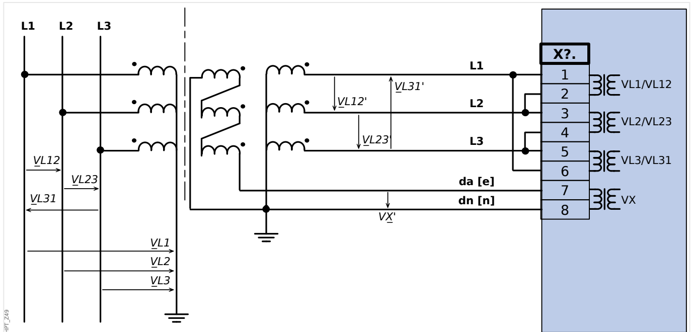
Fig. 37: Medição VG tensão residual por meio de "delta aberto" (e-n) de circuito auxiliar
