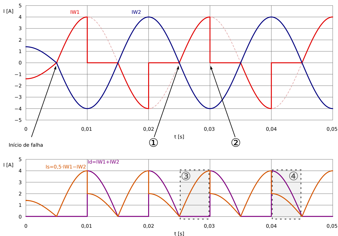
Fig. 77: Característica de I_d e I_s com a saturação no lado W1 para uma falha externa.
