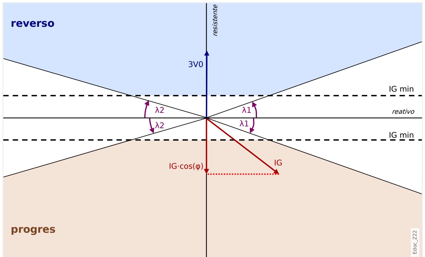
Fig. 69: Princípio de determinação da direção para o método " \cos(\phi) ".
