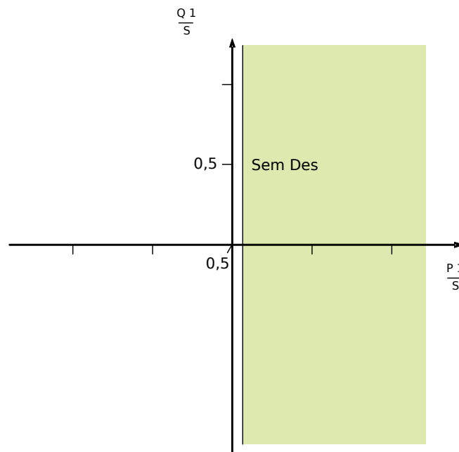
Fig. 112: Método 2 (Supervisão de Energia Ativa Pura): “Método UFLS” = “Superv. de Energia Ativa Pura”.
