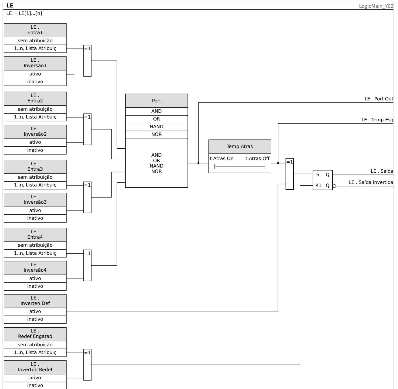
Fig. 136: Visão Geral Detalhada - Diagrama Lógico Geral.
