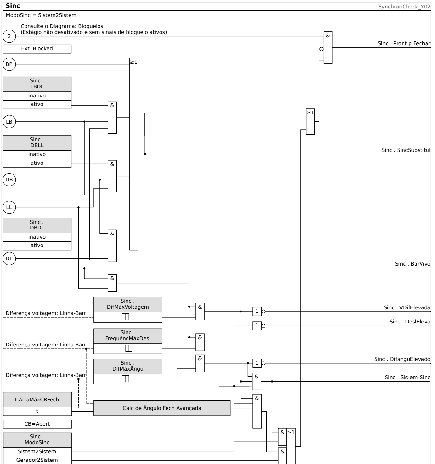
Fig. 101: Funcionalidade do módulo »Sinc«, "Sistem2Sistem".
