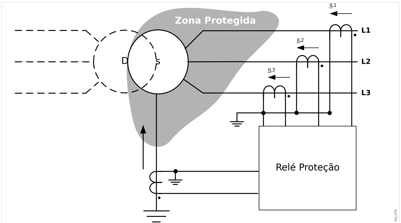
Fig. 79: Princípio de Proteção da Proteção Diferencial de Corrente de Aterramento no enrolamento lateral wye do transformador.
