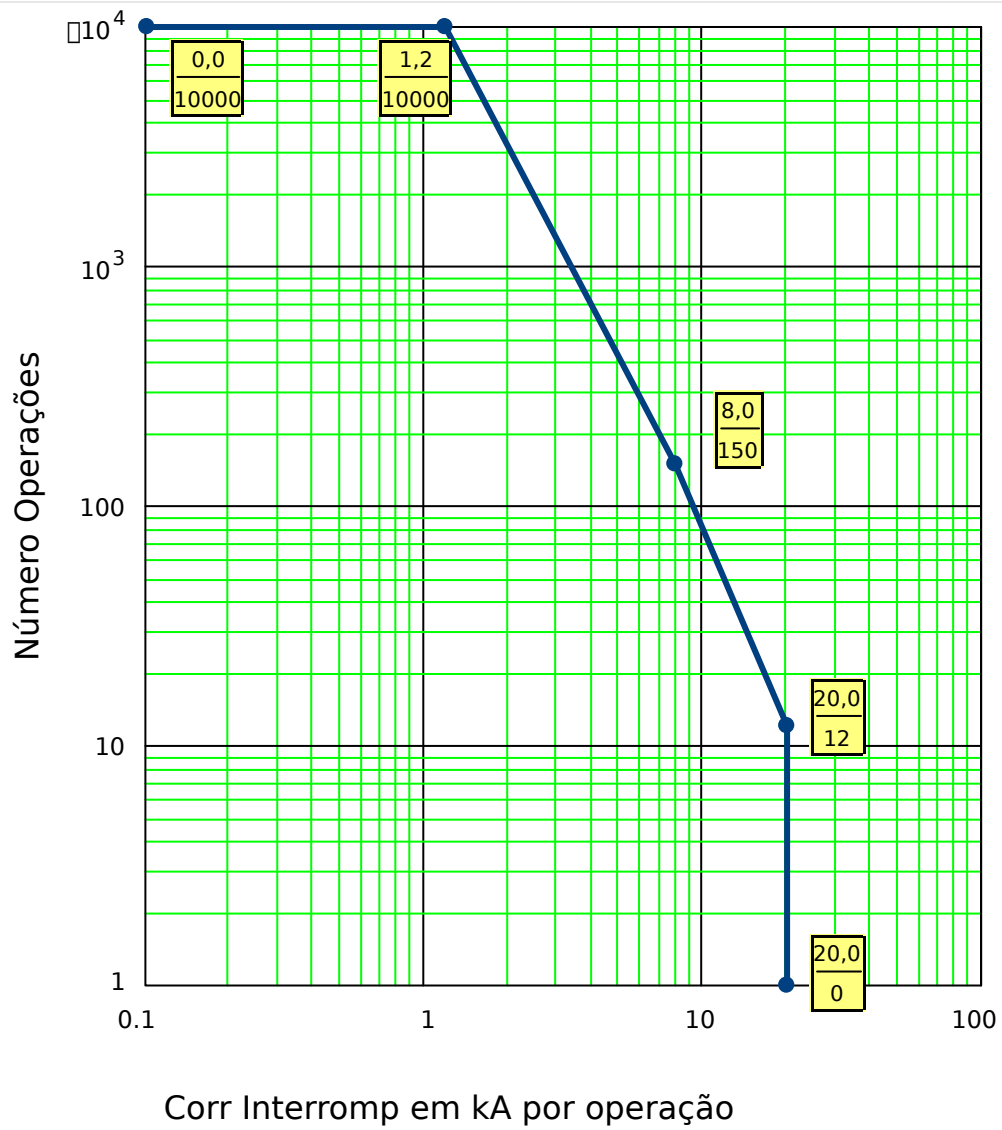
Fig. 129: Curva Manutenção de Disjuntor para Disjuntor normal 25kV
