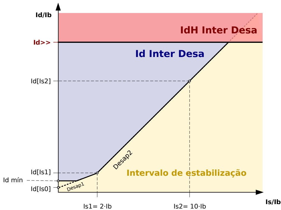
Fig. 78: Etapa da Proteção Diferencial Irrestrita de Alta Definição IdH.
