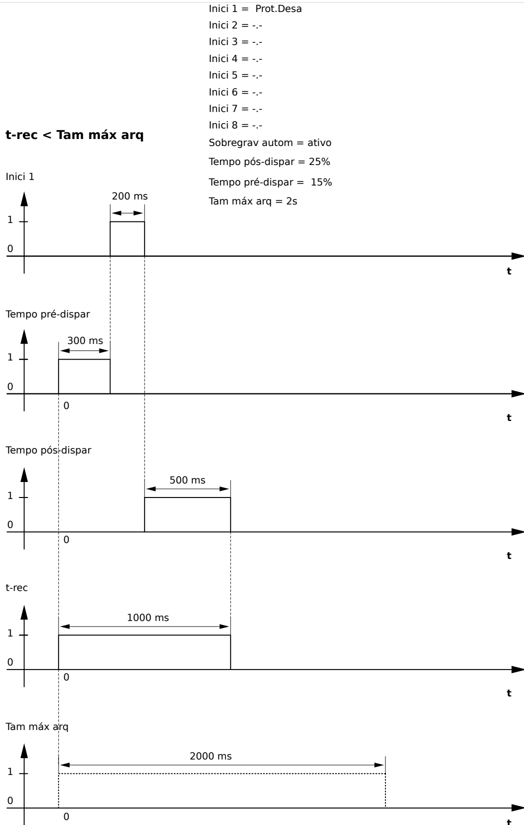
Fig. 133: Exemplo de Gráfico de Prazo do Gravador de Perturbação II
