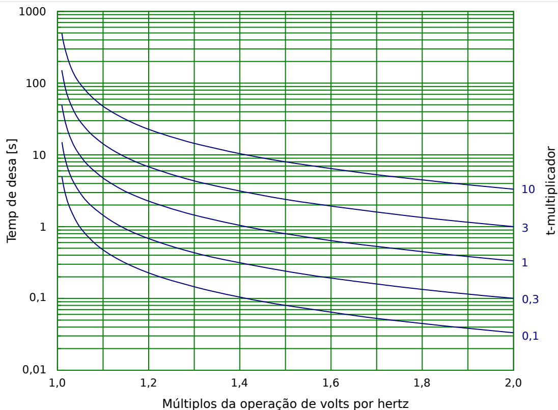
Fig. 84: Característica/formato da curva: INV A
