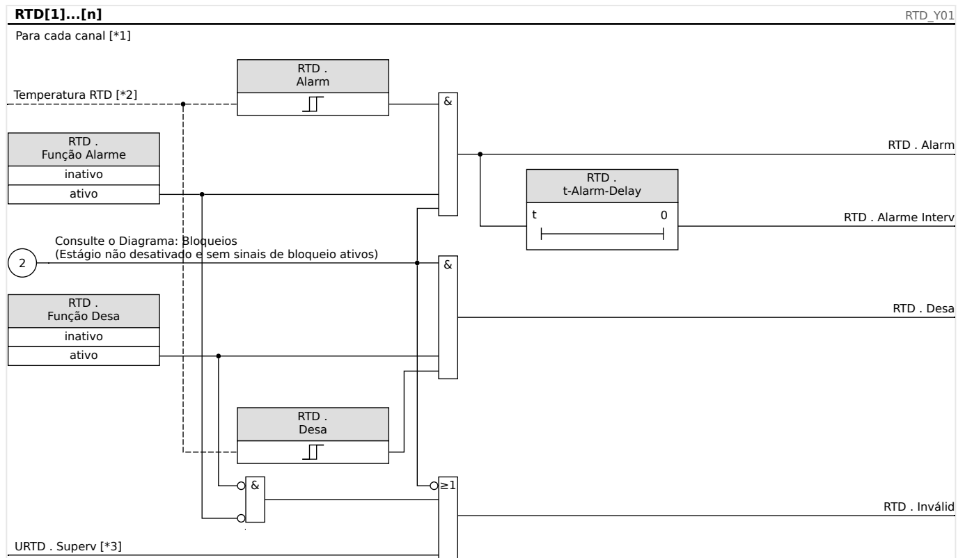
Fig. 119: O princípio geral de funcionamento (alarme atrasado, disparo sem atraso).
