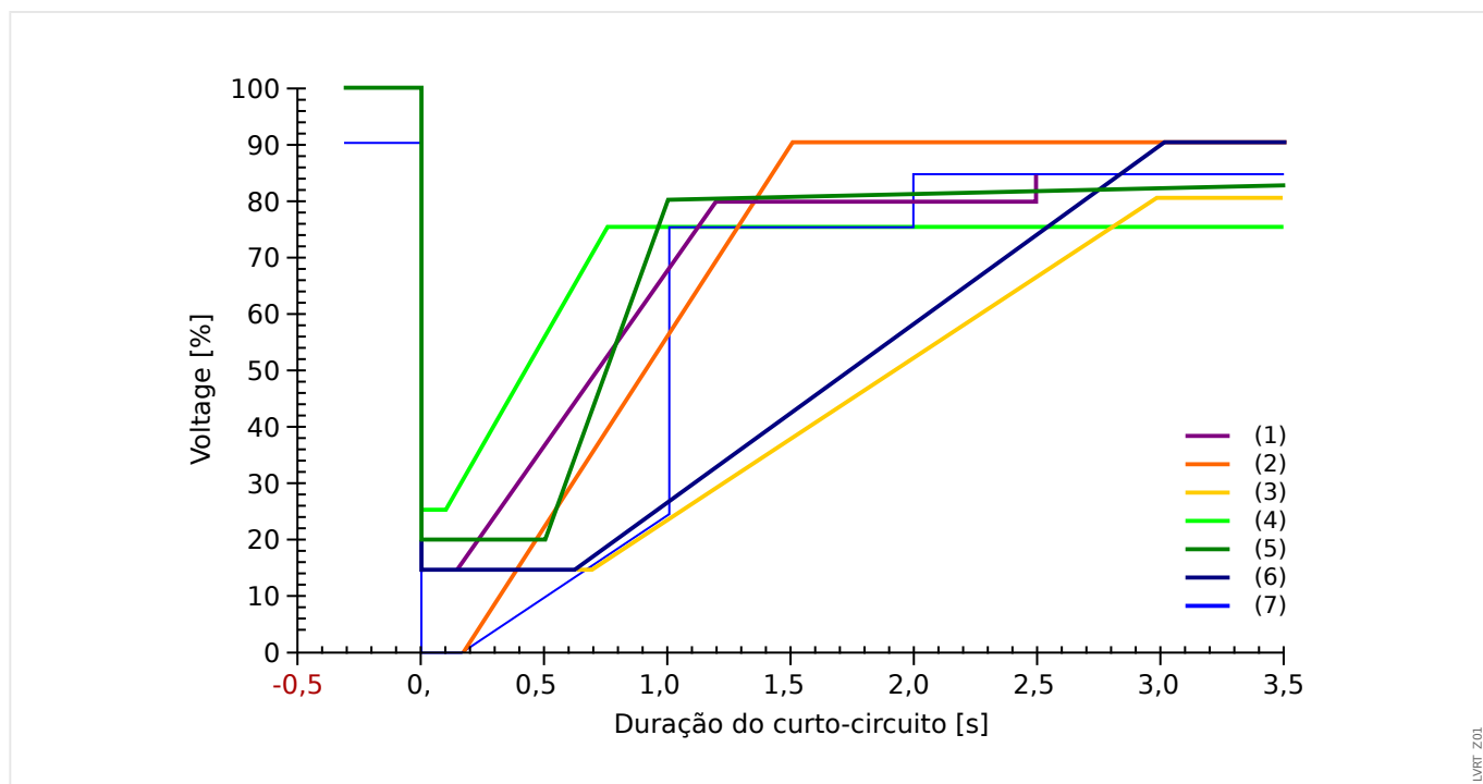
Fig. 113: Padrões LVRT; fonte: eBWK Bd. 60 (2008) Nr. 4. Autores: Dipl.-Ing. Thomas Smolka, Dr.-Ing. Karl-Heinz Weck, Zertifizierungstelle der FGH e.V., Mannheim, sowie Dipl.-Ing. (FH) Matthias Bartsch, Enercon GmbH, Aurich.
