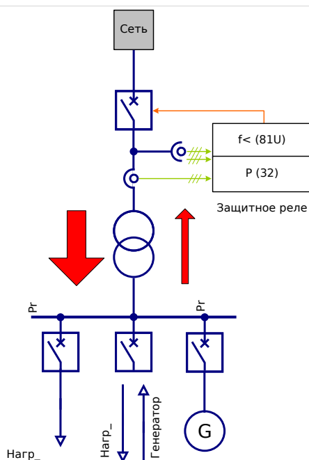
Рис. 107: Централизованная автоматическая частотная разгрузка в сетях с временным электроснабжением
