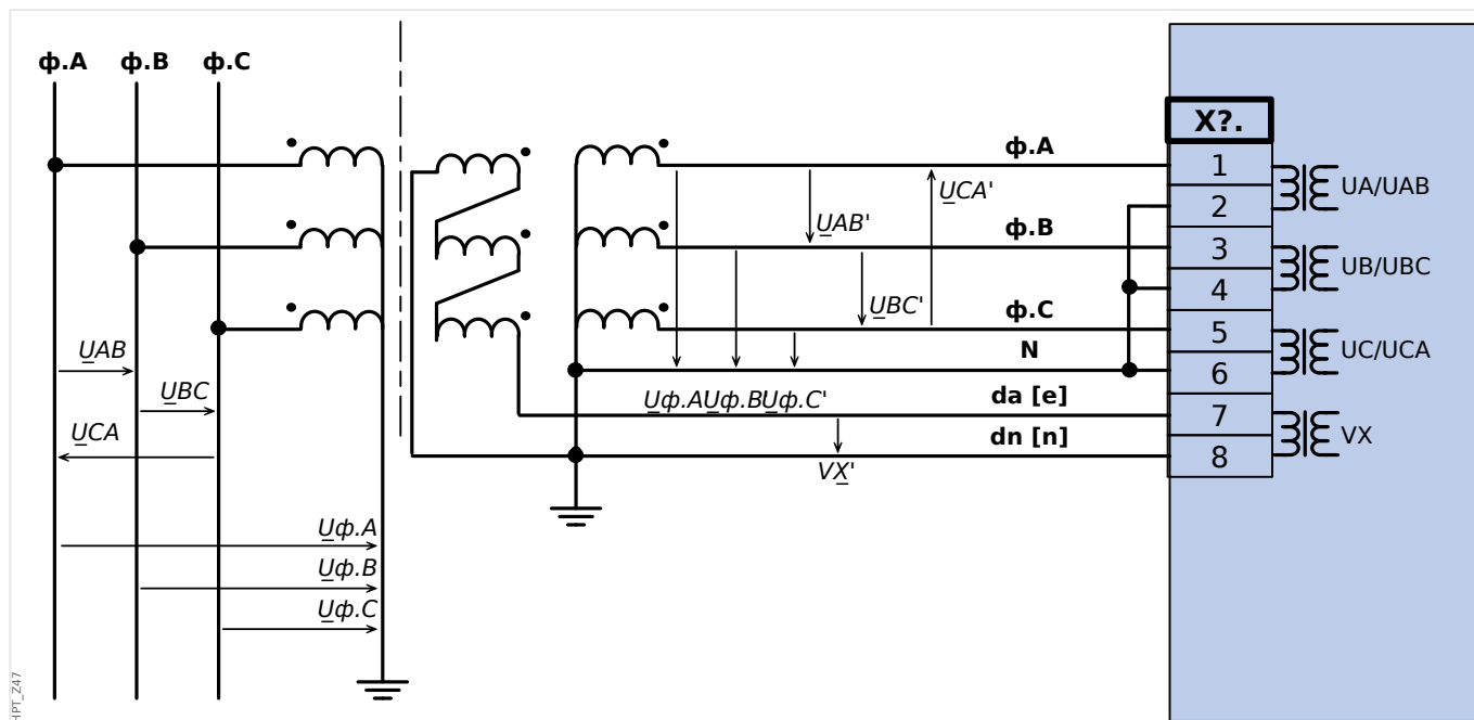
Рис. 35: VT Wye с соединением разомкнутого треугольника.
