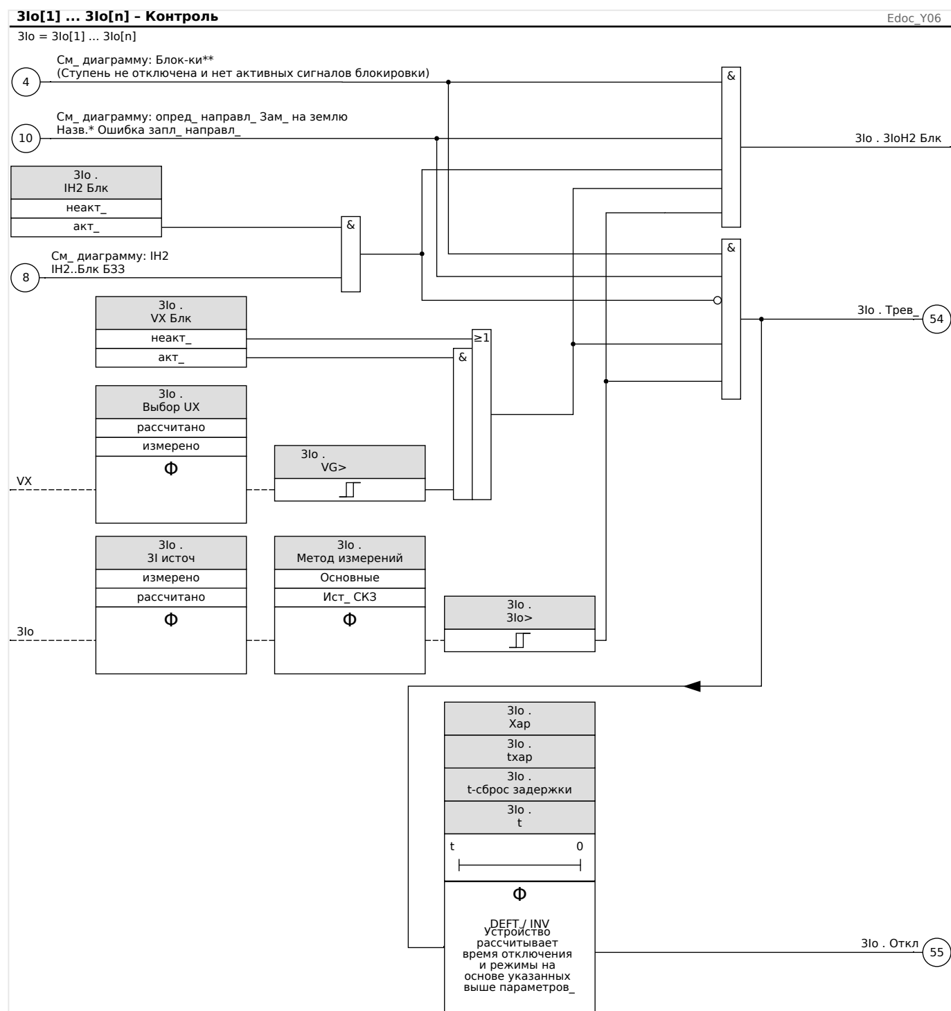
Рис. 81: Защита от максимального тока на землю, часть 1 (функция контроля, отключение).
