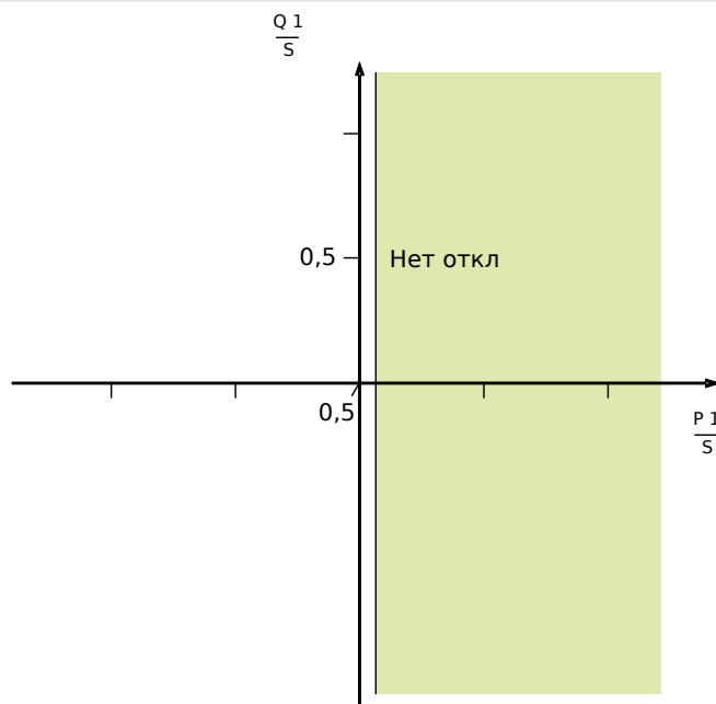
Рис. 112: Метод 2 (контроль чистой реактивной мощности): «Метод UFLS» = «Контр. чистой активной мощности».
