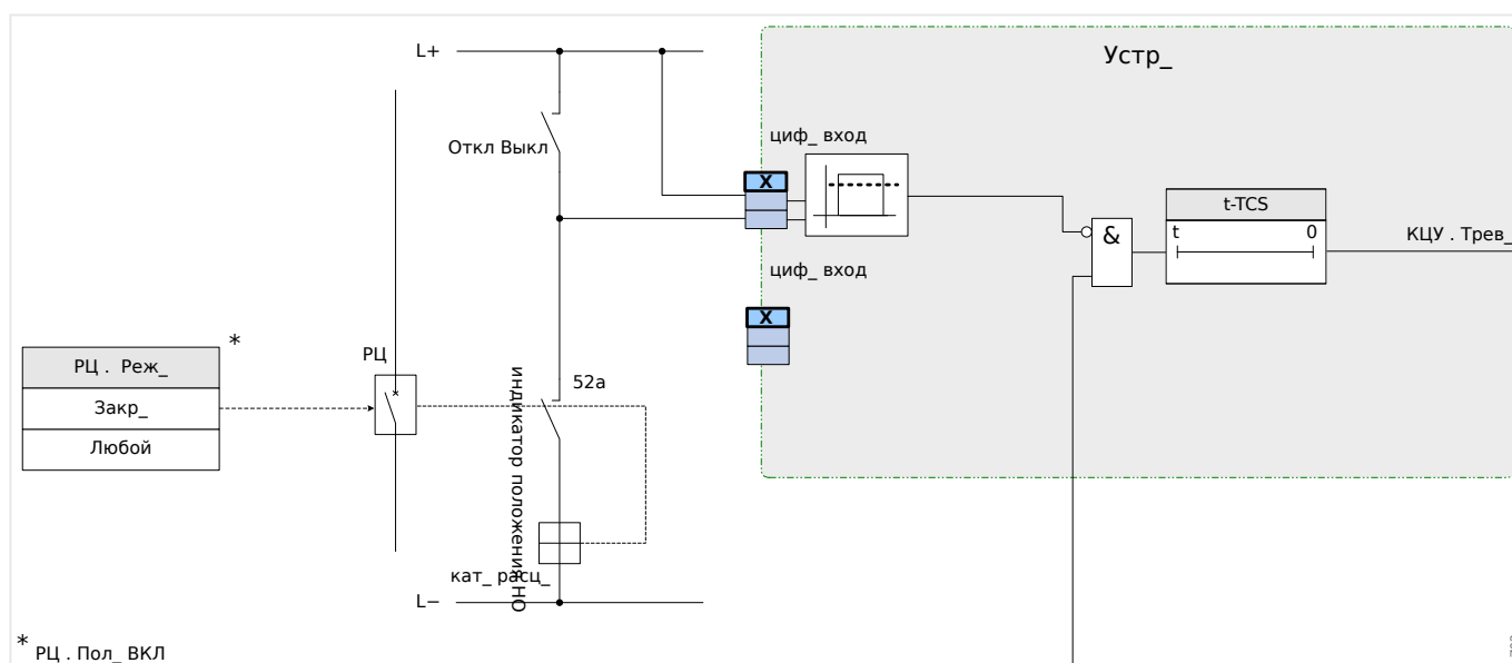
Рис. 121: Пример соединения: контроль цепи отключения только с одним вспомогательным контактом выключателя «Всп Вкл» (52a).
