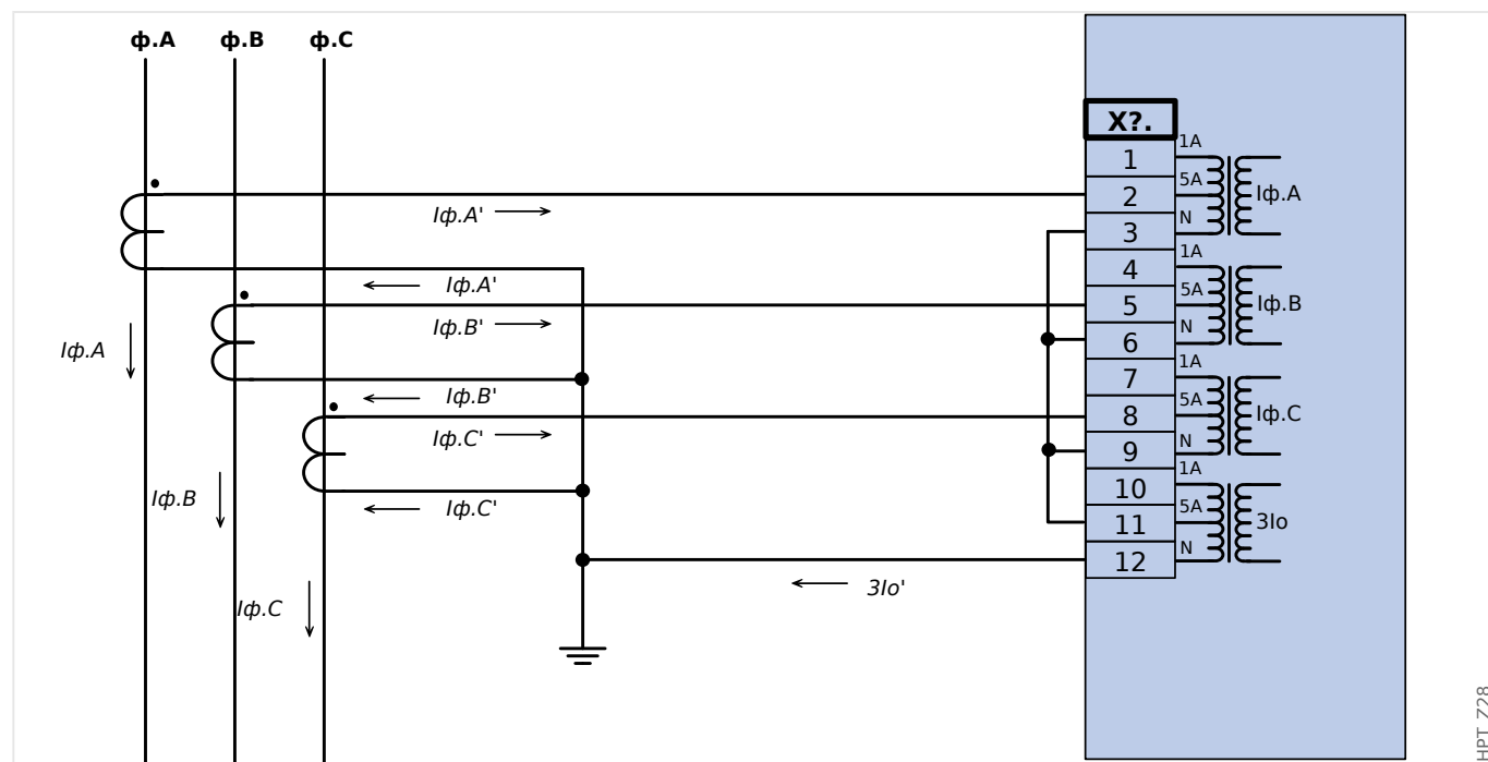
Рис. 22: Измерение фазных токов по схеме «полной» звезды; I_n вторичн. = 5 А. Ток на землю, измеряемый через соединение по схеме Холмгрена 3I_0 .ном.втор. = 5 А.
