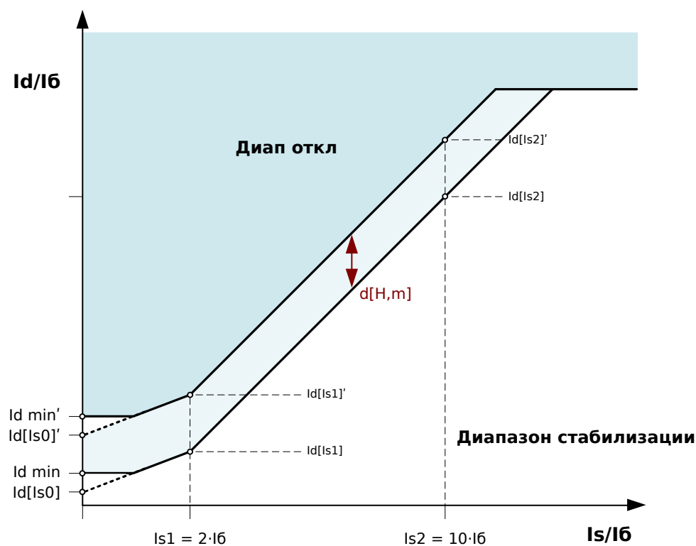
Рис. 76: Временное динамическое повышение статических характеристик отключения.
