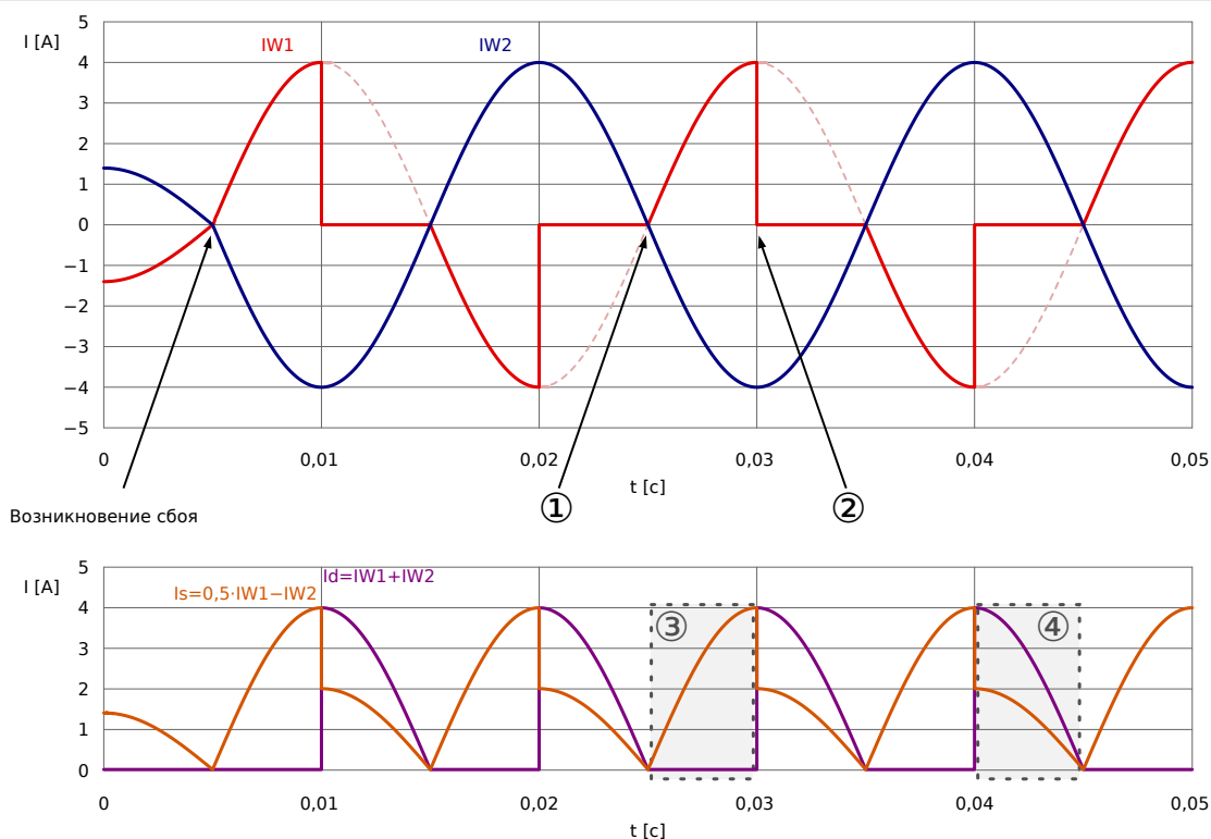
Рис. 77: Характеристики I_d и I_s при насыщении на стороне W1 ТТ при внешнем сбое.
