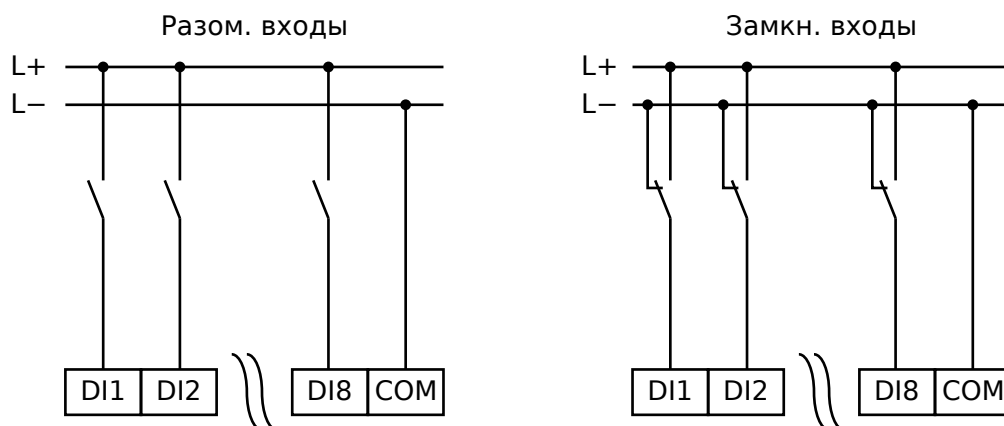
Рис. 144: Безопасное состояние цифровых входов
