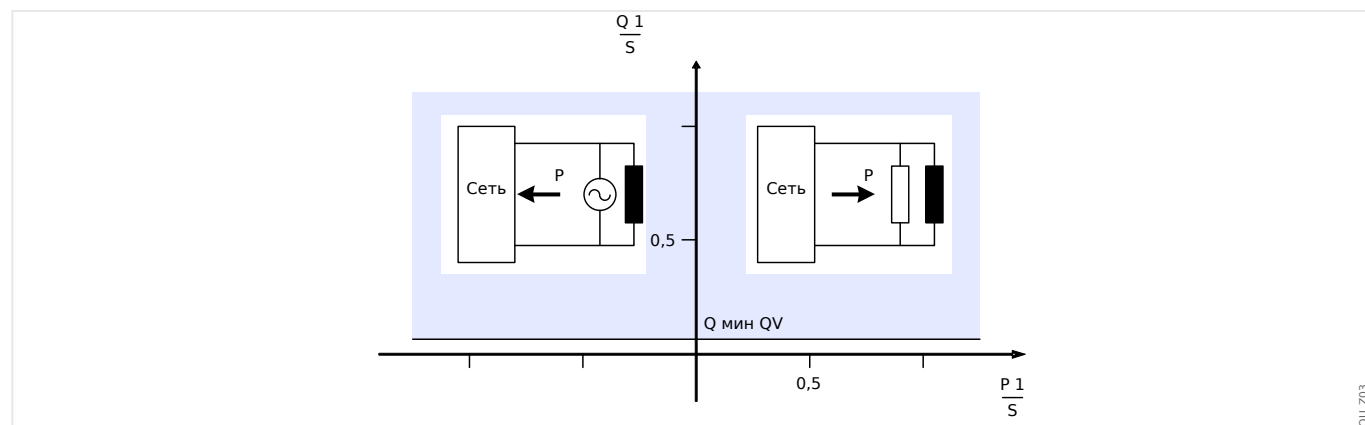
Рис. 104: Метод 2: контроль чистой реактивной мощности.
