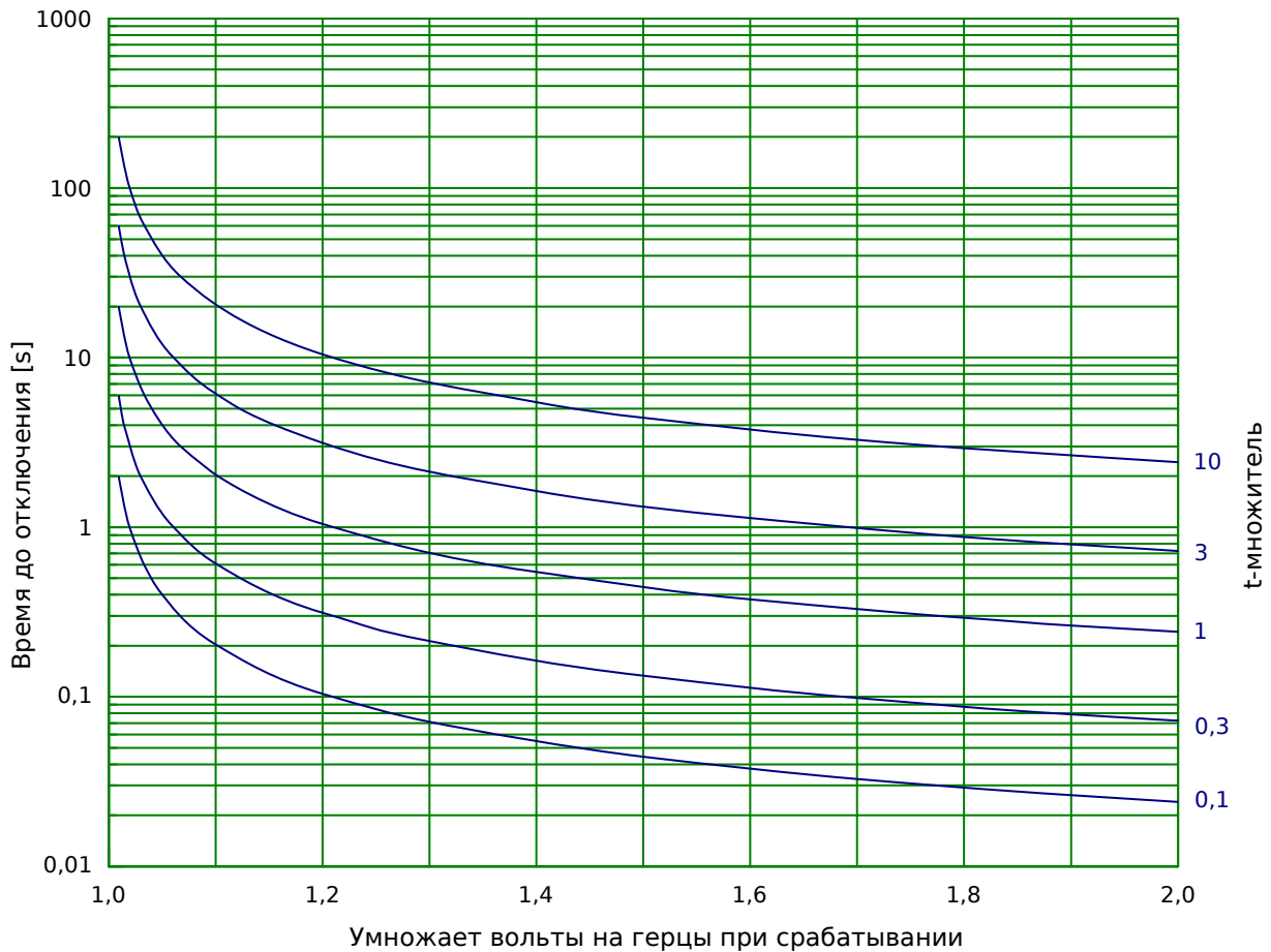
Рис. 86: Характеристика/форма кривой: INV C
