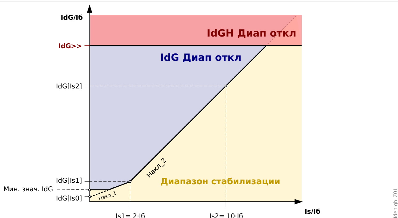
Рис. 80: Значение срабатывания « I_{dG}>> » по дифференциальному току утечки на землю, основанное на номинальной величине тока « I_6 » соответствующего объекта защиты.
