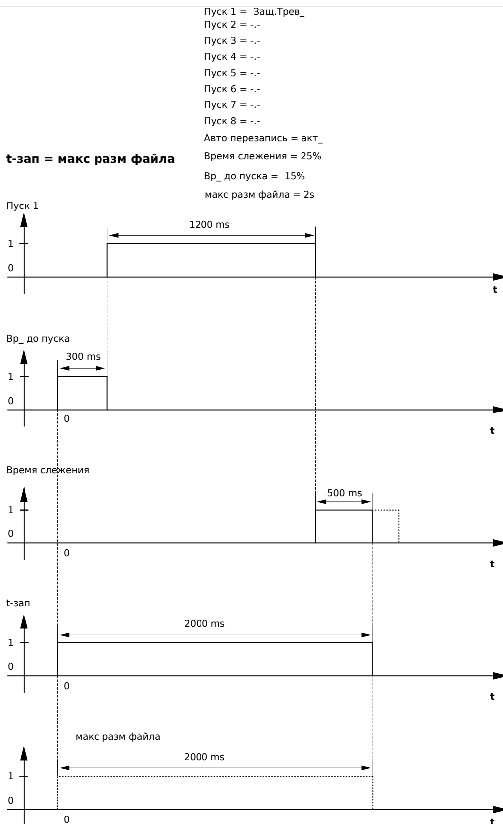
Рис. 132: Пример временной диаграммы регистратора аварийных нарушений I
