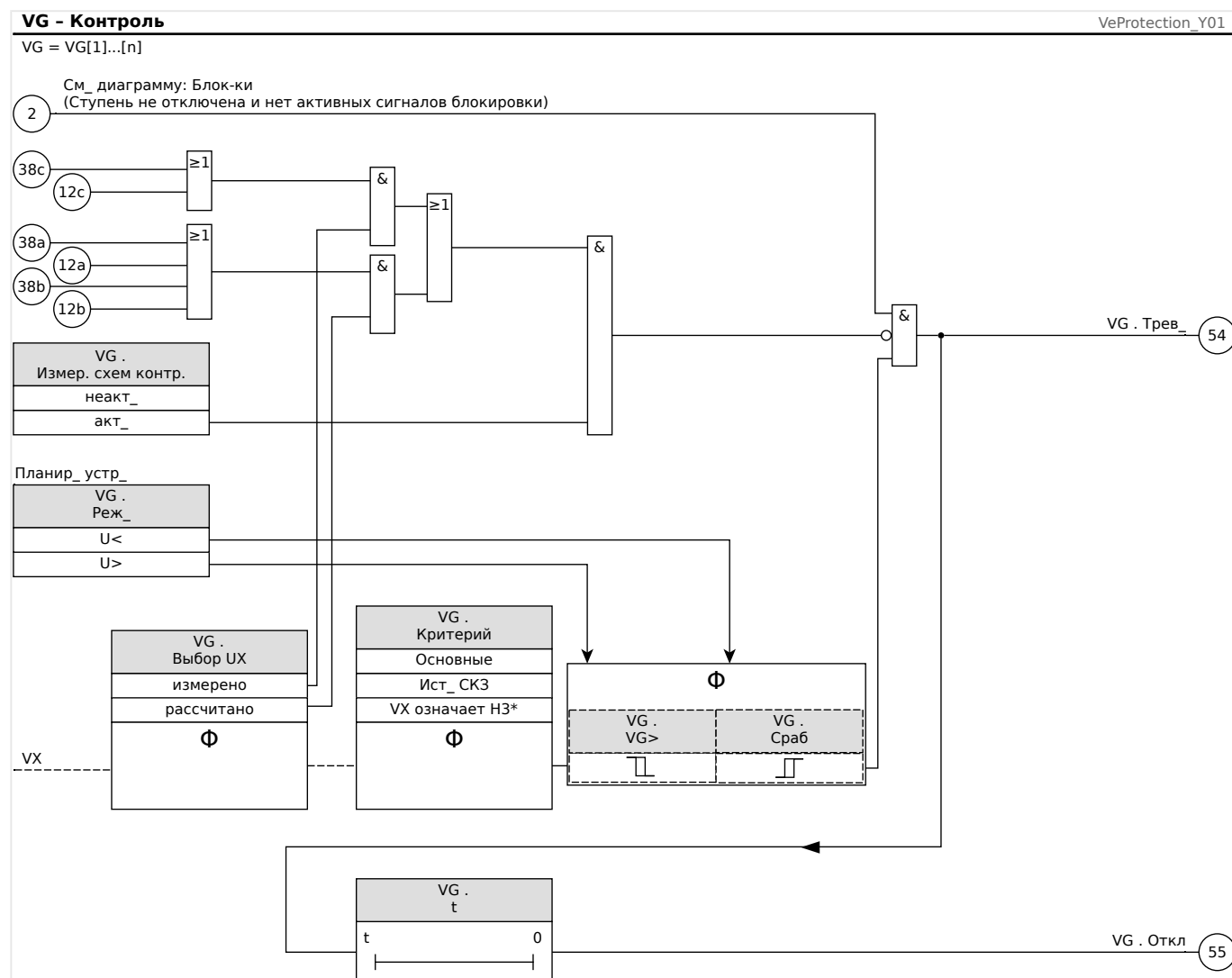
Рис. 90: Контроль напряжения VG, VX, часть 1 (функция контроля, отключение).
