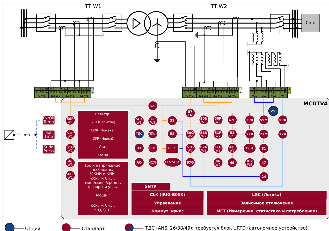
Рис. 1: Обзор функций MCDTV4.
