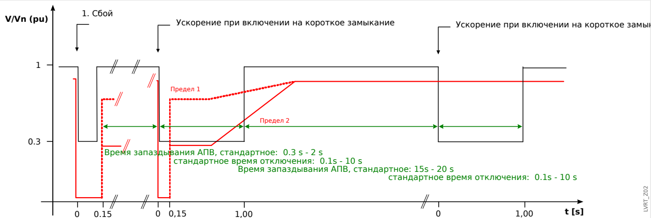
Рис. 114: Кривая напряжения во время двух неудачных попыток автоматического повторного включения; источник: Technische Richtlinie, Erzeugungsanlagen am Mittelspannungsnetz, Ausgabe Juni 2008, BDEW Bundesverband der Energie- und Wasserwirtschaft e.V. (стр. 89.).
