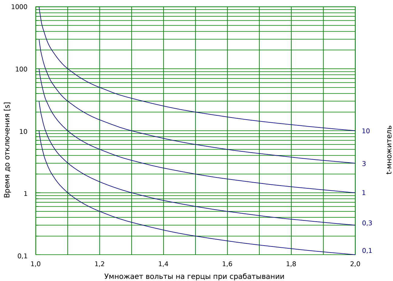
Рис. 85: Характеристика/форма кривой: INV B
