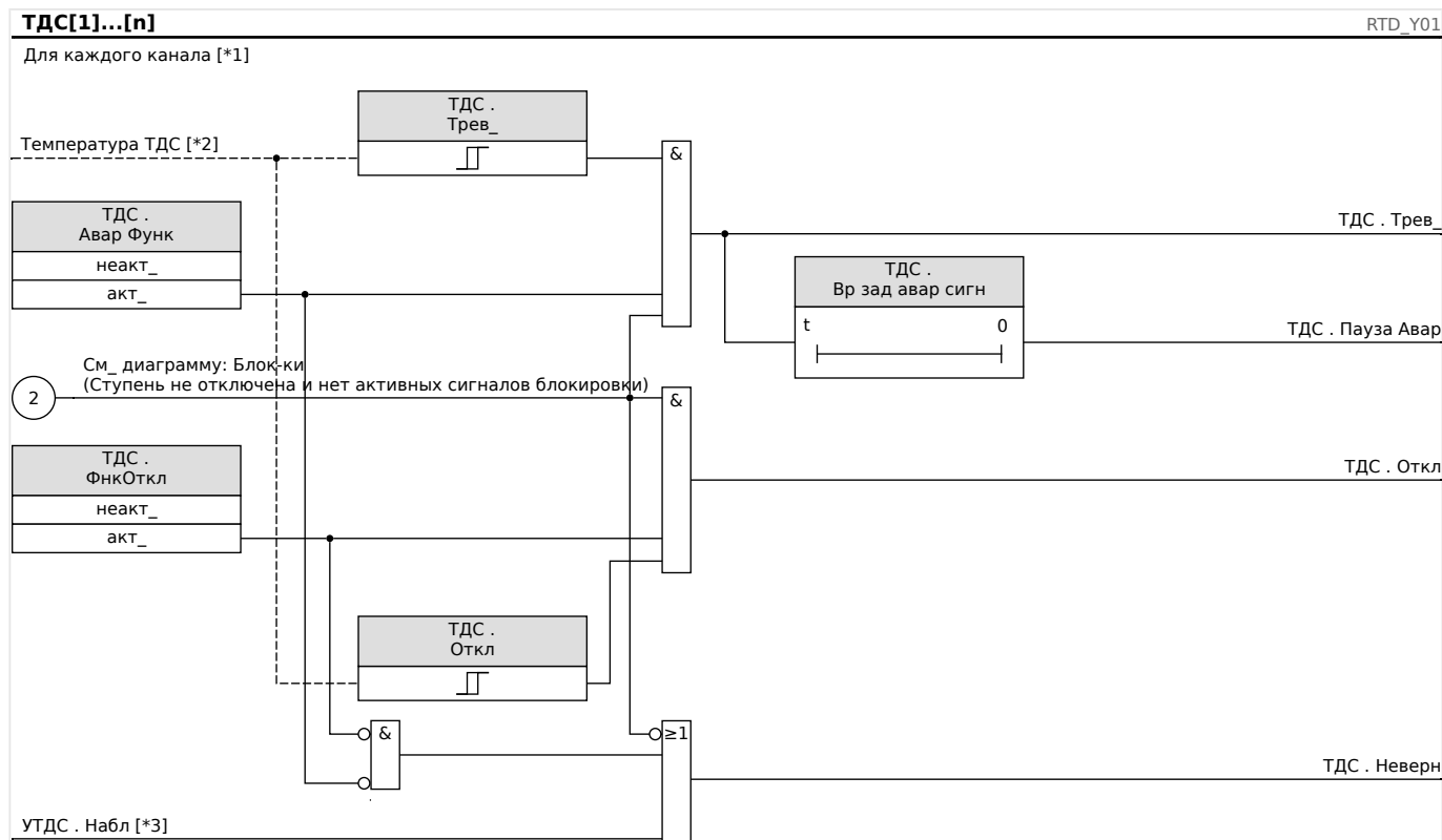
Рис. 119: Общий принцип работы (аварийный сигнал с задержкой, отключение без задержки).
