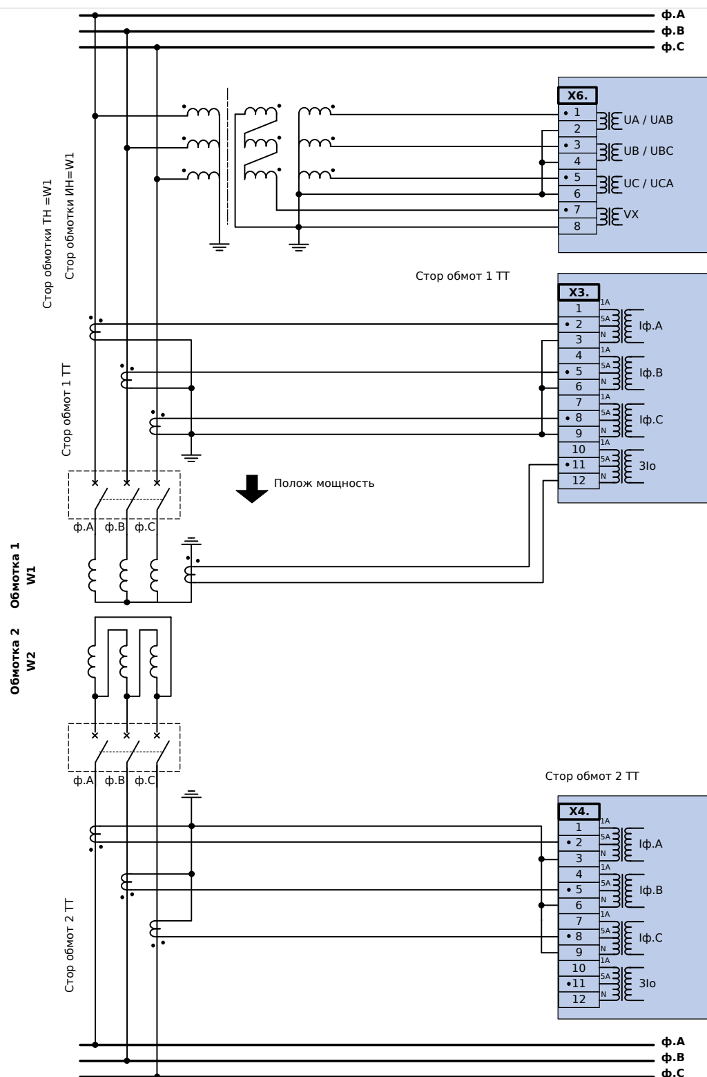
Рис. 39: Трансформатор DY с фазовой дифференциальной защитой и дифференциальной защитой от замыкания на землю только на W1.
