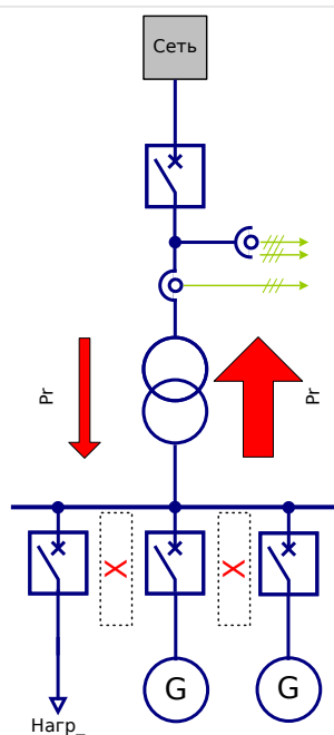
Рис. 110: Децентрализованное использование в сетях с преобладанием энергоснабжения.
