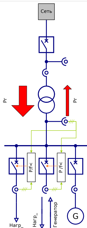
Рис. 108: Децентрализованная автоматическая частотная разгрузка в сетях с временным электроснабжением.
