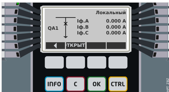
Рис. 124: Пример страницы управления, выключатель в замкнутом положении.
