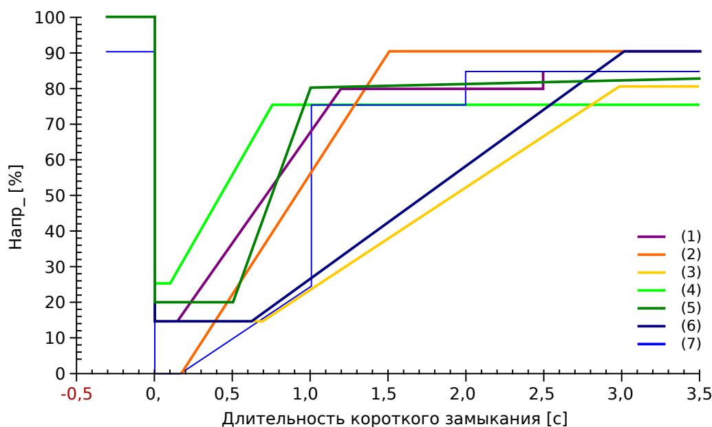
Рис. 113: Стандарты РПН; источник: eBWK Bd. 60 (2008 г.), № 4. Авторы: дипломированный инженер Томас Смолка, д. т. н. Карл-Хайнц Век, центр сертификации FGH e.V., Мангейм, а также дипломированный инженер (FH) Матиас Барч, Enercon GmbH, Аурих.
