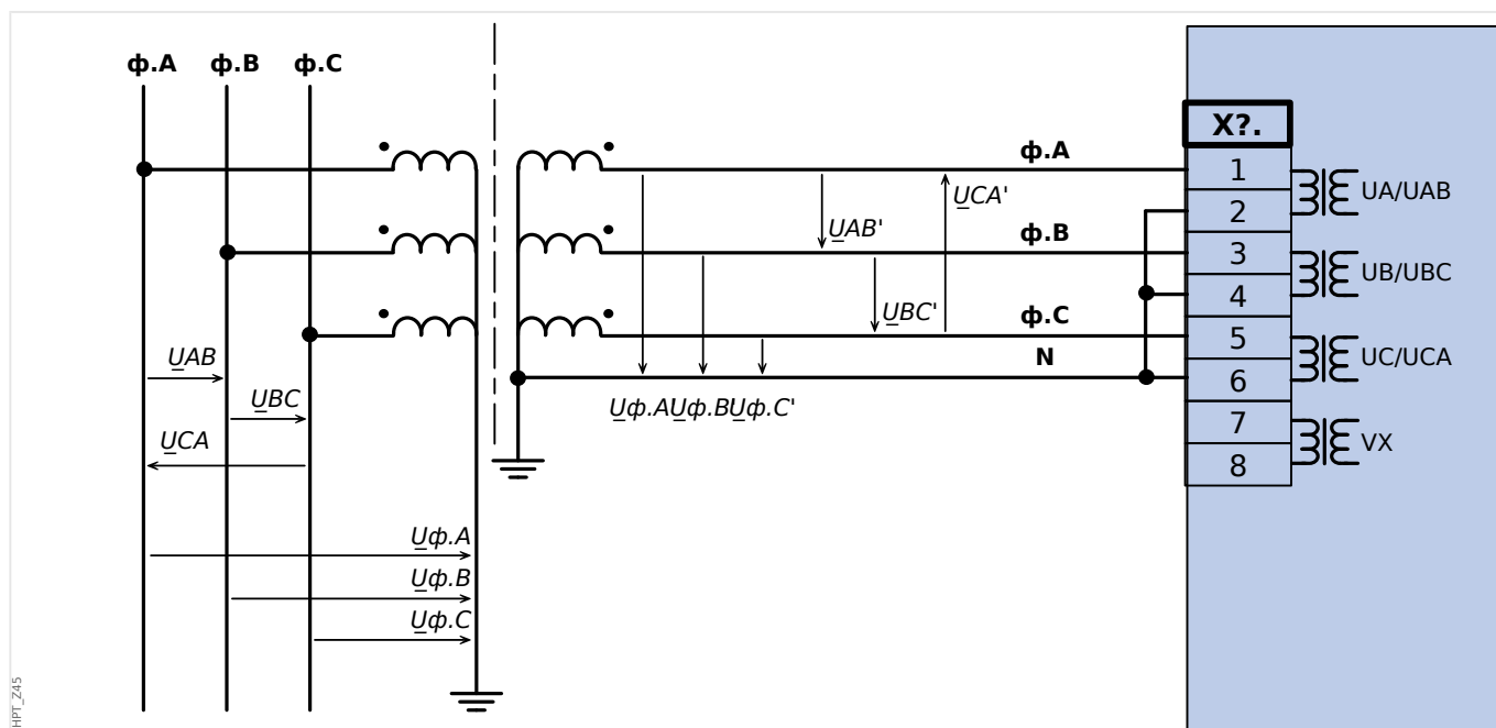
Рис. 34: VT Wye: Измерение трехфазного напряжения по схеме «звезда»
