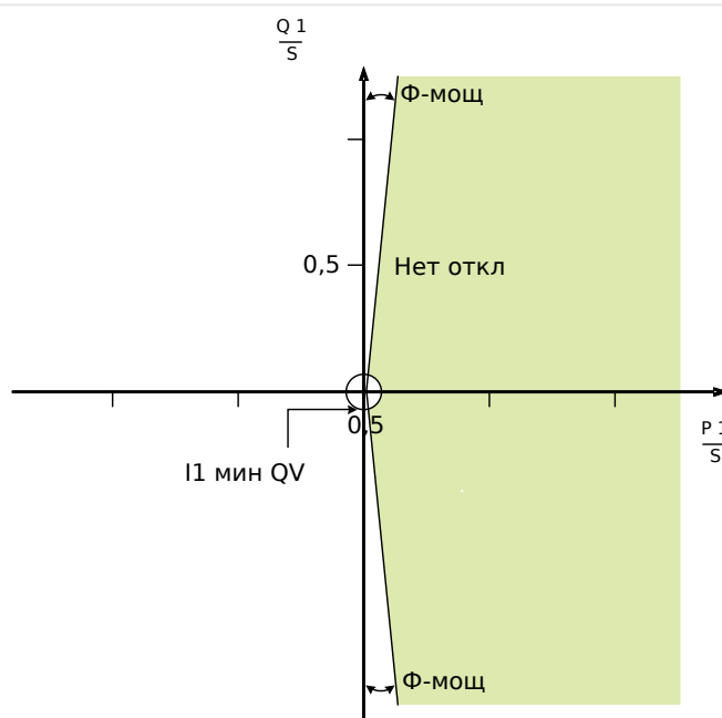
Рис. 111: Метод 1 (контроль угла мощности): «Метод UFLS» = «Контроль угла мощности».
