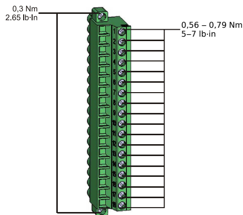
Abb. 138: Spannungsmessstecker der Spannungsmesskarten „TU-OR5“ und „TU-DI8“.
