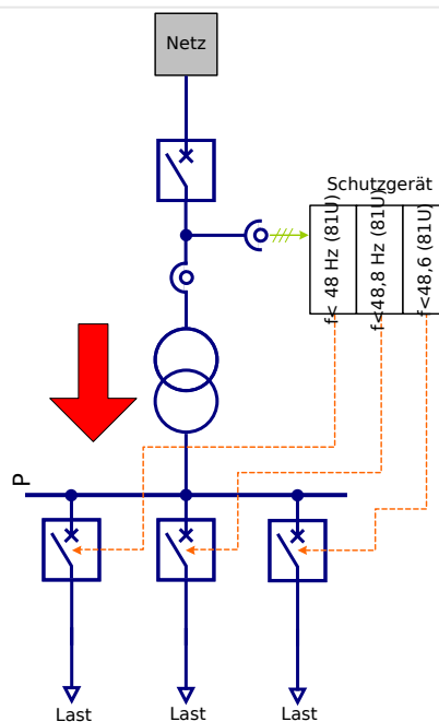
Abb. 93: Klassischer gestufter dezentraler Lastabwurf.
