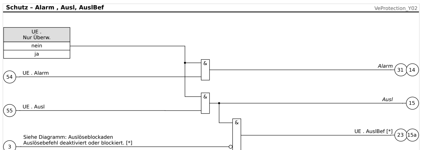
Abb. 81: UE/UX-Spannungsüberwachung, Teil 2 (Aus-Befehl und Anstoßen von Generalanregung und General-Auslösung).
