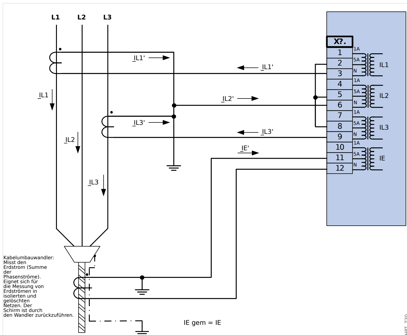
Abb. 23: Zweiphasiger Stromwandleranschluss in V-Schaltung; In sekundär = 5 A. Erdstromerfassung über Kabelumbauwandler; IEn sekundär = 5 A.
