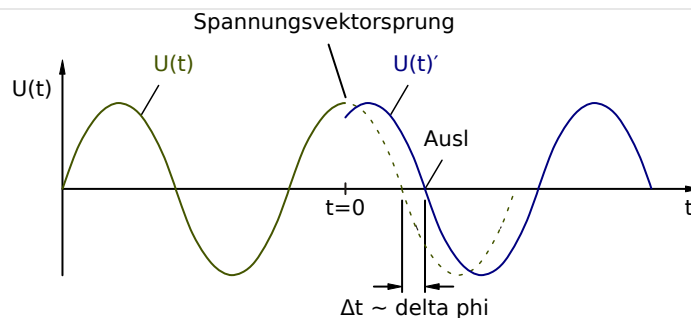
Abb. 87: Spannungsvektorsprung.
