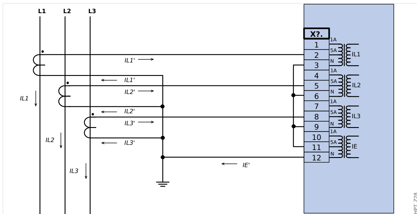
Abb. 21: Dreiphasiger Stromwandleranschluss; In sekundär = 5 A. Erdstromerfassung über Holmgreenschaltung IEn sekundär = 5 A.
