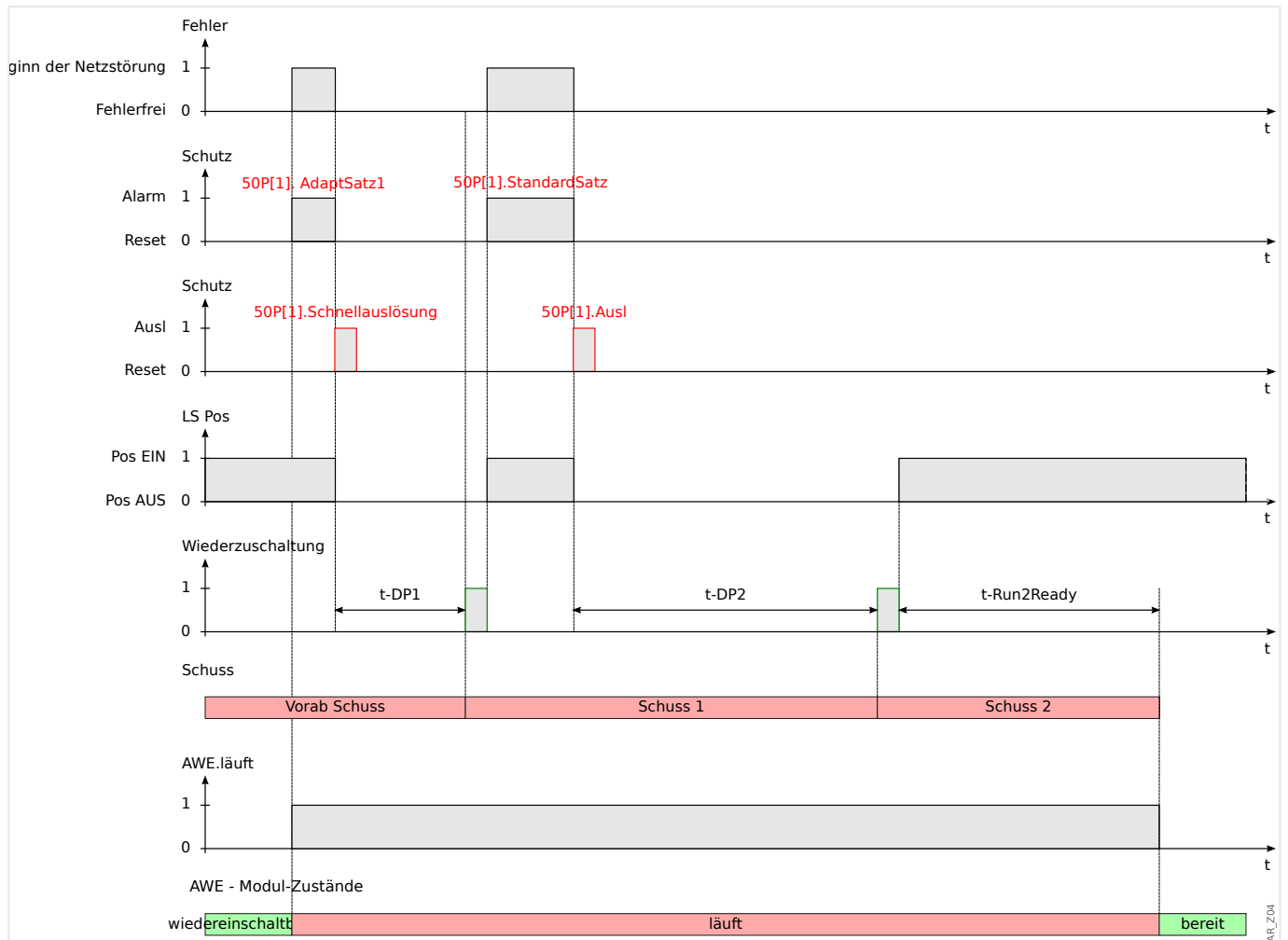
Abb. 103: Zweischißige, erfolgreiche Wiedereinschaltung mit Schnellauslösung (Prä-Schuss).
