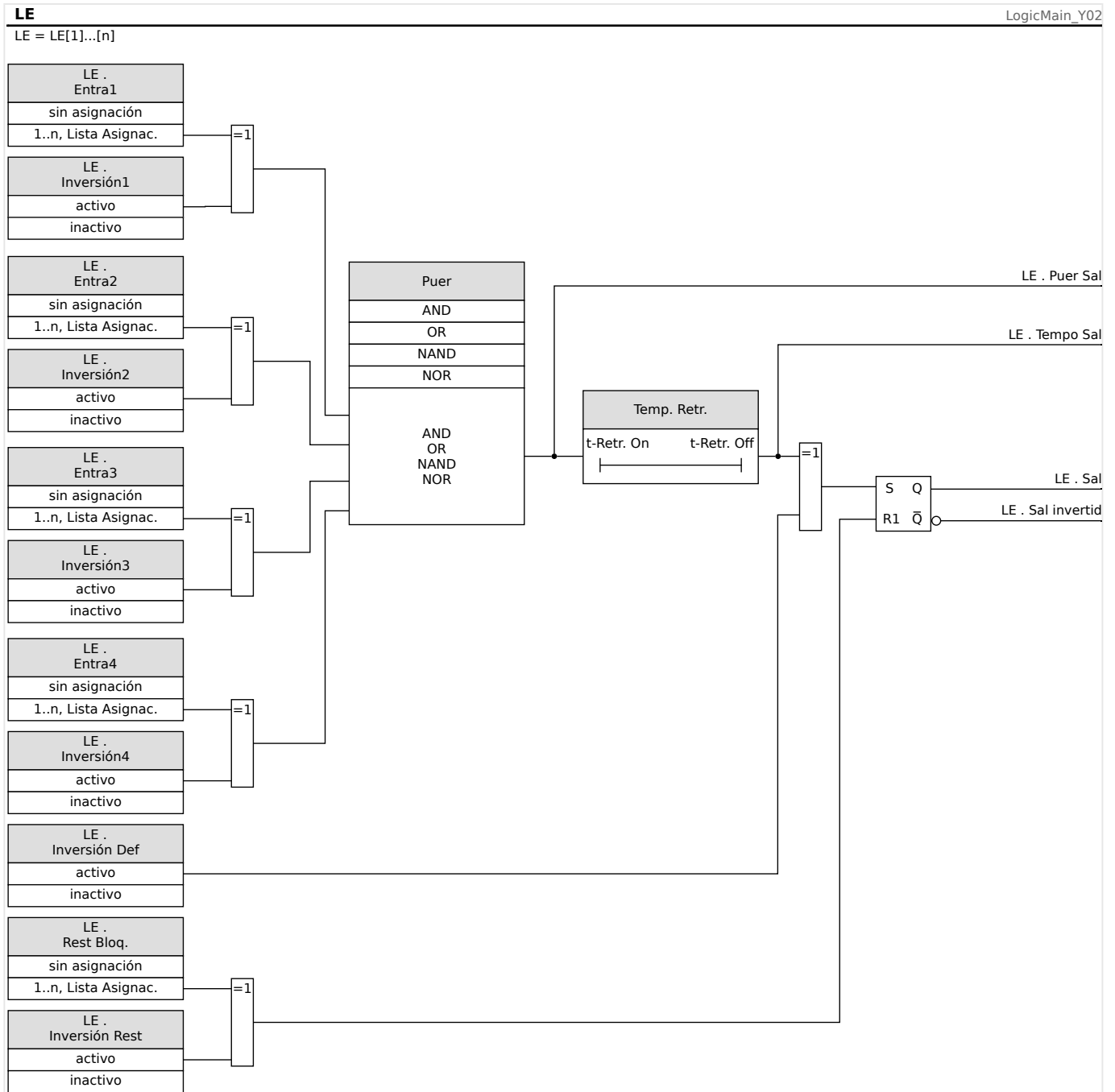
Fig. 131: Descripción detallada - Diagrama de lógica general.
