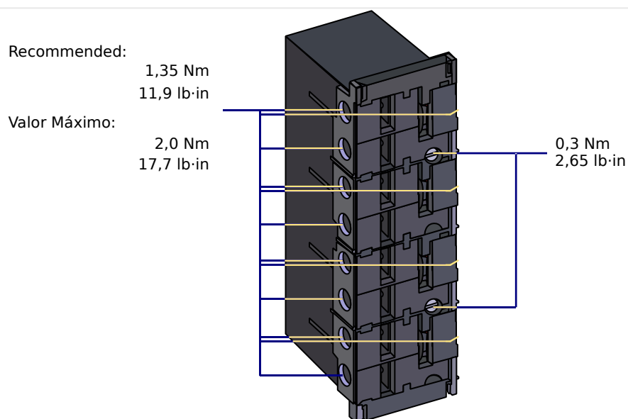
Fig. 137: Conector enchufable con cortocircuitador integrado (entradas de corriente convencionales)
