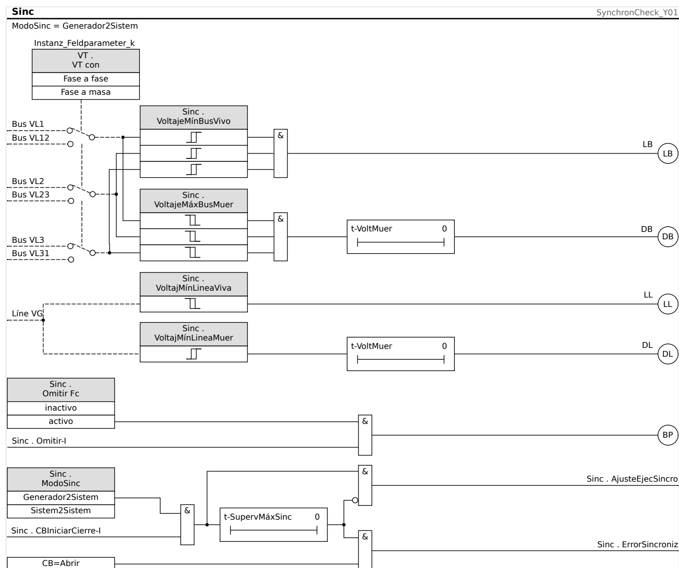
Fig. 111: Funcionalidad del módulo »Sinc«, «Generador2Sistem».
