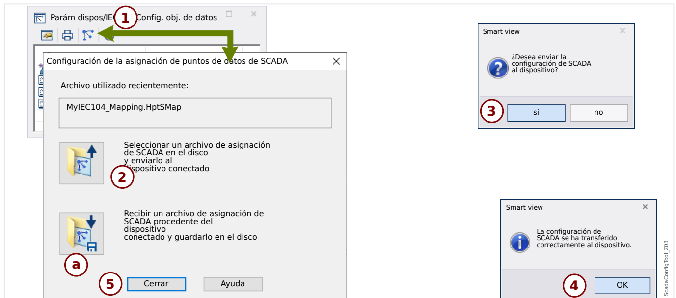
Fig. 59: Ejemplo de uso de Smart view para transferir el archivo *.HptSMap al dispositivo de protección.
