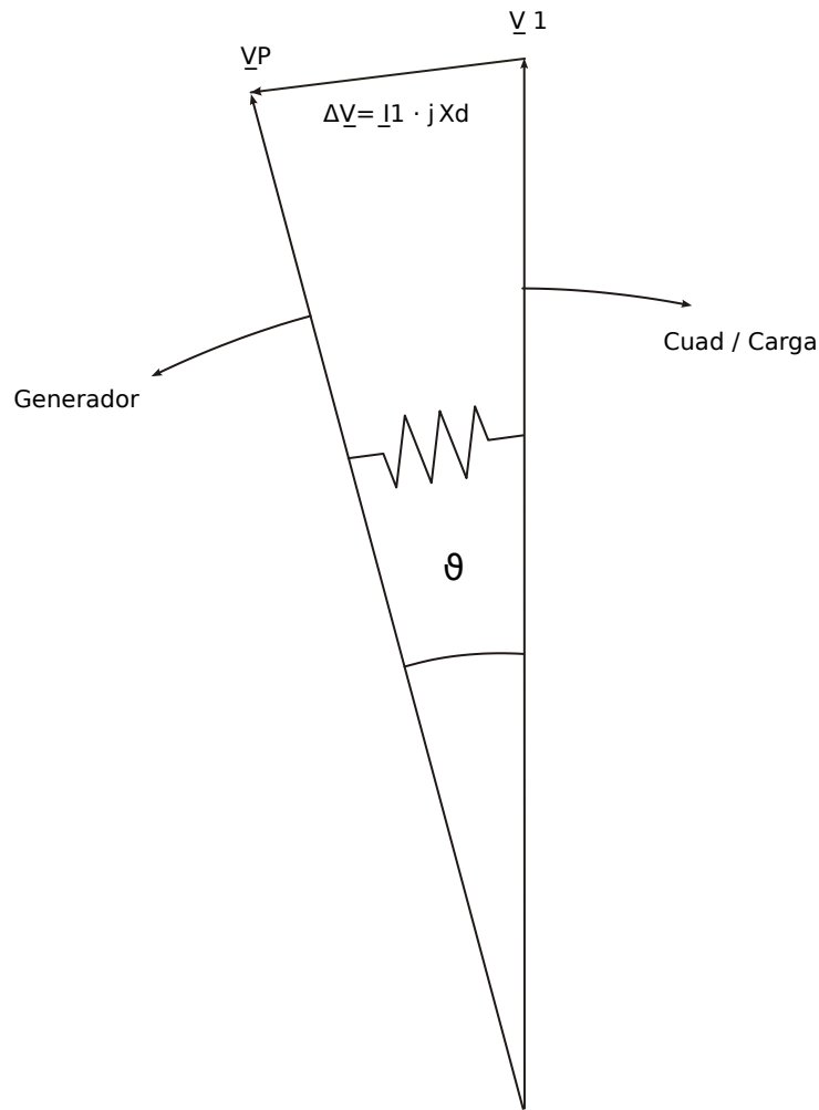
Fig. 85: Vectores de tensión en funcionamiento en paralelo con la red de suministro eléctrico.
