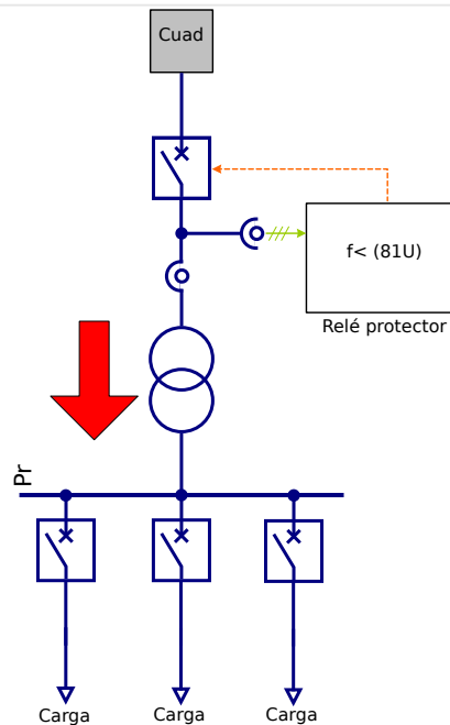
Fig. 93: Reducción de carga centralizada convencional.
