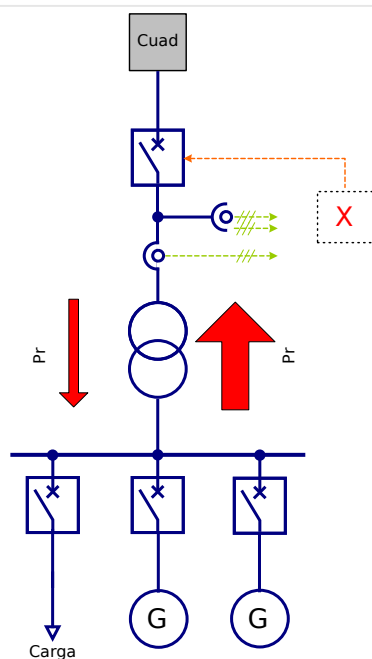
Fig. 97: Uso centralizado en redes con alimentación predominante.
