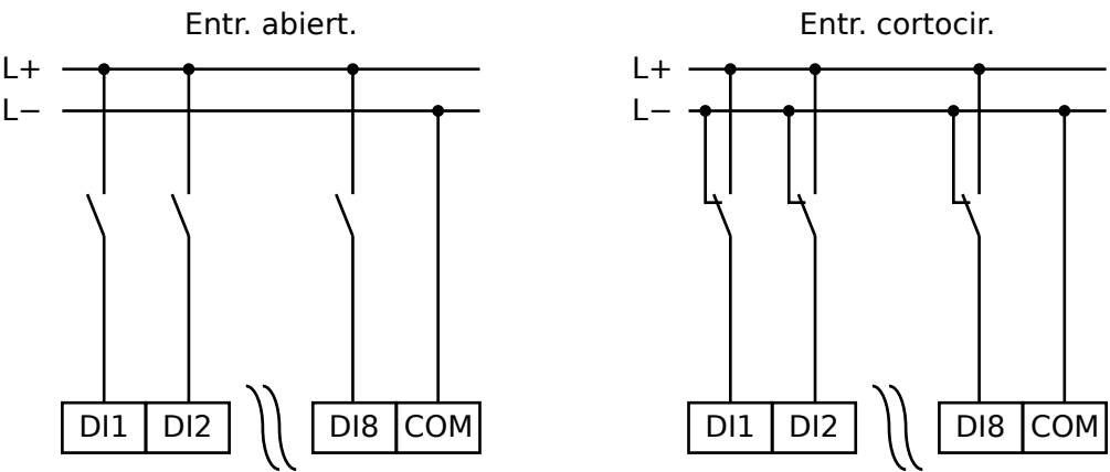
Fig. 140: Estado seguro de entradas digitales
