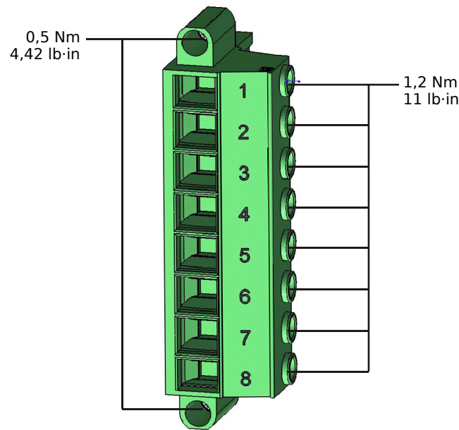
Fig. 138: Terminales de medición de tensión de la tarjeta de medición "TU" (→ «2.6.1 TU - Entradas de medición de tensión»).
