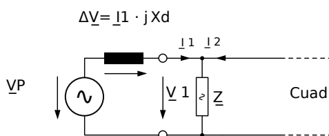
Fig. 84: Circuito equivalente en generador sincrónico en paralelo con la red de suministro eléctrico.
