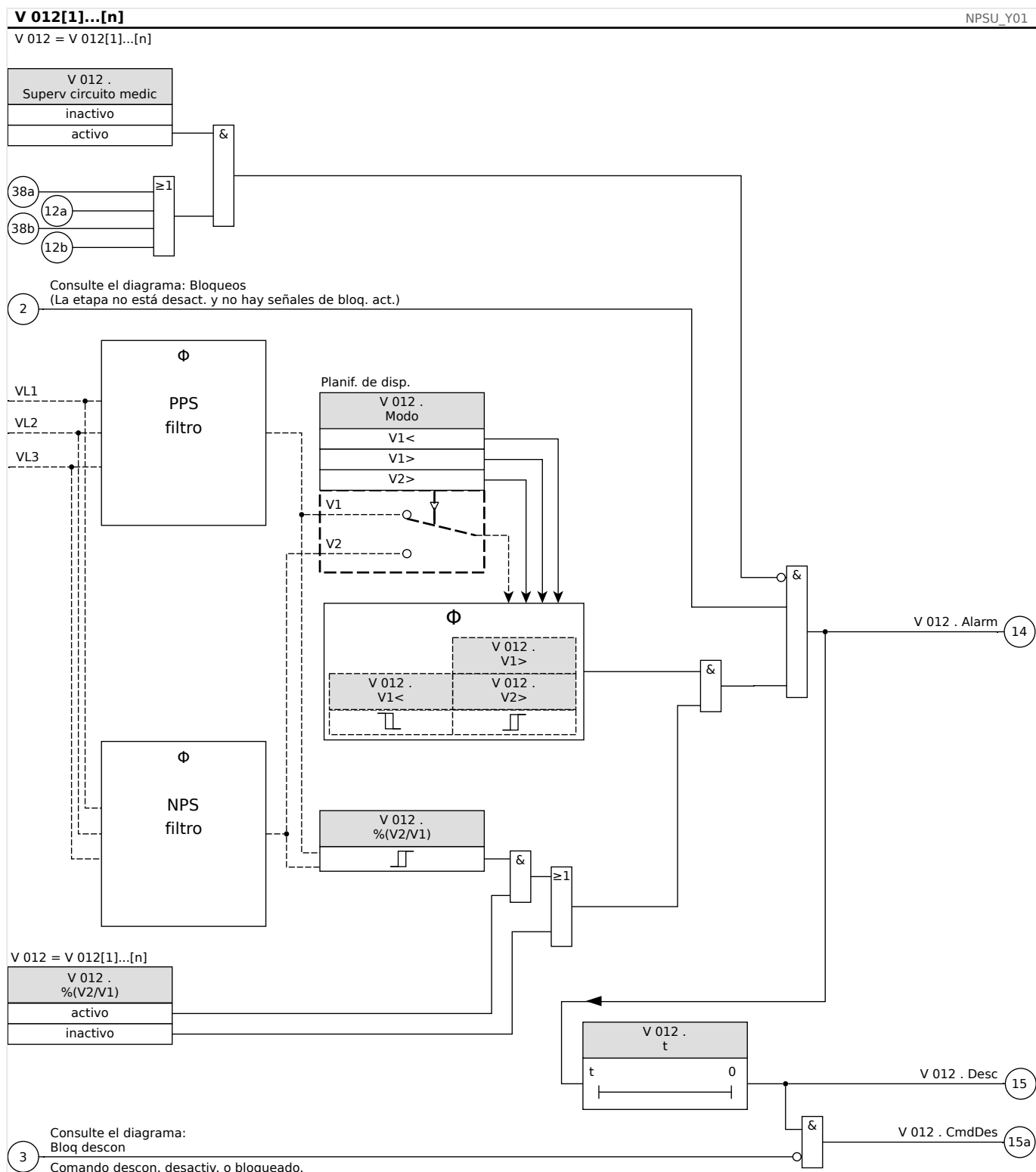
Fig. 83: Funcionalidad del módulo »V 012«.
