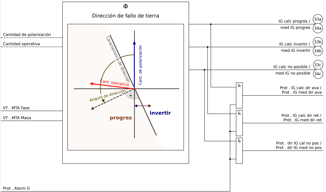
Fig. 65: Detección de dirección en todos los métodos, excepto " \cos(\phi) ", " \sin(\phi) ".
