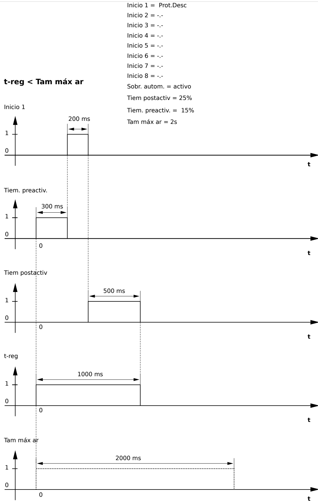
Fig. 128: Ejemplo 2: cuadro de intervalos del registrador de perturbaciones
