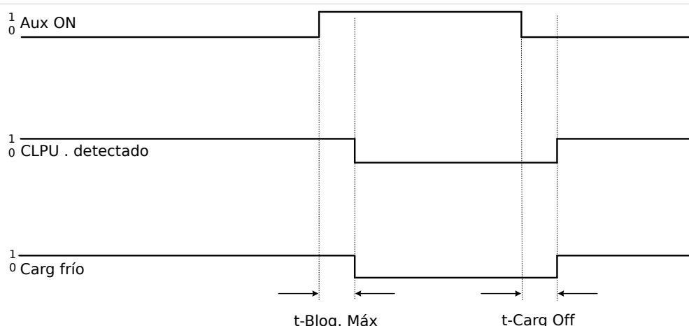
Fig. 113: Modo de ejemplo: Posición de interruptor.
