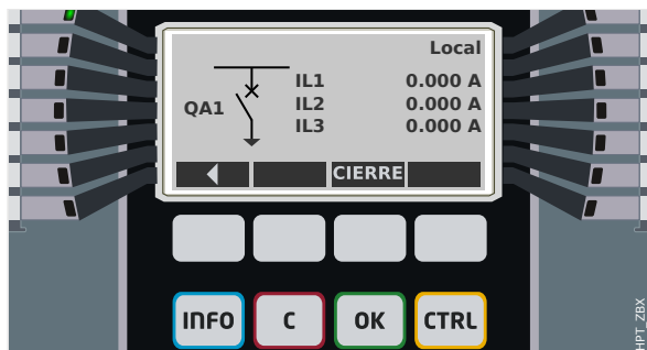
Fig. 121: Ejemplo de página de control, con el circuito en posición abierta.
