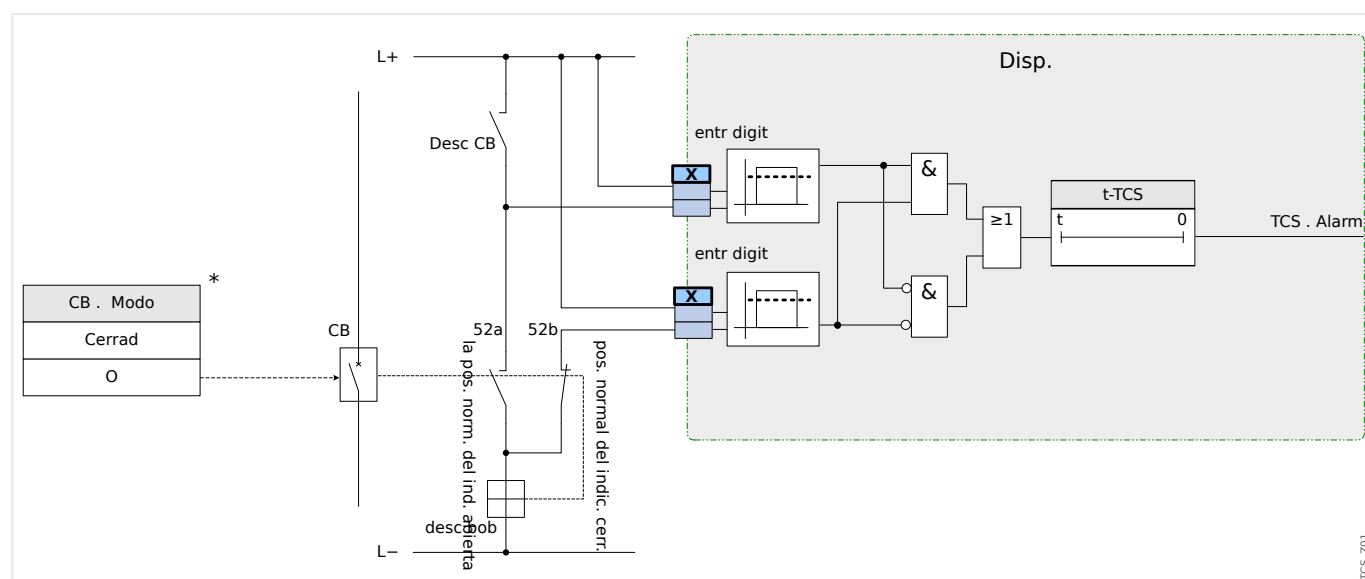
Fig. 115: Ejemplo de conexión: Supervisión del circuito de desconexión con dos contactos auxiliares CB »Aux ON« (52a) and »Aux OFF« (52b).
