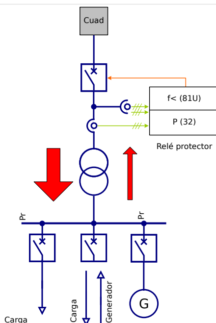
Fig. 95: Reducción de carga centralizada por subfrecuencia en redes eléctricas con alimentación temporal
