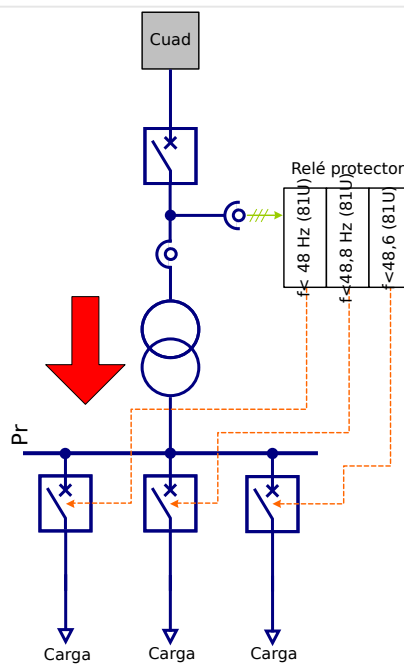
Fig. 94: Reducción de carga descentralizada convencional.
