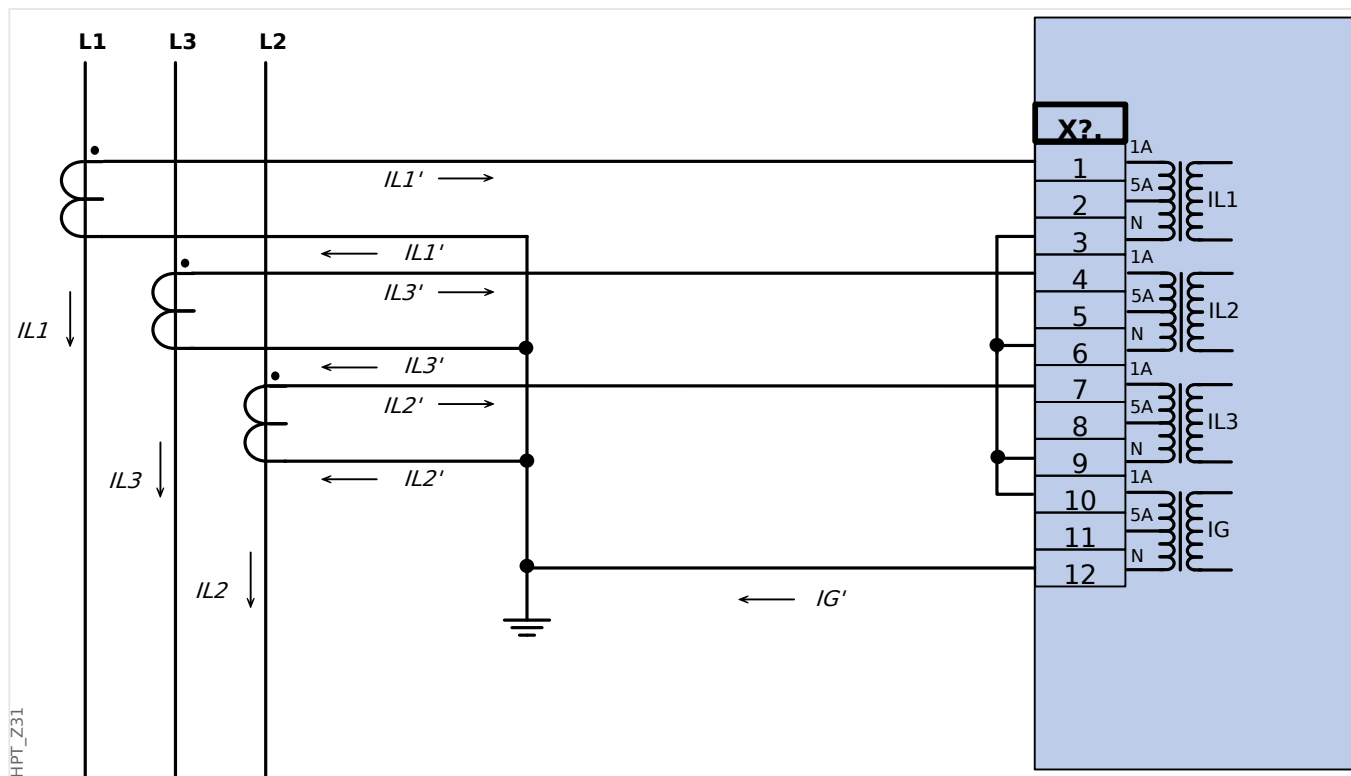
Fig. 24: Medida corriente trifásica; En secundario = 1 A. Medic corr de tierra mediante conexión Holmgreen; IG_{nom\ secund} = 1\text{ A} .
