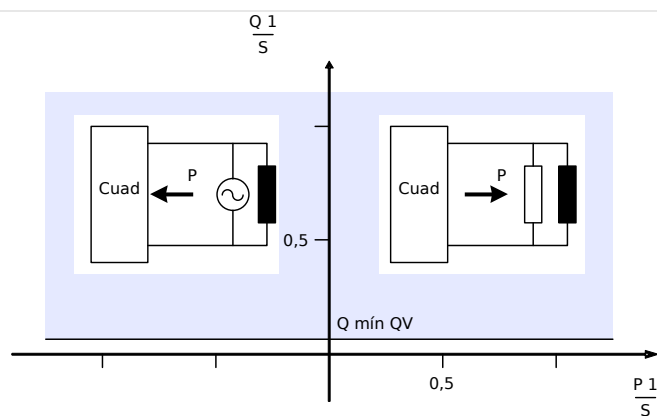
Fig. 92: Método 2: Supervisión de potencia reactiva pura.
