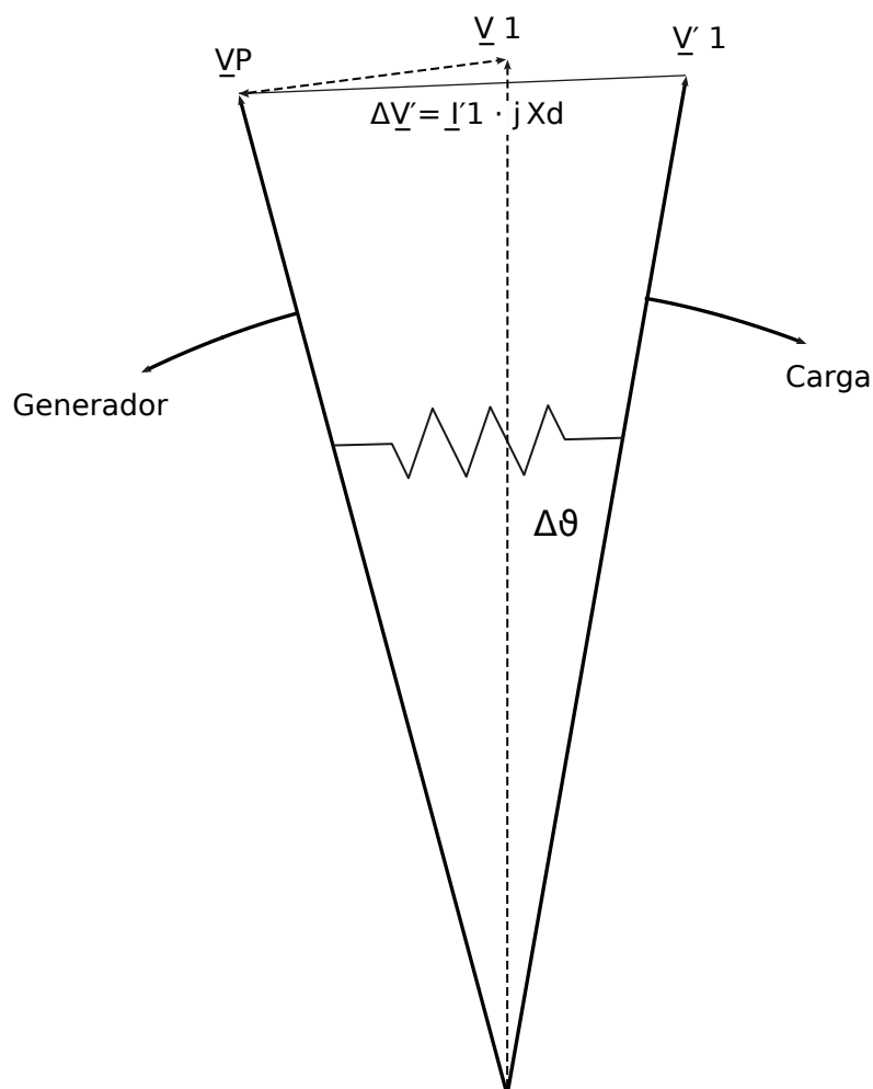
Fig. 87: Fallo de los vectores de tensión en la red.
