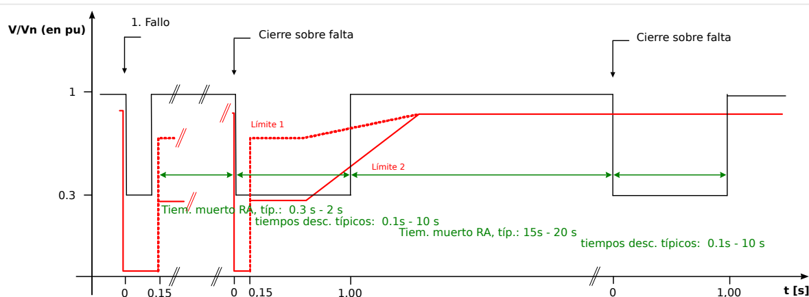
Fig. 78: Recorrido de la curva de tensión durante dos intentos fallidos de reconexión automática; fuente: Technische Richtlinie, Erzeugungsanlagen am Mittelspannungsnetz, Ausgabe Juni 2008, BDEW Bundesverband der Energie- und Wasserwirtschaft e.V. (Página 89).
