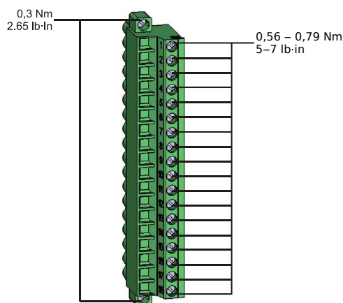
Fig. 139: Terminales de medición de tensión de tarjetas de medición "TU-OR5" y "TU-DI8" , ).
