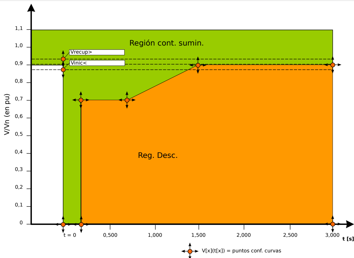
Fig. 79: Regiones de continuidad y desconexión.
