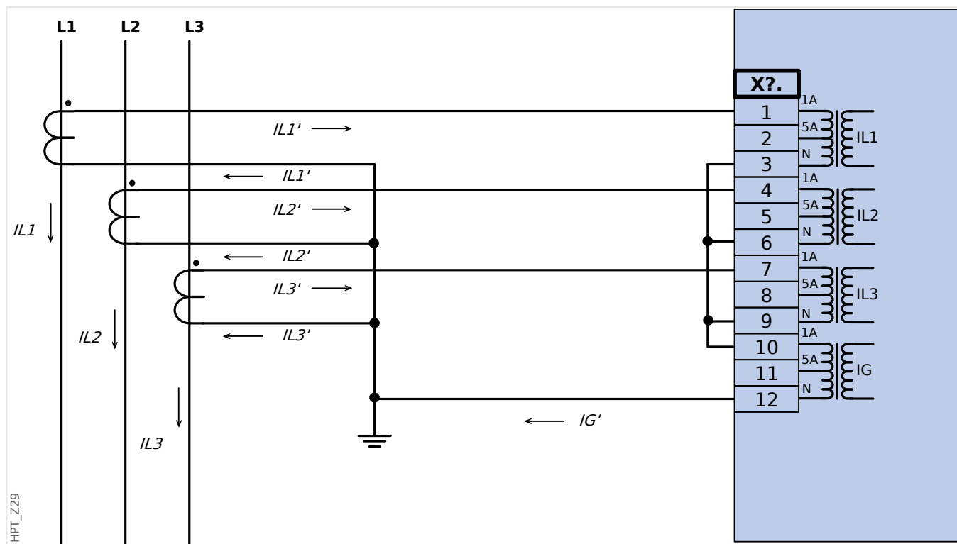
Fig. 22: Medida corriente trifásica; En secundario = 1 A. Medic corr de tierra mediante conexión Holmgreen; IG_{nom} \text{ secund} = 1 \text{ A} .
