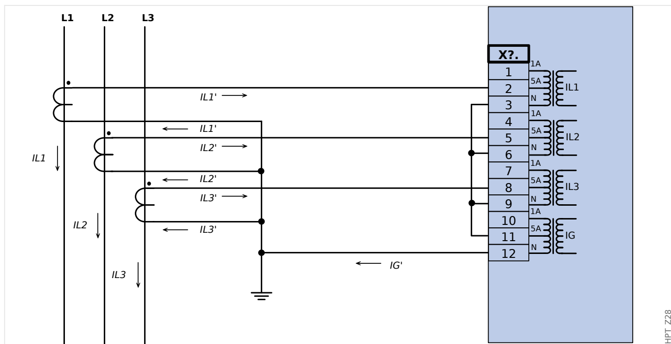
Fig. 21: Medida corriente trifásica; En secundario = 5 A. Medic corr de tierra mediante conexión Holmgreen; IG_{nom} \text{ secund} = 5 \text{ A} .
