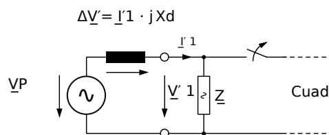
Fig. 86: Circuito equivalente en fallo de red eléctrica.
