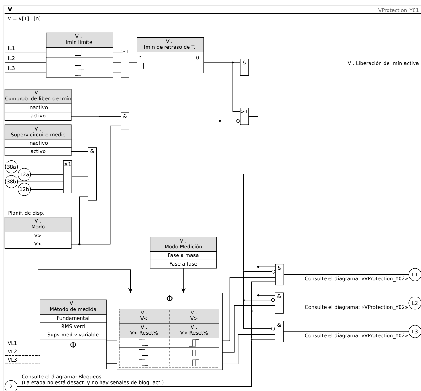
Fig. 74: Funcionalidad del módulo de protección de tensión, parte 1.
