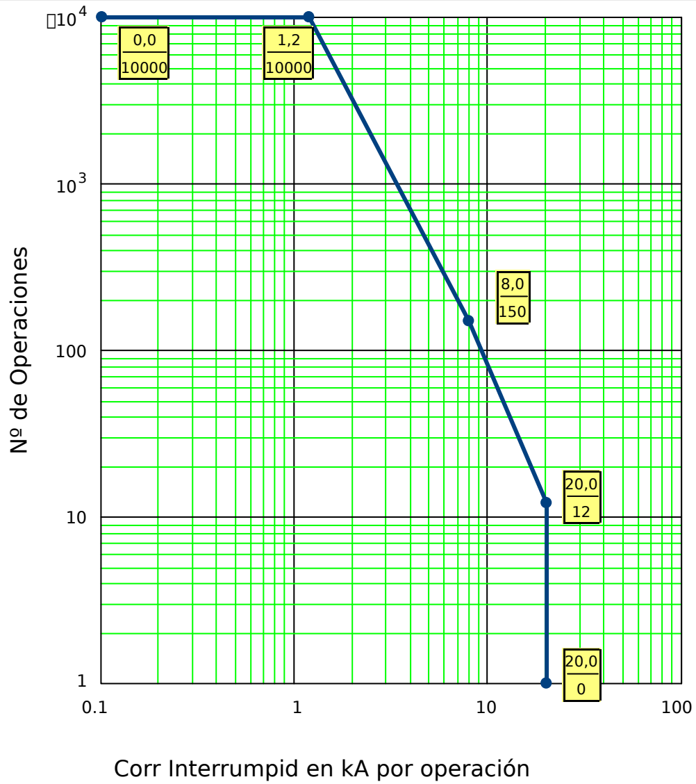
Fig. 124: Curva Mantenim Interruptor para Interrupt Circuito típico 25kV
