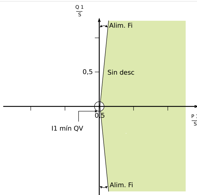
Fig. 99: Método 1 (supervisión de ángulo de potencia): «Método UFLS» = “Supervisión Ángulo Potencia”.
