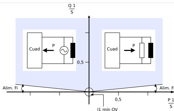
Fig. 91: Método 1: Supervisión de ángulo de potencia
