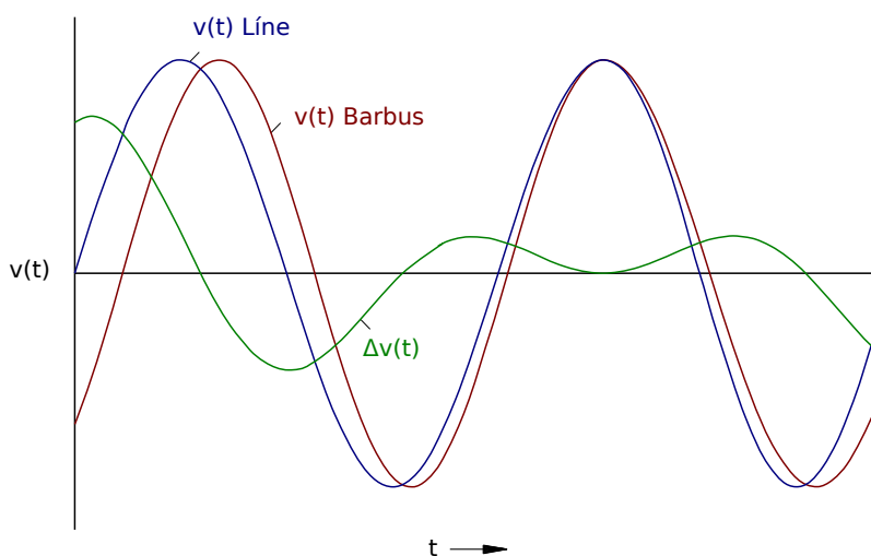
Fig. 110: Curva de tensión con resolución ampliada.
