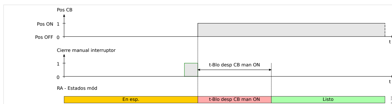
Fig. 105: Estados de reconexión automática durante el cierre manual del interruptor.
