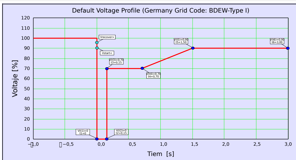
Fig. 80: Perfil de LVRT predeterminado (Tipo I de BDEW).
