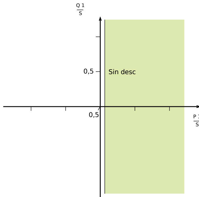
Fig. 100: Método 2 (supervisión de potencia activa pura): »Método UFLS« = "Superv. de potencia activa pura".
