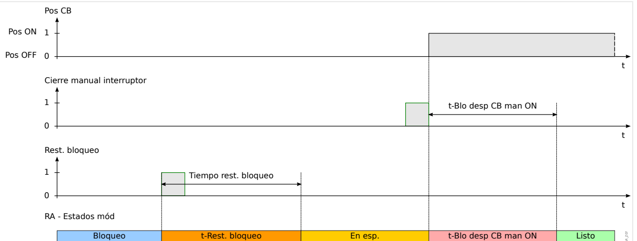
Fig. 107: Lógica de reinicio de bloqueo de AR en caso de que el reinicio de bloqueo llegue antes de que se cierre el interruptor manualmente.
