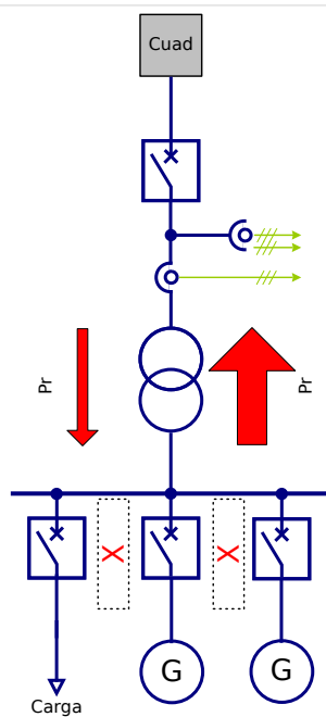
Fig. 98: Uso descentralizado en redes con alimentación predominante.
