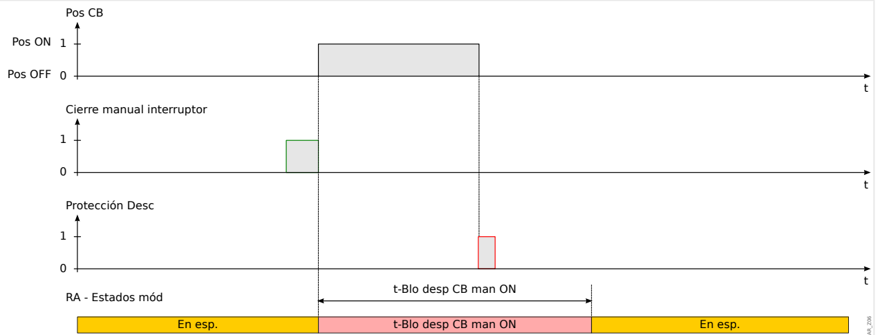
Fig. 106: Desconexión de protección mientras transcurre el tiempo de bloqueo de cierre manual.
