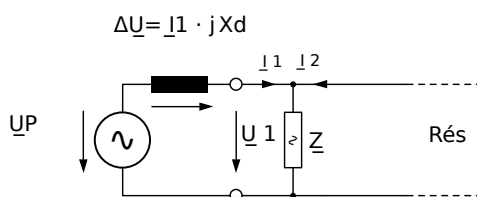
Fig. 84: Circuit équivalent au niveau du générateur synchrone en parallèle avec le réseau.
