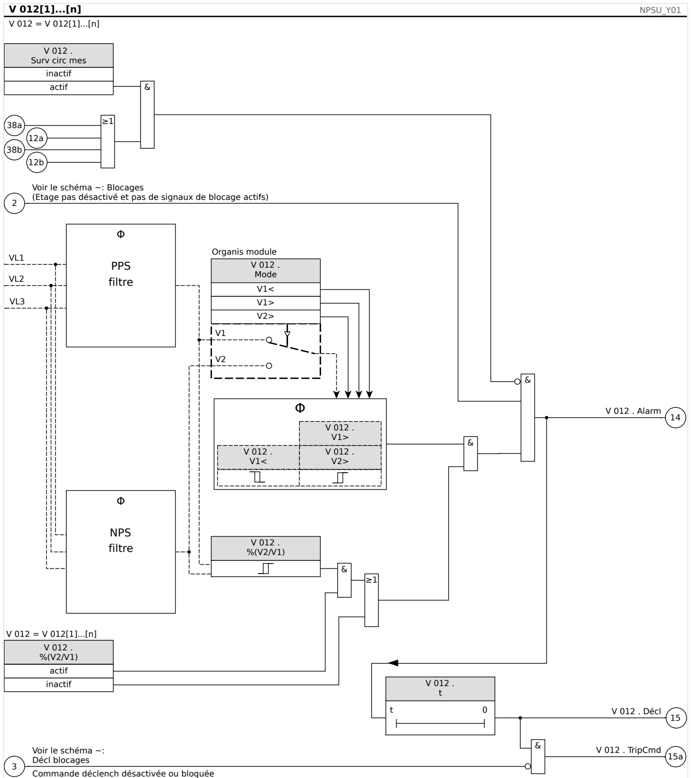
Fig. 83: Fonctionnalité du module »V 012«.
