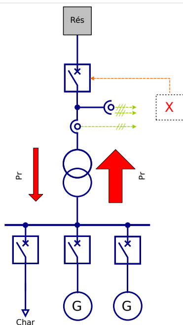
Fig. 97: Utilisation centralisée au sein de réseaux avec alimentation prédominante.
