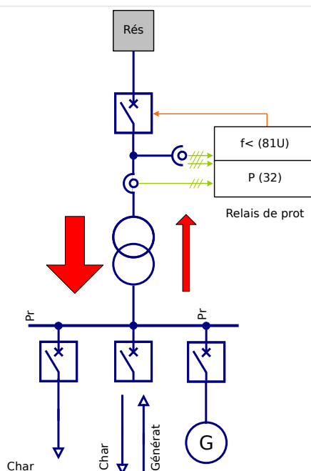
Fig. 95: Délestage de charge de sous-fréquence centralisé au sein de réseaux avec alimentation temporaire.
