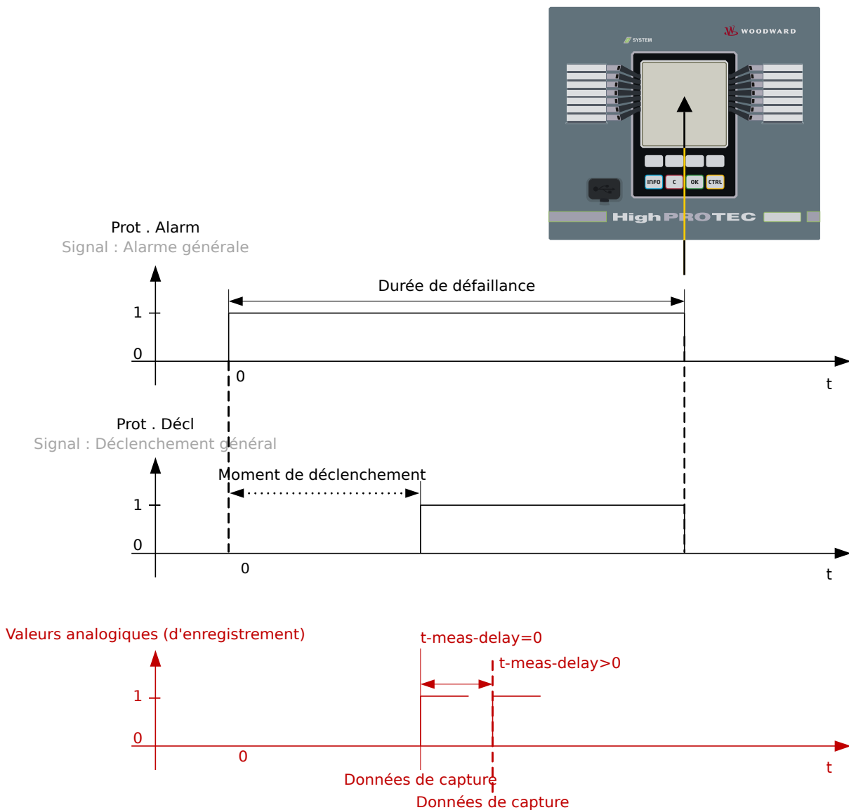
Fig. 129: Enregistreur de défaut : temps et durées
