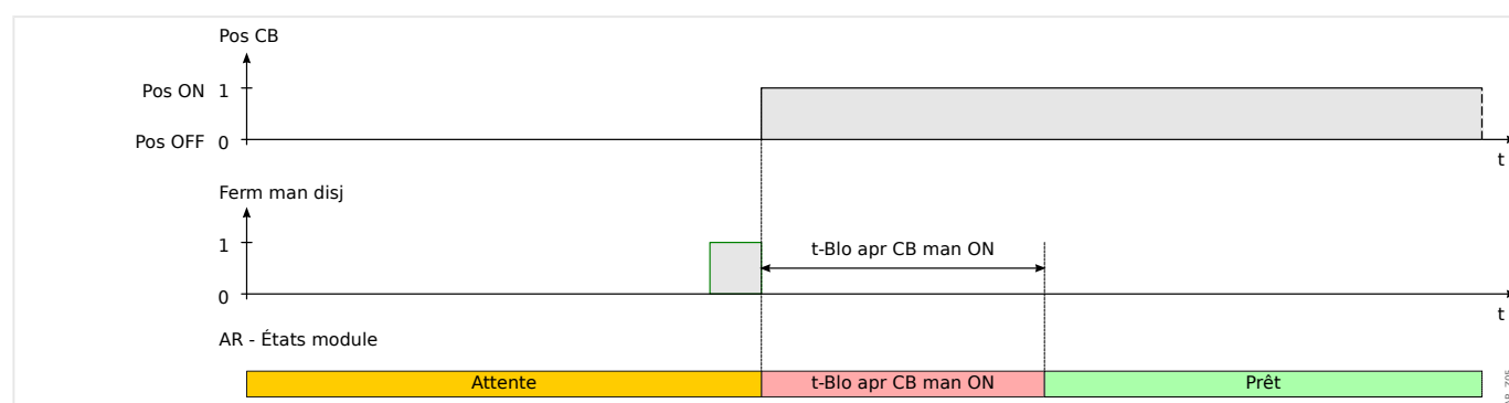
Fig. 105: États du réenclenchement automatique pendant la fermeture manuelle du disjoncteur.
