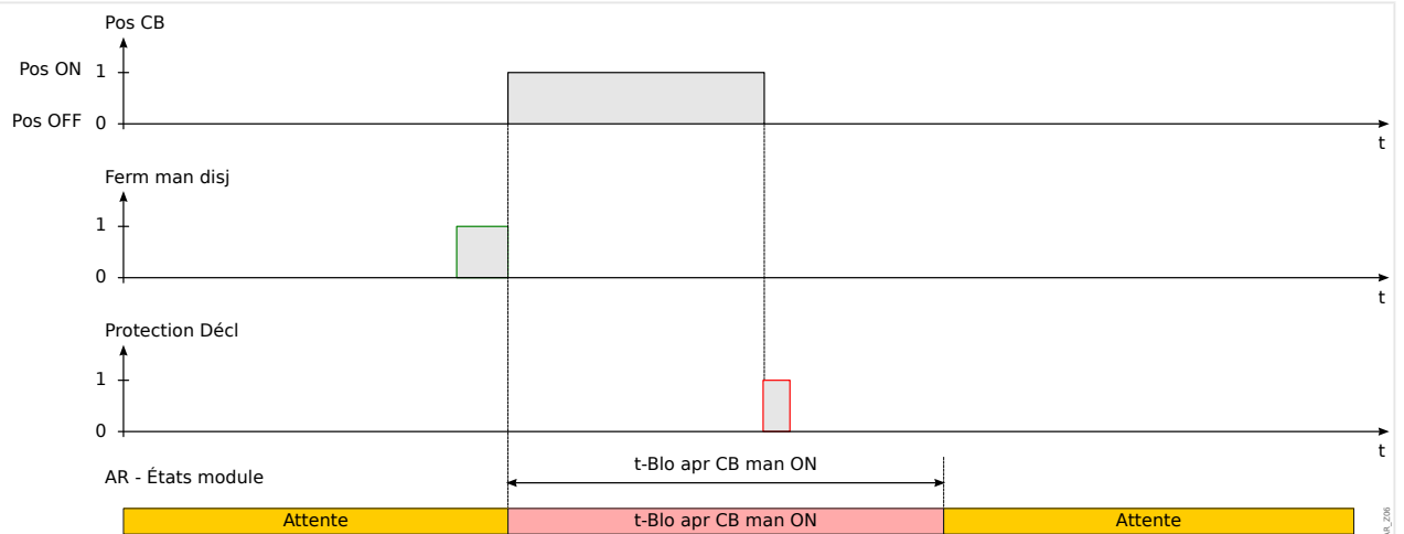
Fig. 106: Déclenchement de la protection pendant l'écoulement de la temporisation du blocage de fermeture manuelle.
