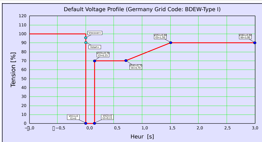
Fig. 80: Profil LVRT prédéfini en usine (BDEW-Type I).
