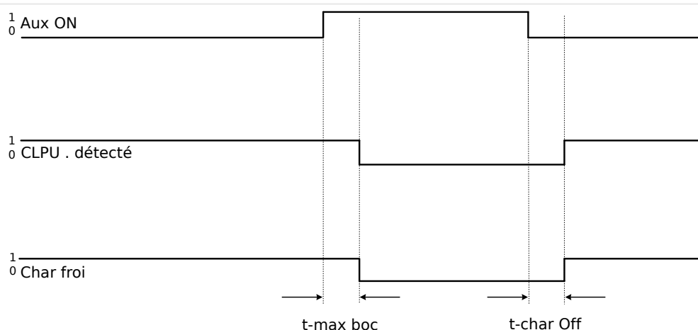
Fig. 113: Exemple de mode : Position du disjoncteur.
