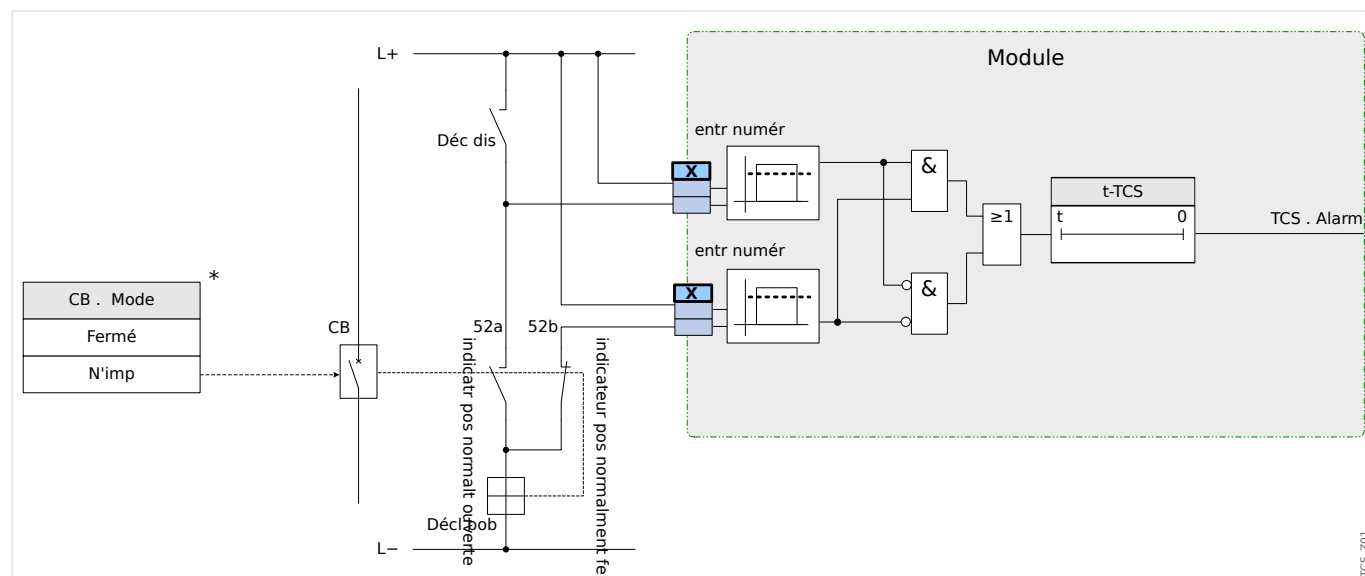
Fig. 115: Exemple de connexion : Surveillance du circuit de déclenchement avec de contacts auxiliaires de disjoncteur »Aux ON« (52a) et »Aux OFF« (52b).
