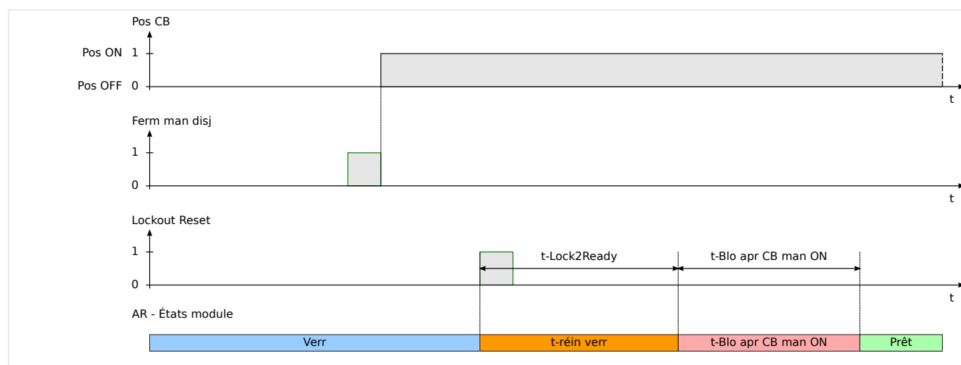
Fig. 108: Logique de réinitialisation du verrouillage du réenclenchement automatique si la réinitialisation du verrouillage se produit après la fermeture du disjoncteur manuelle.
