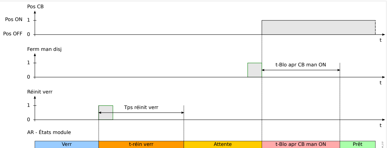
Fig. 107: Logique de réinitialisation du verrouillage du réenclenchement automatique si la réinitialisation du verrouillage se produit avant la fermeture du disjoncteur manuelle.
