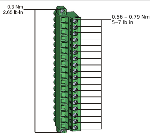
Fig. 139: Bornes de mesure de tension des cartes de mesure « TU-OR5 » et « TU-DI8 ».
