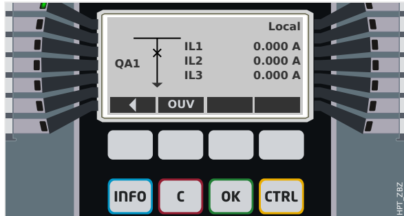
Fig. 119: Exemple de page de contrôle, avec le « disjoncteur » en position fermée.
