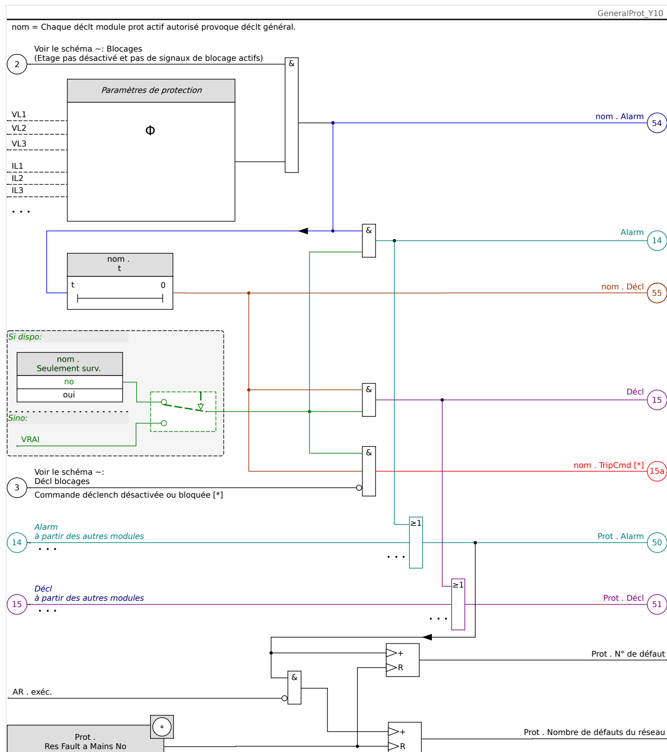
Fig. 61: Schéma de fonctionnalité des éléments de protection HighPROTEC.
