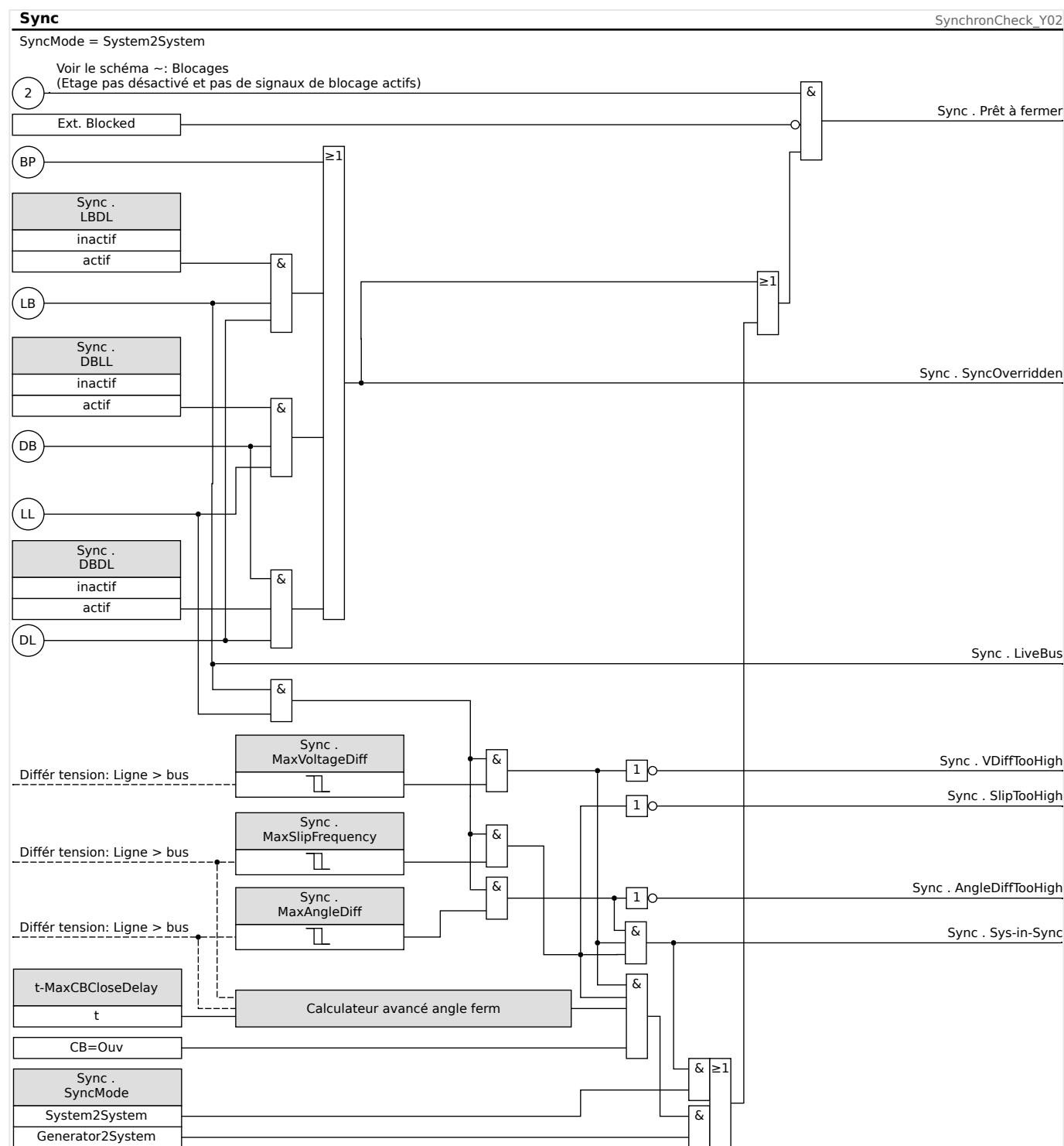
Fig. 112: Fonctionnalité du module »Sync«, « System2System ».
