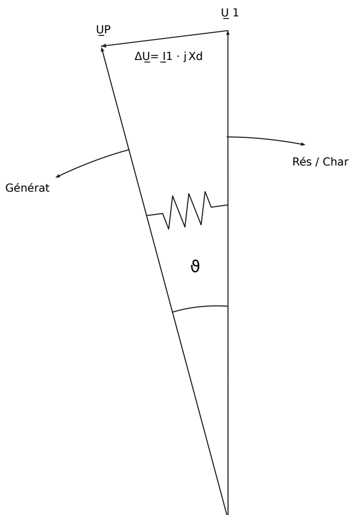
Fig. 85: Vecteurs de tension en fonctionnement parallèle du réseau.
