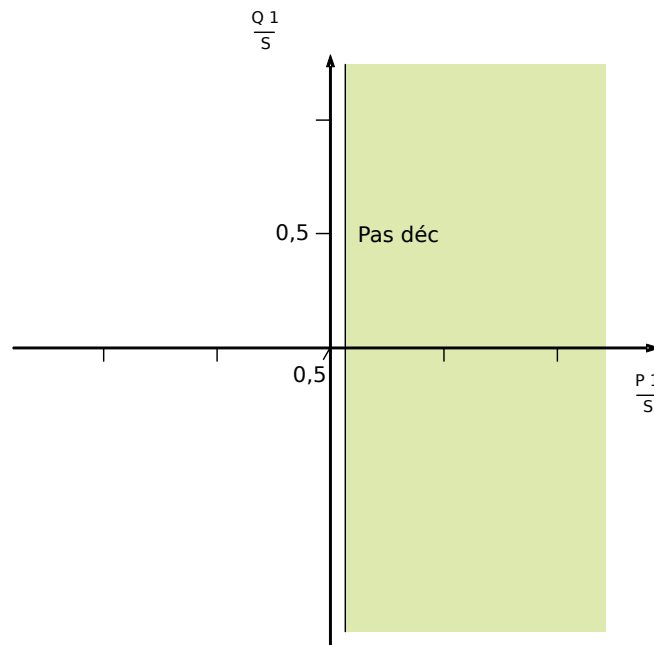
Fig. 100: Méthode 2 (Surveillance de la puissance active pure) : »Méthode UFLS« = "Surveillance de la puissance active pure".
