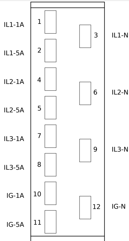
Fig. 18: TIs - Affectation électromécanique
