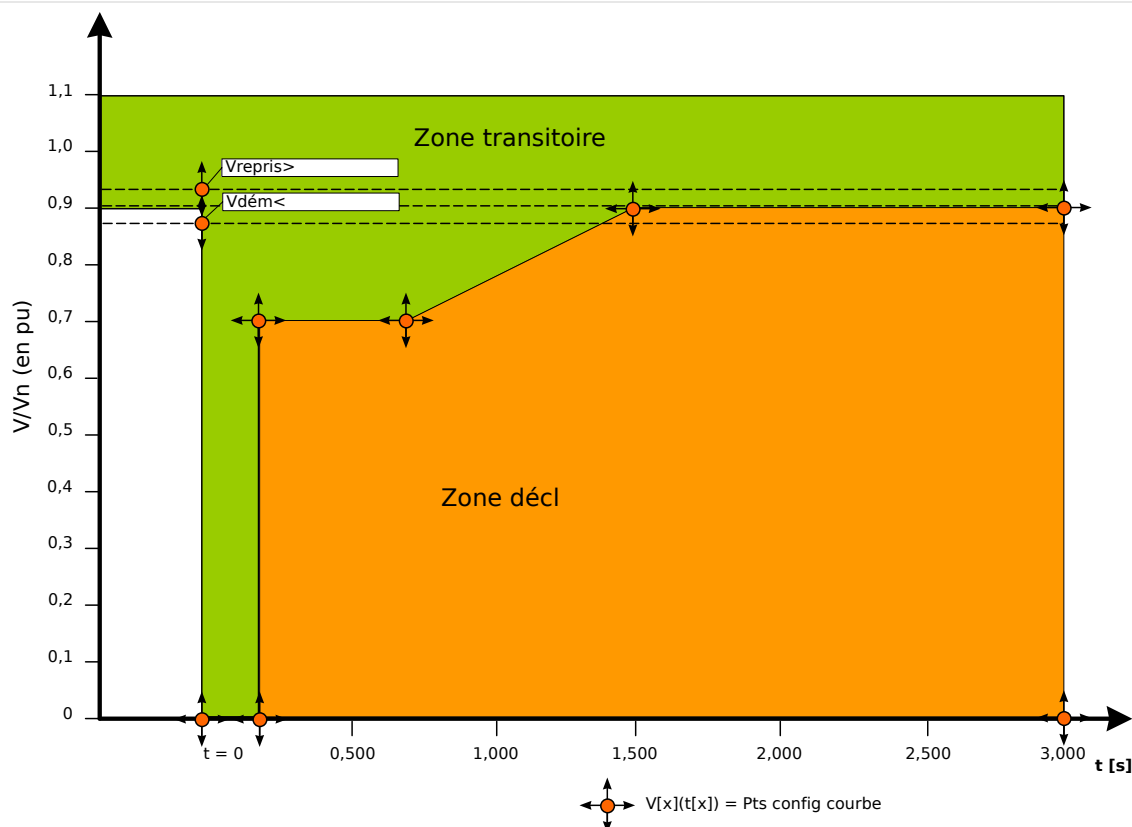
Fig. 79: Zone transitoire et zone de déclenchement
