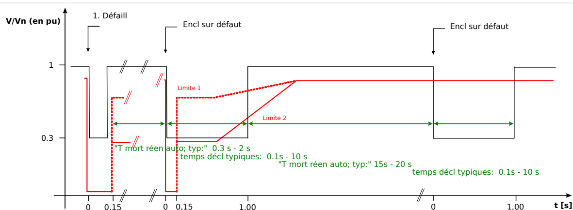
Fig. 78: Exécution d'une courbe de tension lors de l'échec d'un réenclenchement automatique en deux étapes ; source : Technische Richtlinie, Erzeugungsanlagen am Mittelspannungsnetz, Ausgabe Juni 2008, BDEW Bundesverband der Energie- und Wasserwirtschaft e.V. (Page 89).
