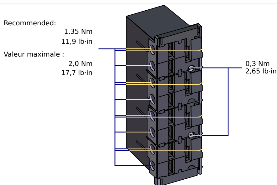
Fig. 137: Connecteur enfichable avec sectionneur intégré (Entrées de courant conventionnelles)
