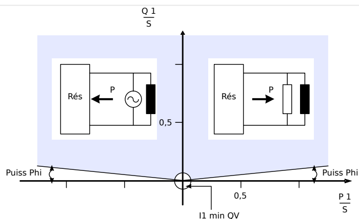
Fig. 91: Méthode 1 : Surveillance de l'angle de charge
