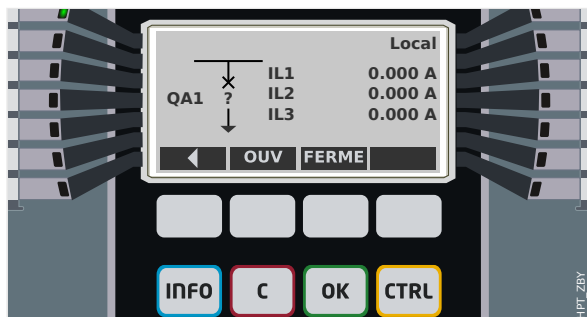
Fig. 120: Exemple de page de contrôle, avec le « disjoncteur » en position de dysfonctionnement (ou invraisemblable).
