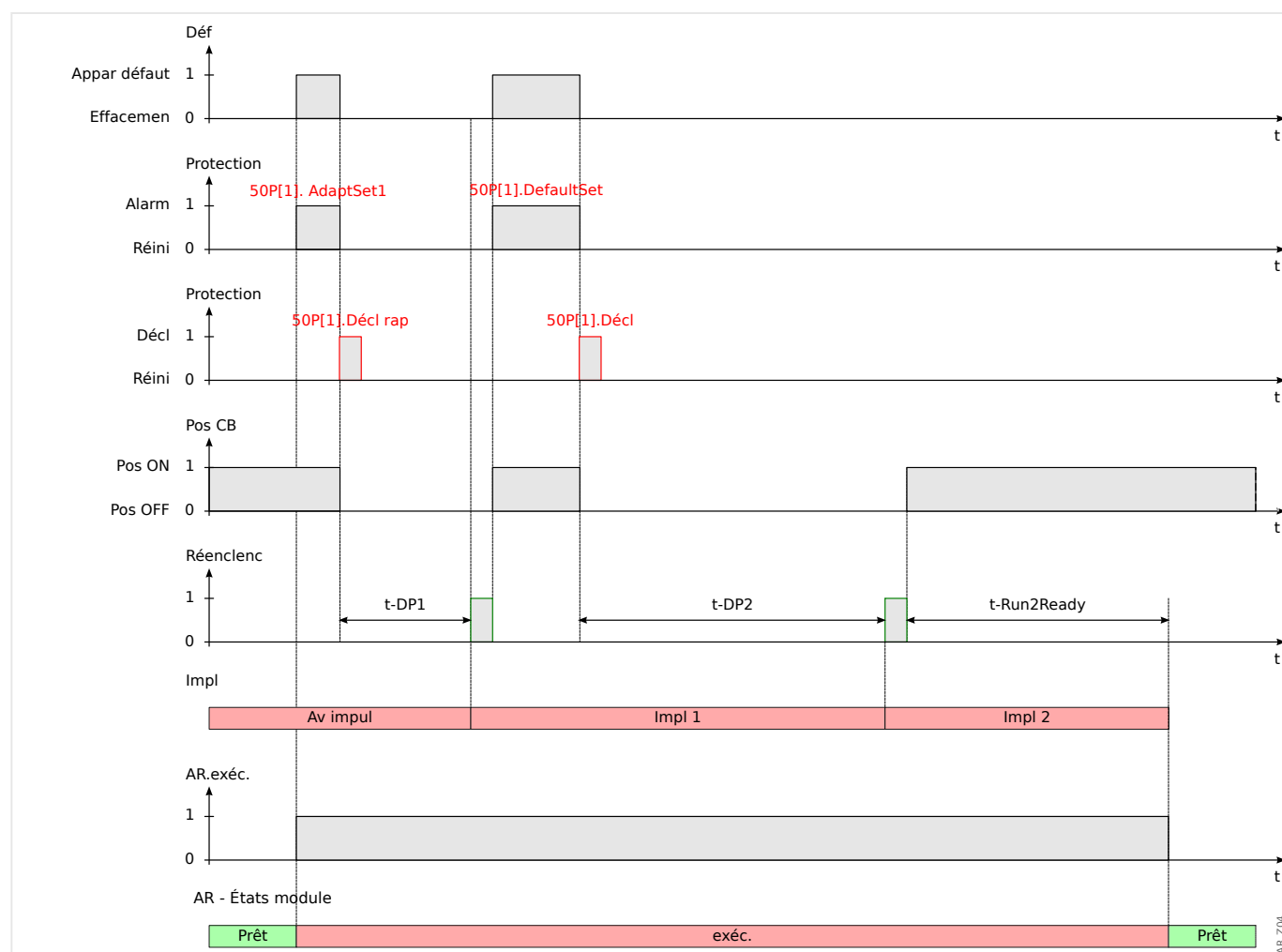
Fig. 104: Diagramme de temporisation de réenclenchement automatique pour un schéma de réenclenchement automatique à 2 impulsions réussi avec une accélération à la pré-impulsion.
