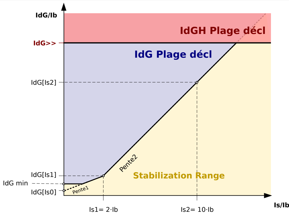
Fig. 53: Valeur d'excitation »IdG>>« du courant différentiel à la terre en fonction du courant nominal »Ib« de l'objet de protection associé.
