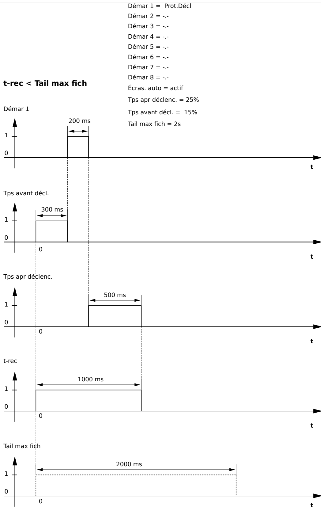
Fig. 72: Exemple de diagramme des temps de l'enregistreur de perturbations II
