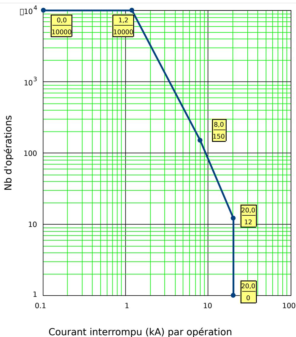
Fig. 68: Courbe de maintenance du disj pour un disj 25 ~kV typique
