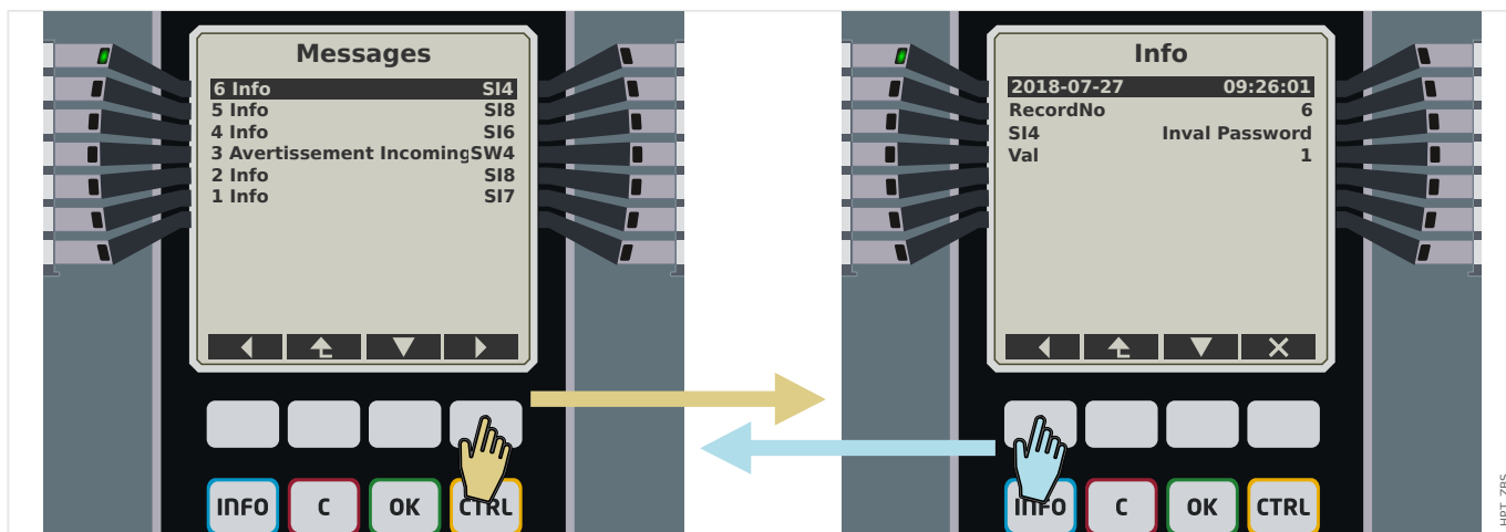
Fig. 80: Exemple d'affichage des messages d'auto-surveillance.
