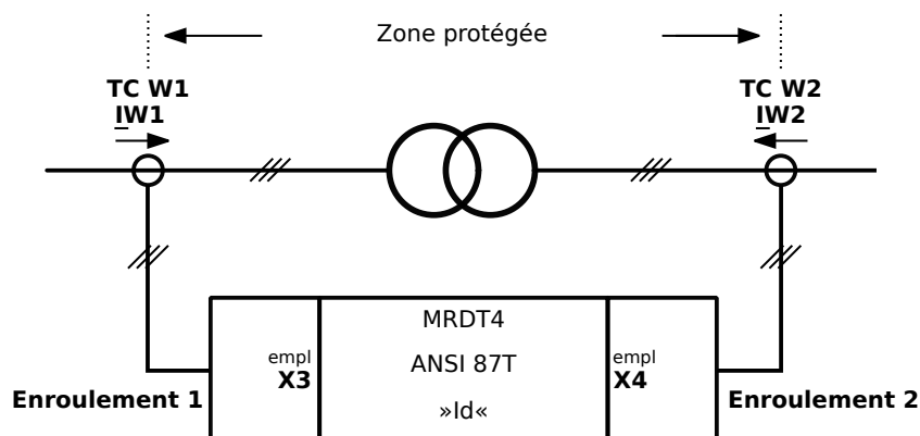
Fig. 47: ANSI 87T : Protection différentielle de phase de transformateur
