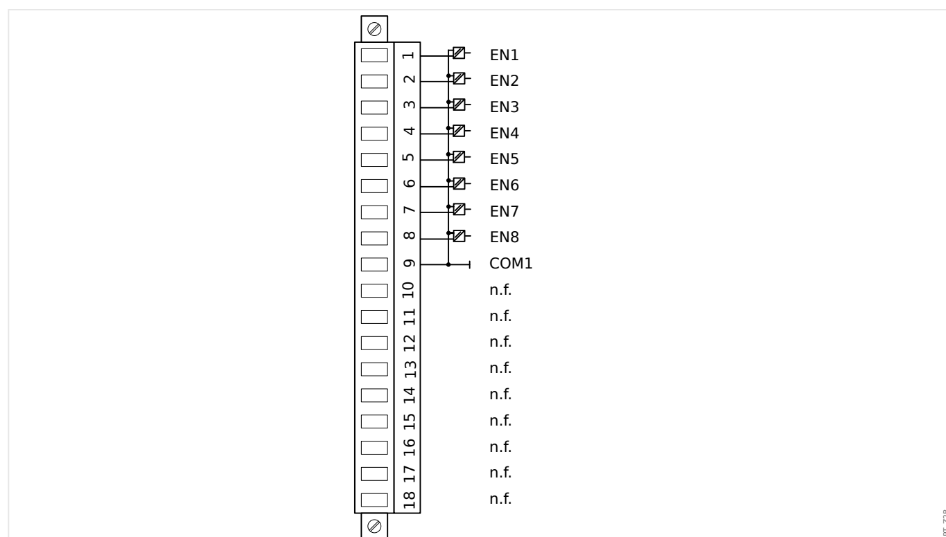
Fig. 23: Affectation électromécanique.
