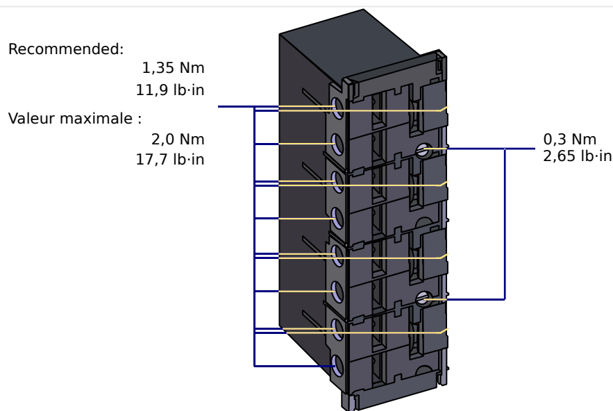
Fig. 81: Connecteur enfichable avec sectionneur intégré (Entrées de courant conventionnelles)
