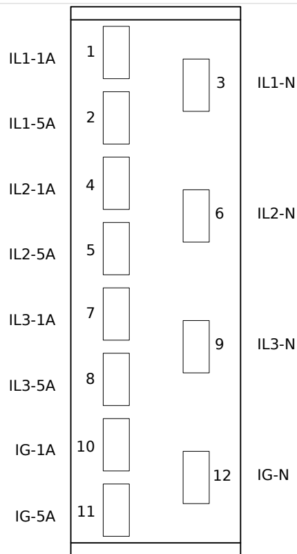
Fig. 18: TIs - Affectation électromécanique
