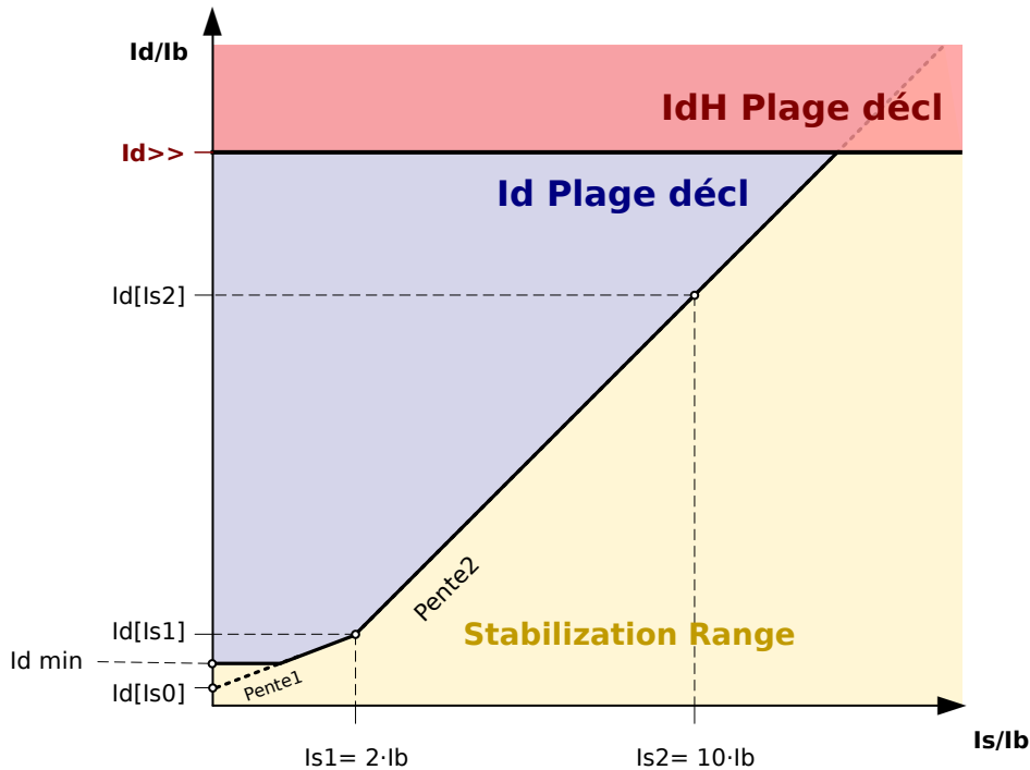
Fig. 48: Courbes de déclenchement des fonctions de protection »Id« (zone bleue) et »IdH« (zone rouge).
