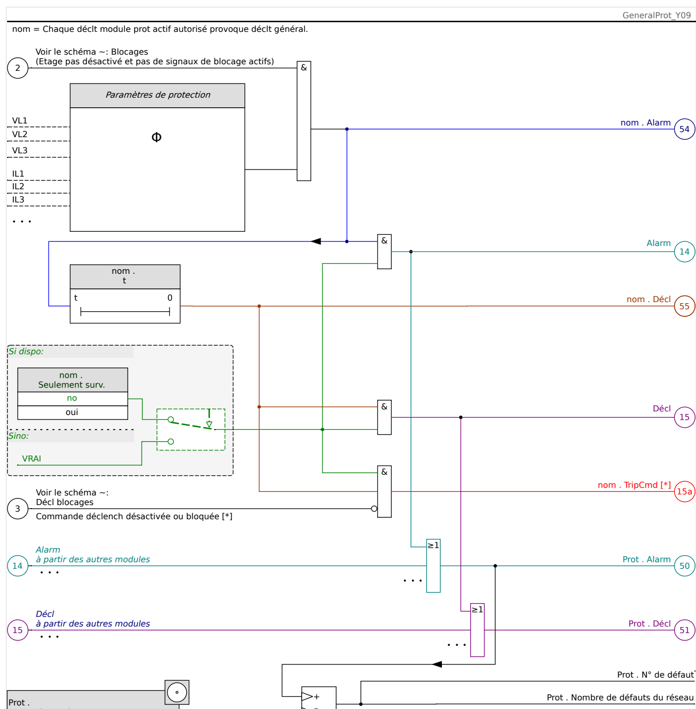
Fig. 45: Schéma de fonctionnalité des éléments de protection HighPROTEC.
