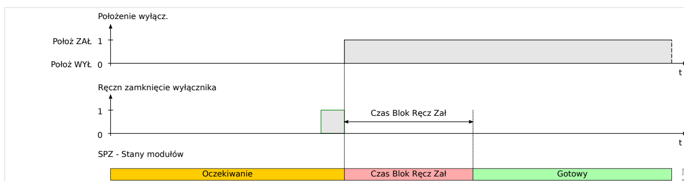
Rys. 52: Stany SPZ podczas ręcznego zamykania wyłącznika.
