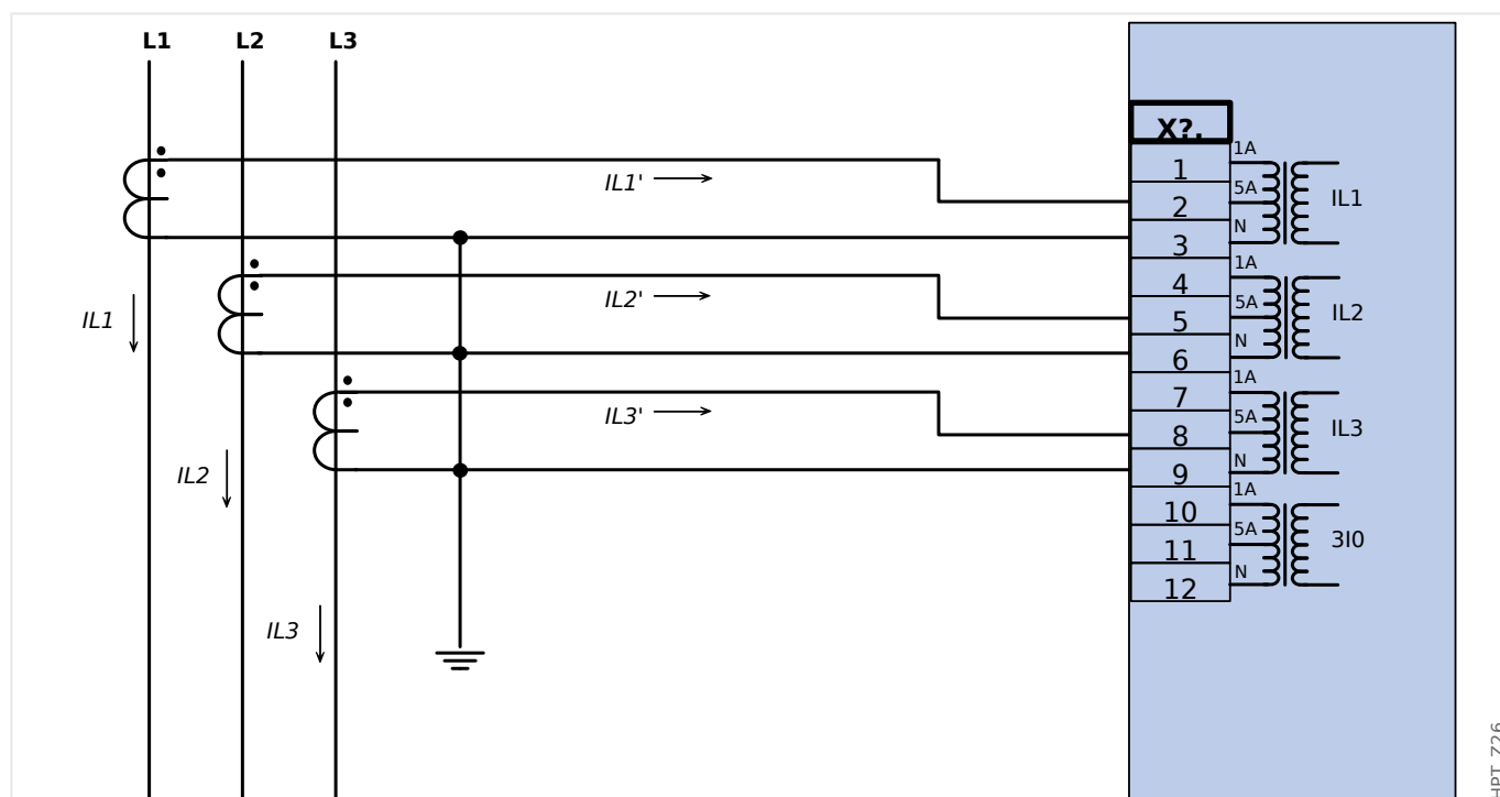
Rys. 19: Trójfazowy pomiar prądu; I_n wtórny = 5 A.
