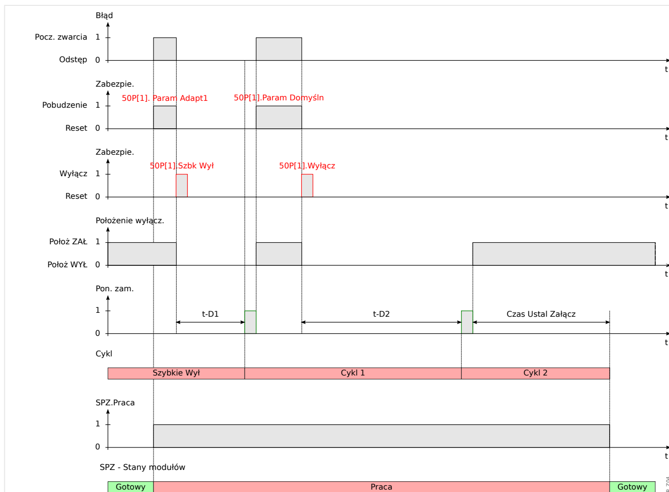
Rys. 51: Schemat czasów SPZ w przypadku udanego planu SPZ z 2 próbami i przyspieszeniem przy próbie wstępnej
