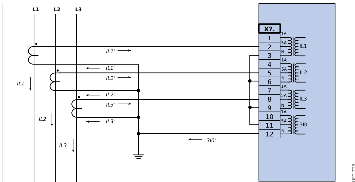
Rys. 21: Trójfazowy pomiar prądu; I_n wtórny = 5 A. Pomiar prądu doziemnego w układzie Holmgreena 3I0n wtórny = 5 A.
