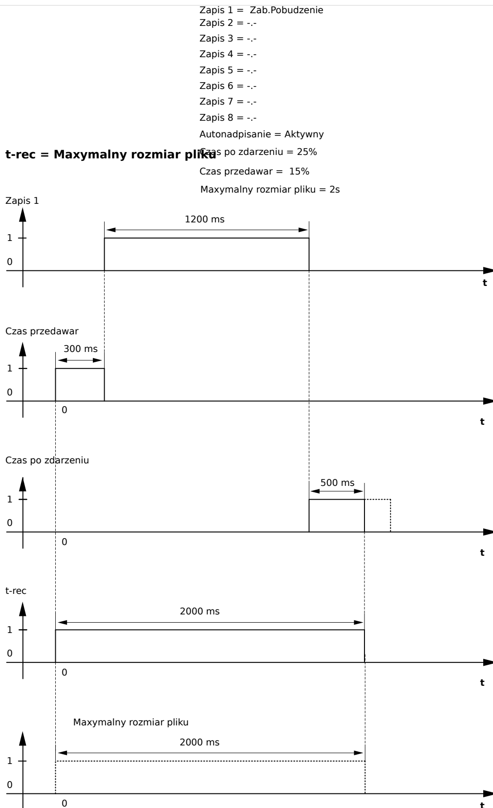
Rys. 69: Przykładowy wykres czasów pracy rejestratora zakłóceń I
