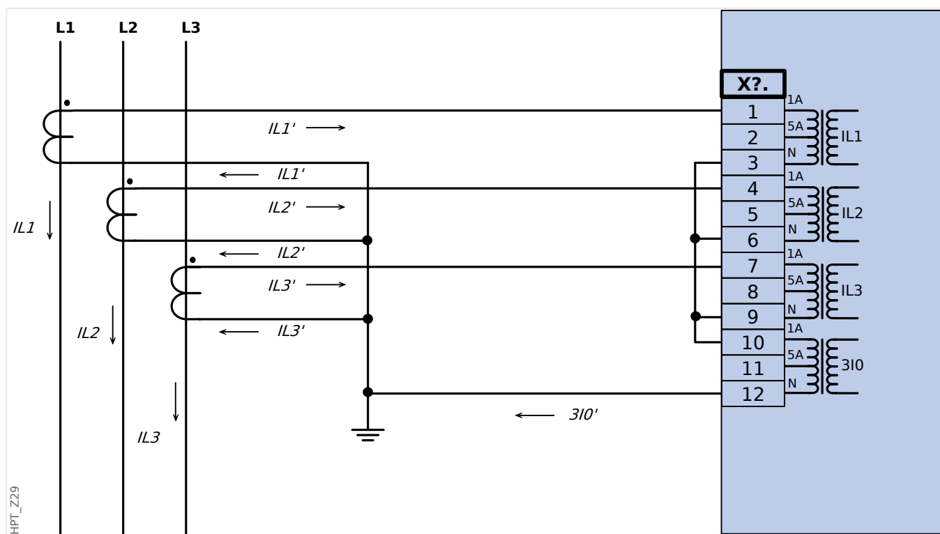
Rys. 22: Trójfazowy pomiar prądu; I_n wtórny = 1 A. Pomiar prądu doziemnego w układzie Holmgreena 3I0n wtórny = 1 A.
