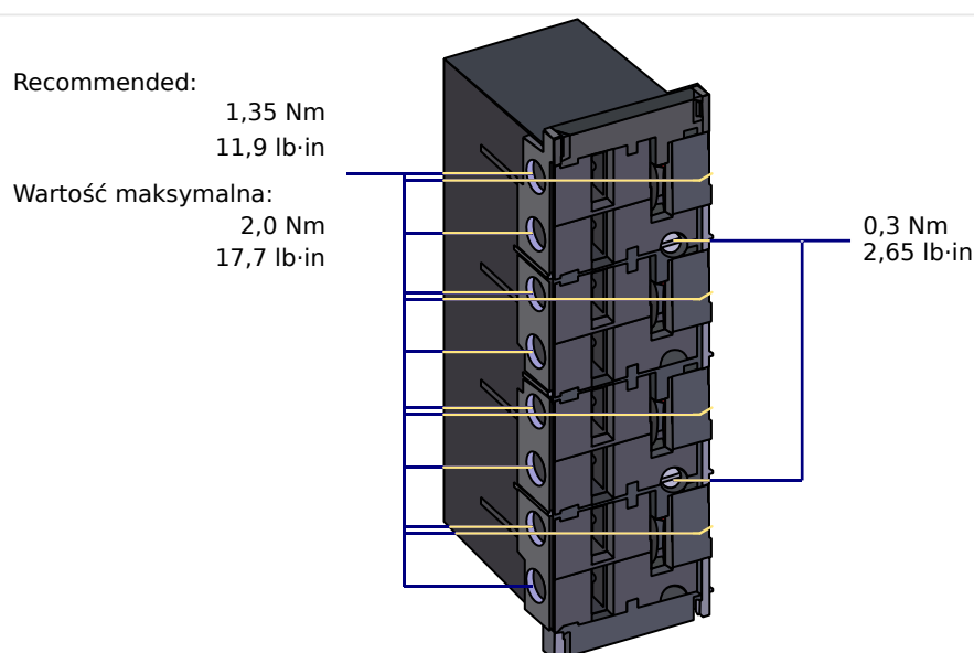
Rys. 79: Łącznik wtykowy ze zintegrowanym elementem zwarciovym (konwencjonalne wejścia prądowe)
