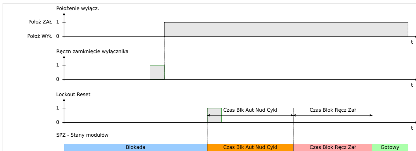
Rys. 55: Logika resetowania blokady automatyki SPZ w przypadku odebrania sygnału resetowania blokady po ręcznym zamknięciu wyłącznika.
