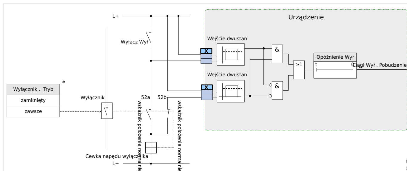
Rys. 58: Przykład okablowania: Układ kontroli ciągłości obwodów wyłącznika z dwoma stykami pomocniczymi wyłącznika „Położ ZAŁ” (52a) i „Położ WYŁ” (52b).
