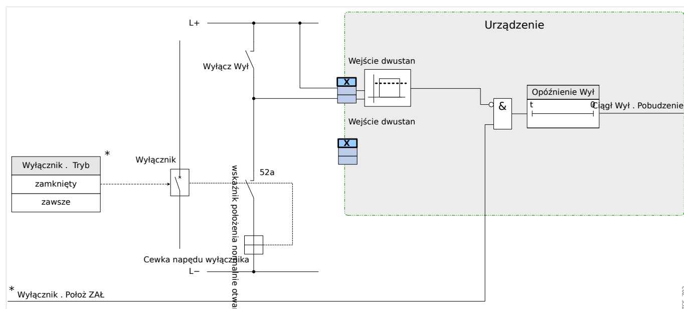
Rys. 59: Przykład okablowania: Układ kontroli ciągłości obwodów wyłącznika z tylko jednym stykiem pomocniczym wyłącznika „Położ ZAŁ” (52a).
