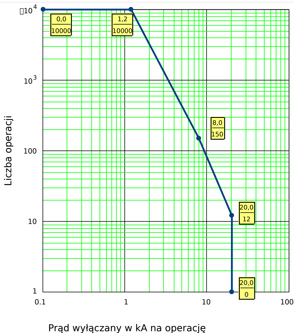
Rys. 66: Krzywa konserwacji wyłącznika typowego wyłącznika 25 kV
