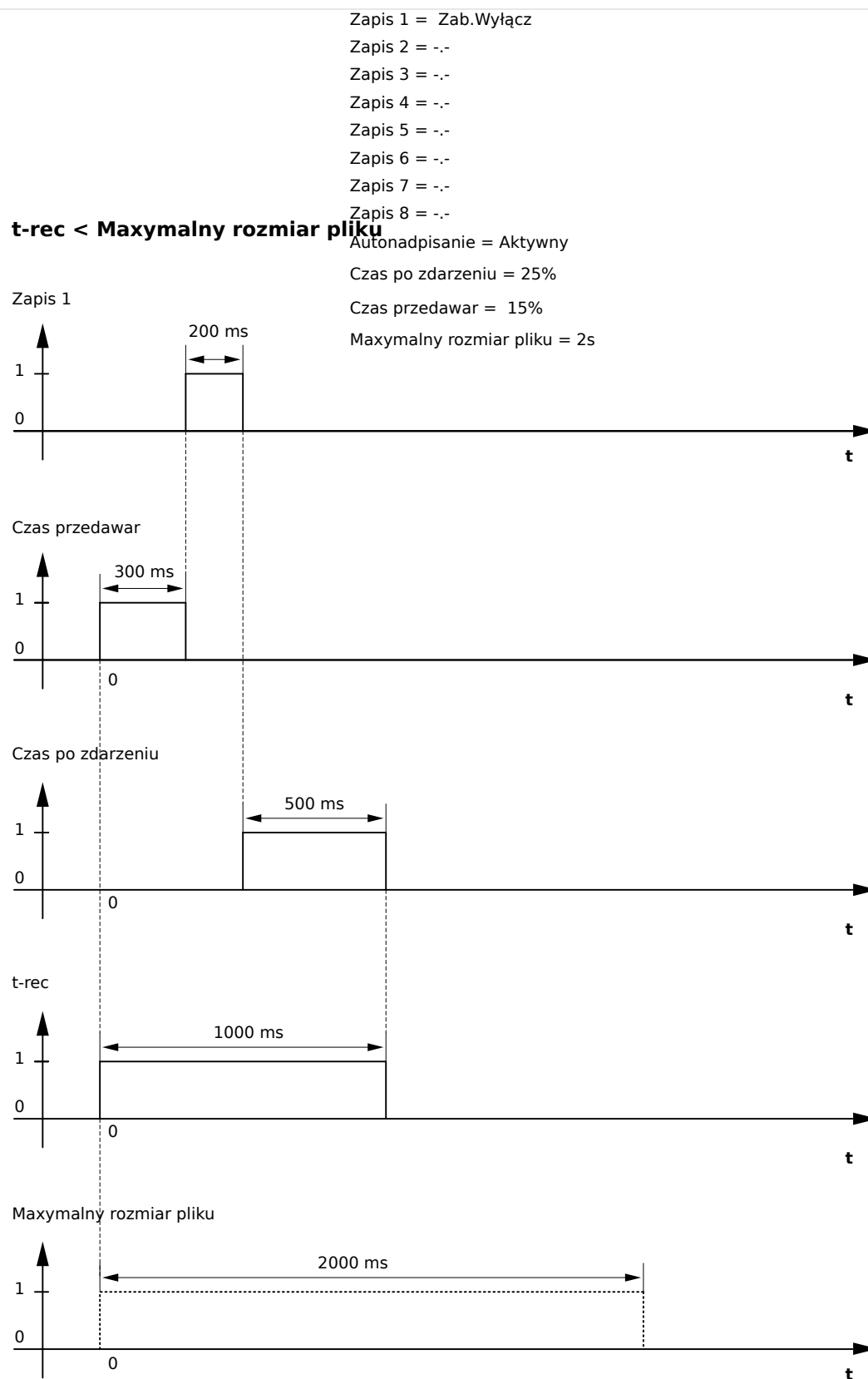
Rys. 70: Przykładowy wykres czasów pracy rejestratora zakłóceń II
