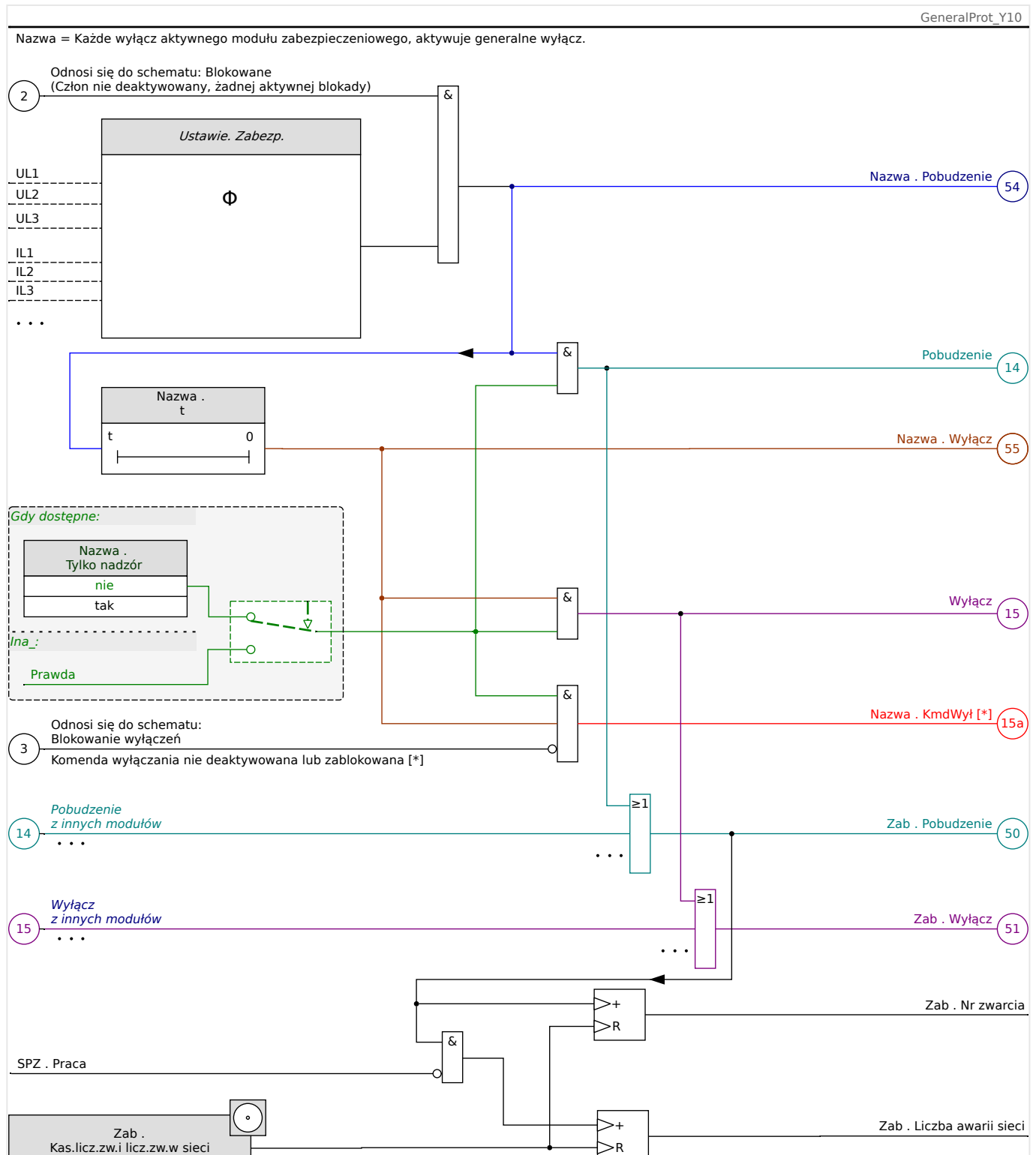
Rys. 43: Schemat ogólny działania każdego elementu zabezpieczającego HighPROTEC.
