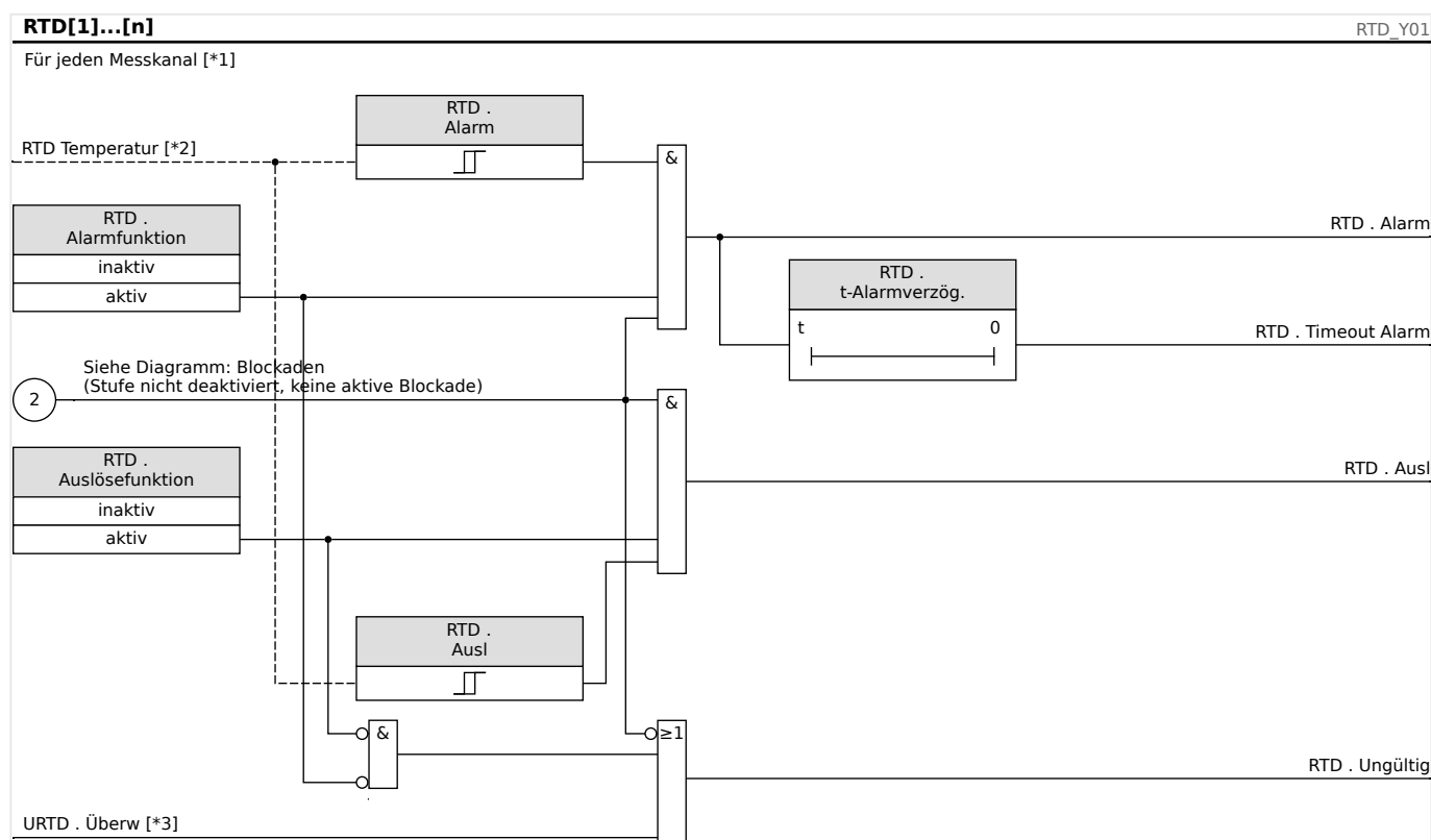
Abb. 65: Generelles RTD-Funktionsprinzip.
