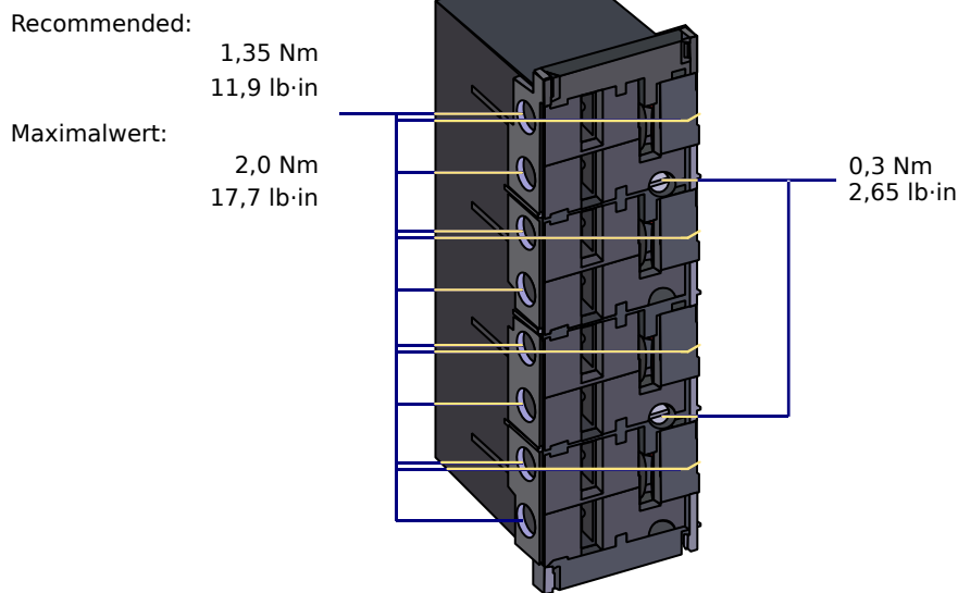
Abb. 87: Steckverbinder mit integrierten Kurzschließern (konventionelle Stromeingänge)
