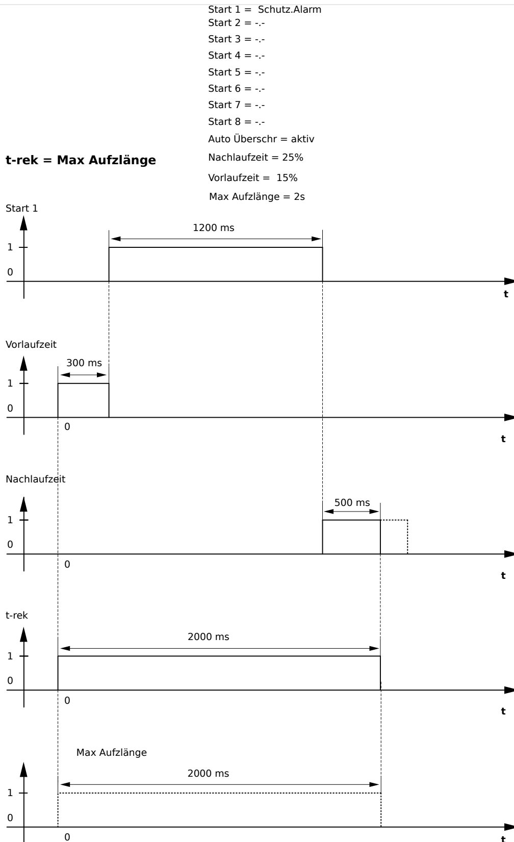
Abb. 77: Beispiel I Störschreiber-Ablaufdiagramm
