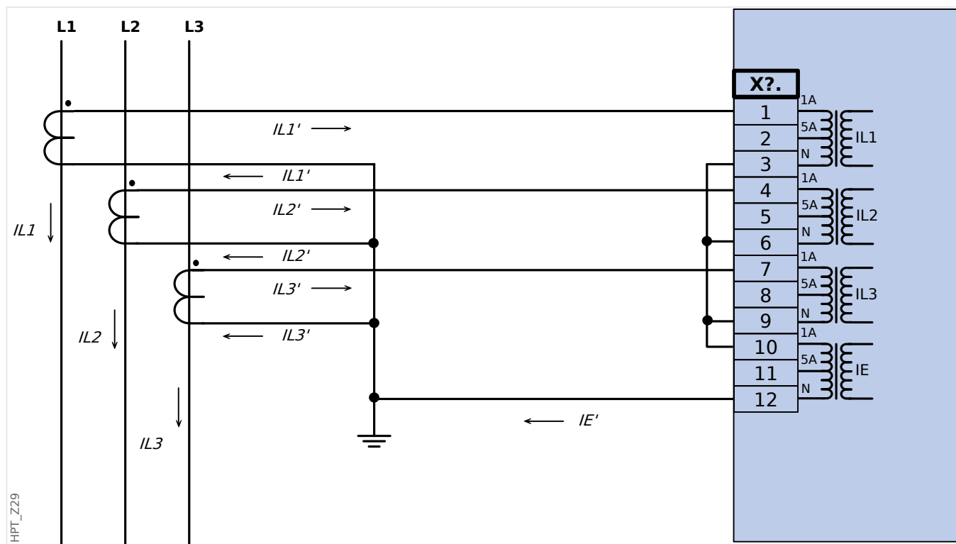
Abb. 26: Dreiphasiger Stromwandleranschluss; In sekundär = 1 A. Erdstromerfassung über Holmgreenschaltung IEn sekundär = 1 A.
