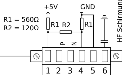
Abb. 37: Elektromechanische Zuordnung
