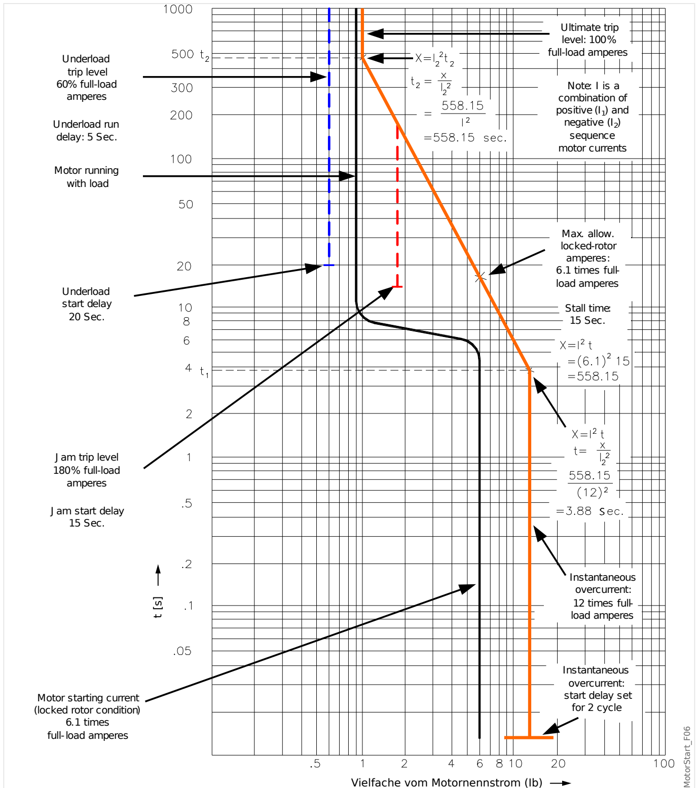
Abb. 58: Auslösekennlinie (Beispiel 2 - ohne RTDs).
