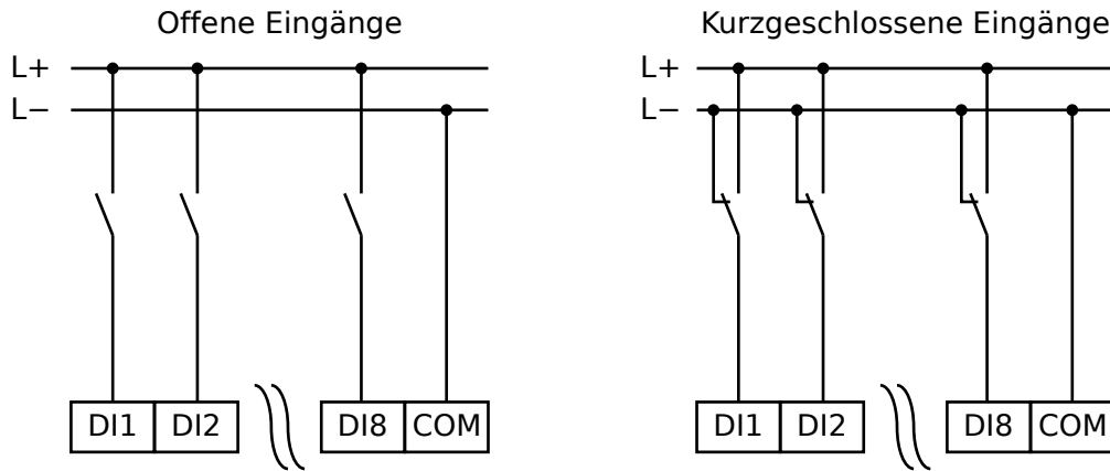
Abb. 88: Sicherer Zustand der digitalen Eingänge
