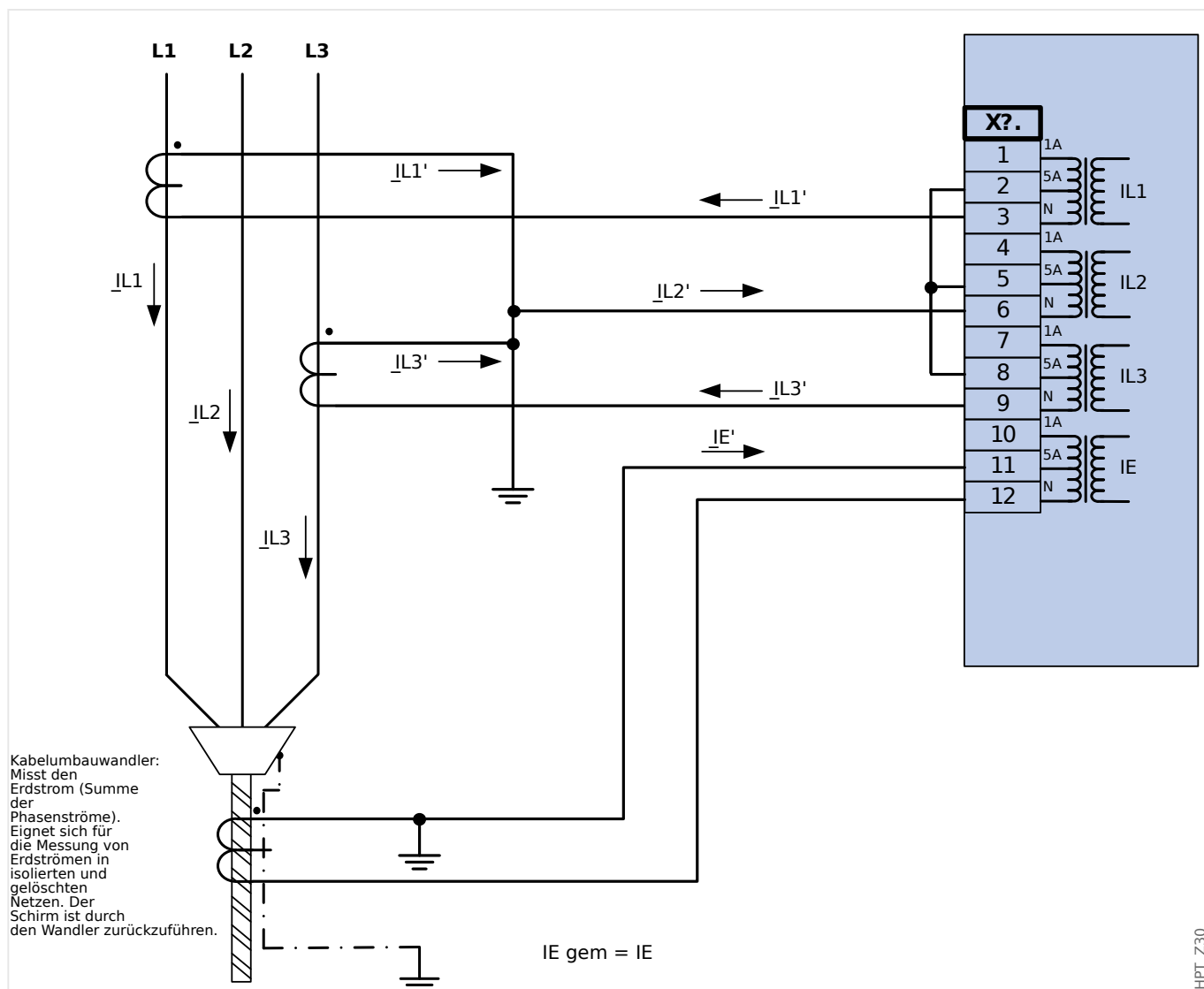
Abb. 27: Zweiphasiger Stromwandleranschluss in V-Schaltung; In sekundär = 5 A. Erdstromerfassung über Kabelumbauwandler; IEn sekundär = 5 A.
