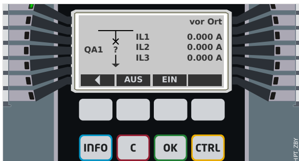
Abb. 70: Beispiel einer Steuer-Seite mit „Leistungsschalter“ in Störstellung (bzw. unplausiblem Zustand).
