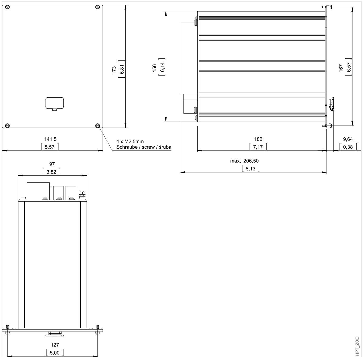
Abb. 4: 3-Seiten-Ansicht B1-Gehäuse in 19“-Ausführung. (Alle Angaben in mm, Maße in eckigen Klammern in Zoll.)
