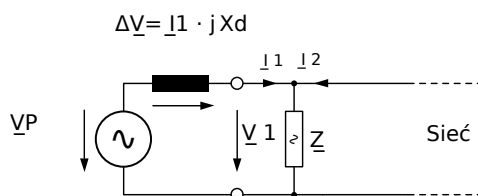
Rys. 78: Schemat zastępczy dla prądnicy synchronicznej pracującej równolegle z siecią.
