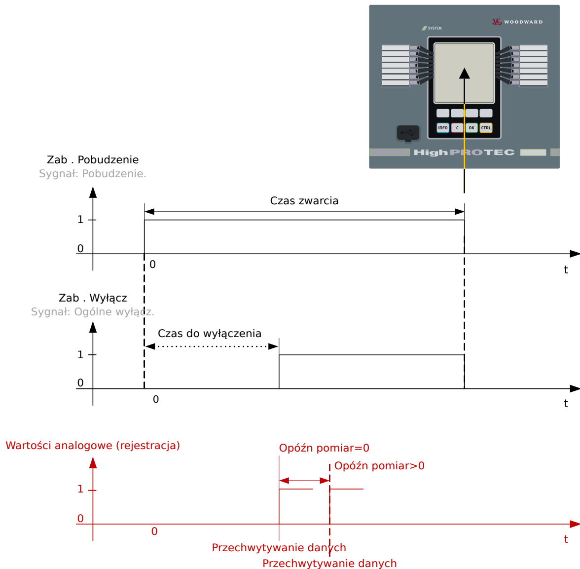
Rys. 101: Rejestrator zwarć: czasy (trwania).
