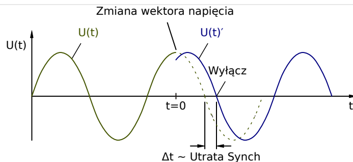
Rys. 82: Zmiana wektora napięcia.
