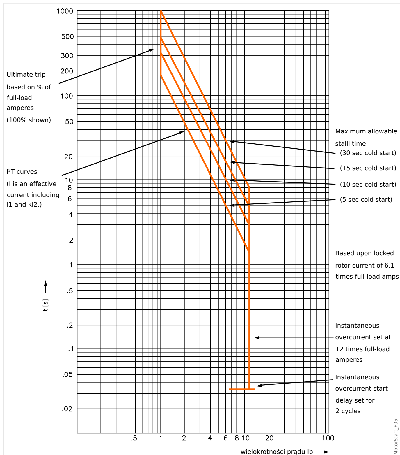
Rys. 67: Krzywa zabezpieczenia silnika (przykład 1).
