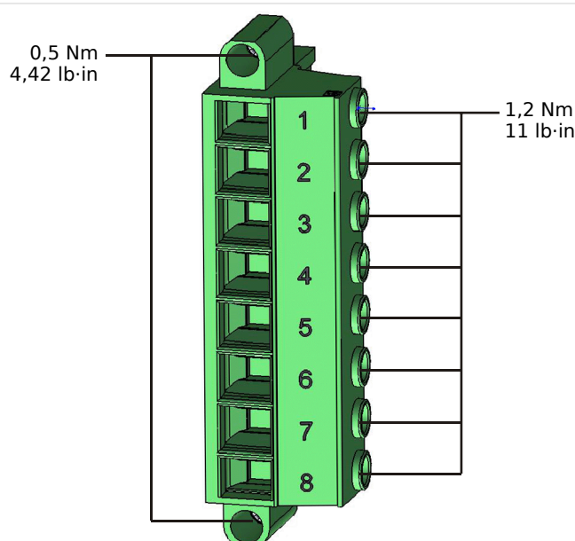
Rys. 110: Zaciski pomiaru napięcia karty pomiarowej „TU” (➡ „2.6.1 TU — wejścia do pomiaru napięcia”).
