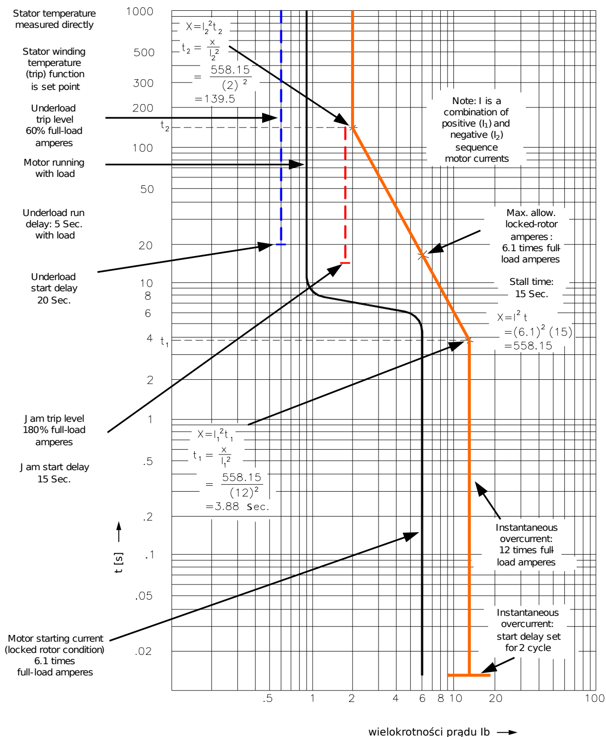
Rys. 69: Krzywa zabezpieczenia silnika (przykład 3 — z RCT).
