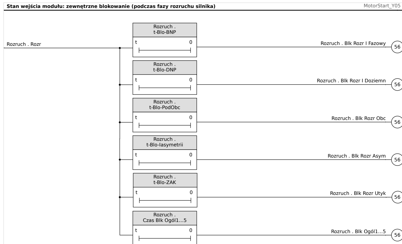
Rys. 60: Tymczasowe zablokowanie funkcji zabezpieczenia prądowego podczas rozruchu silnika.
