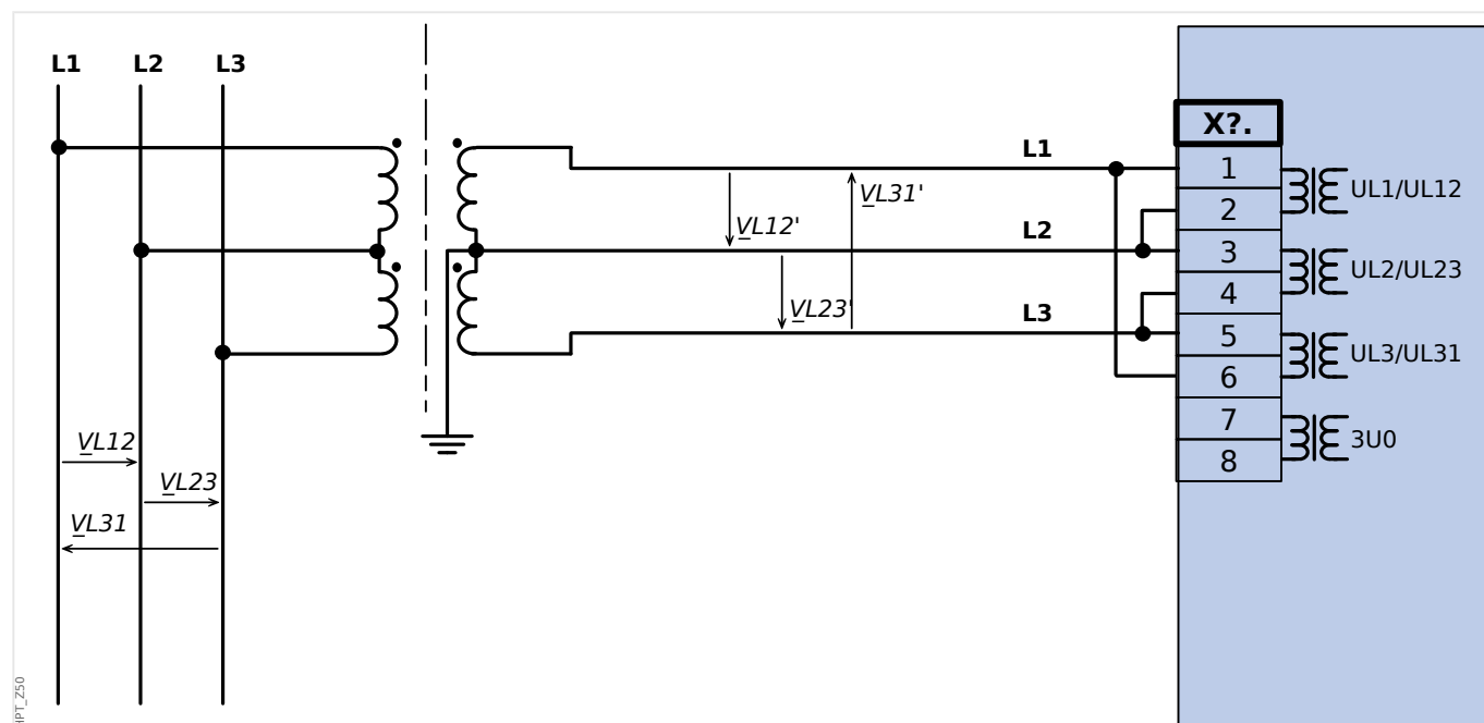
Rys. 32: Pomiar napięcia dla dwóch faz w układzie otwartego trójkąta
