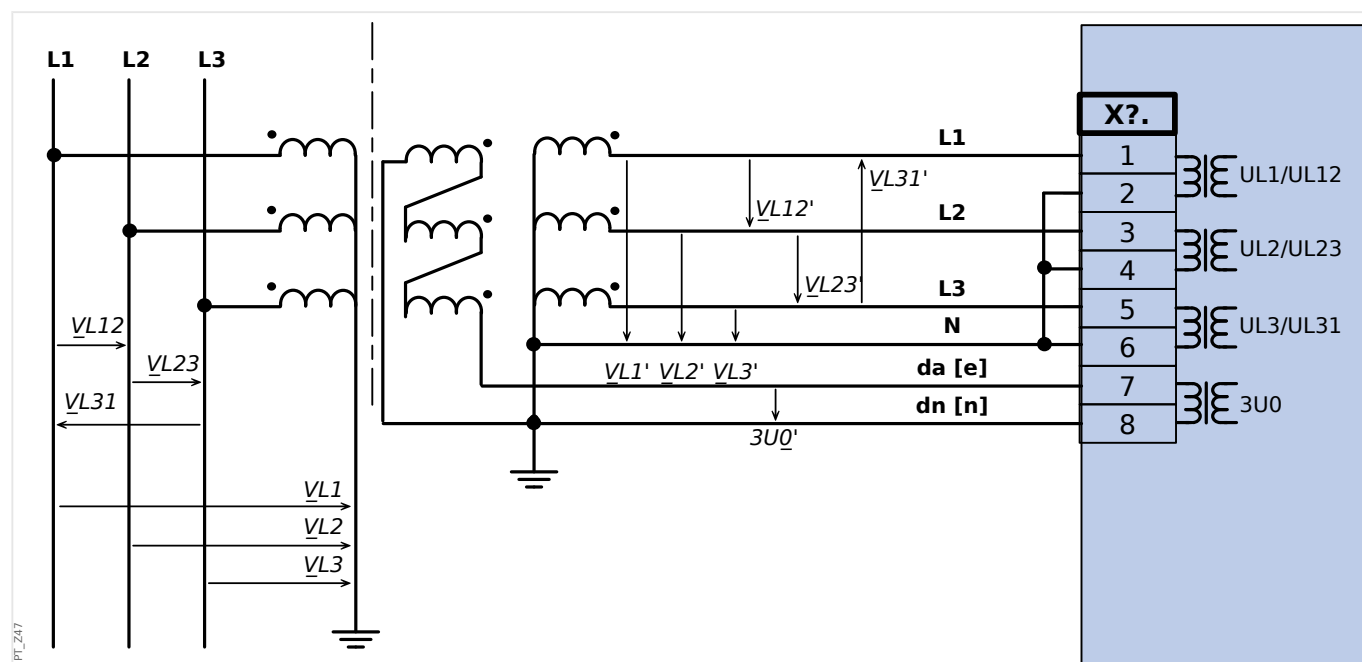
Rys. 29: Przekładnik napięciowy połączony w gwiazdę z otwartym trójkątem.
