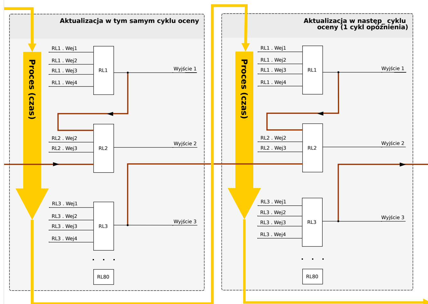
Rys. 106: Ukł. kaskadowy w porządku malejącym.
