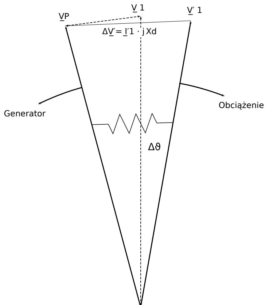
Rys. 81: Wektory napięcia przy awarii sieci.
