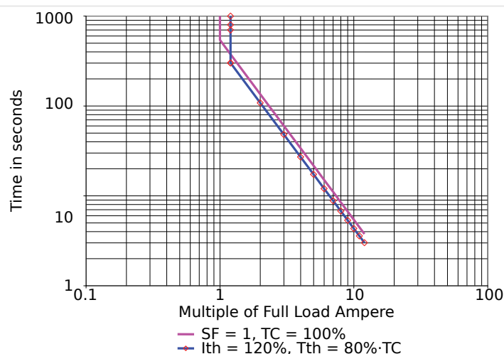
Rys. 65: Limit modelu cieplnego i krzywe wyzwalania bez RCT.
