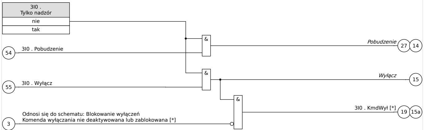
Rys. 73: Zabezpieczenie nadprądowe ziemnozwarciowe, część 2 (komenda wyzwolenia oraz inicjowanie alarmu ogólnego i wyzwolenia ogólnego).
