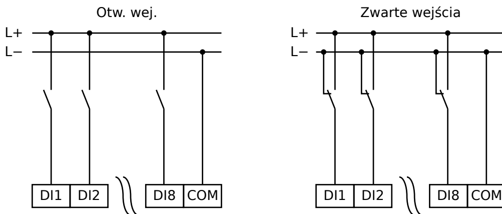
Rys. 111: Stan bezpieczny wejść dwustanowych
