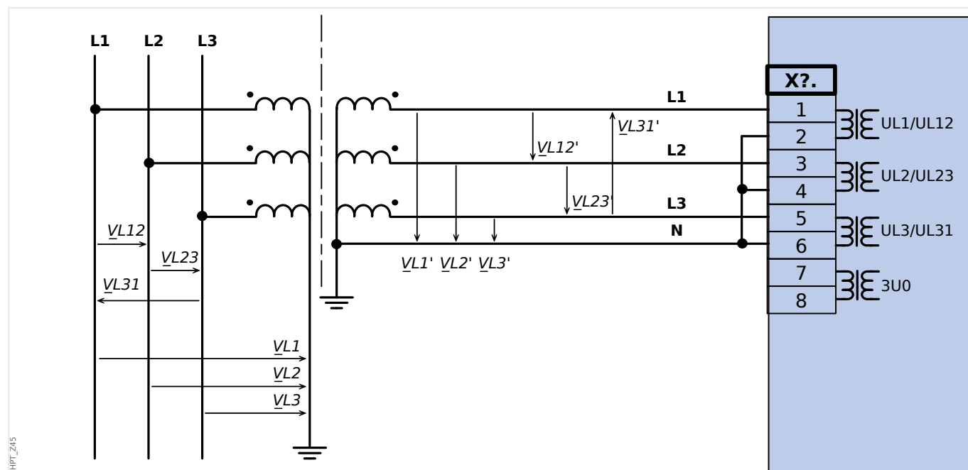
Rys. 28: Przekładnik napięciowy połączony w gwiazdę: Trójfazowy pomiar napięcia w układzie gwiazdy
