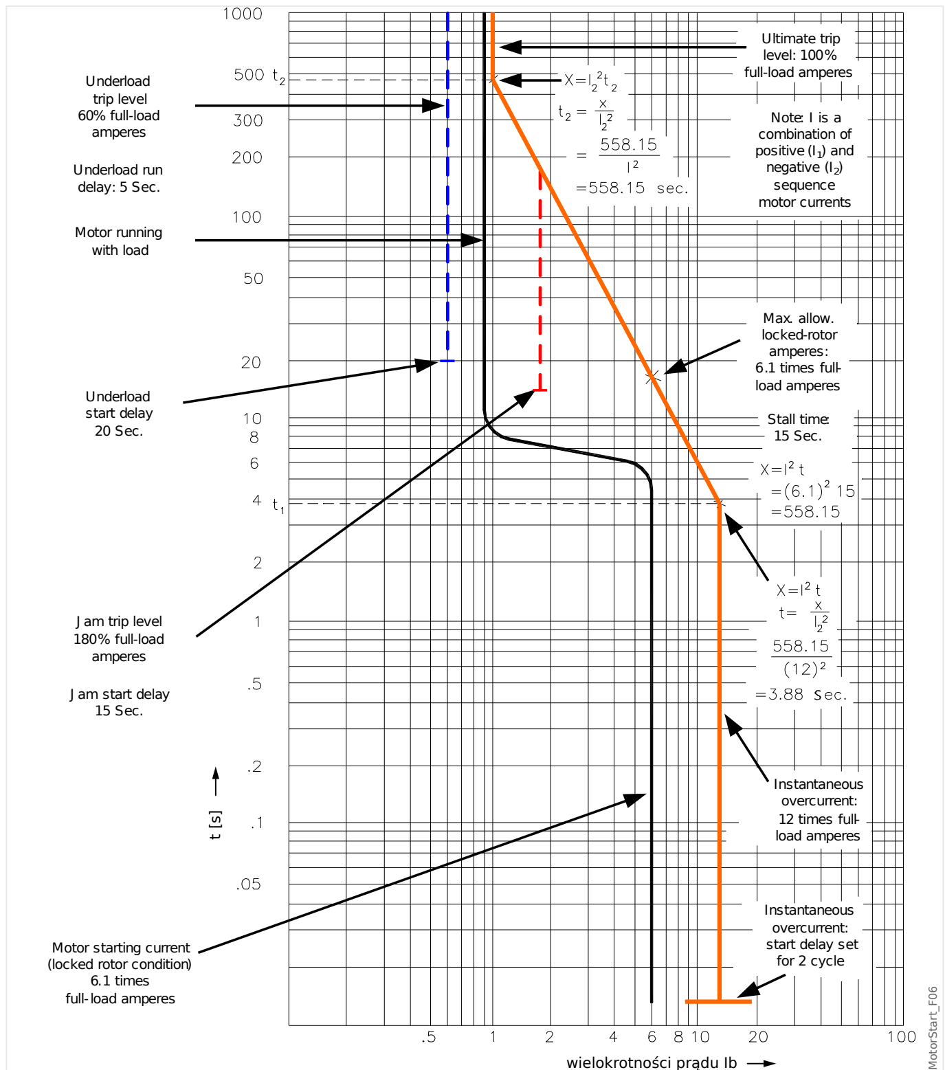
Rys. 68: Krzywa zabezpieczenia silnika (przykład 2 — bez RCT).
