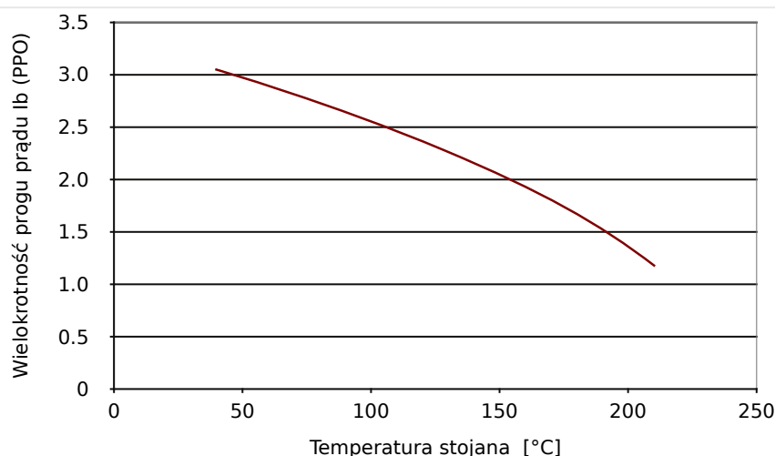
Rys. 64: Próg prądu skutecznego w stosunku do maksymalnej temperatury stojana.
