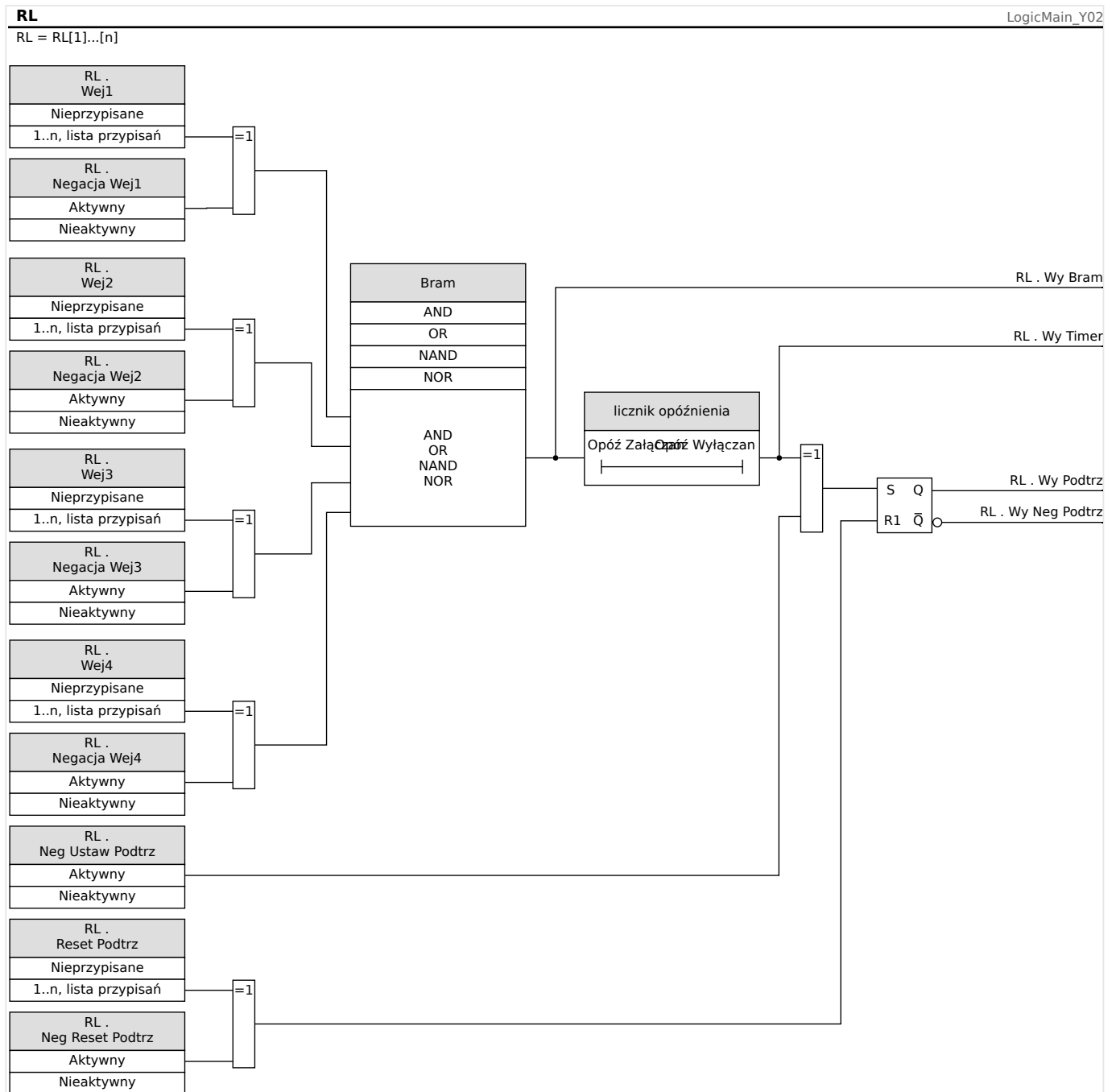
Rys. 103: Przegląd szczegółowy — ogólny schemat logiczny.
