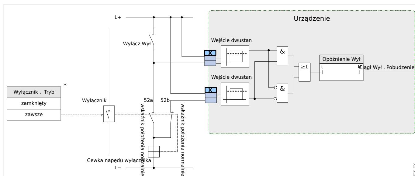
Rys. 87: Przykład okablowania: Układ kontroli ciągłości obwodów wyłącznika z dwoma stykami pomocniczymi wyłącznika „Położ ZAŁ” (52a) i „Położ WYŁ” (52b).
