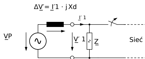
Rys. 80: Schemat zastępczy przy awarii sieci.
