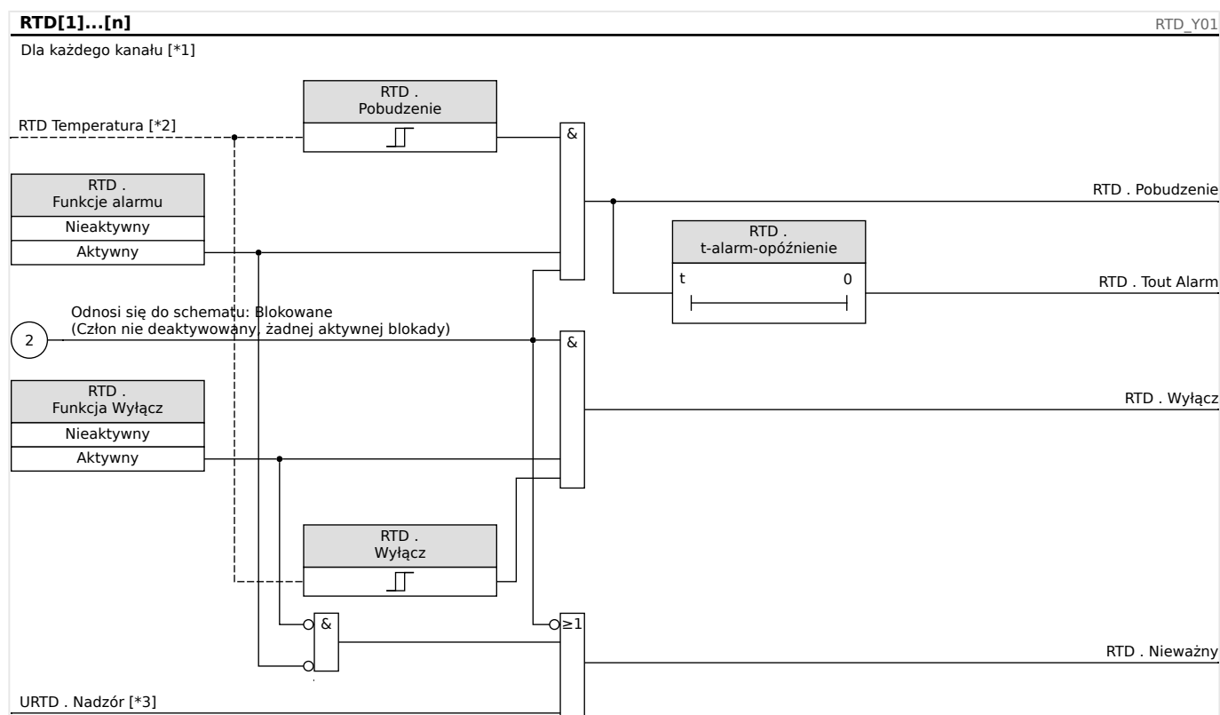
Rys. 86: Ogólna zasada działania (alarm z opóźnieniem, wyzwolenie bezzwłoczne).
