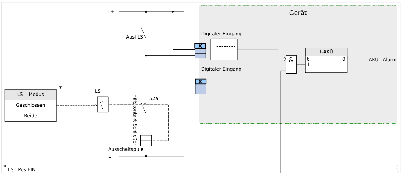
Abb. 62: Anschlussbeispiel: Auslösekreisüberwachung mit einem Hilfskontakt »Hiko EIN« (52a).
