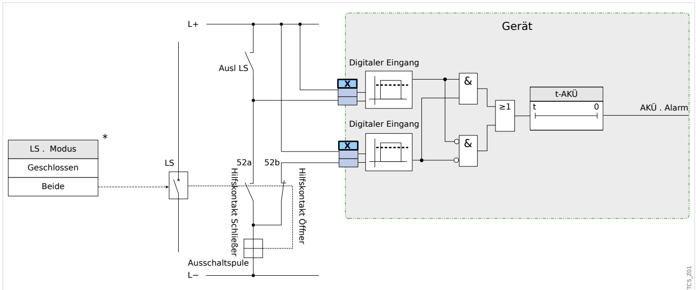
Abb. 61: Anschlussbeispiel (Empfehlung): Auslösekreisüberwachung mit zwei Hilfskontakten »Hiko EIN« (52a) und »Hiko AUS« (52b).
