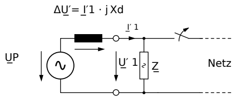
Abb. 48: Ersatzschaltbild Synchrongenerator bei Netzausfall.
