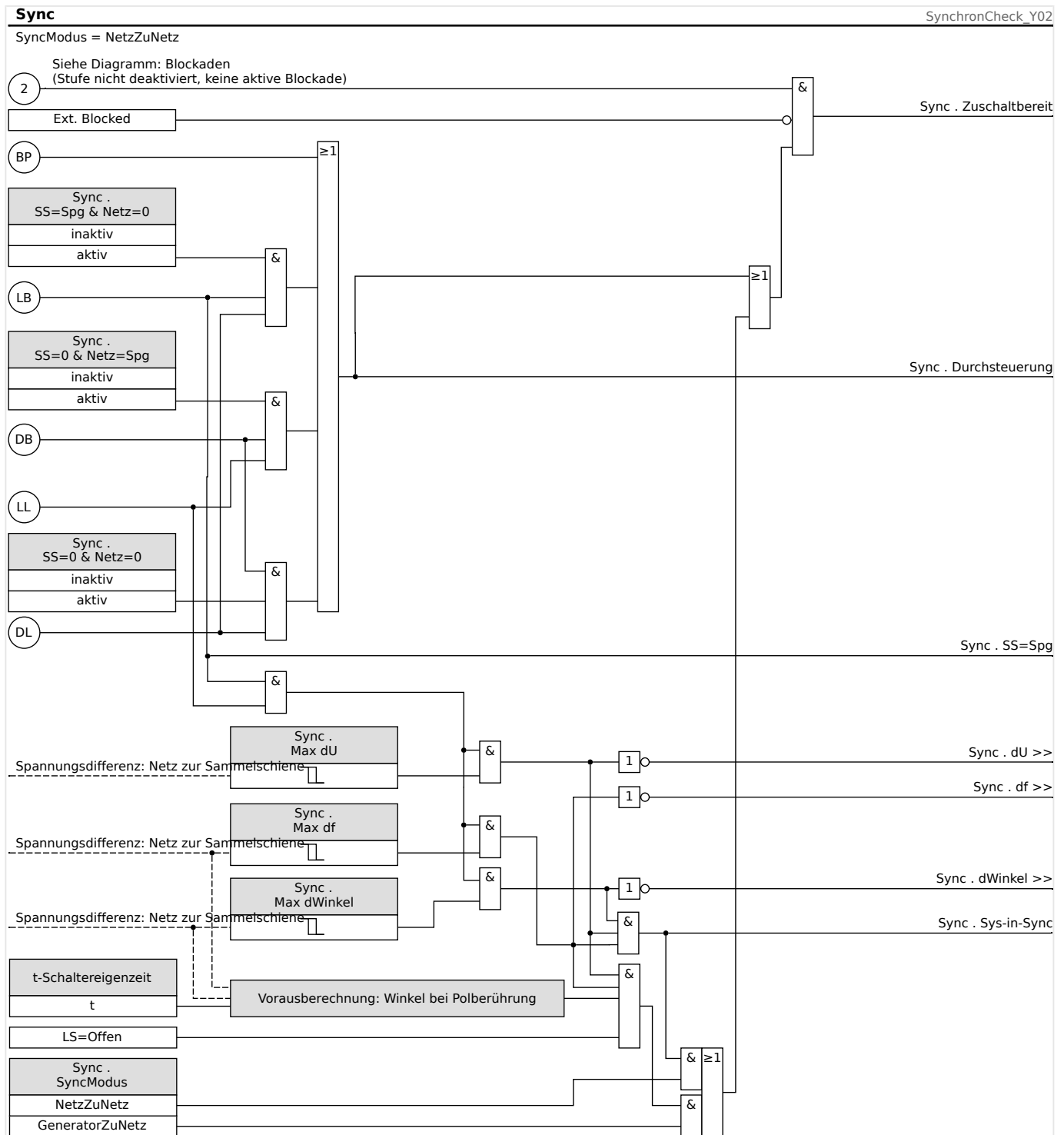
Abb. 55: Funktionalität des »Sync«-Moduls, „NetzZuNetz“.
