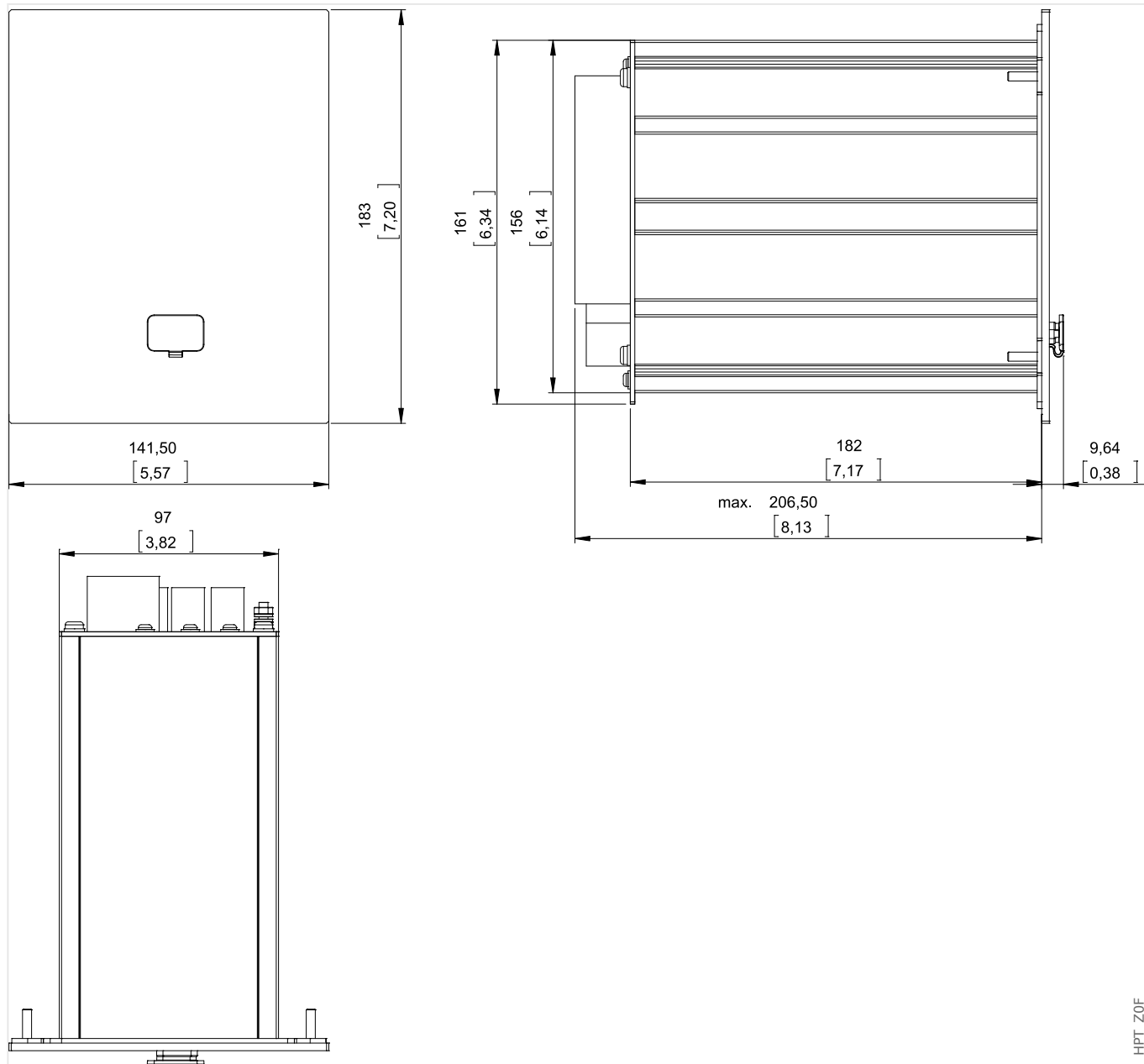
Abb. 5: 3-Seiten-Ansicht B1-Gehäuse. (Alle Angaben in mm, Maße in eckigen Klammern in Zoll.)
