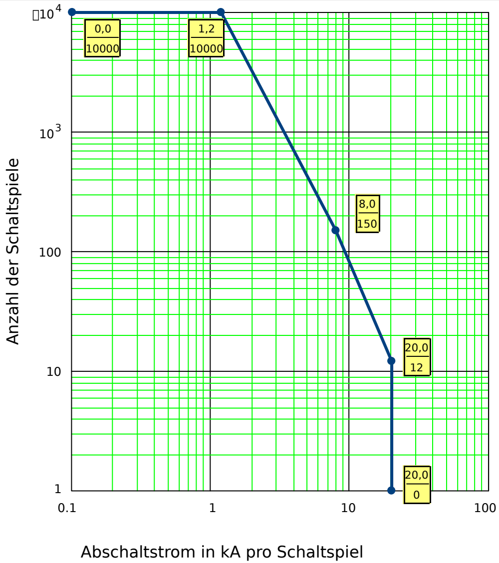
Abb. 69: Wartungskurve für einen typischen 25 kV Leistungsschalter
