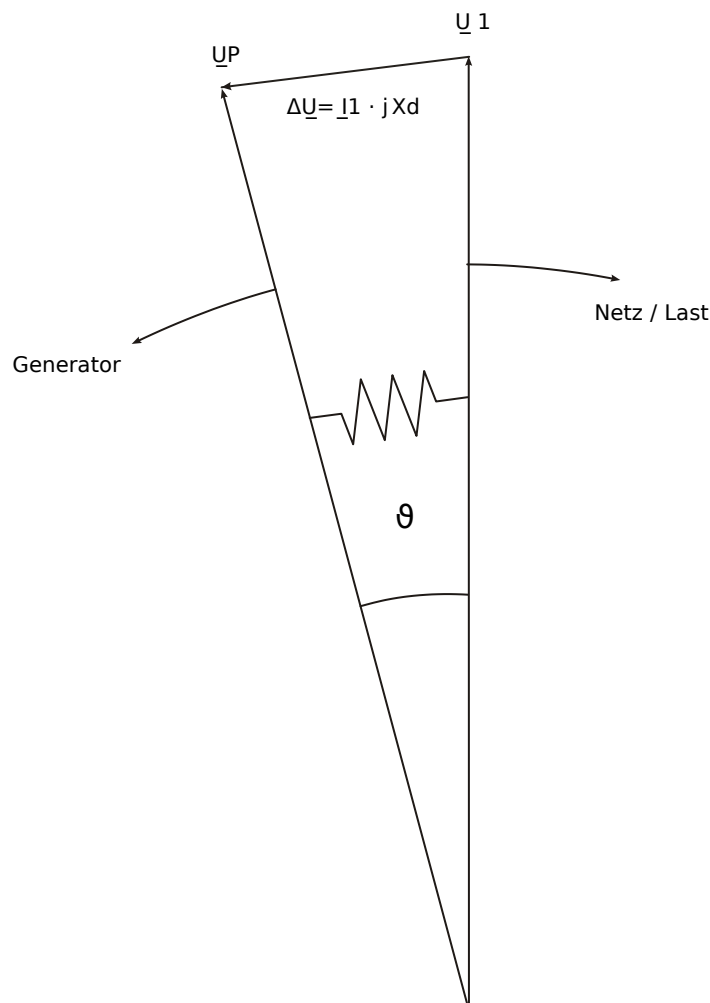
Abb. 47: Polradwinkel bei konstanter Belastung des Generators.
