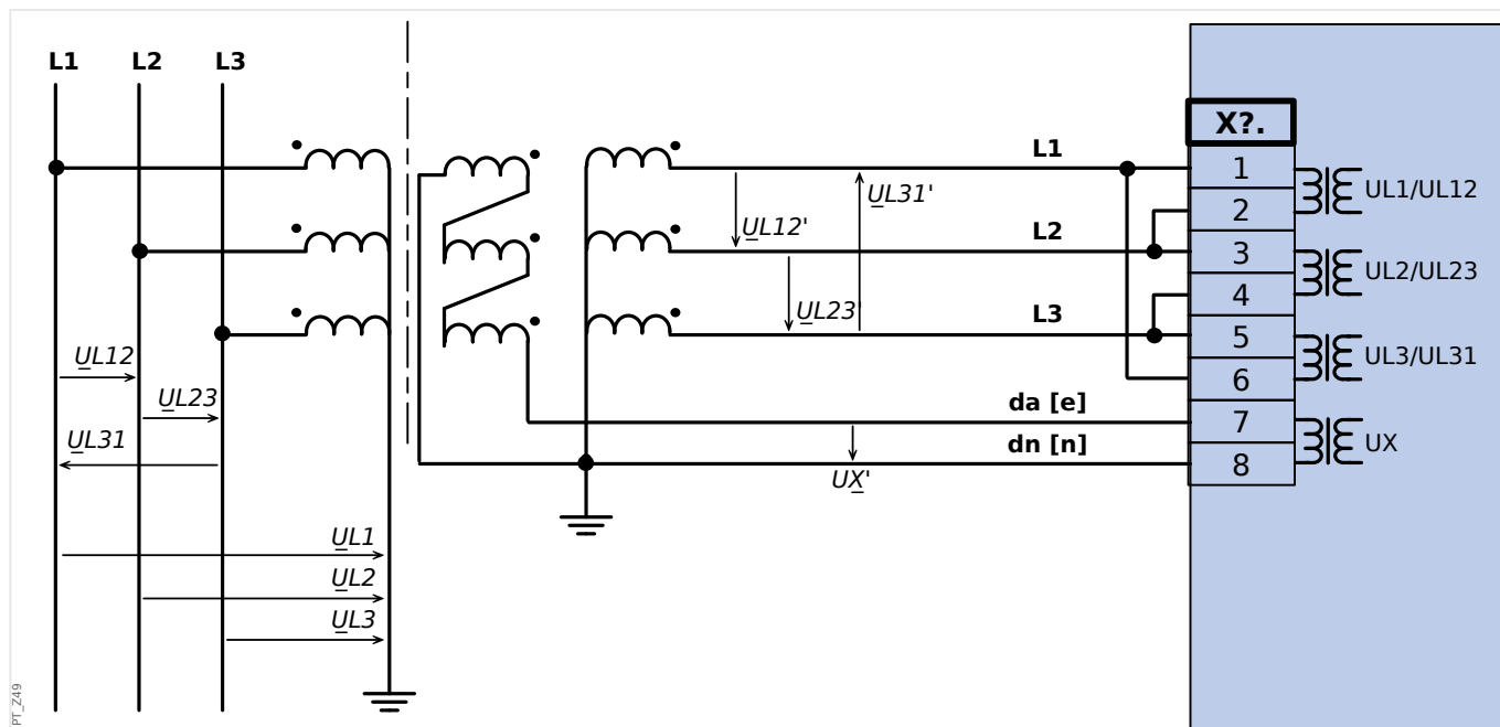
Abb. 20: Drei Spannungswandler mit Geräteanschluss in Dreieckschaltung Erfassung der Verlagerungsspannung U_E mit offener Dreieckswicklung e-n
