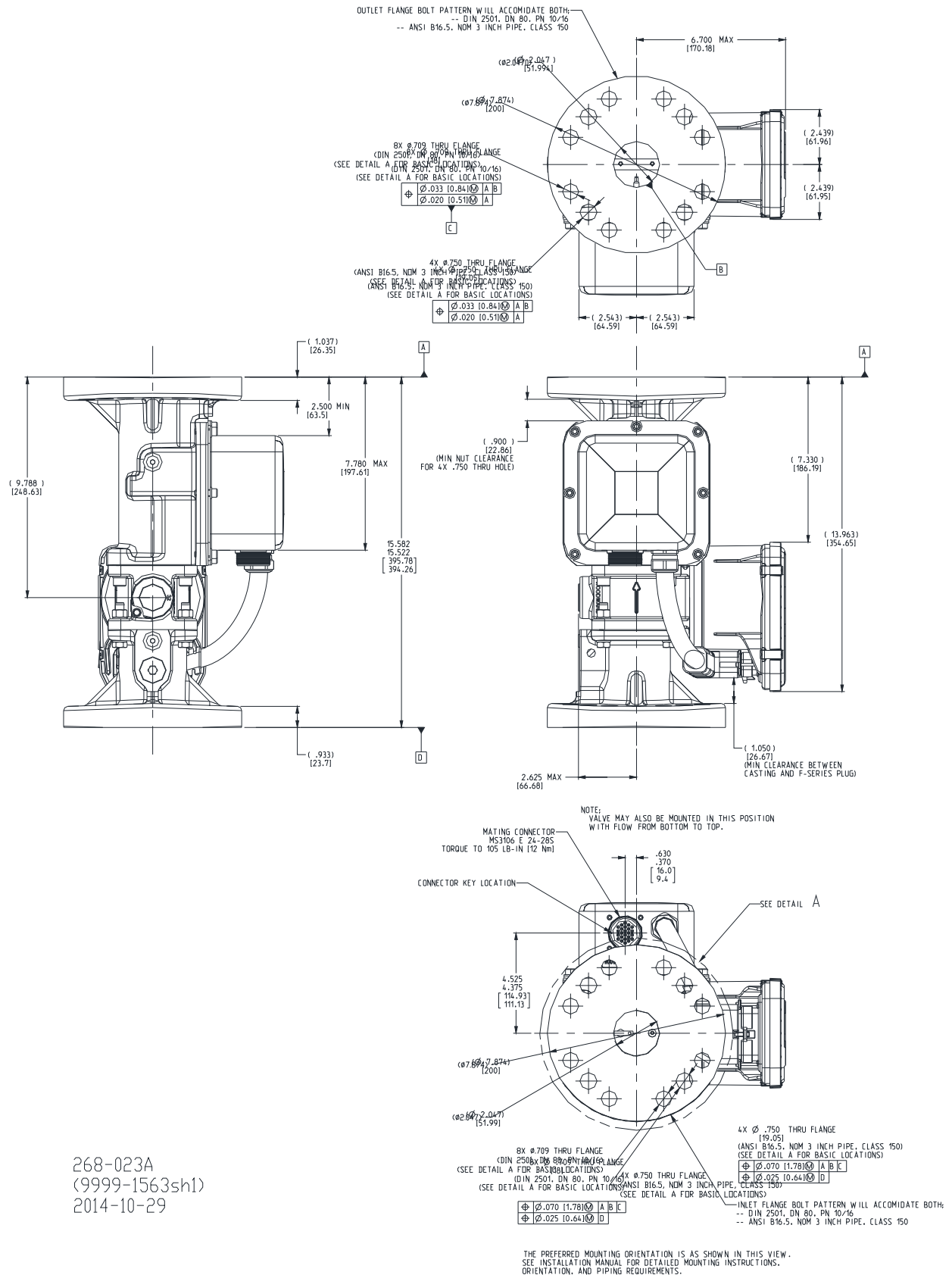
Диаграмма 1-1а. Контурный чертеж TecJet 52
